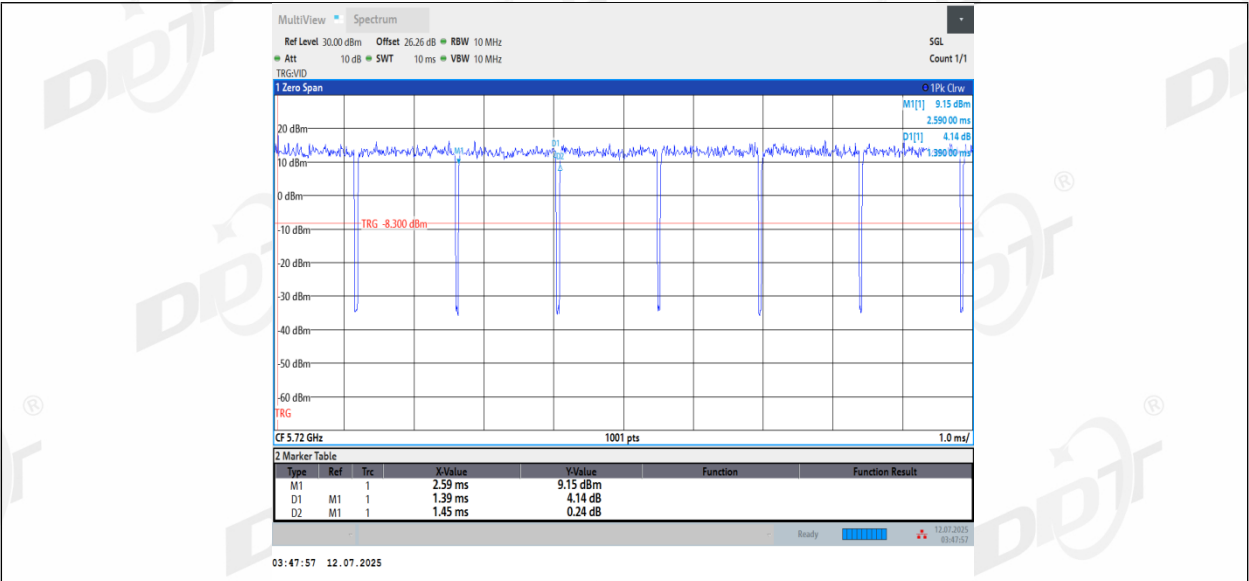
11A-CDD_Ant2_5720
