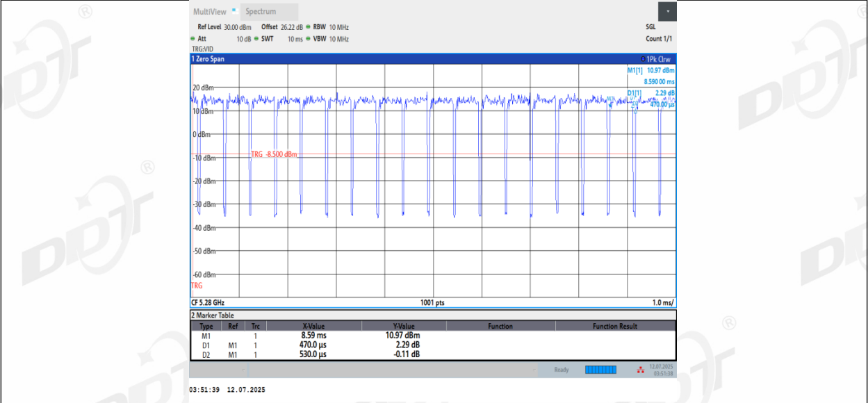
11N20MIMO_Ant3_5280
