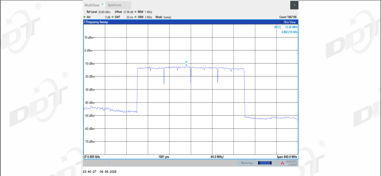
11BE320MIMO_Ant3_6905
