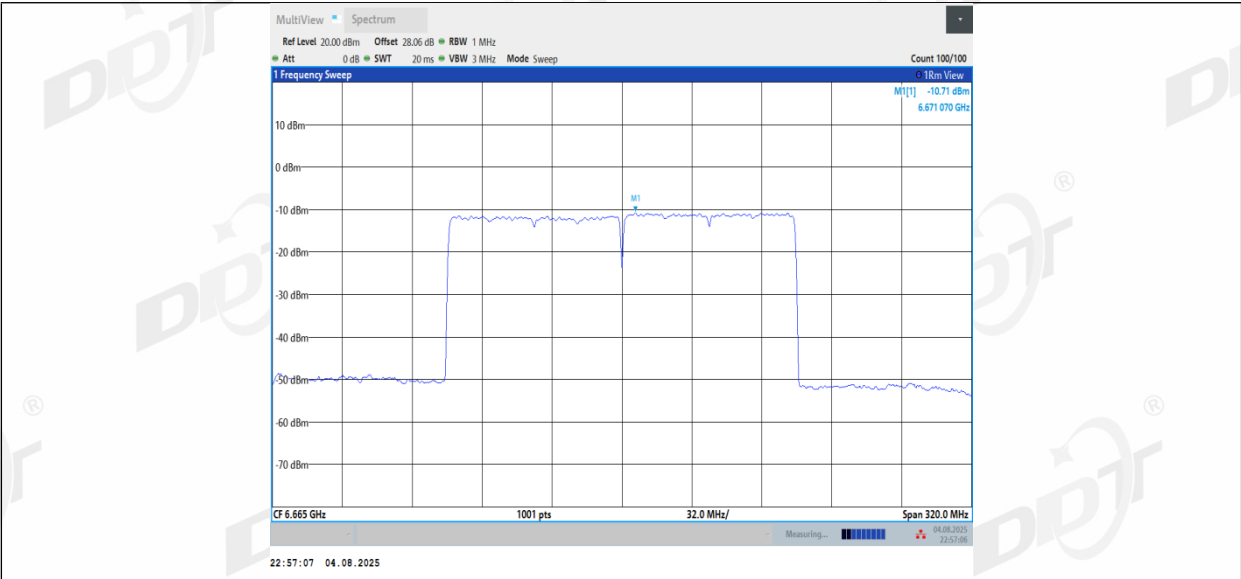
11BE160MIMO_Ant2_6665
