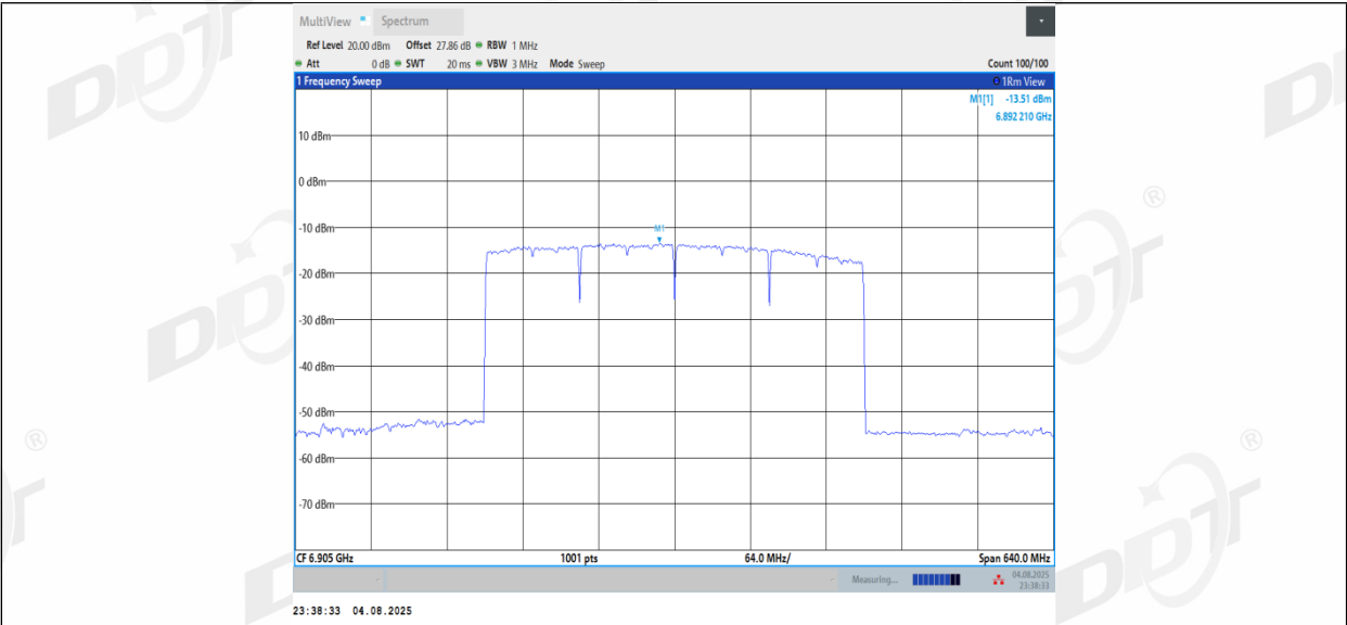
11BE320MIMO_Ant2_6905
