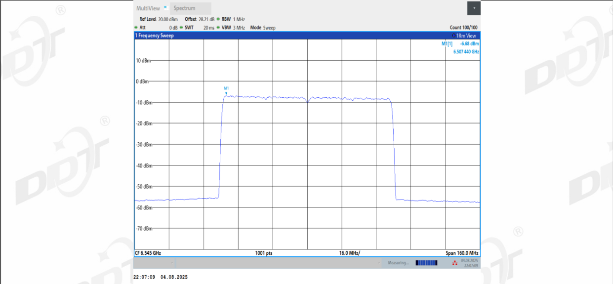
11BE80MIMO_Ant3_6545
