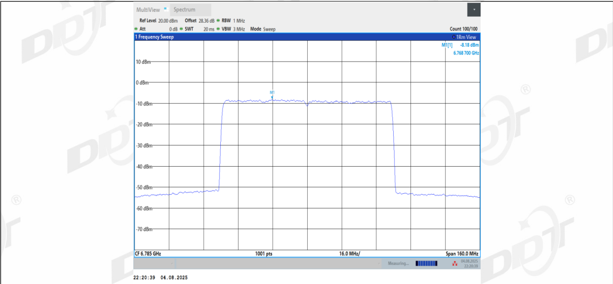
11BE80MIMO_Ant2_6785
