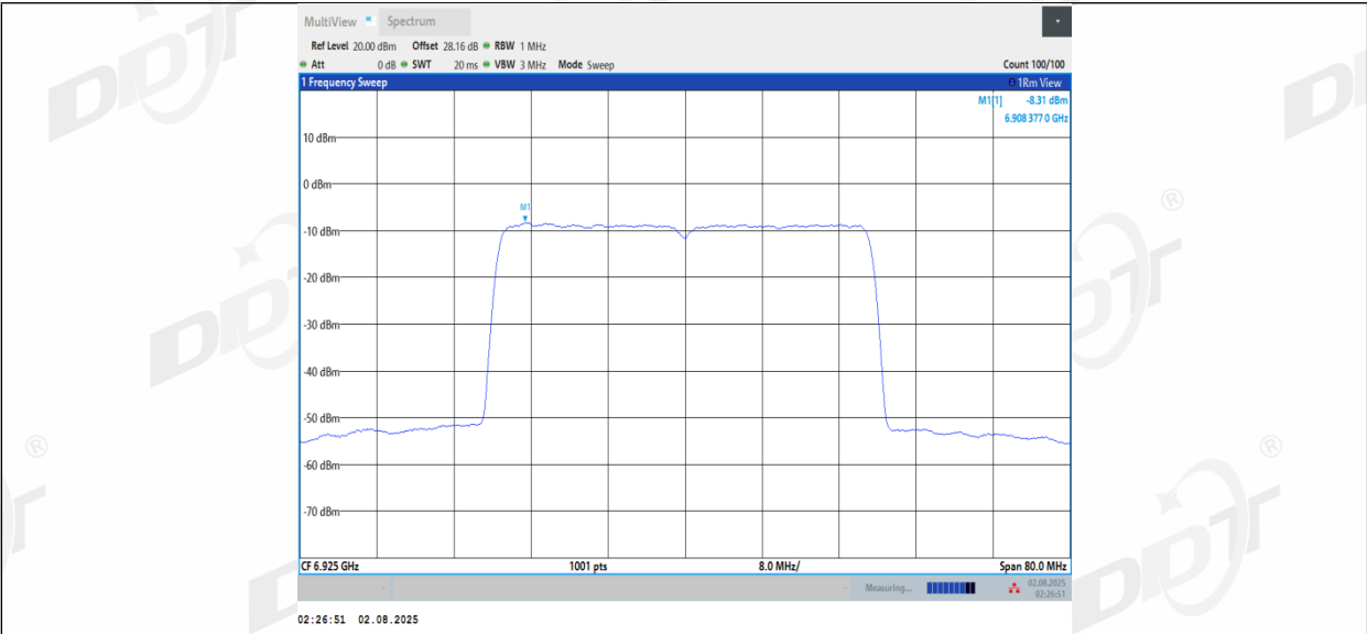
11BE40MIMO_Ant2_6925
