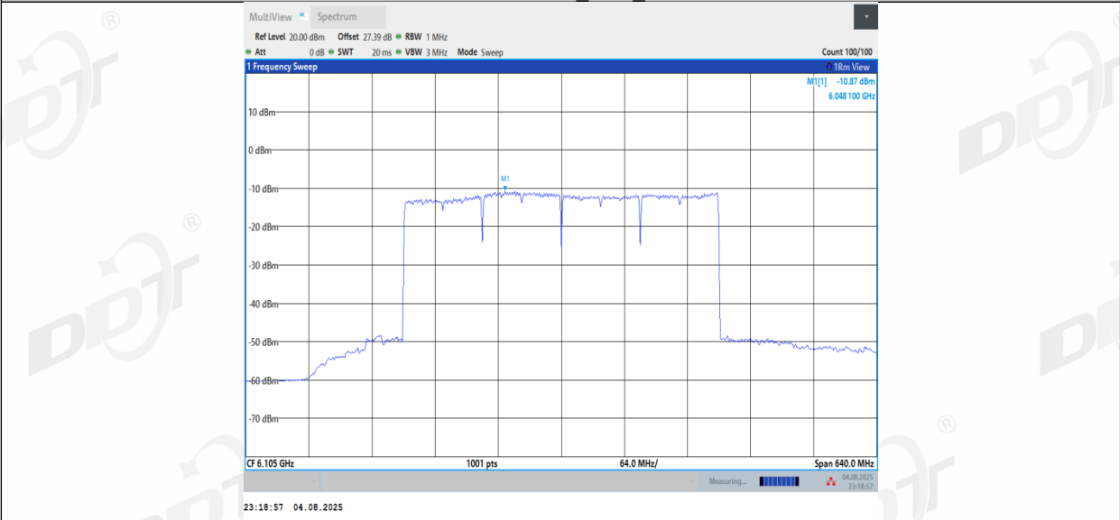
11BE320MIMO_Ant3_6105
