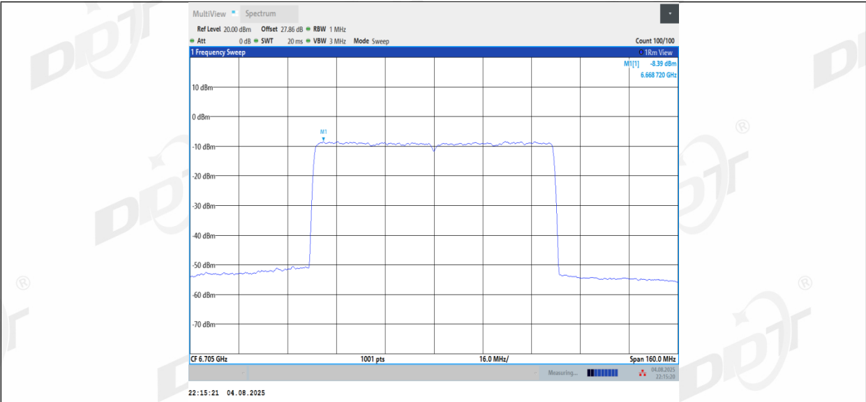
11BE80MIMO_Ant2_6705
