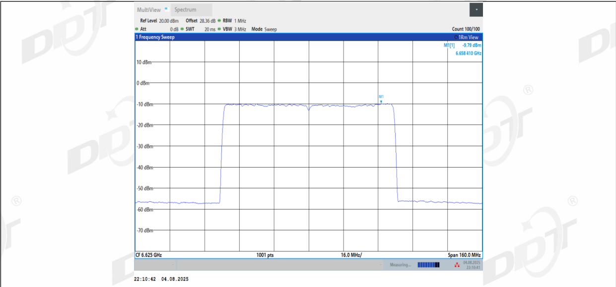
11BE80MIMO_Ant2_6625
