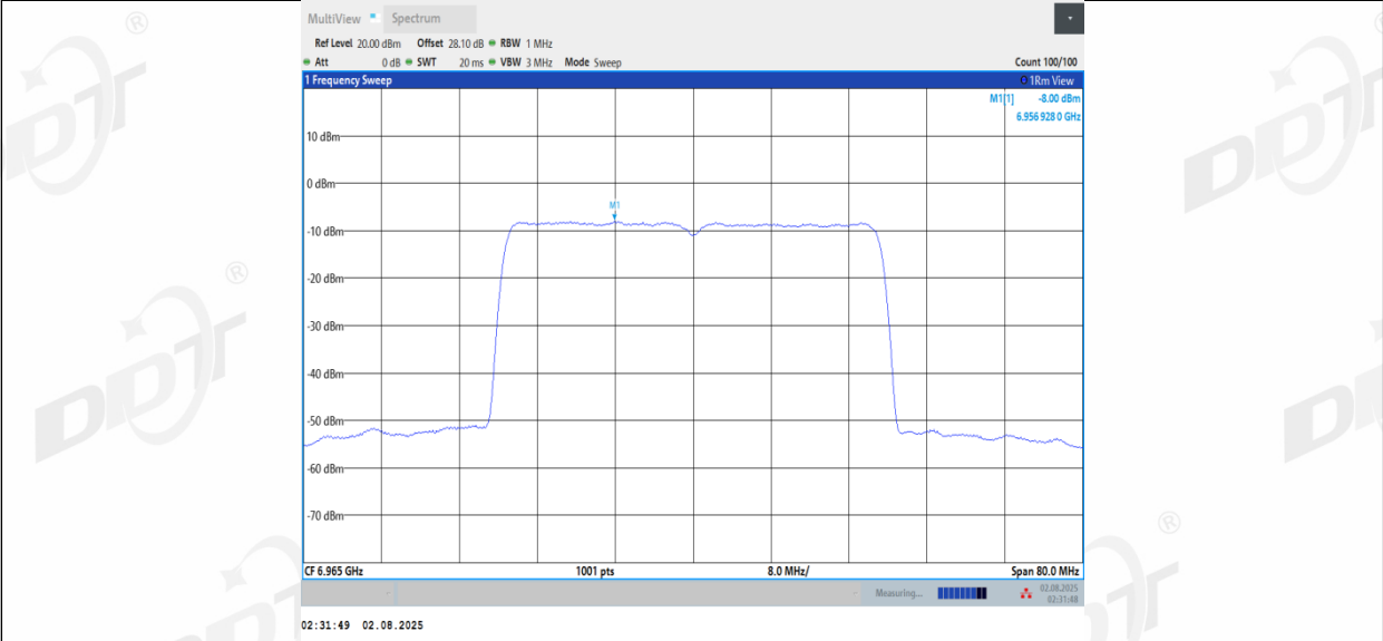
11BE40MIMO_Ant3_6965
