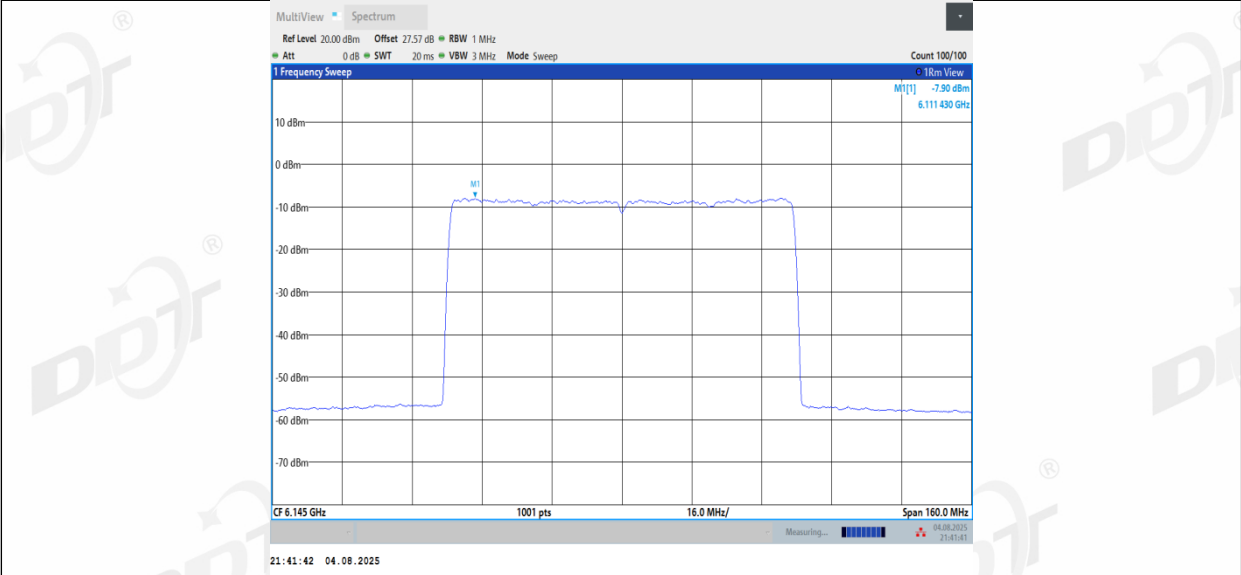
11BE80MIMO_Ant3_6145
