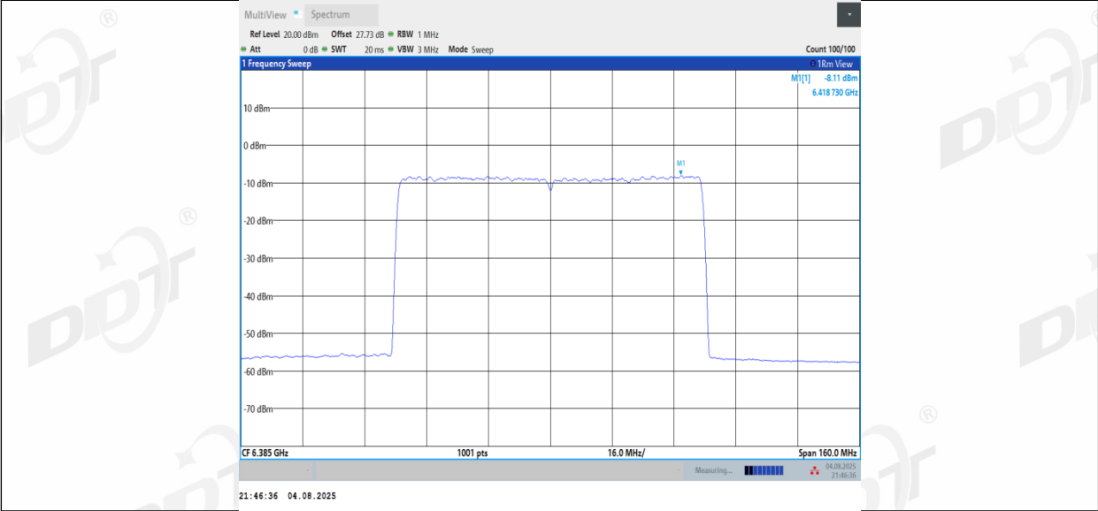
11BE80MIMO_Ant3_6385
