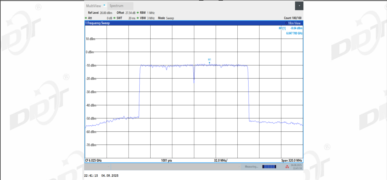
11BE160MIMO_Ant3_6025
