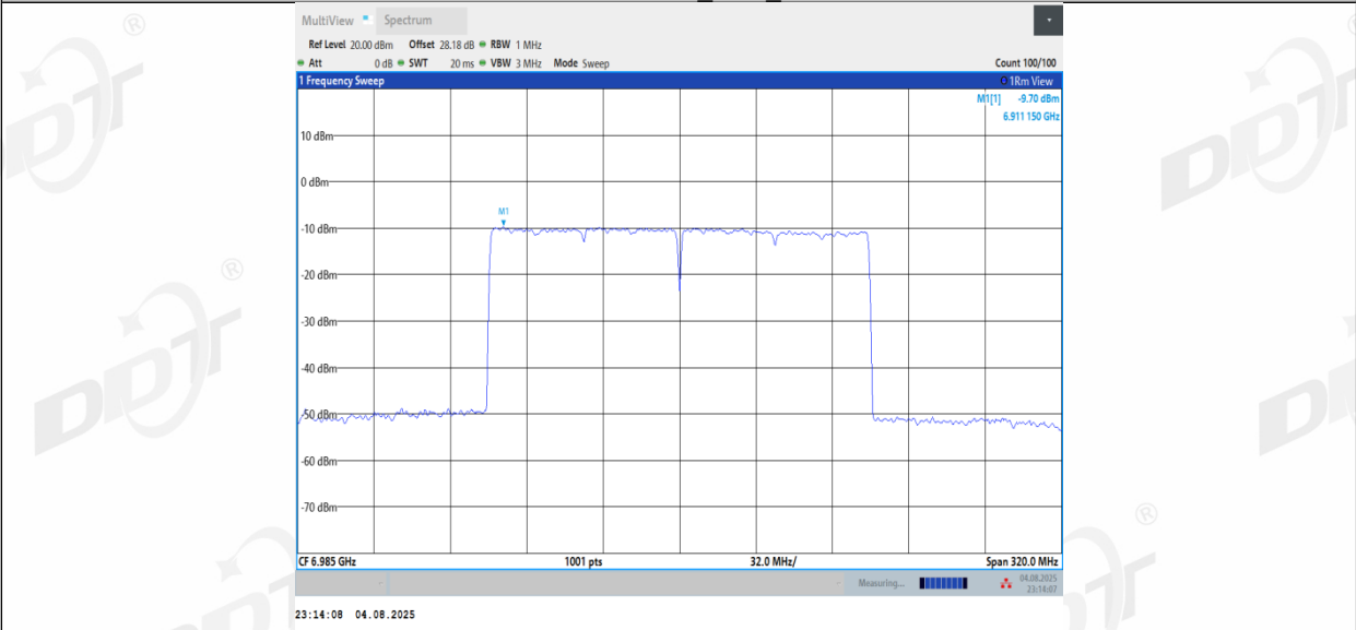
11BE160MIMO_Ant3_6985
