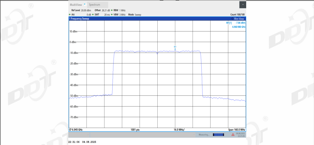
11BE80MIMO_Ant3_6945
