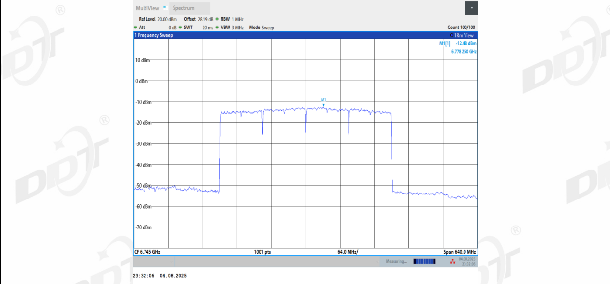
11BE320MIMO_Ant3_6745
