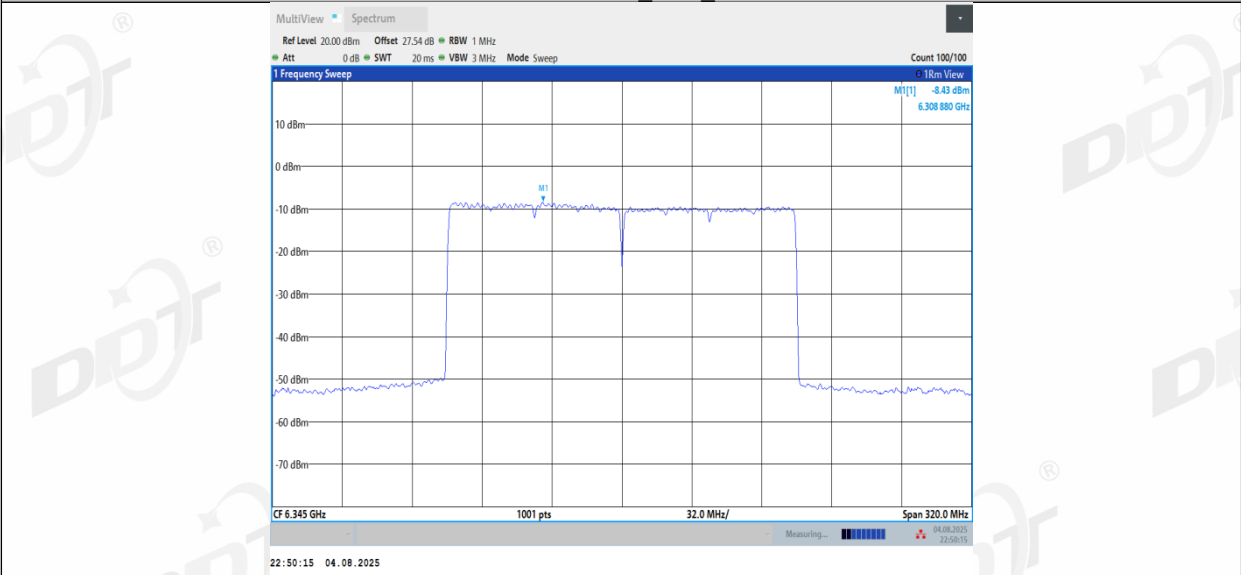
11BE160MIMO_Ant3_6345
