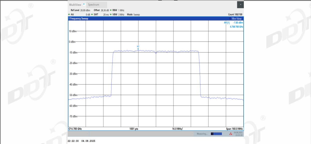
11BE80MIMO_Ant3_6785
