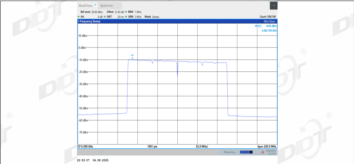
11BE160MIMO_Ant2_6505
