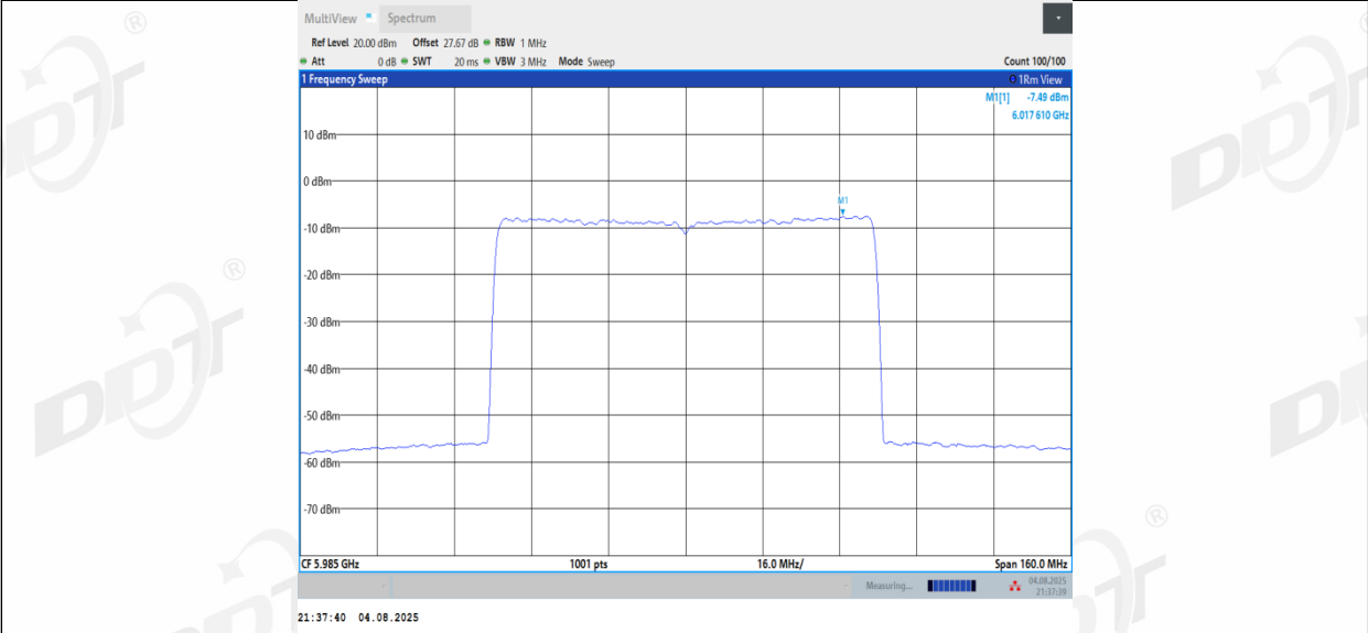
11BE80MIMO_Ant3_5985
