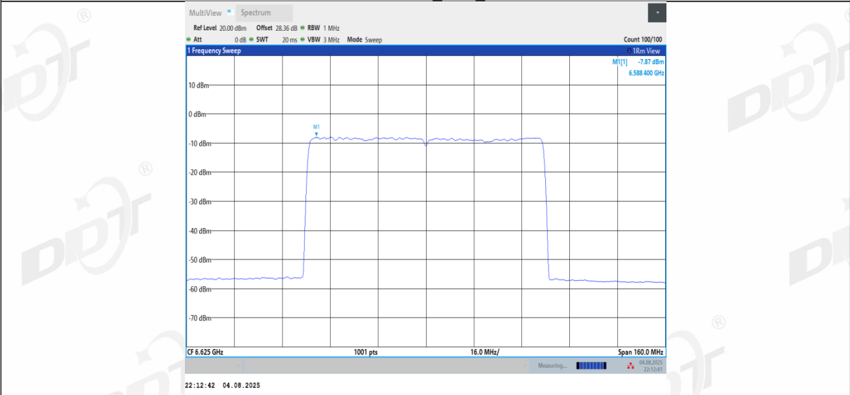
11BE80MIMO_Ant3_6625
