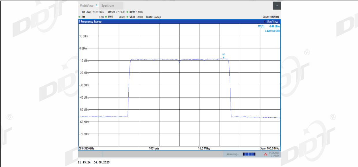
11BE80MIMO_Ant2_6385
