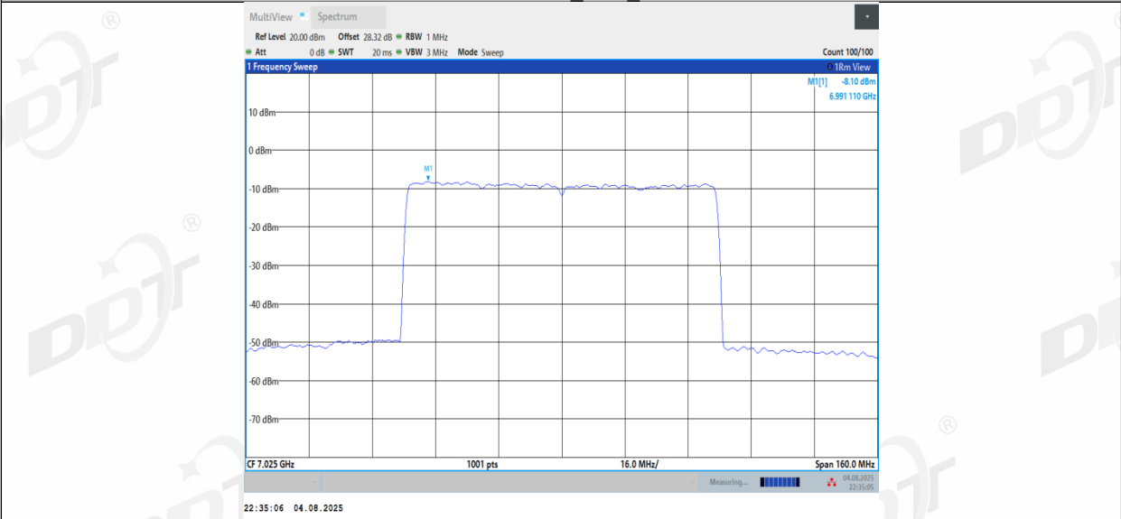
11BE80MIMO_Ant3_7025
