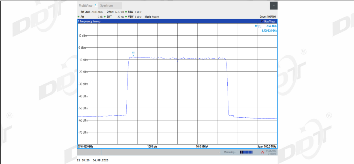
11BE80MIMO_Ant2_6465
