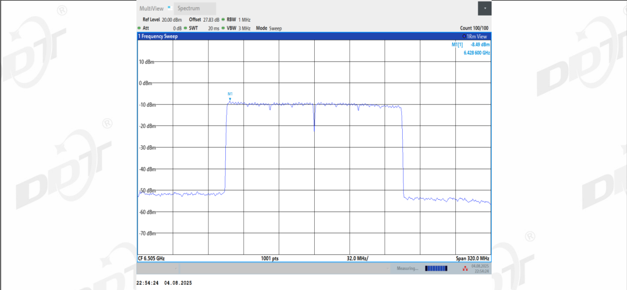
11BE160MIMO_Ant3_6505
