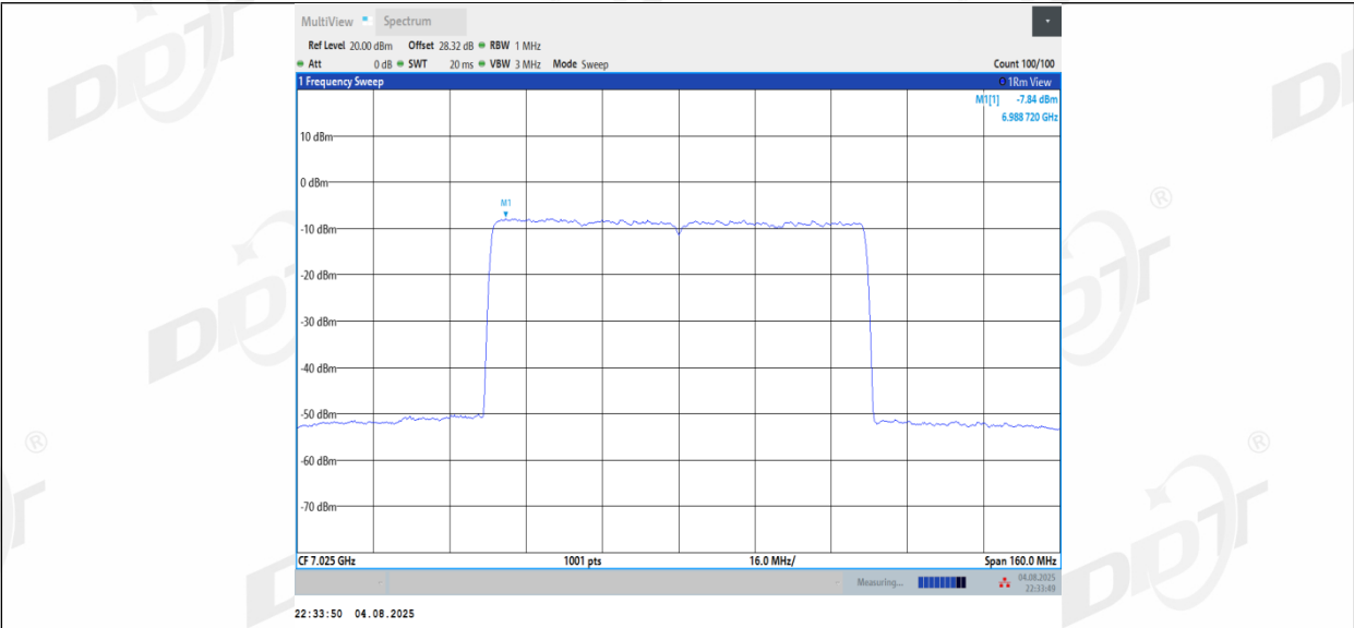
11BE80MIMO_Ant2_7025
