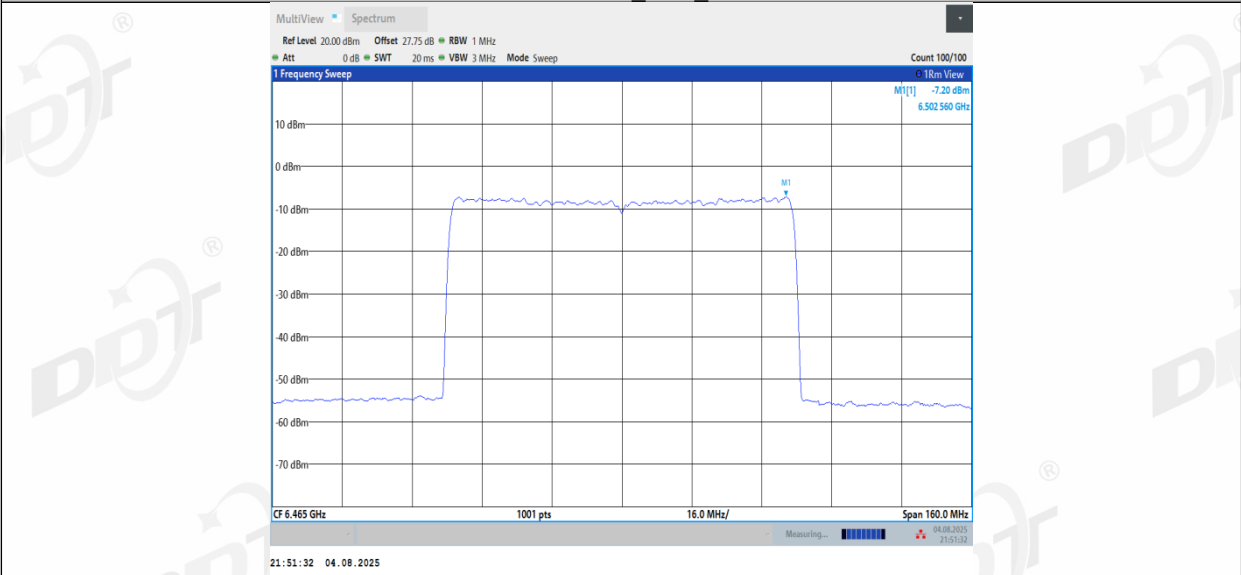
11BE80MIMO_Ant3_6465
