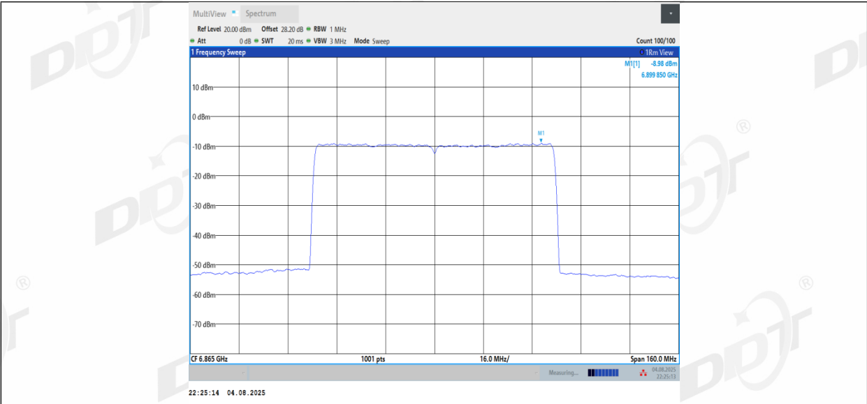
11BE80MIMO_Ant2_6865
