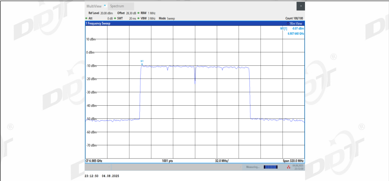
11BE160MIMO_Ant2_6985
