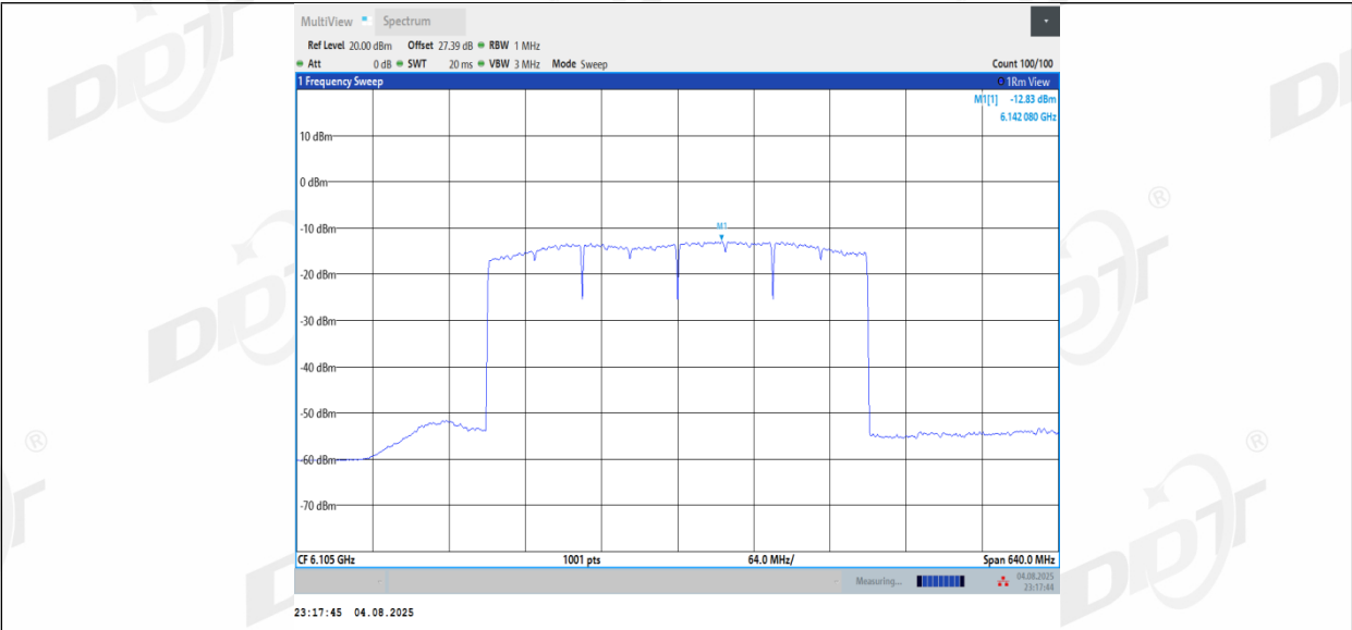
11BE320MIMO_Ant2_6105
