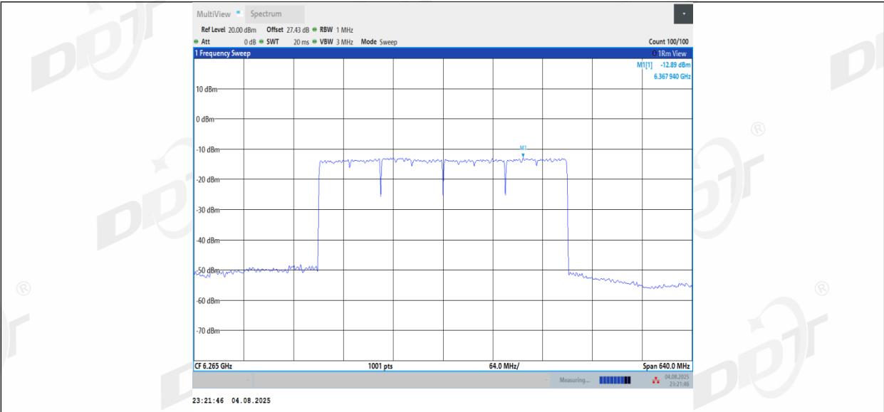
11BE320MIMO_Ant2_6265
