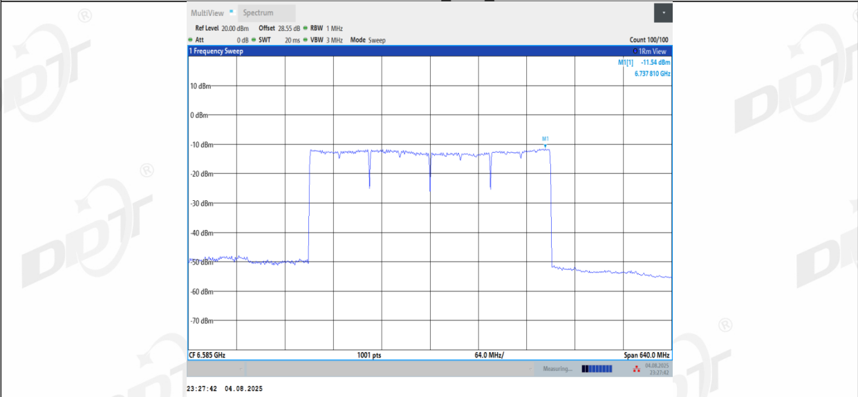
11BE320MIMO_Ant3_6585
