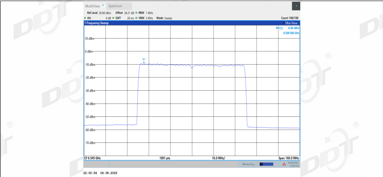
11BE80MIMO_Ant2_6545
