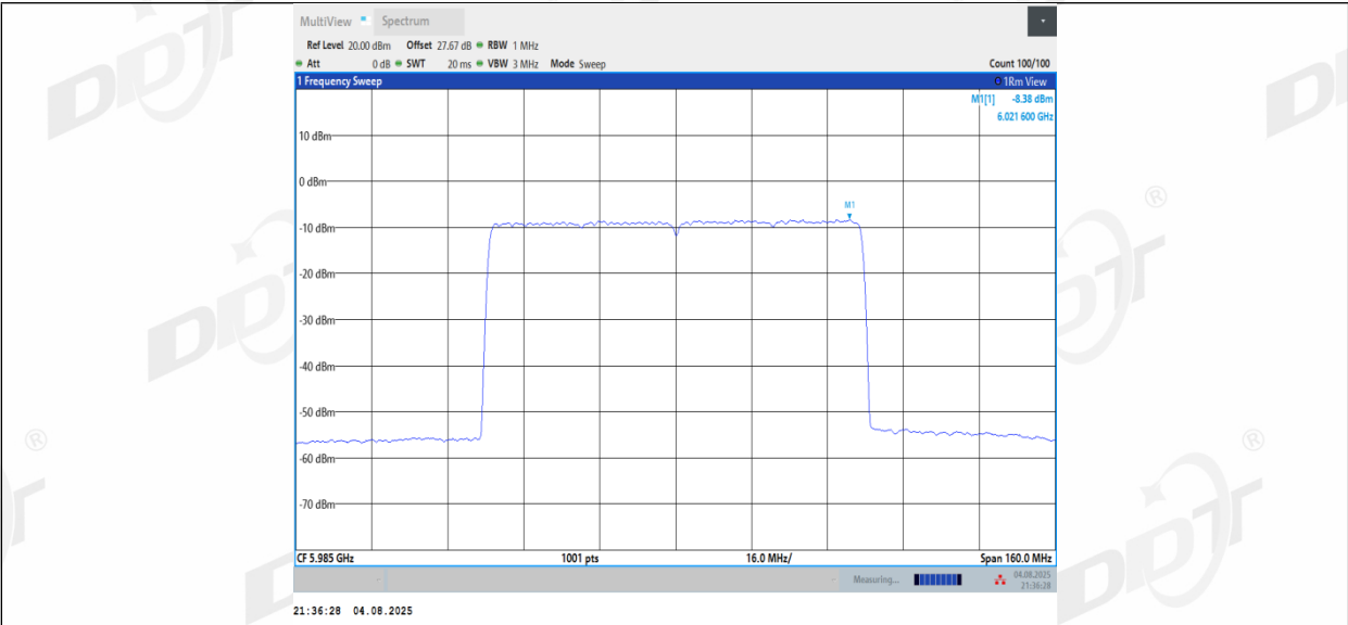
11BE80MIMO_Ant2_5985
