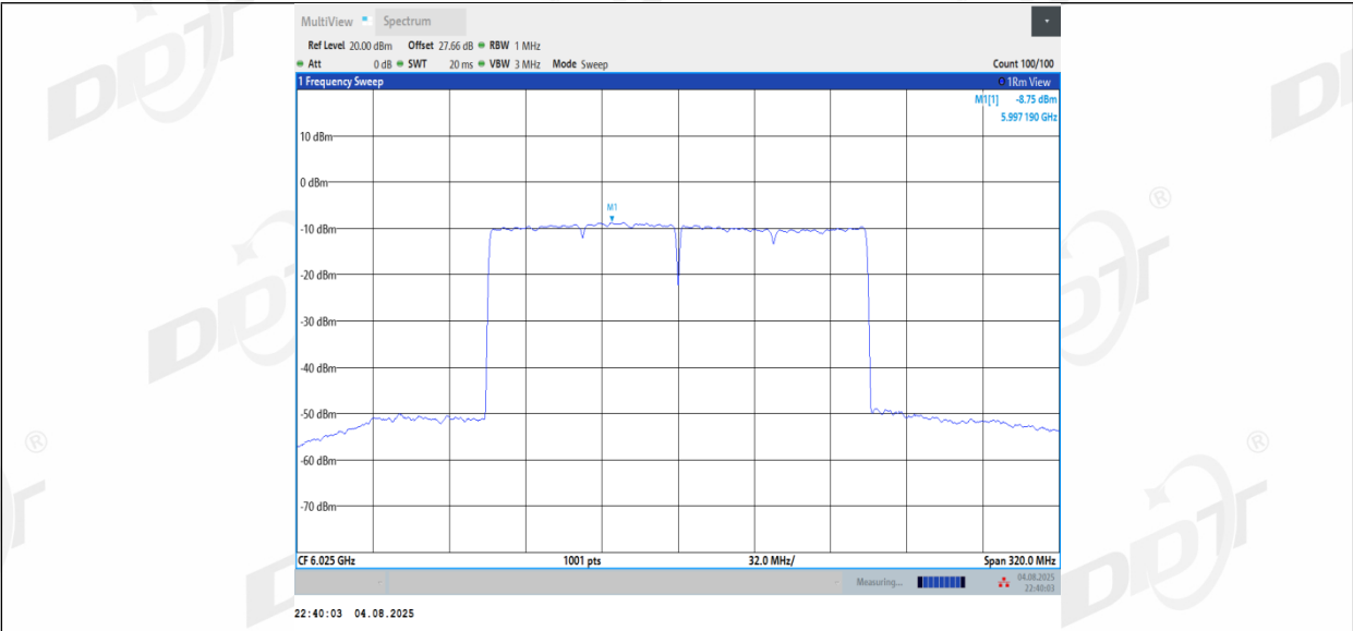
11BE160MIMO_Ant2_6025
