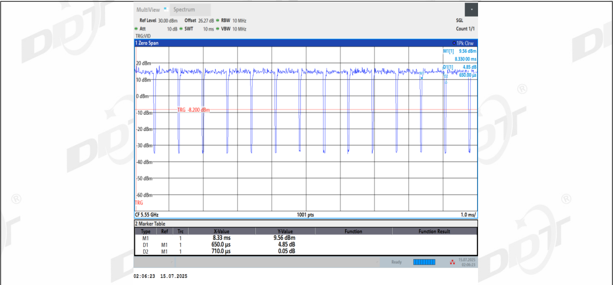
11AC40MIMO_Ant2_5550
