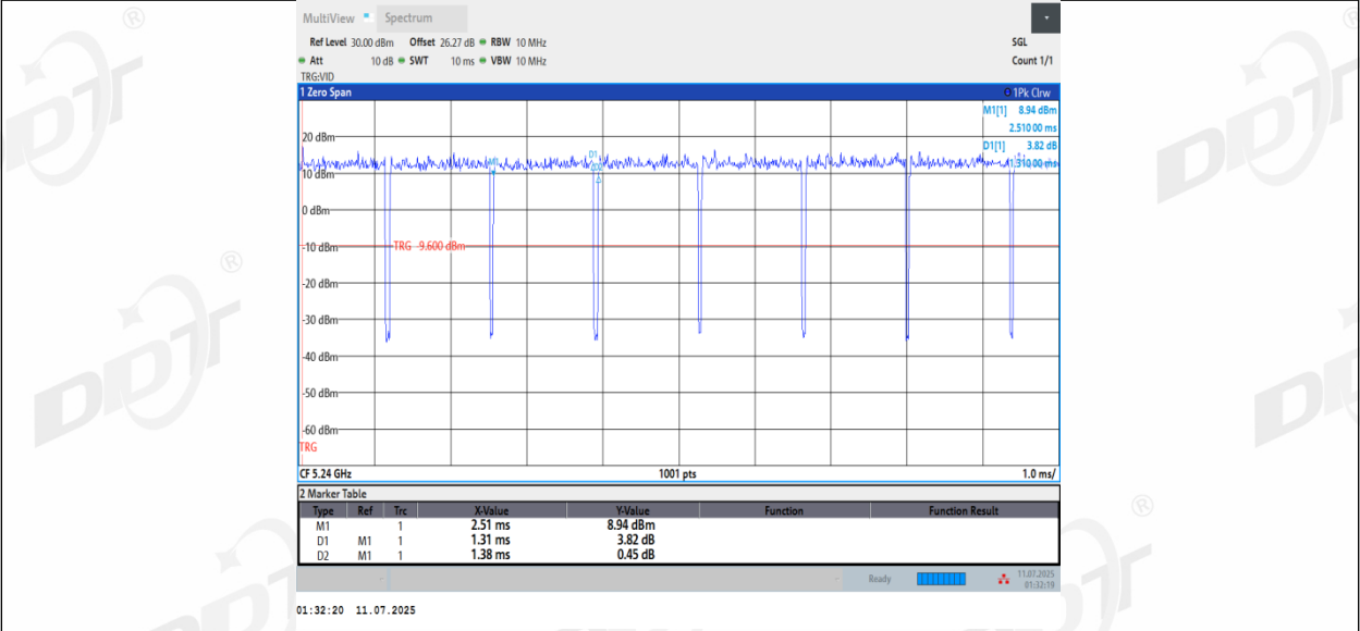
11AC20MIMO_Ant3_5240
