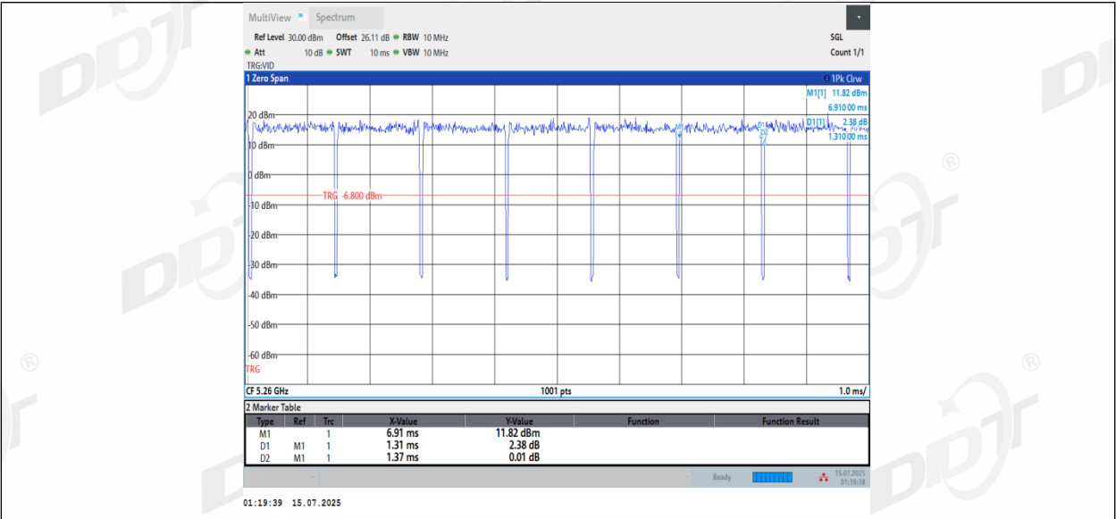
11AC20MIMO_Ant2_5260
