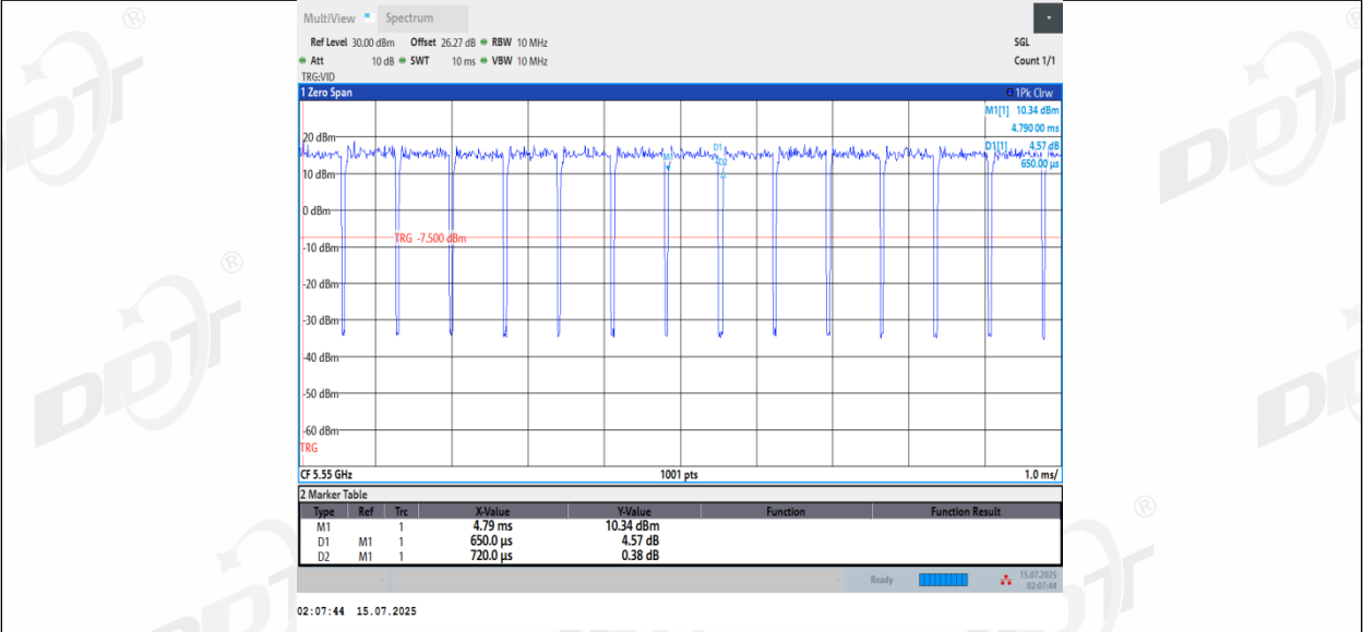
11AC40MIMO_Ant3_5550
