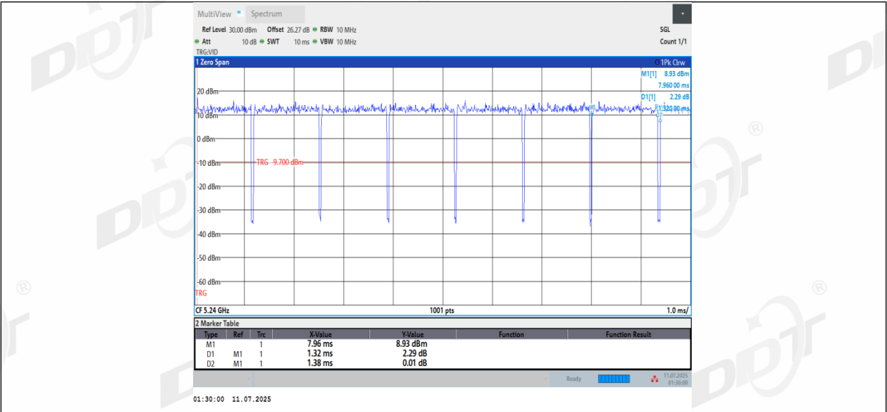
11AC20MIMO_Ant2_5240
