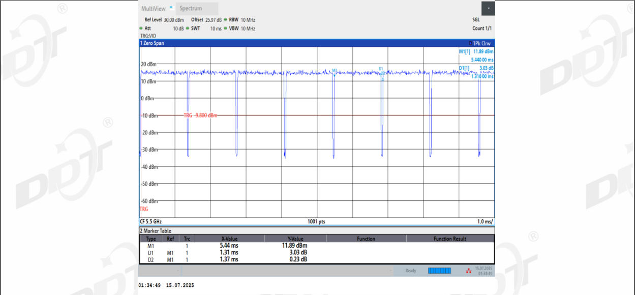
11AC20MIMO_Ant3_5500
