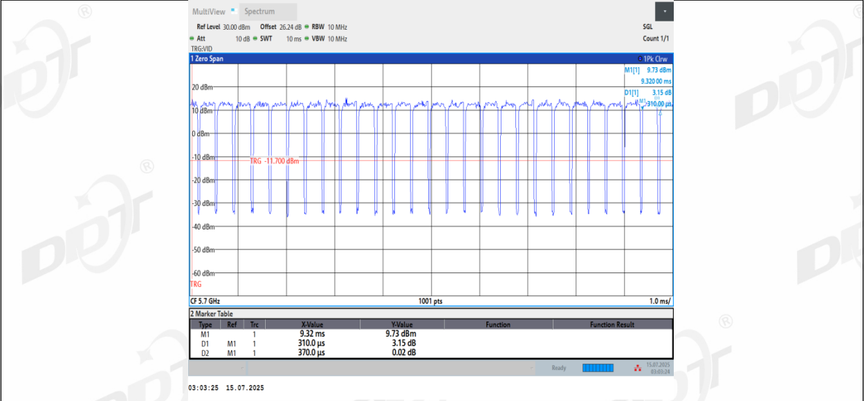
11AX20MIMO_Ant3_5700
