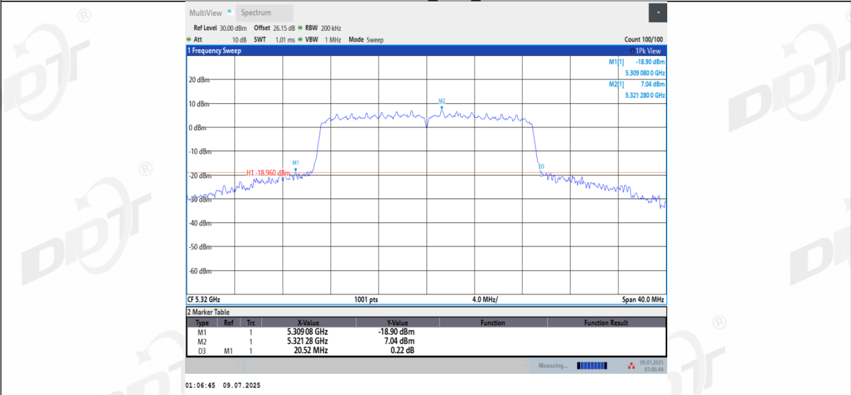
11N20MIMO_Ant3_5320
