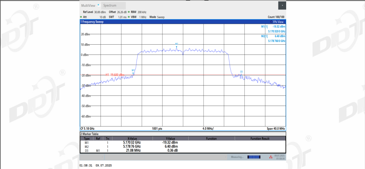
11AC20MIMO_Ant3_5180
