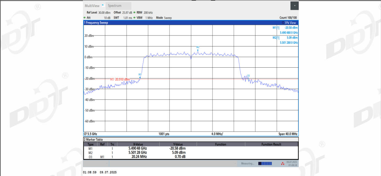
11N20MIMO_Ant3_5500
