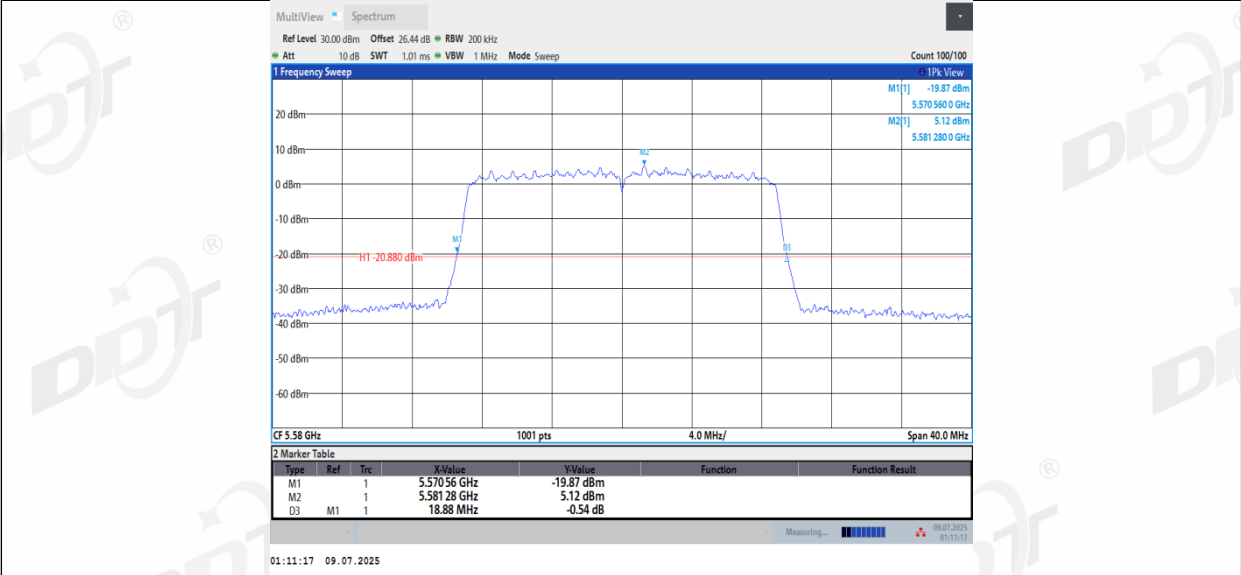
11N20MIMO_Ant3_5580
