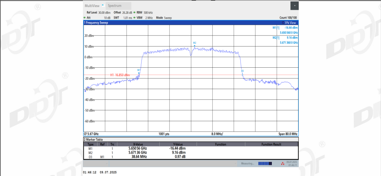
11N40MIMO_Ant3_5670
