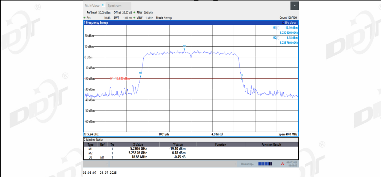
11AC20MIMO_Ant3_5240
