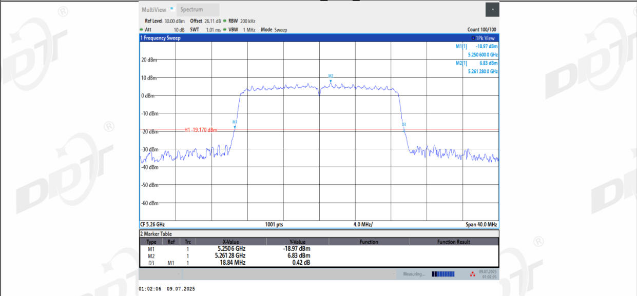
11N20MIMO_Ant3_5260
