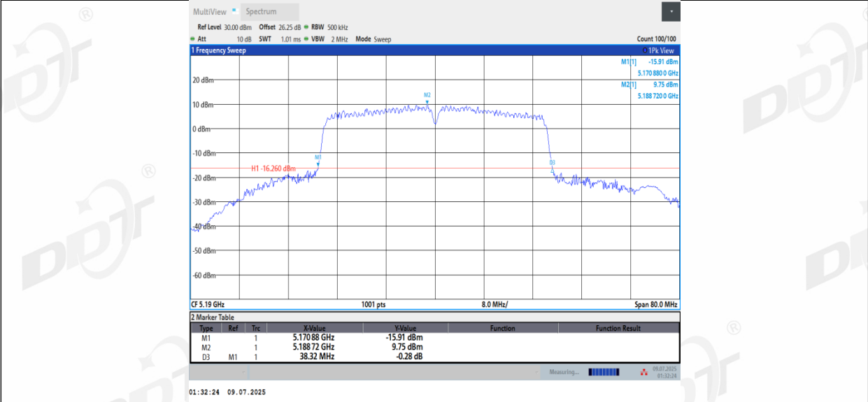
11N40MIMO_Ant3_5190
