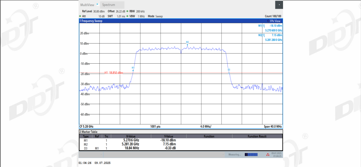
11N20MIMO_Ant3_5280
