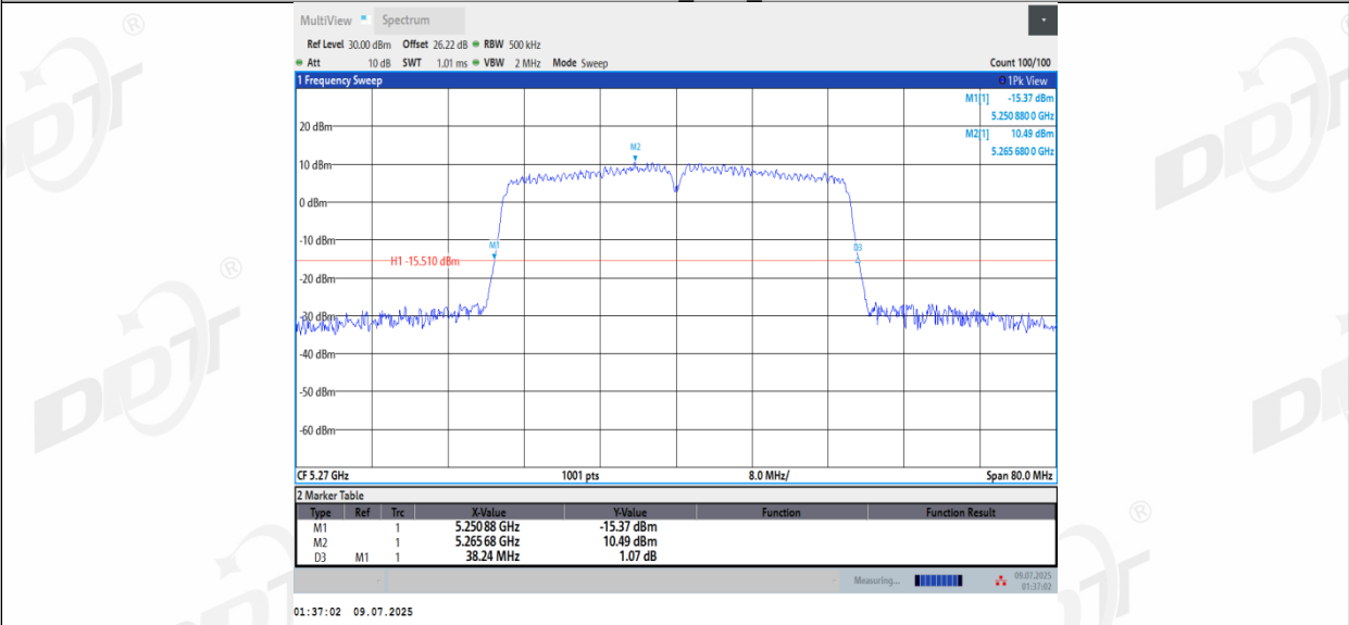
11N40MIMO_Ant3_5270
