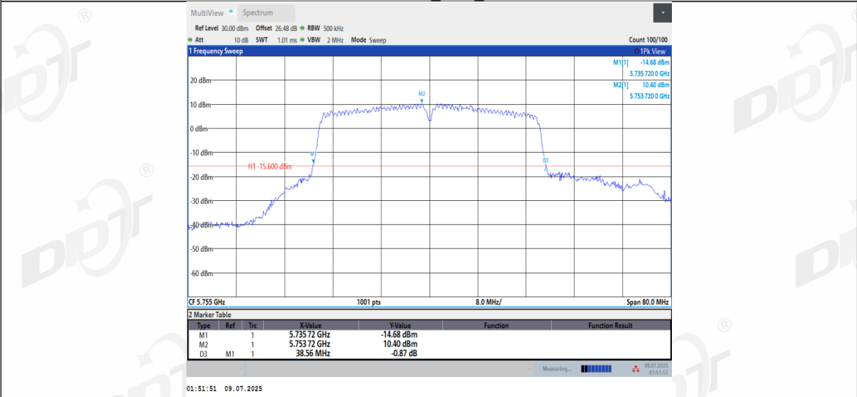
11N40MIMO_Ant3_5755
