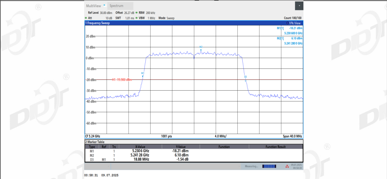
11N20MIMO_Ant3_5240
