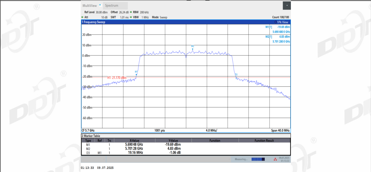
11N20MIMO_Ant3_5700
