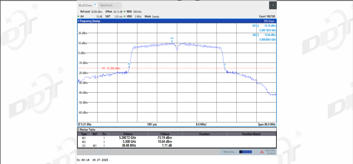
11N40MIMO_Ant3_5310
