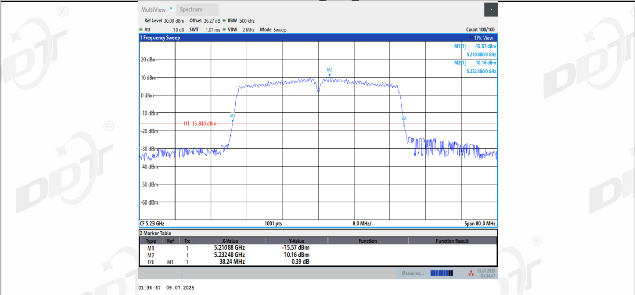
11N40MIMO_Ant3_5230
