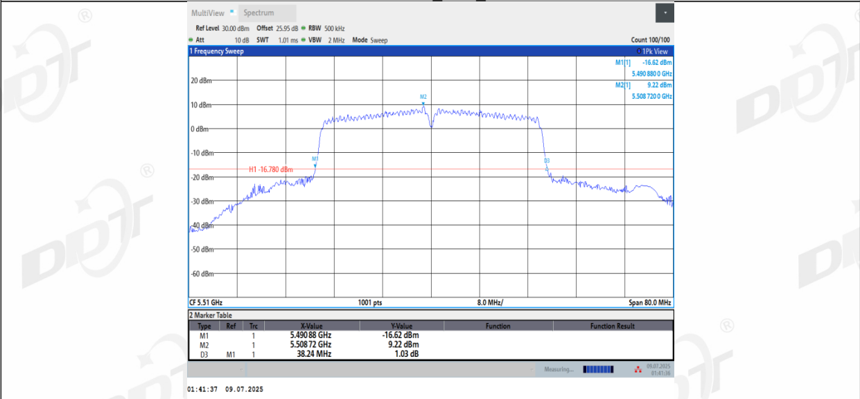
11N40MIMO_Ant3_5510
