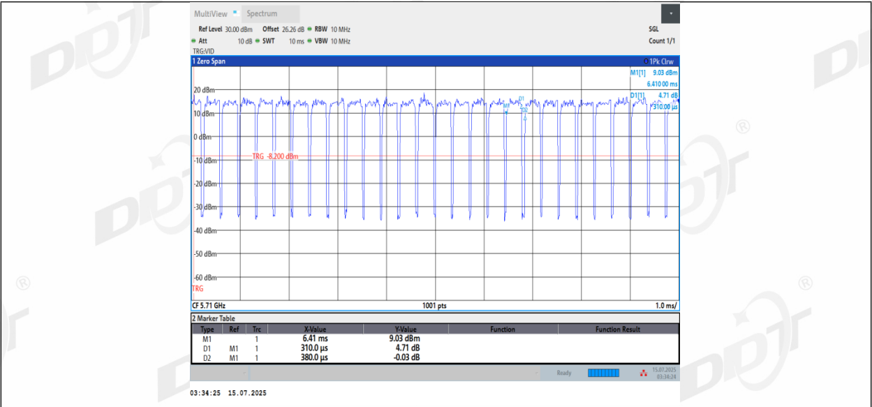
11AX40MIMO_Ant2_5710
