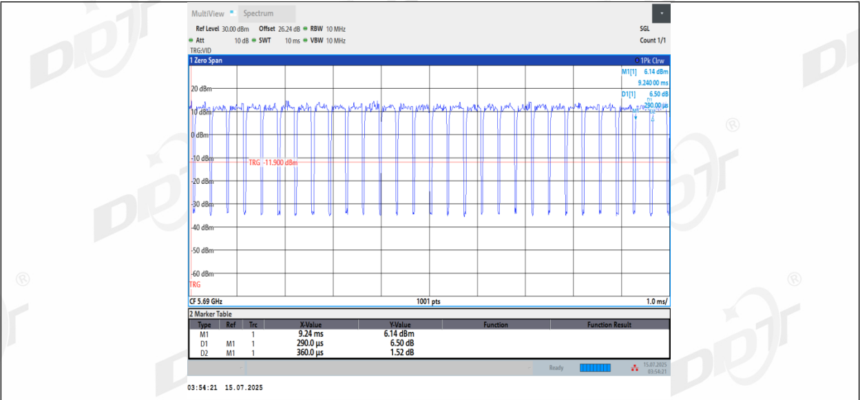
11AX80MIMO_Ant2_5690
