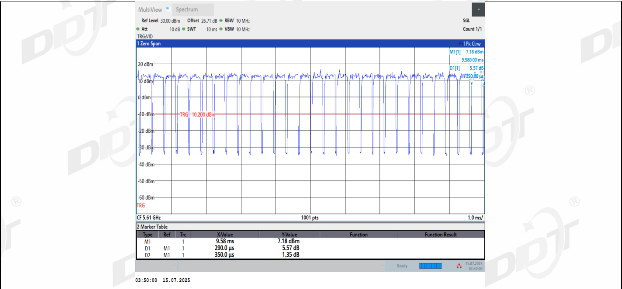
11AX80MIMO_Ant2_5610
