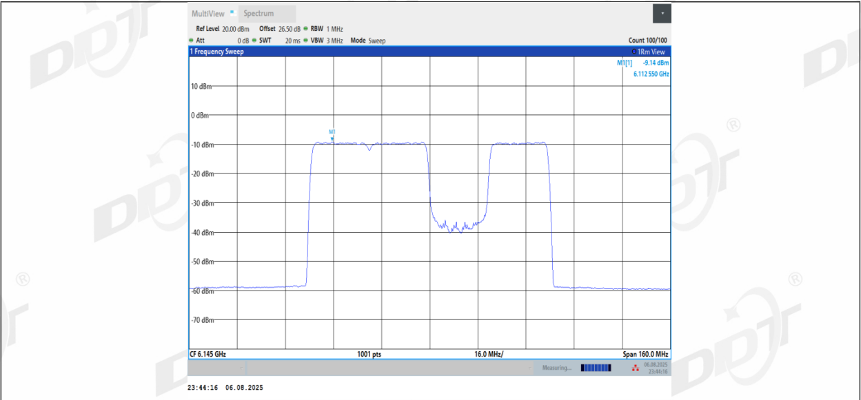
11BE80MIMO_Ant2_6145_484+242_Non-OFDMA_4
