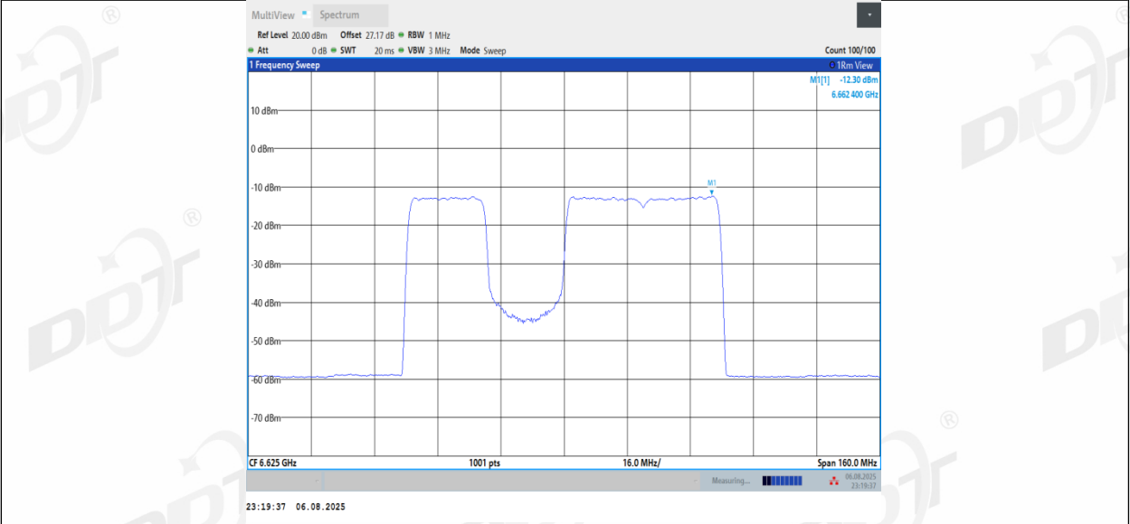
11BE80MIMO_Ant1_6625_484+242_Non-OFDMA_3
