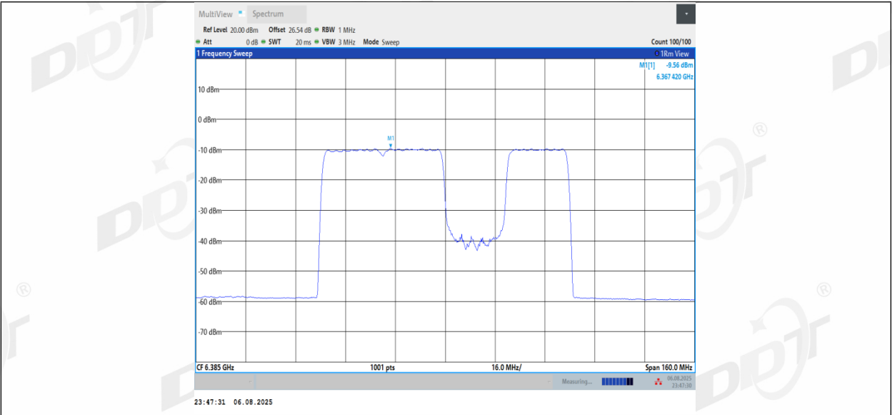
11BE80MIMO_Ant2_6385_484+242_Non-OFDMA_4
