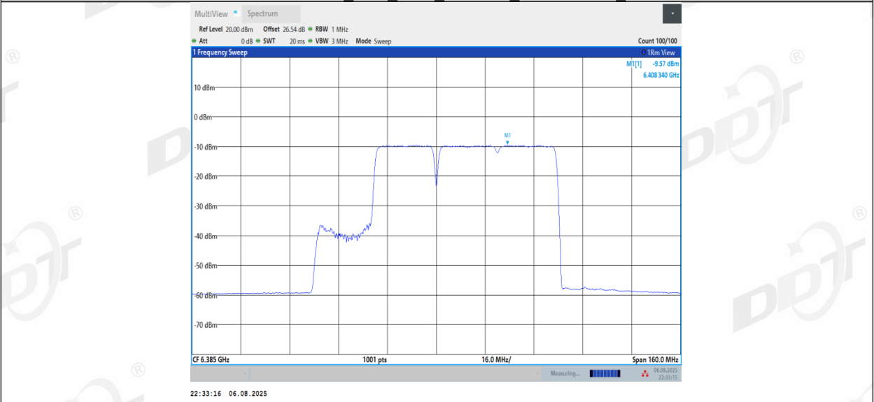
11BE80MIMO_Ant3_6385_484+242_Non-OFDMA_2
