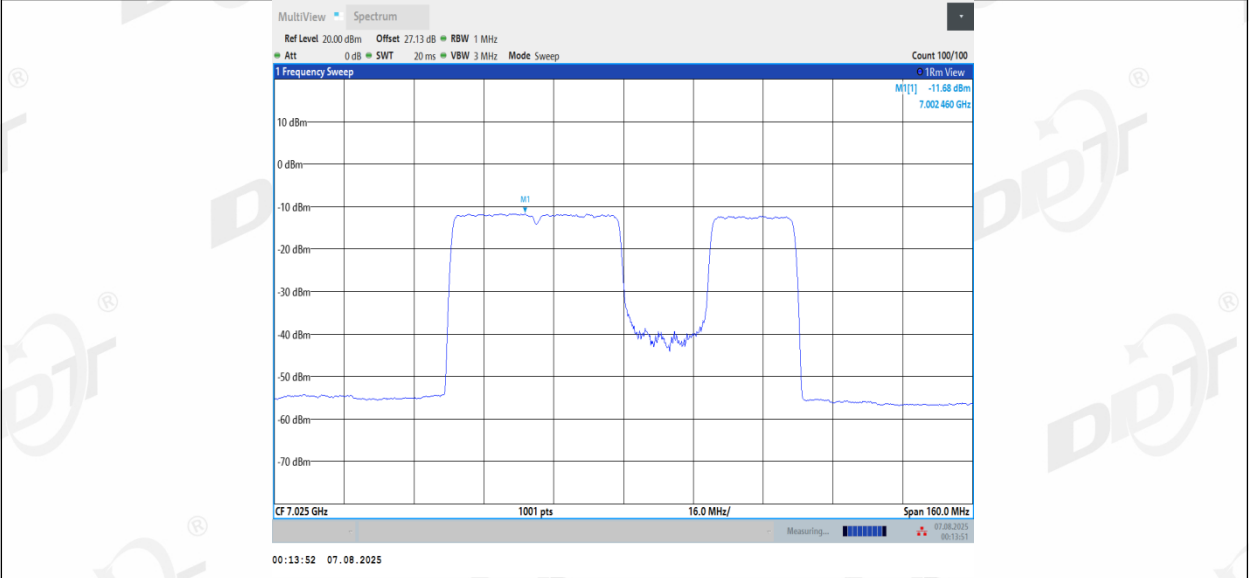
11BE80MIMO_Ant1_7025_484+242_Non-OFDMA_4
