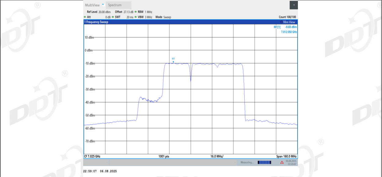
11BE80MIMO_Ant2_7025_484+242_Non-OFDMA_2
