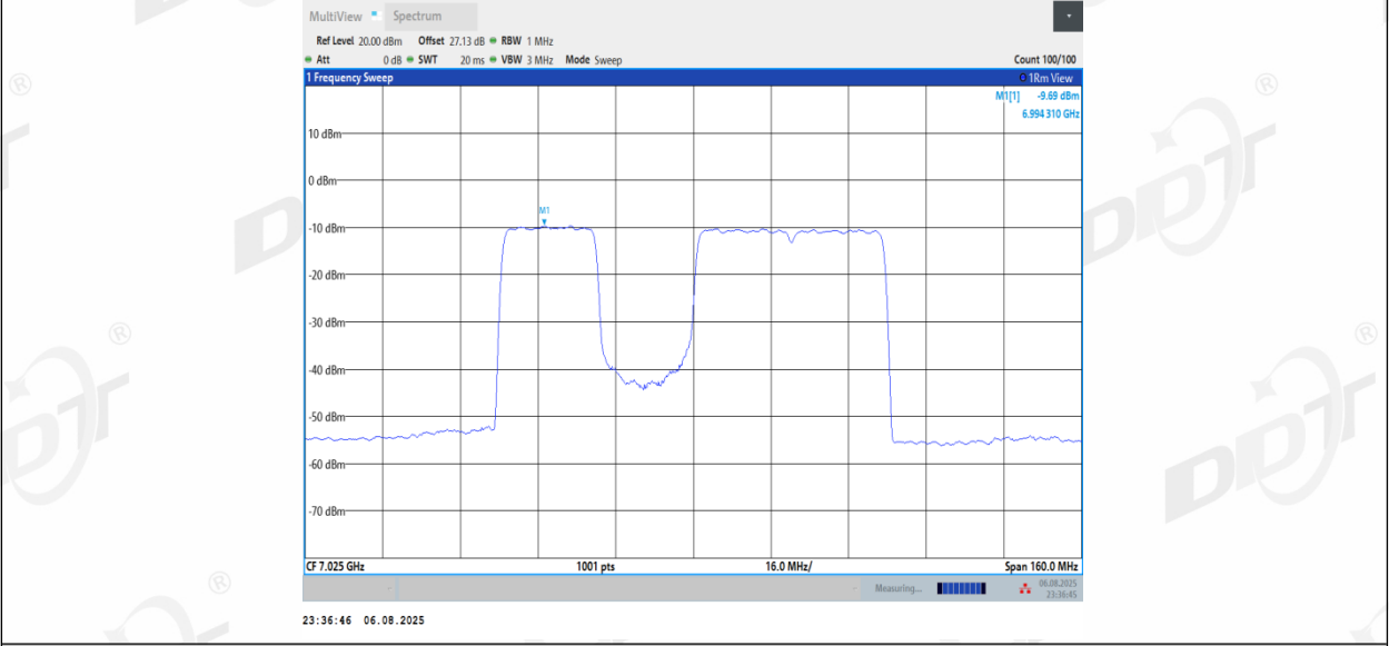
11BE80MIMO_Ant2_7025_484+242_Non-OFDMA_3
