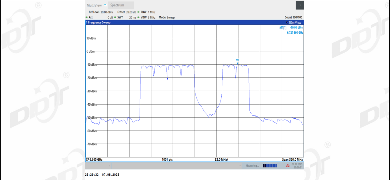
11BE160MIMO_Ant3_6665_996+484_Non-OFDMA_4
