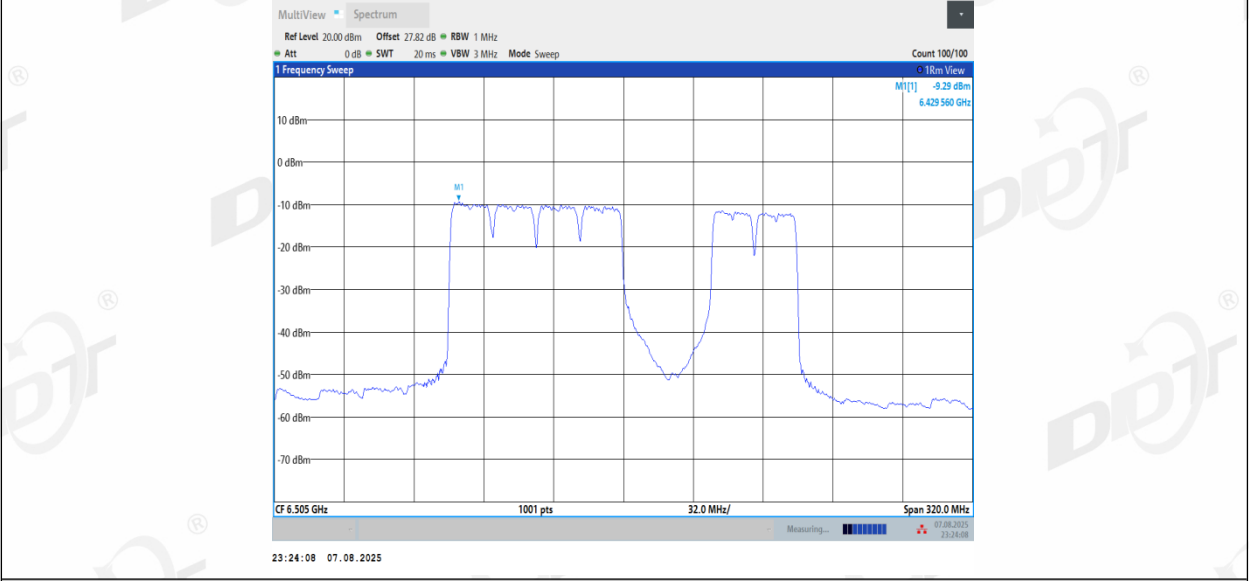
11BE160MIMO_Ant1_6505_996+484_Non-OFDMA_4
