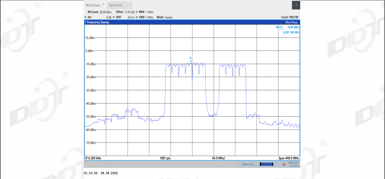
11BE320MIMO_Ant2_6265_2*996+484_Non-OFDMA_11
