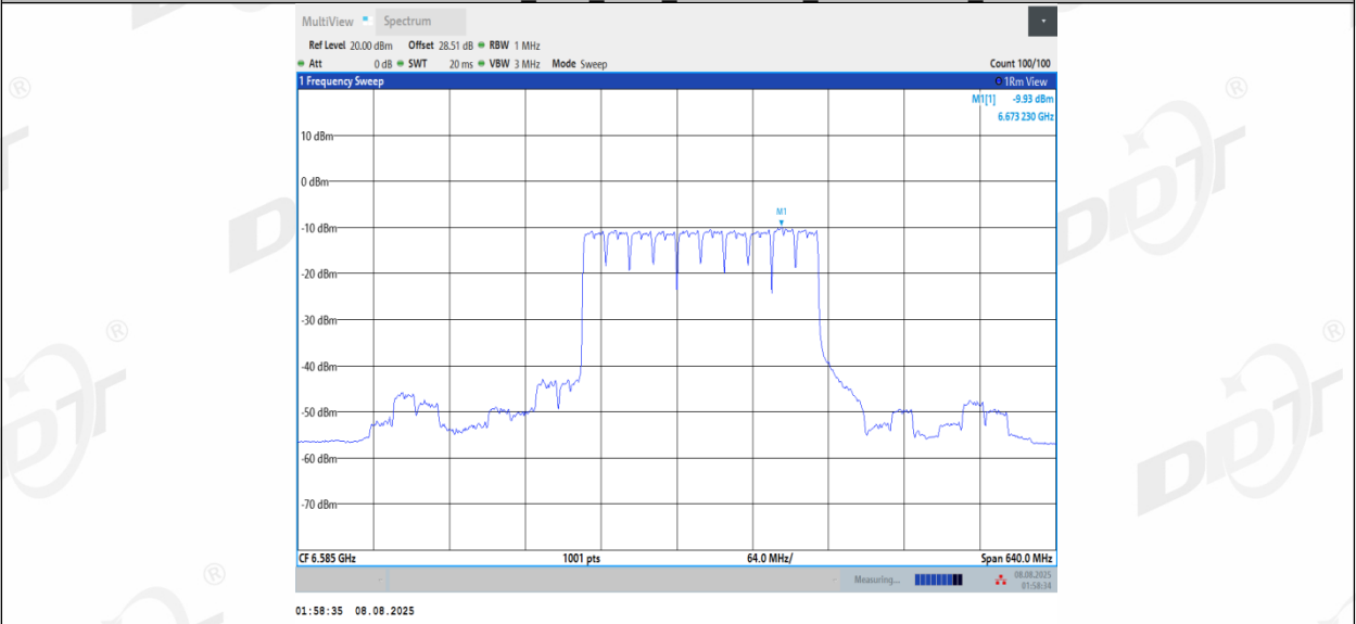
11BE320MIMO_Ant1_6585_3*996_Non-OFDMA_1
