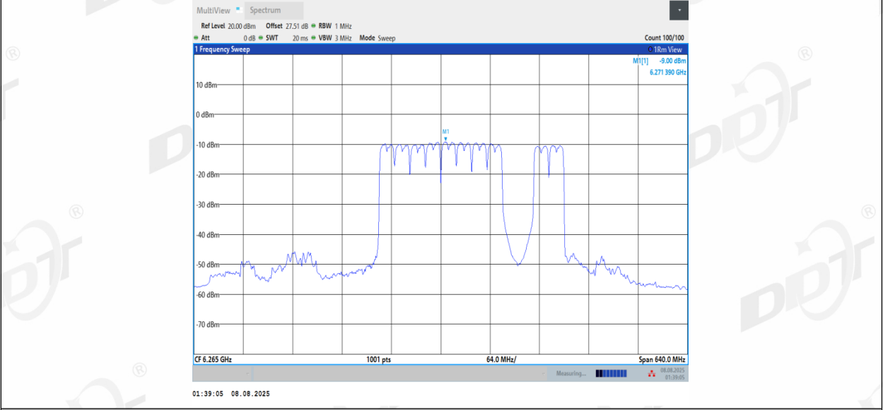
11BE320MIMO_Ant2_6265_2*996+484_Non-OFDMA_12
