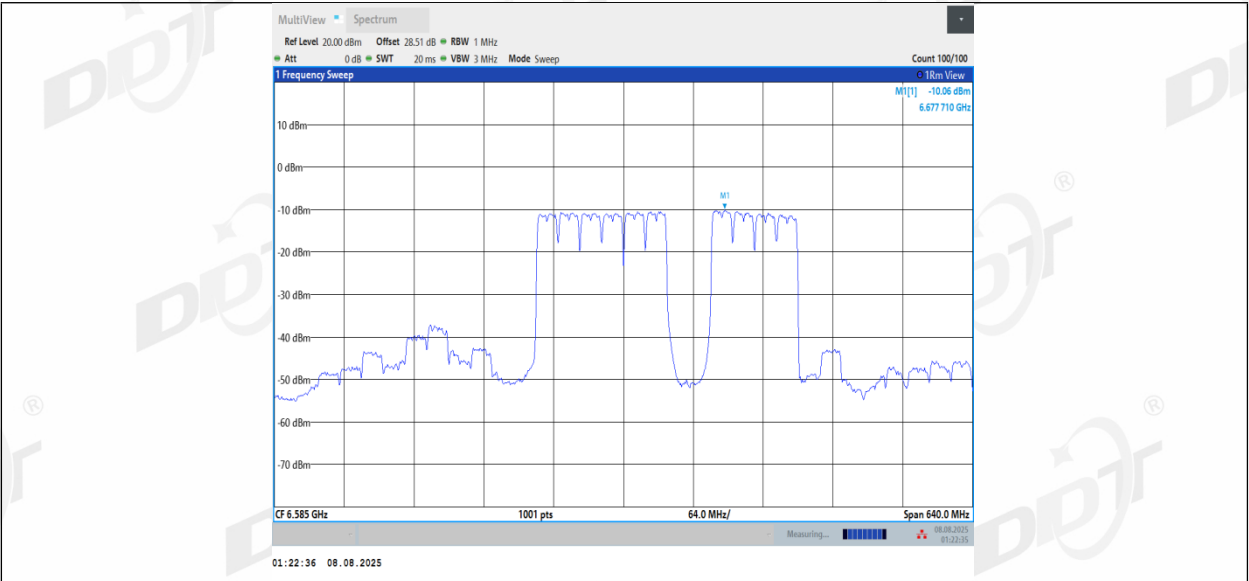
11BE320MIMO_Ant1_6585_2*996+484_Non-OFDMA_11
