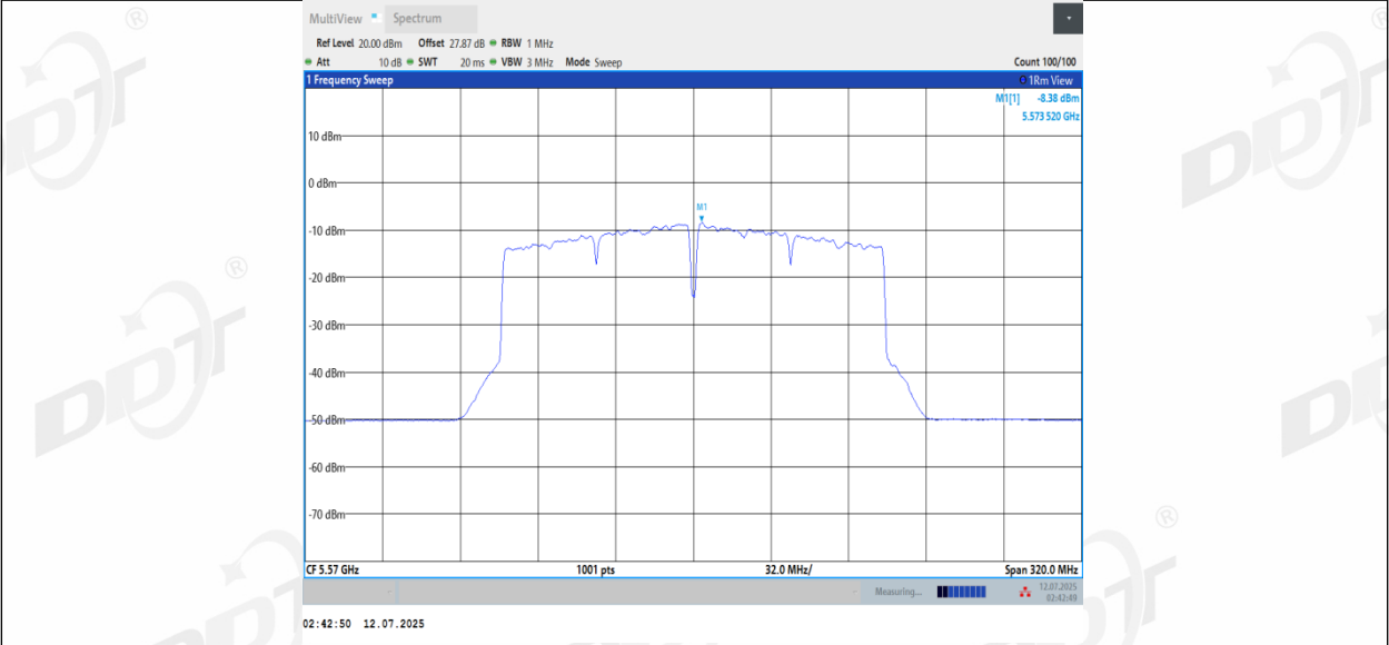
11AC160MIMO_Ant3_5570
