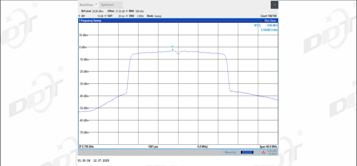
11AX20MIMO_Ant3_5745
