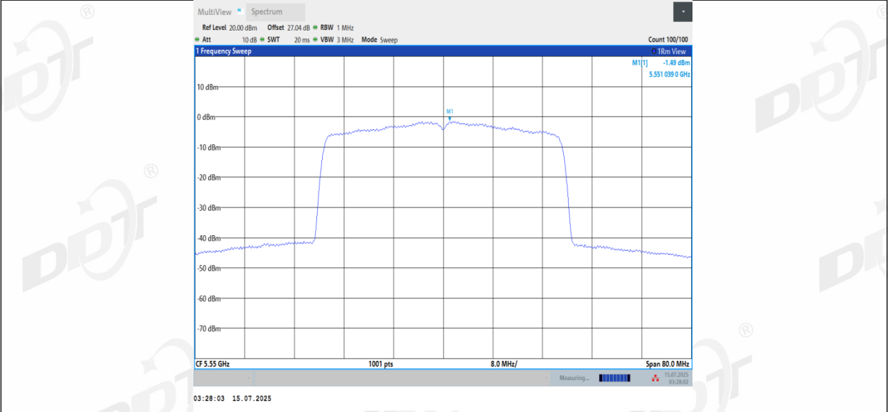
11AX40MIMO_Ant3_5550
