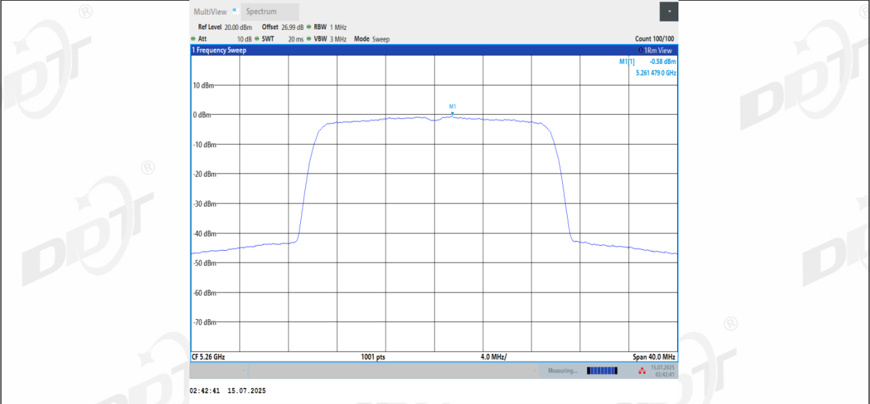
11AX20MIMO_Ant3_5260
