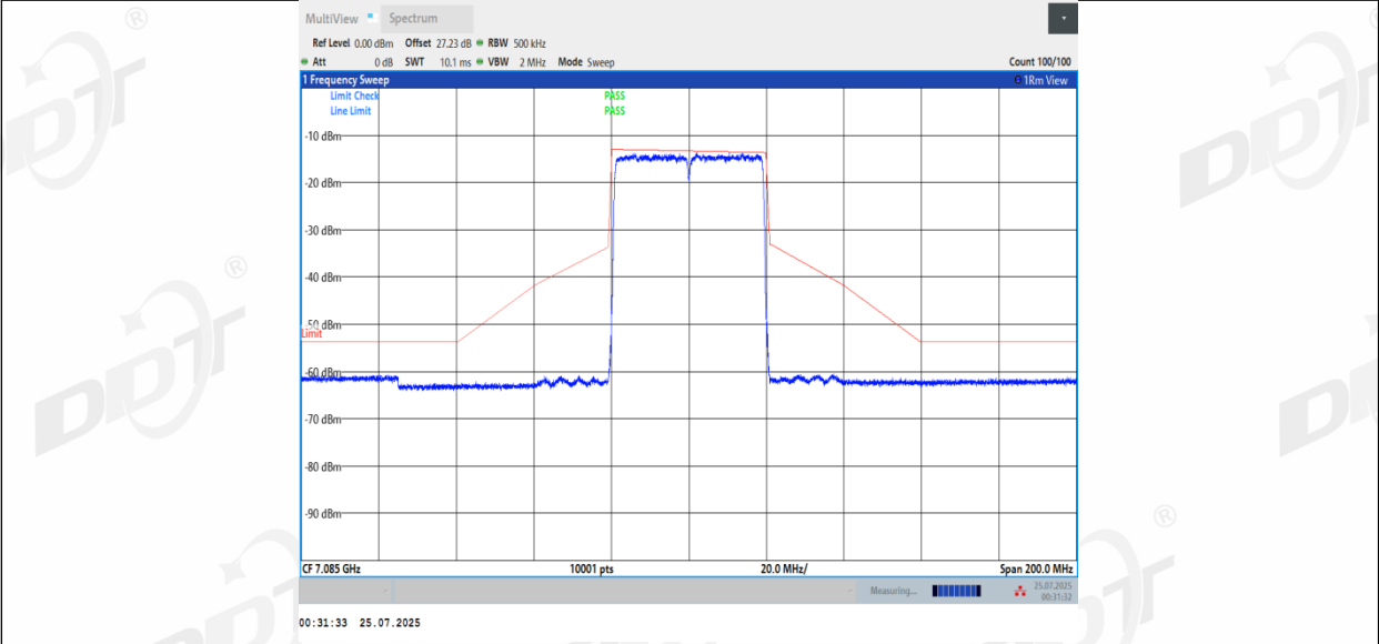
11BE40MIMO_Ant3_7085
