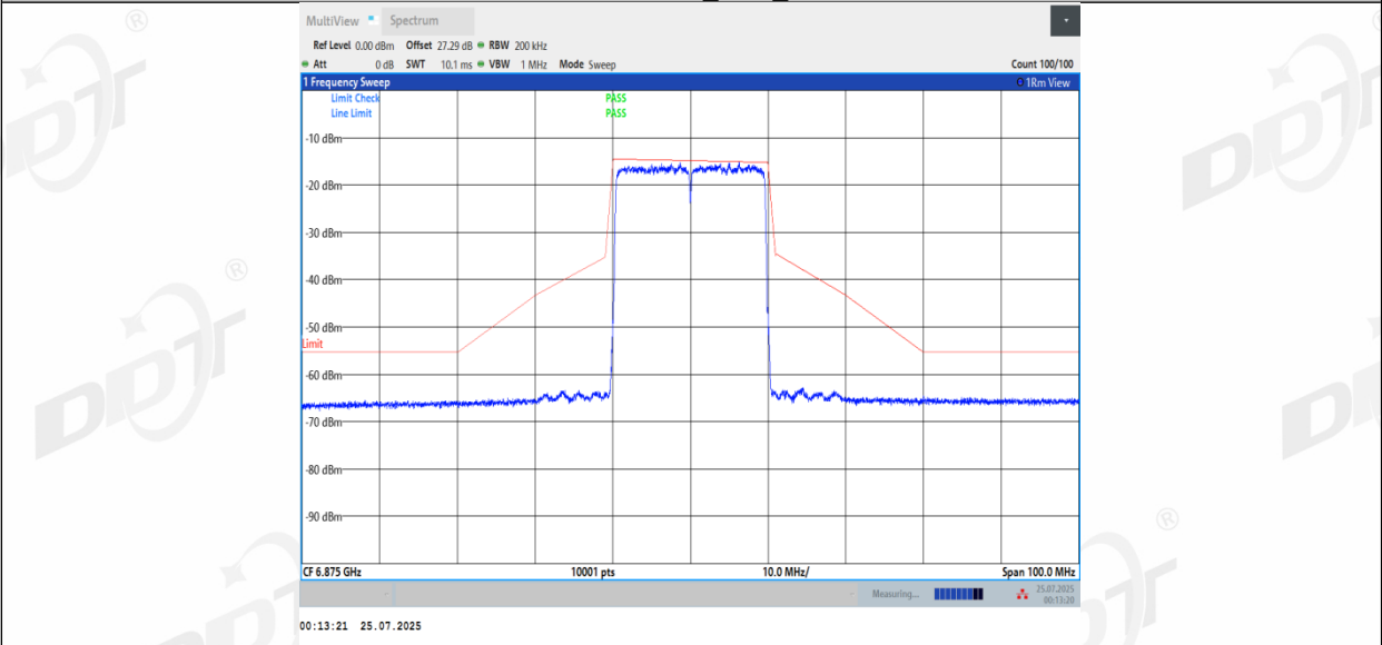
11BE20MIMO_Ant3_6875
