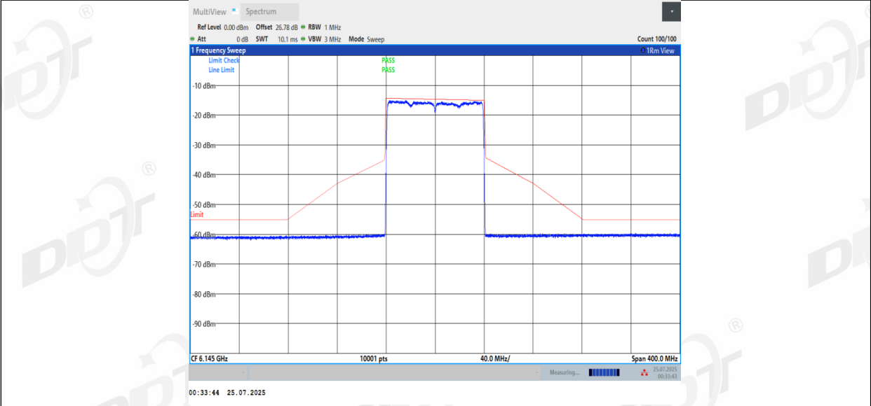
11BE80MIMO_Ant3_6145
