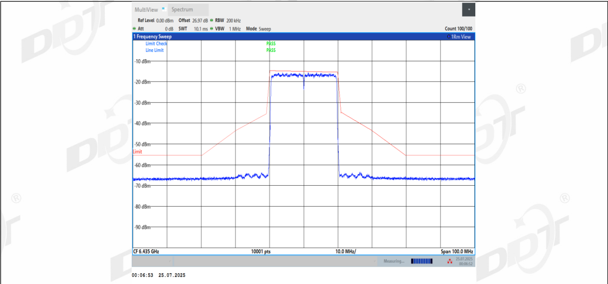
11BE20MIMO_Ant2_6435
