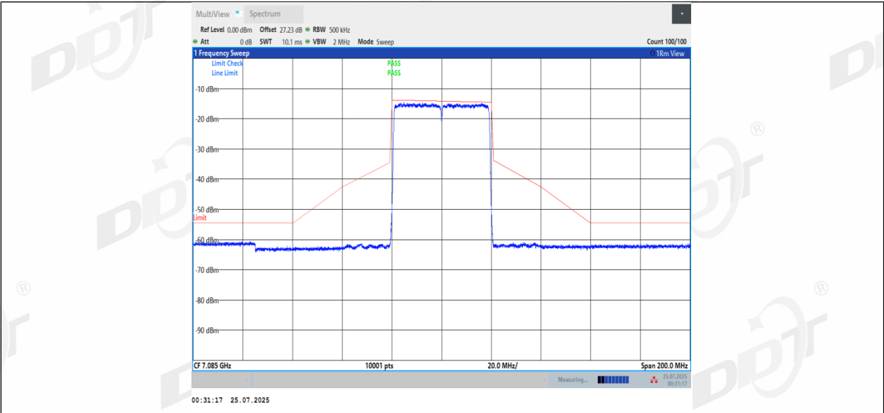
11BE40MIMO_Ant2_7085
