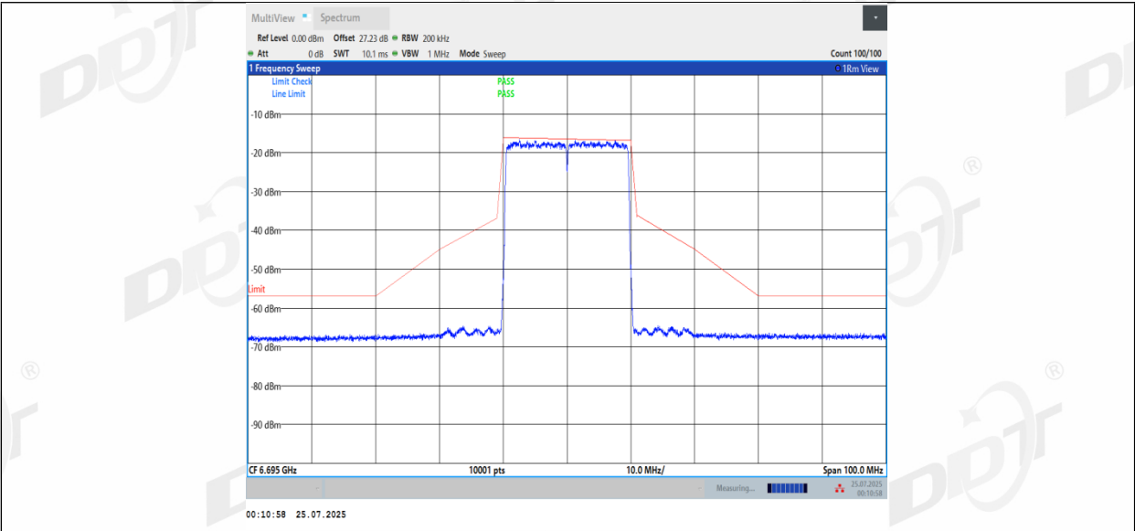
11BE20MIMO_Ant2_6695
