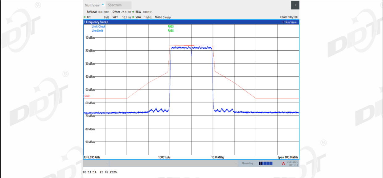
11BE20MIMO_Ant3_6695
