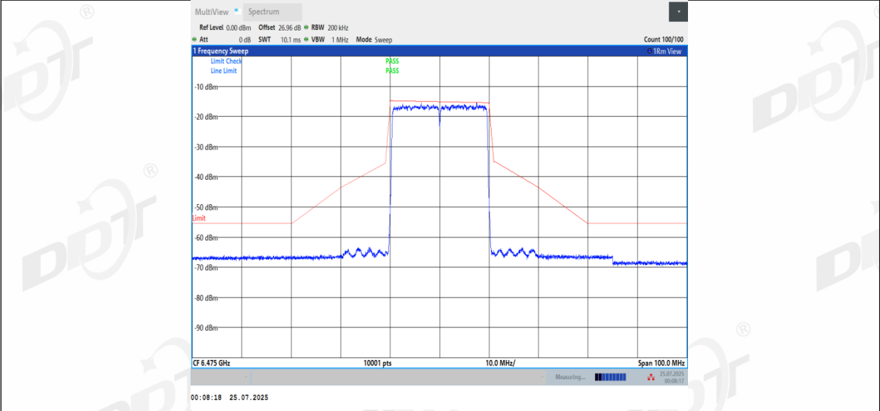
11BE20MIMO_Ant3_6475
