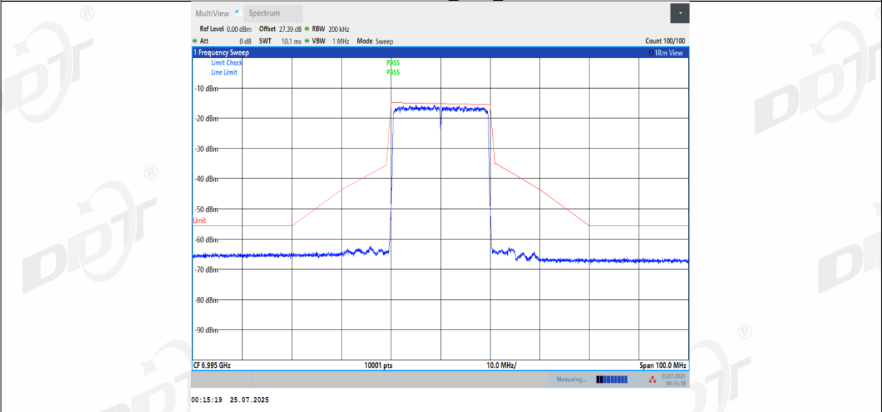
11BE20MIMO_Ant3_6995
