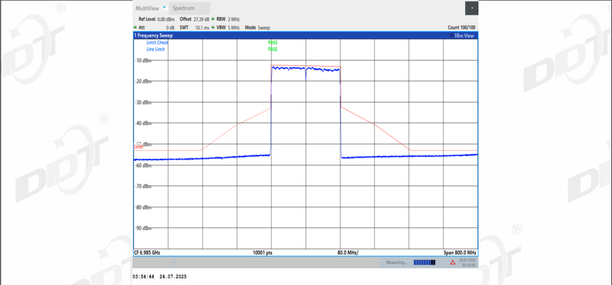
11AX160MIMO_Ant3_6985
