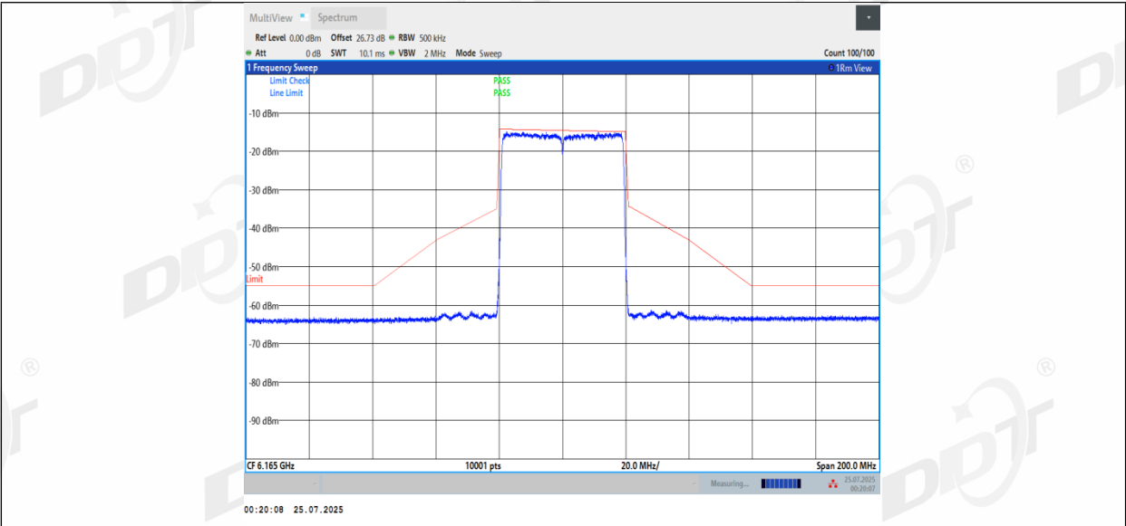
11BE40MIMO_Ant2_6165
