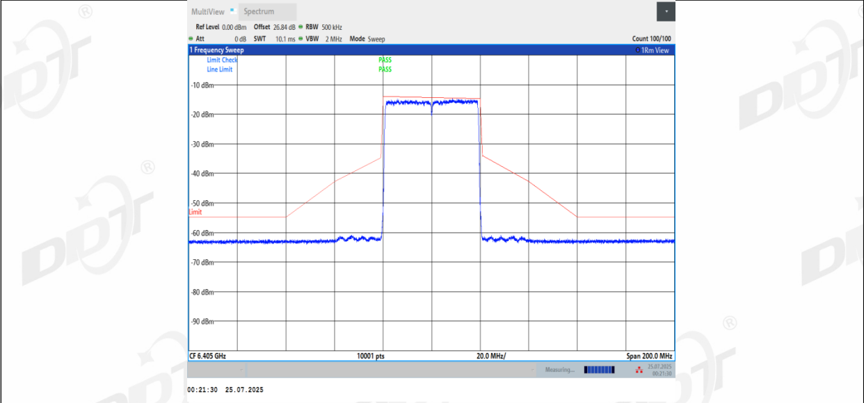
11BE40MIMO_Ant3_6405
