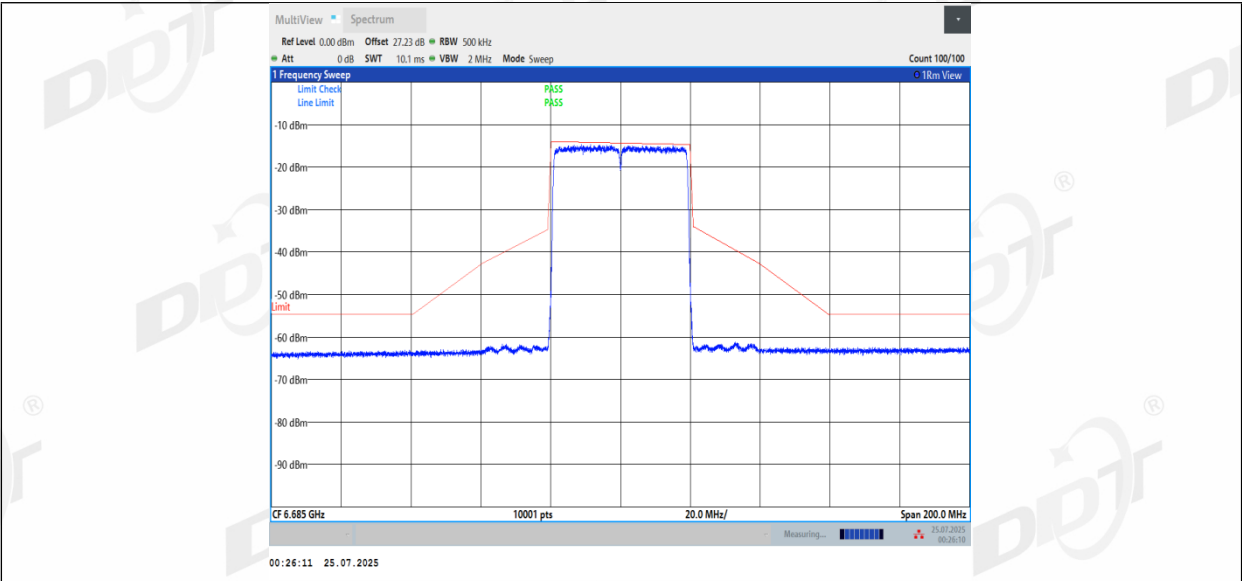
11BE40MIMO_Ant2_6685
