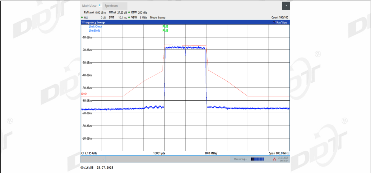
11BE20MIMO_Ant2_7115
