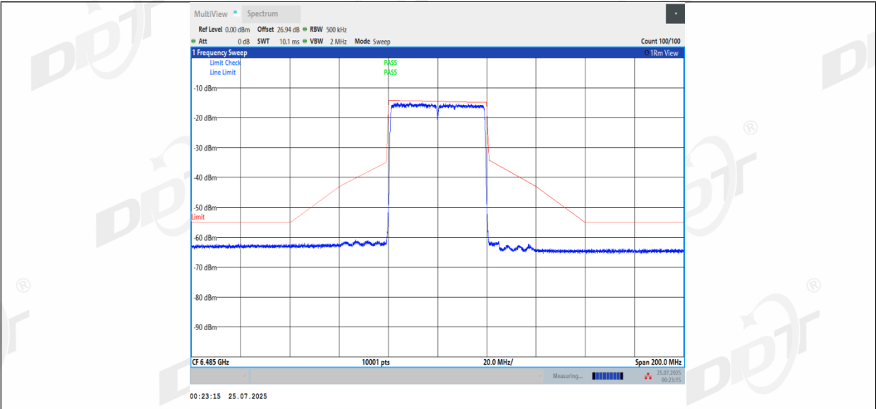
11BE40MIMO_Ant2_6485
