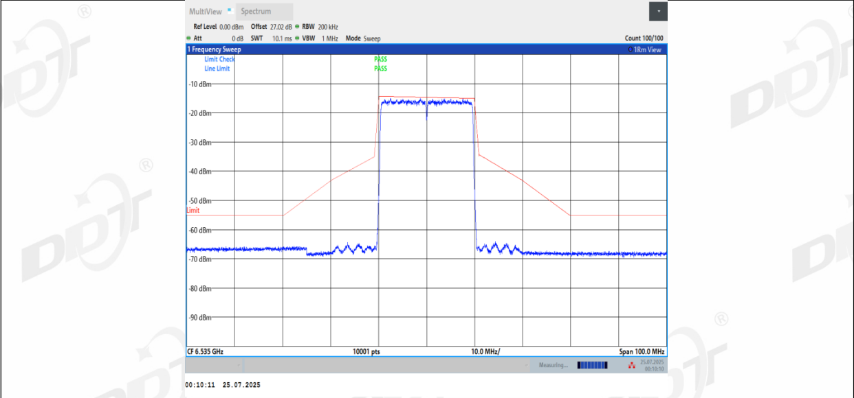
11BE20MIMO_Ant3_6535
