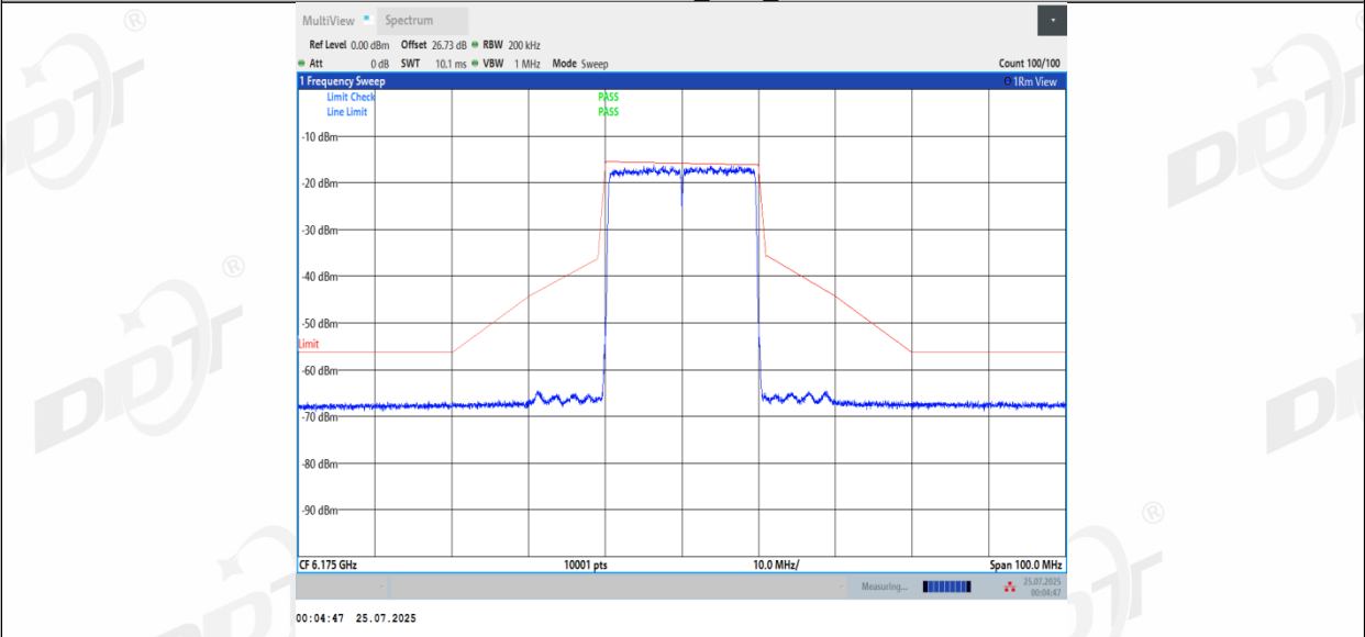
11BE20MIMO_Ant3_6175
