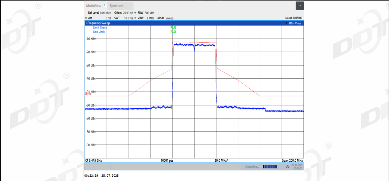
11BE40MIMO_Ant3_6445
