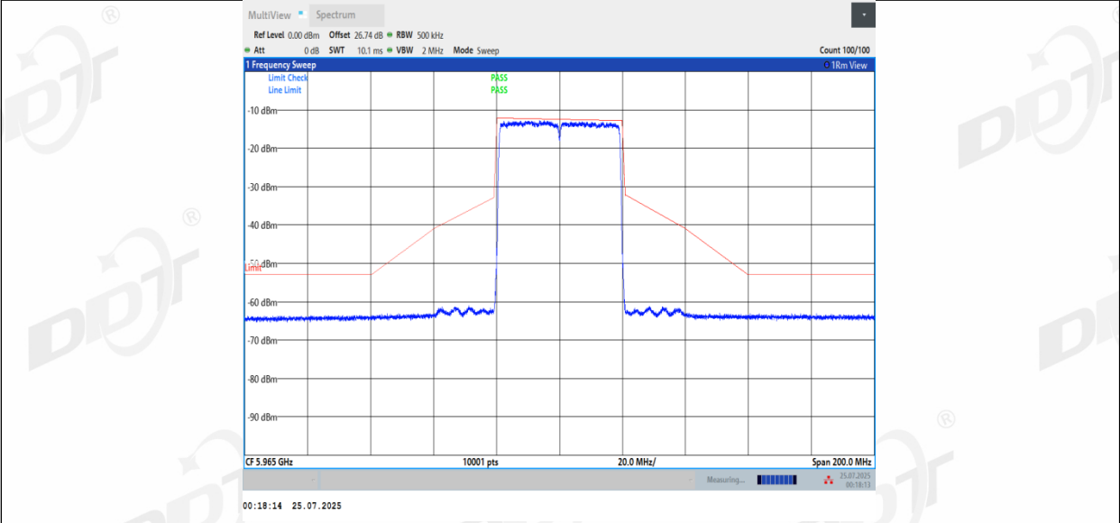
11BE40MIMO_Ant3_5965
