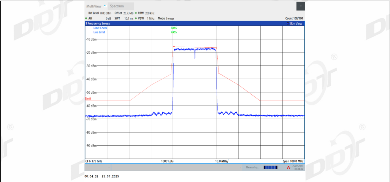
11BE20MIMO_Ant2_6175
