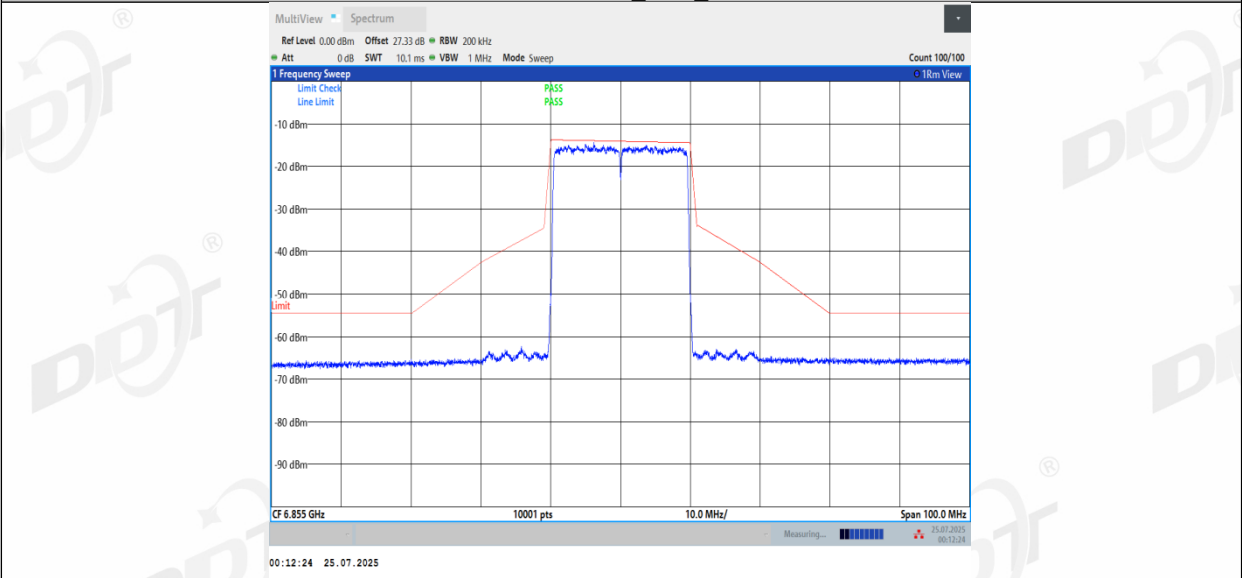
11BE20MIMO_Ant3_6855
