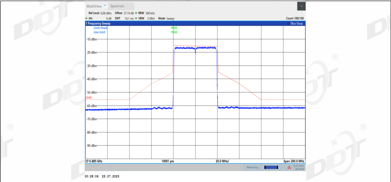
11BE40MIMO_Ant2_6885
