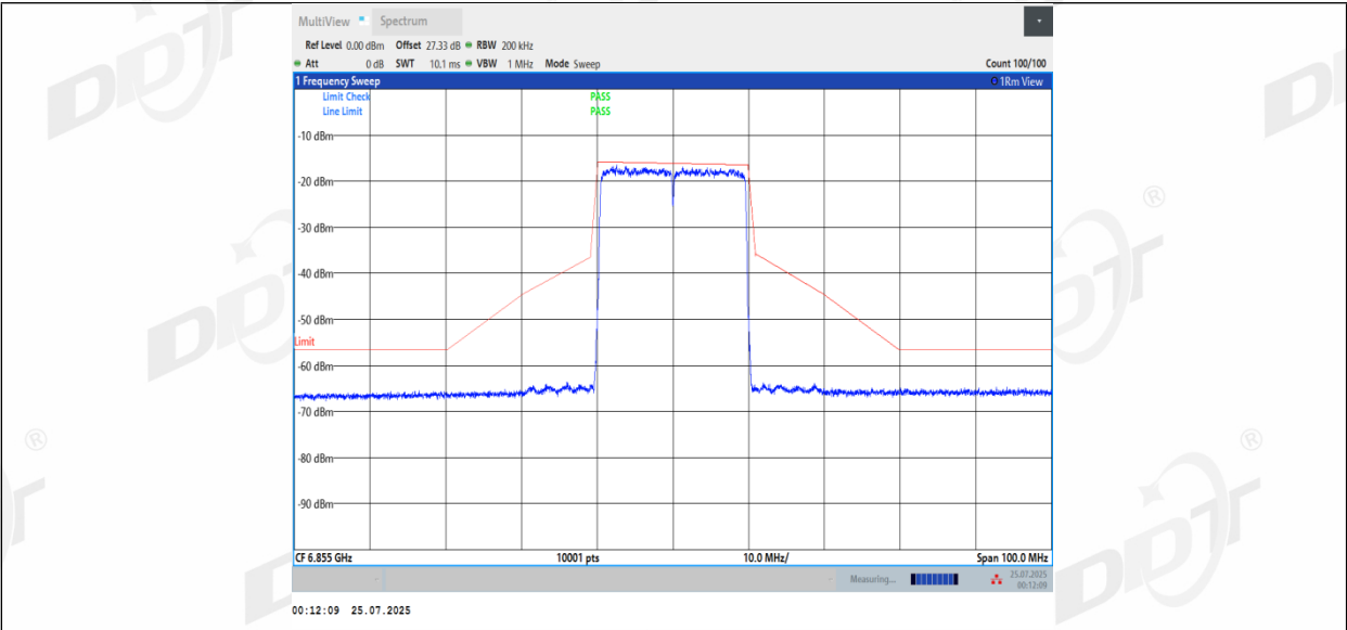
11BE20MIMO_Ant2_6855
