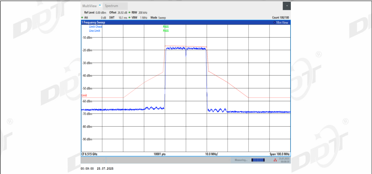
11BE20MIMO_Ant2_6515
