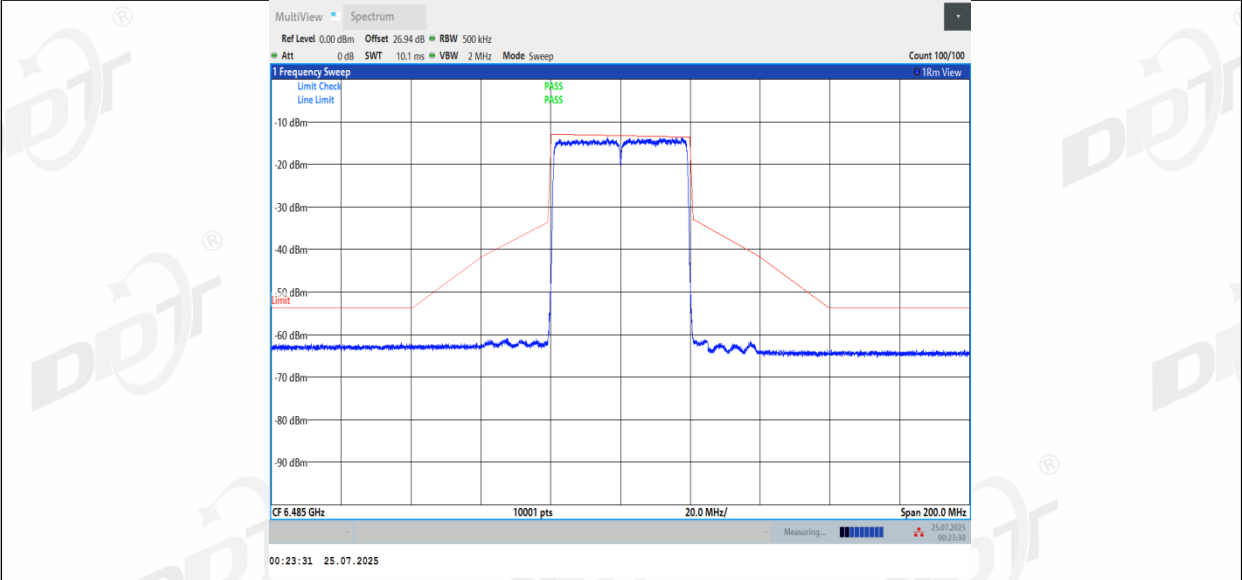
11BE40MIMO_Ant3_6485
