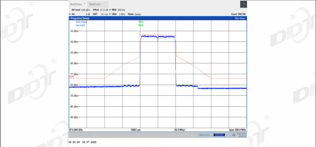
11BE40MIMO_Ant3_6965
