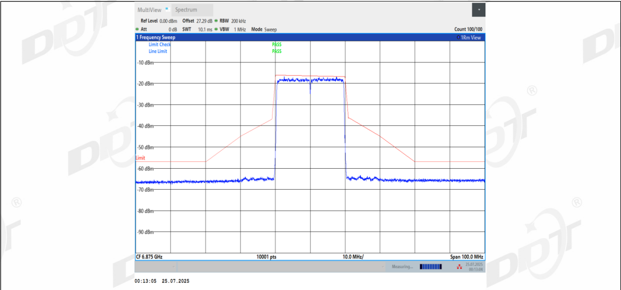
11BE20MIMO_Ant2_6875
