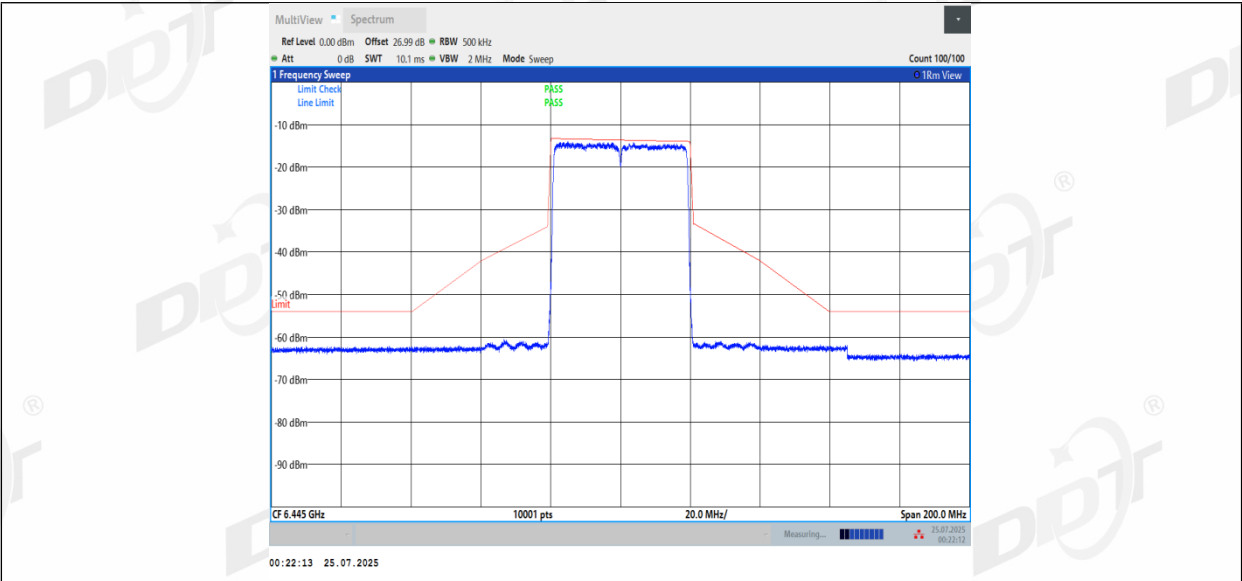
11BE40MIMO_Ant2_6445
