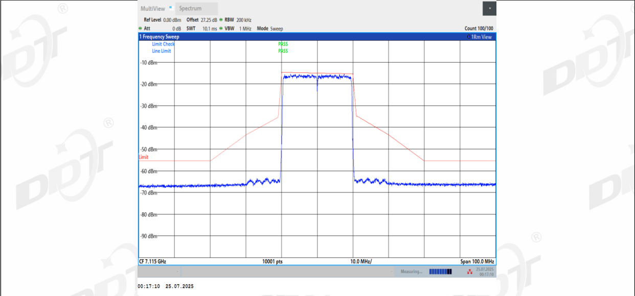
11BE20MIMO_Ant3_7115
