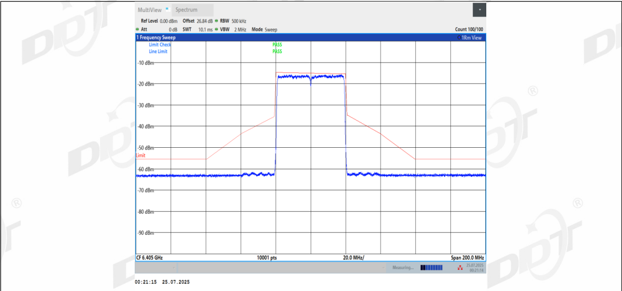
11BE40MIMO_Ant2_6405
