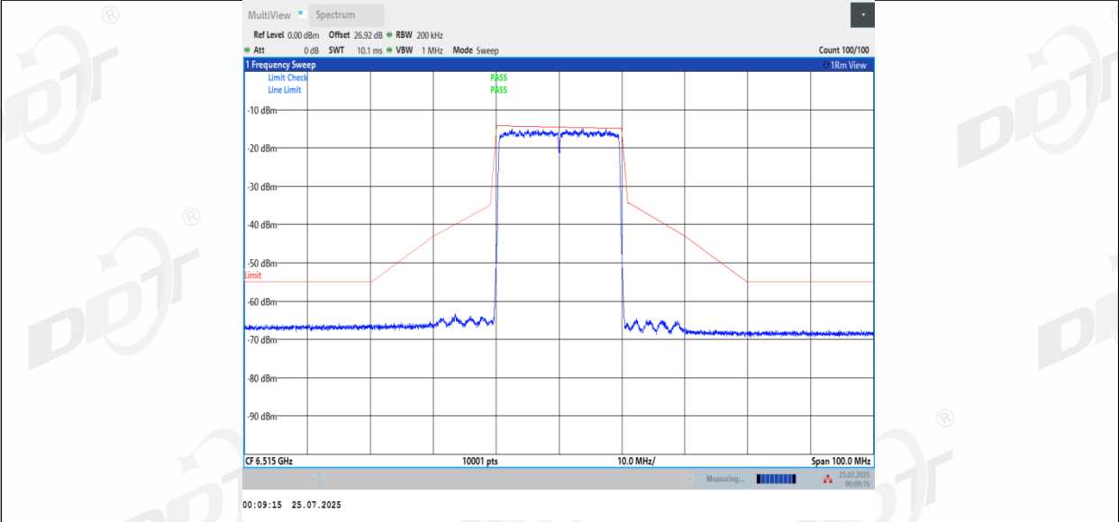
11BE20MIMO_Ant3_6515
