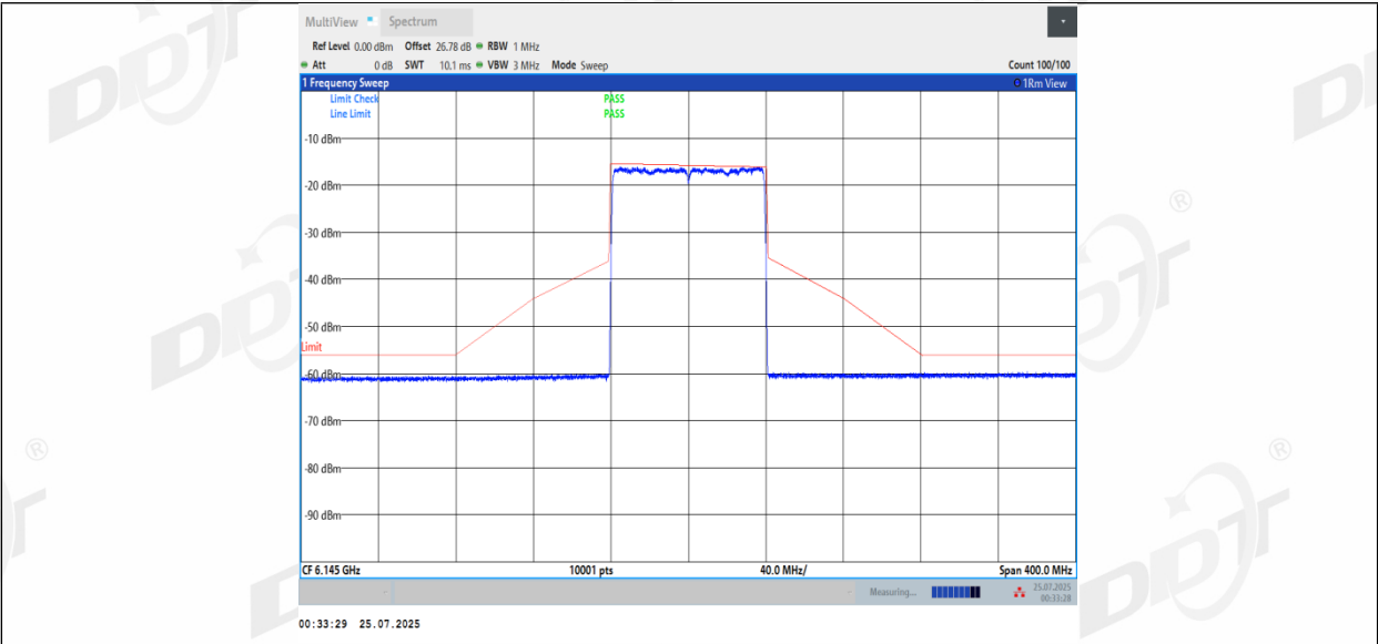
11BE80MIMO_Ant2_6145
