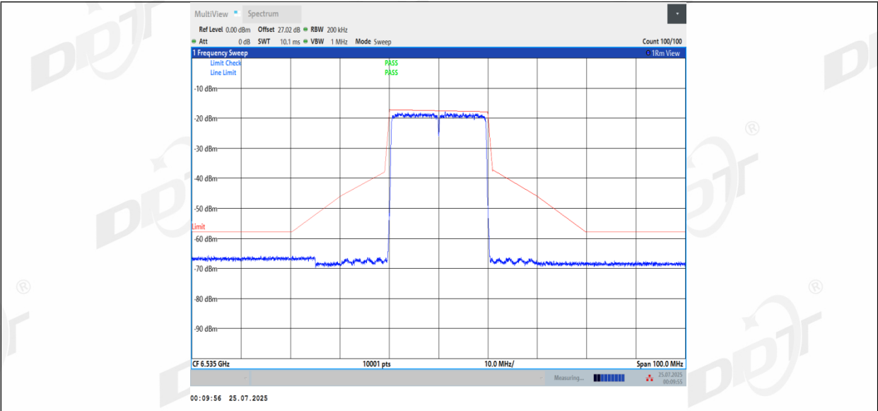
11BE20MIMO_Ant2_6535
