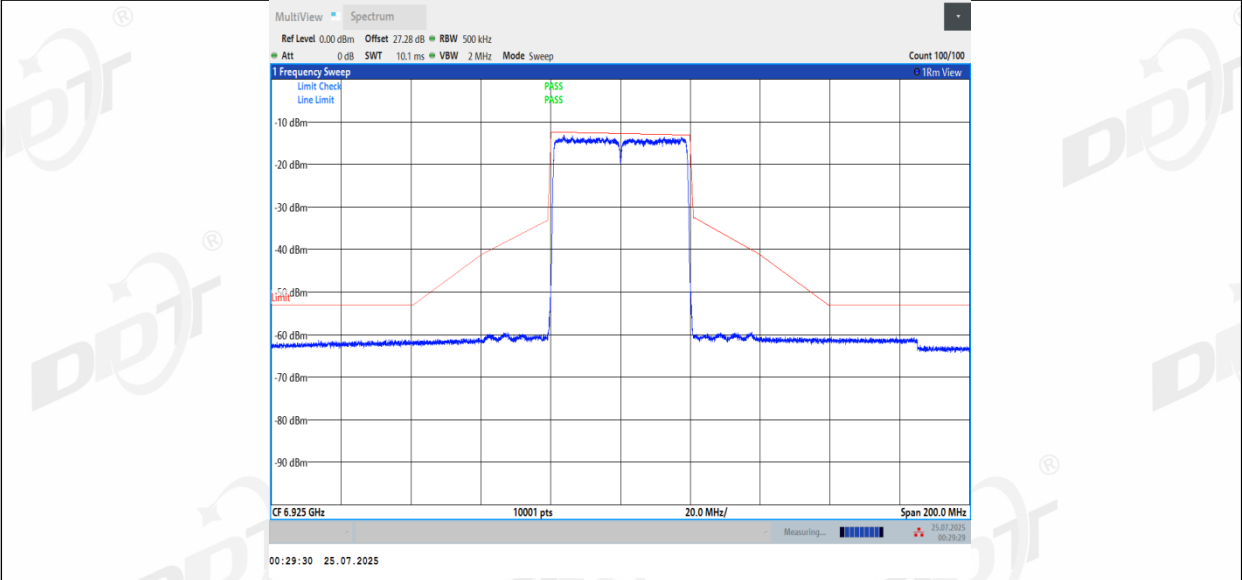
11BE40MIMO_Ant3_6925
