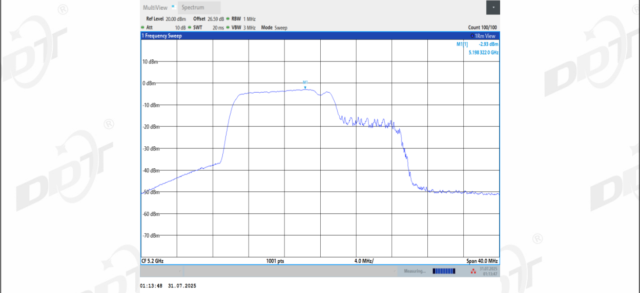
11BE20MIMO_Ant3_5200_106+26_OFDMA_2
