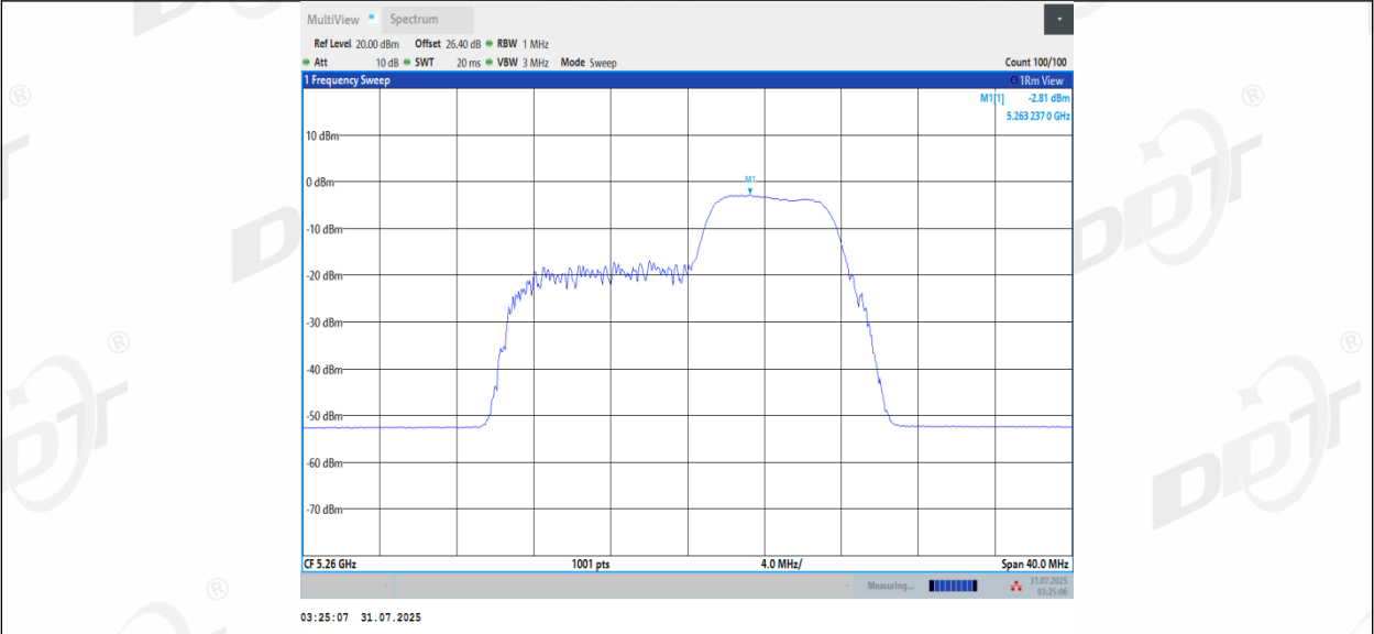
11BE20MIMO_Ant1_5260_106+26_OFDMA_1
