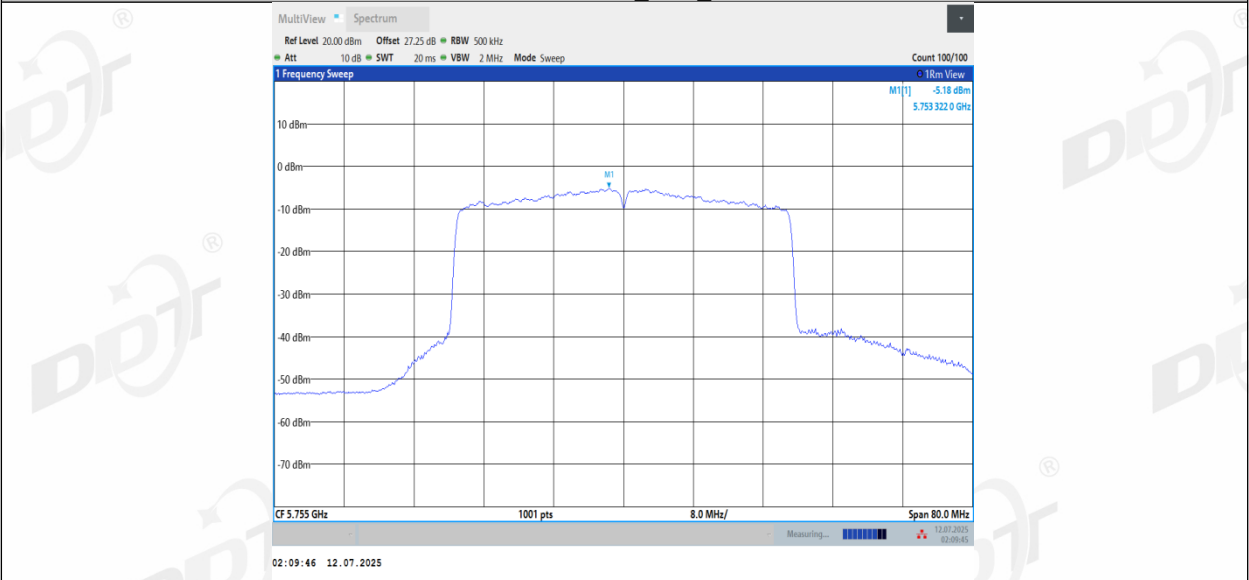
11BE40MIMO_Ant3_5755
