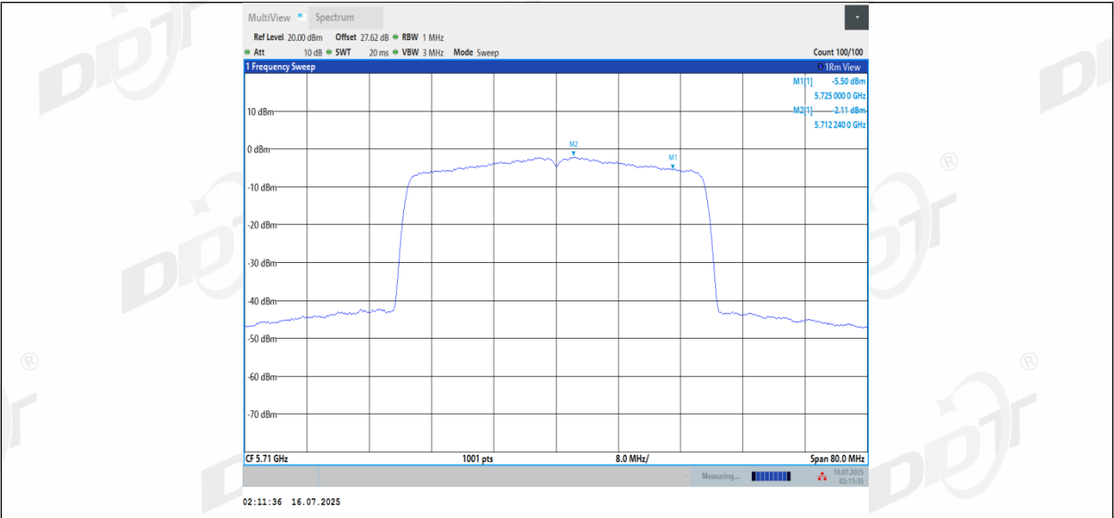
11BE40MIMO_Ant2_5710_UNII-2C
