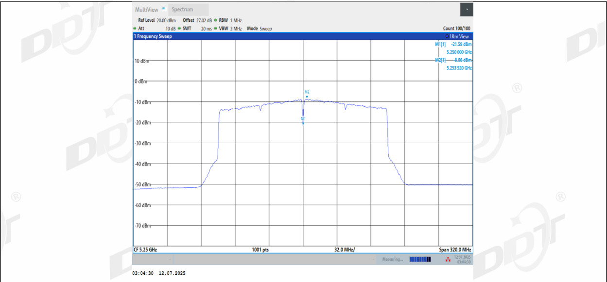
11BE160MIMO_Ant2_5250_UNII-2A
