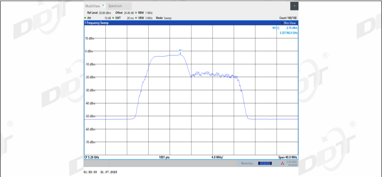
11BE20MIMO_Ant1_5260_52+26_OFDMA_2
