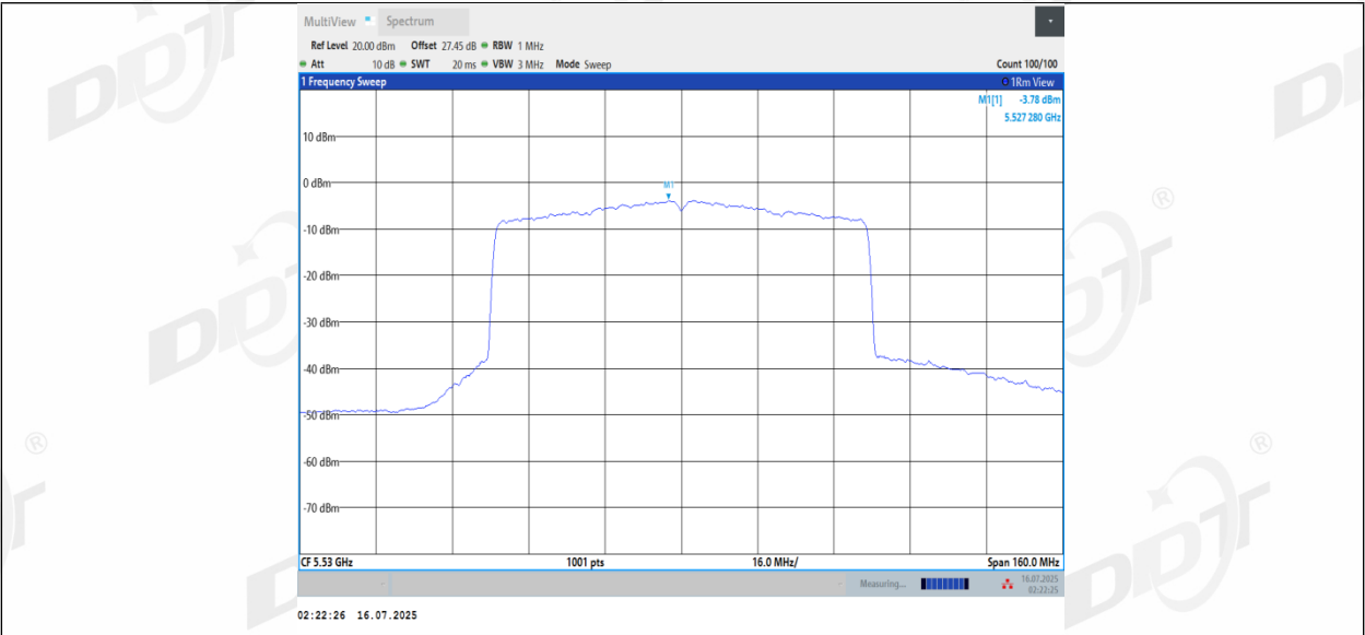
11BE80MIMO_Ant2_5530
