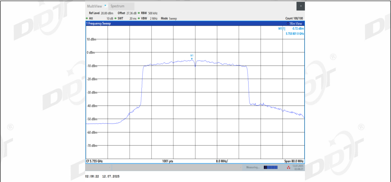
11BE40MIMO_Ant2_5755
