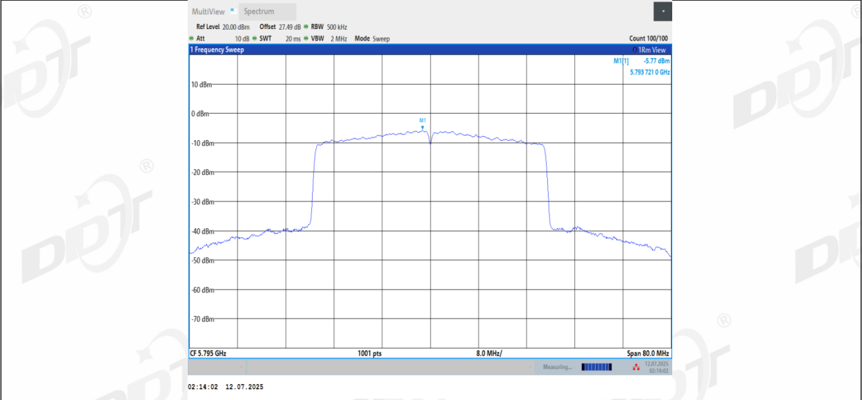
11BE40MIMO_Ant3_5795
