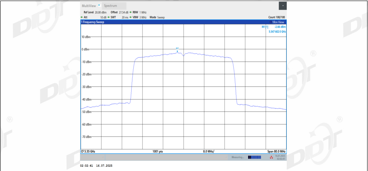
11BE40MIMO_Ant2_5550
