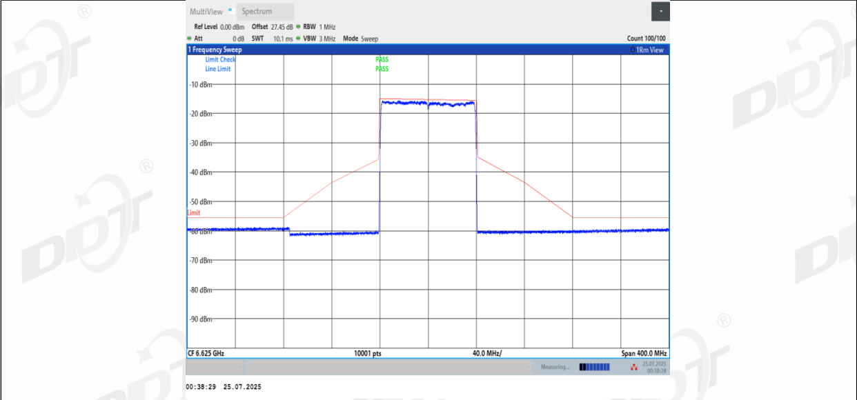
11BE80MIMO_Ant3_6625
