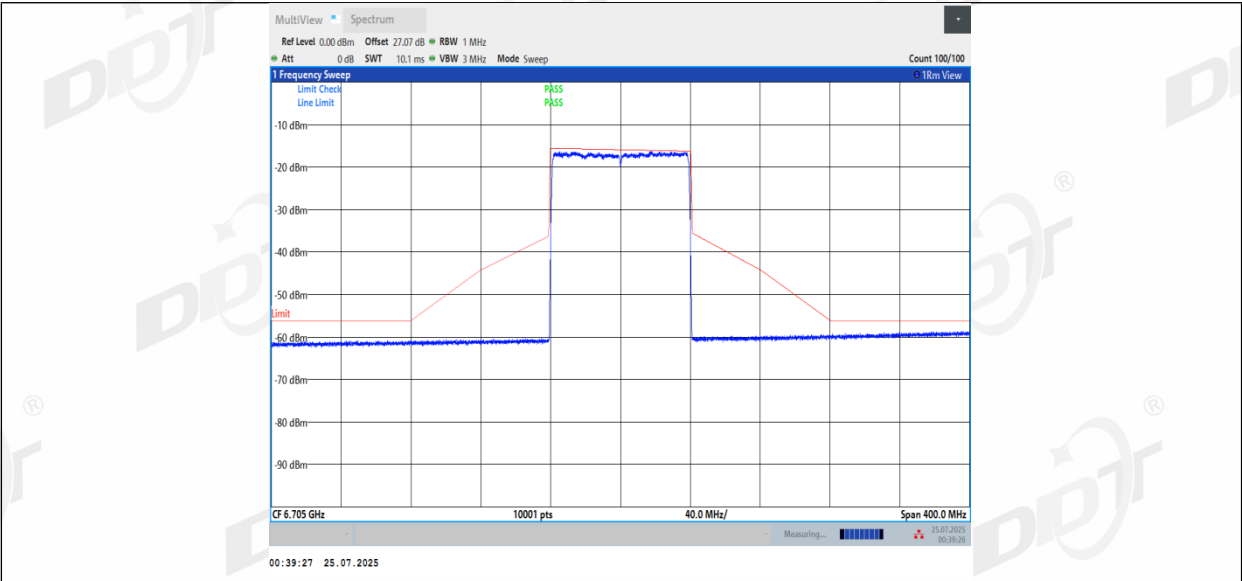
11BE80MIMO_Ant2_6705
