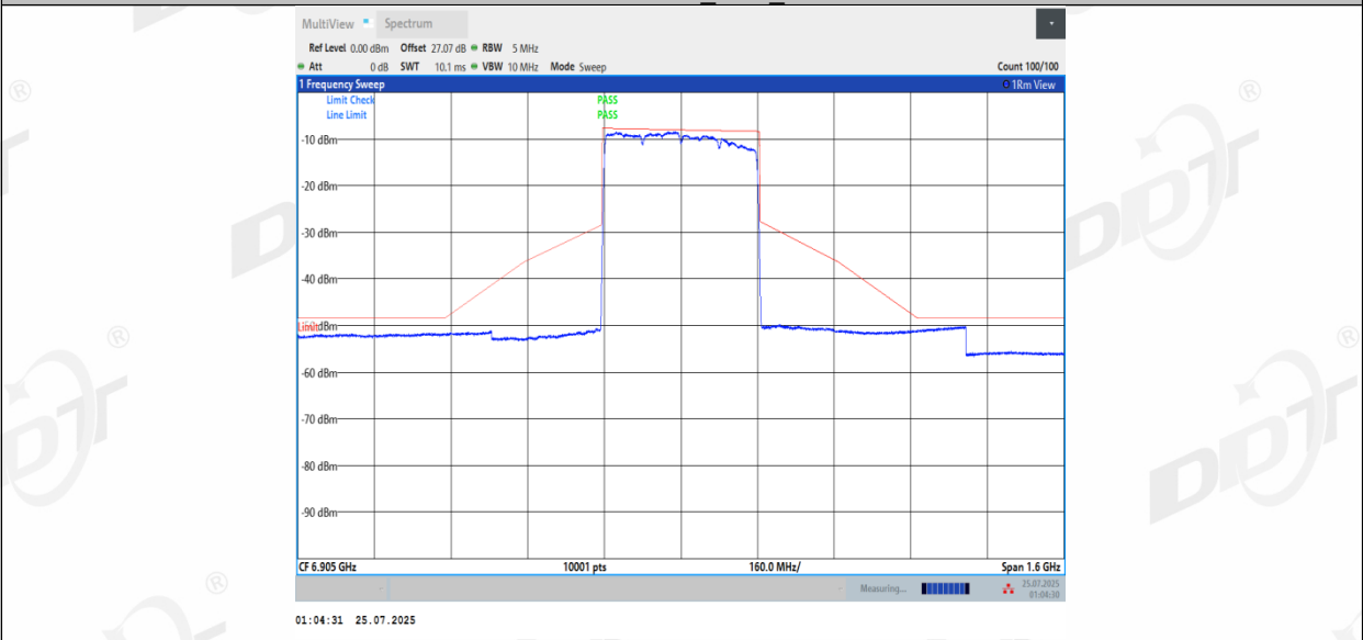
11BE320MIMO_Ant3_6905
