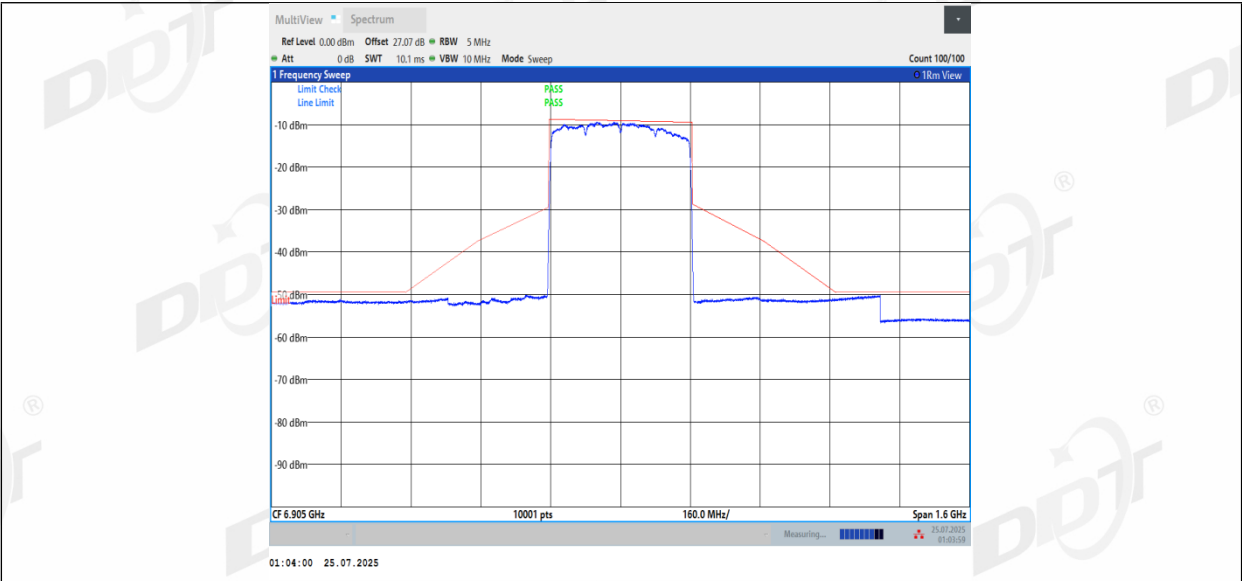
11BE320MIMO_Ant2_6905
