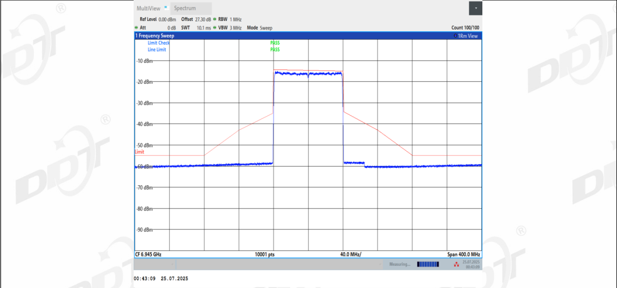
11BE80MIMO_Ant3_6945
