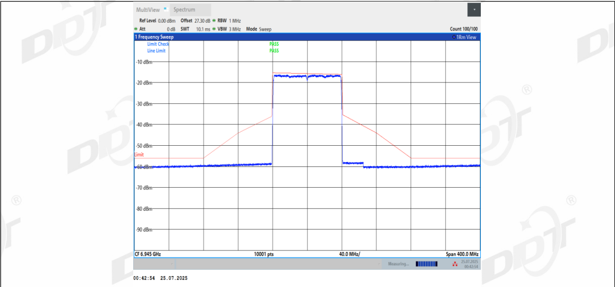
11BE80MIMO_Ant2_6945
