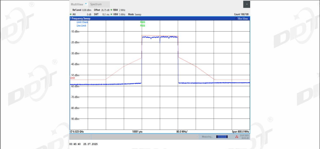
11BE160MIMO_Ant3_6025
