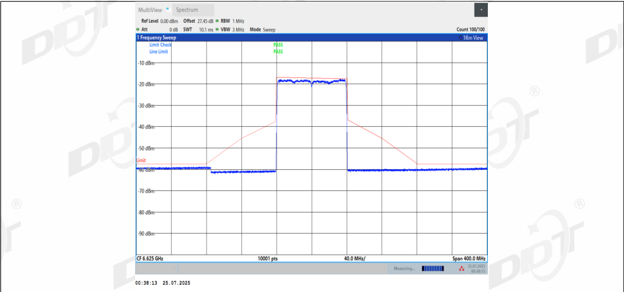
11BE80MIMO_Ant2_6625
