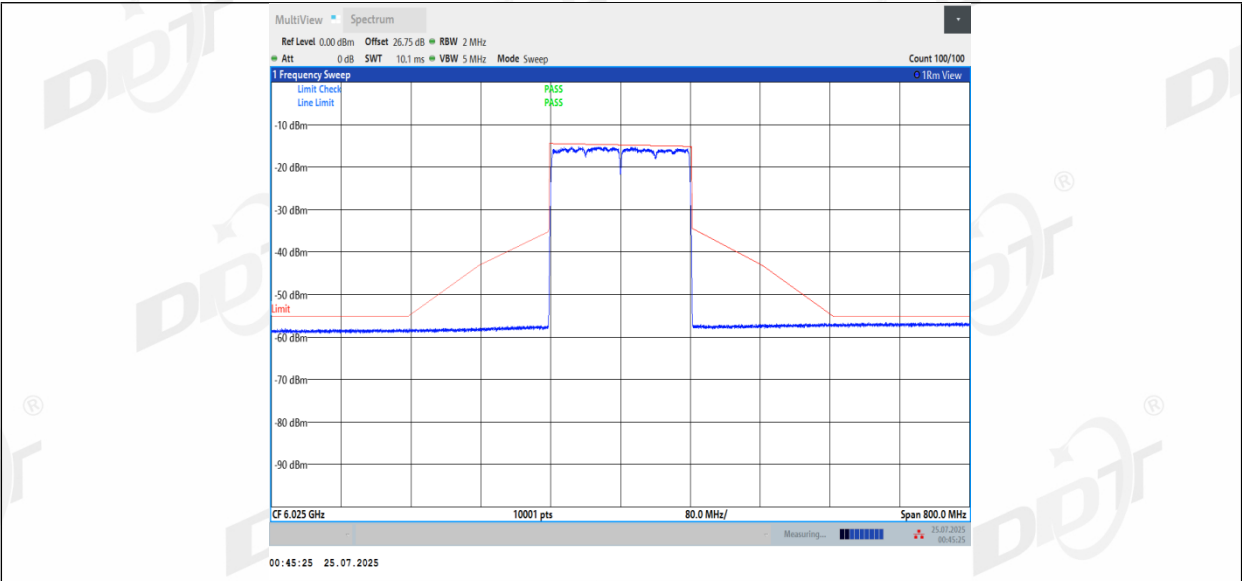
11BE160MIMO_Ant2_6025
