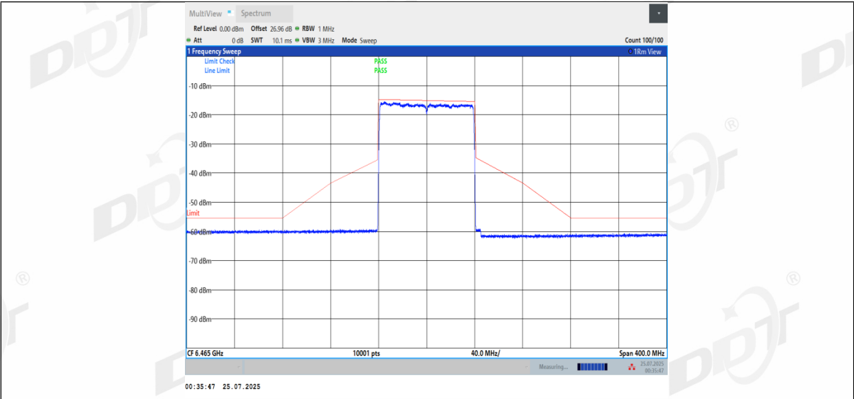
11BE80MIMO_Ant2_6465
