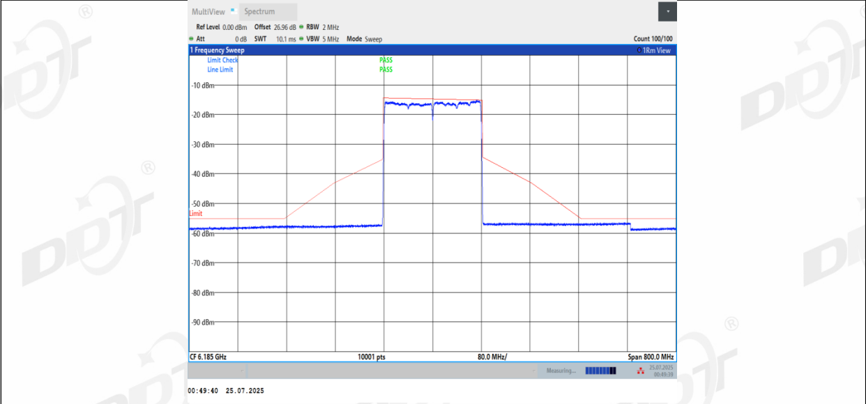
11BE160MIMO_Ant3_6185
