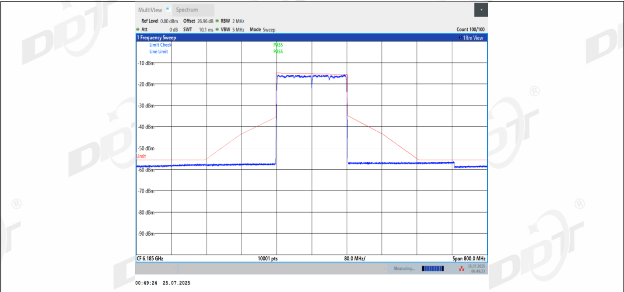
11BE160MIMO_Ant2_6185
