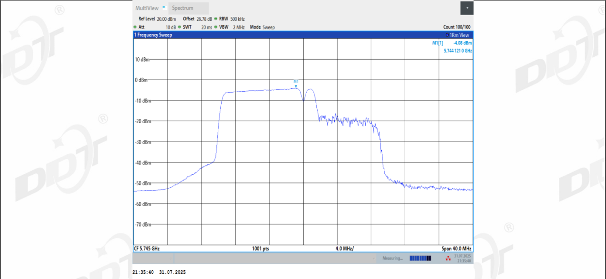
11BE20MIMO_Ant3_5745_106+26_OFDMA_2
