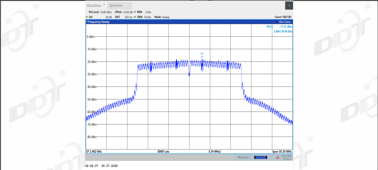
11N20MIMO_Ant2_2462
