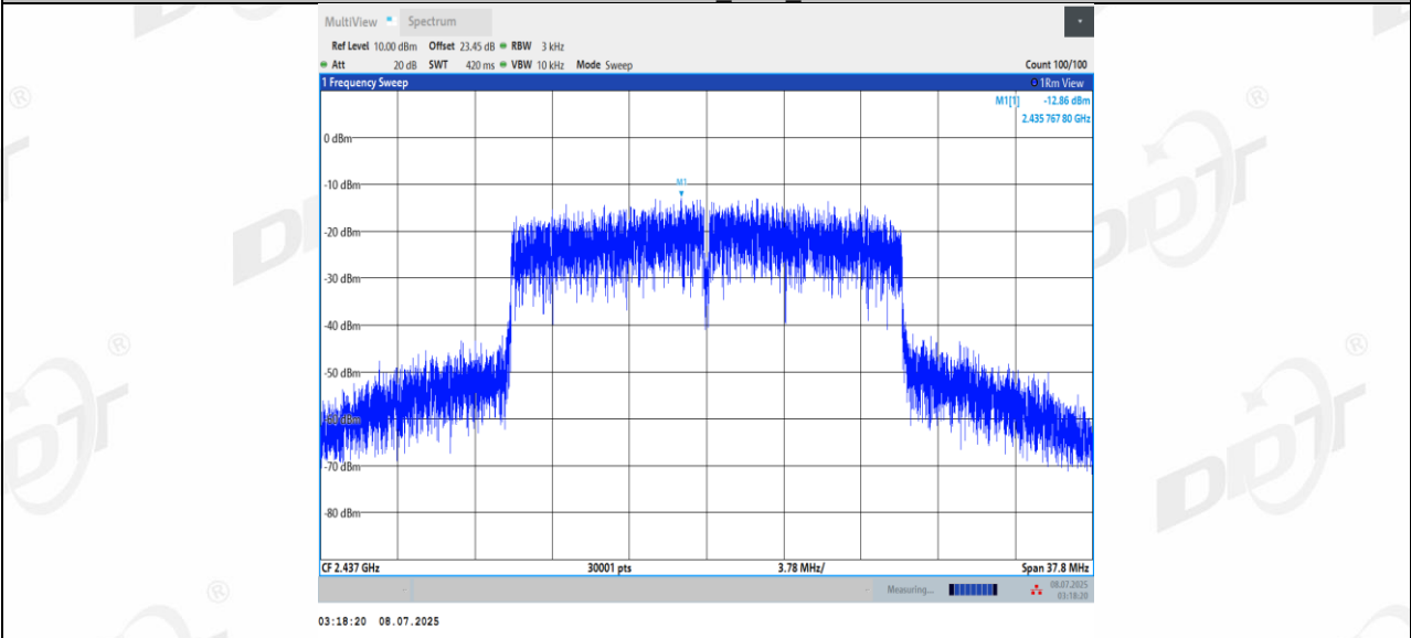
11BE20MIMO Ant2 2437
