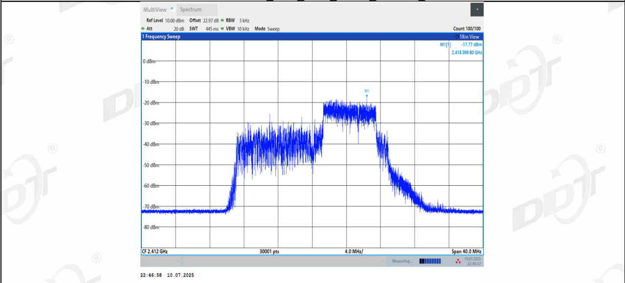
11BE20MIMO_Ant1_2412_106+26_OFDMA_1
