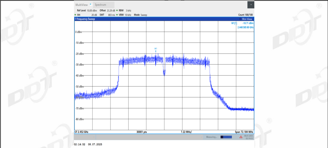
11N40MIMO_Ant2_2452
