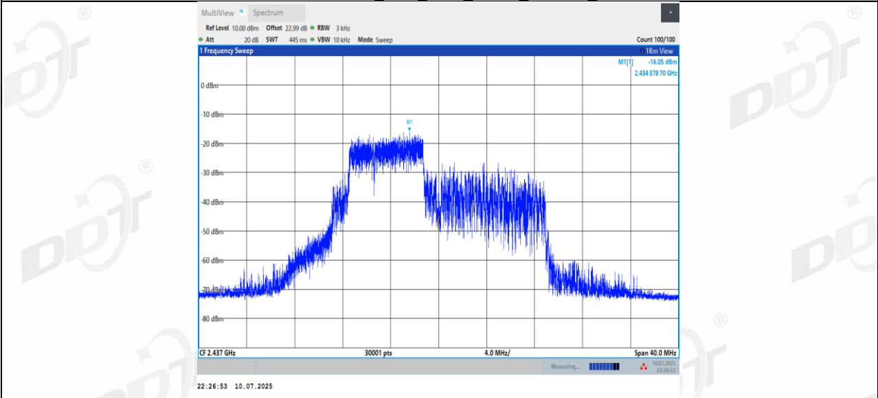
11BE20MIMO_Ant1_2437_52+26_OFDMA_2
