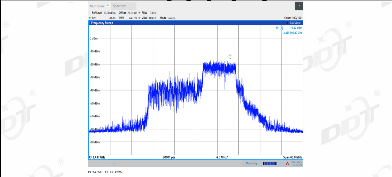
11BE20MIMO_Ant2_2437_106+26_OFDMA_1
