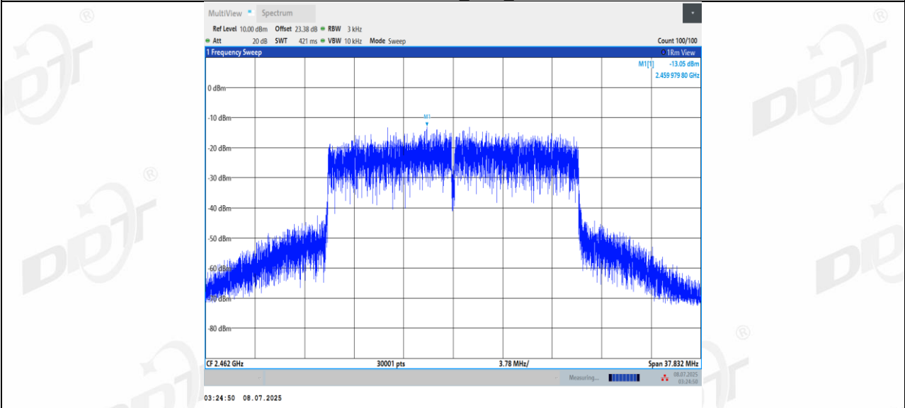
11BE20MIMO Ant2 2462
