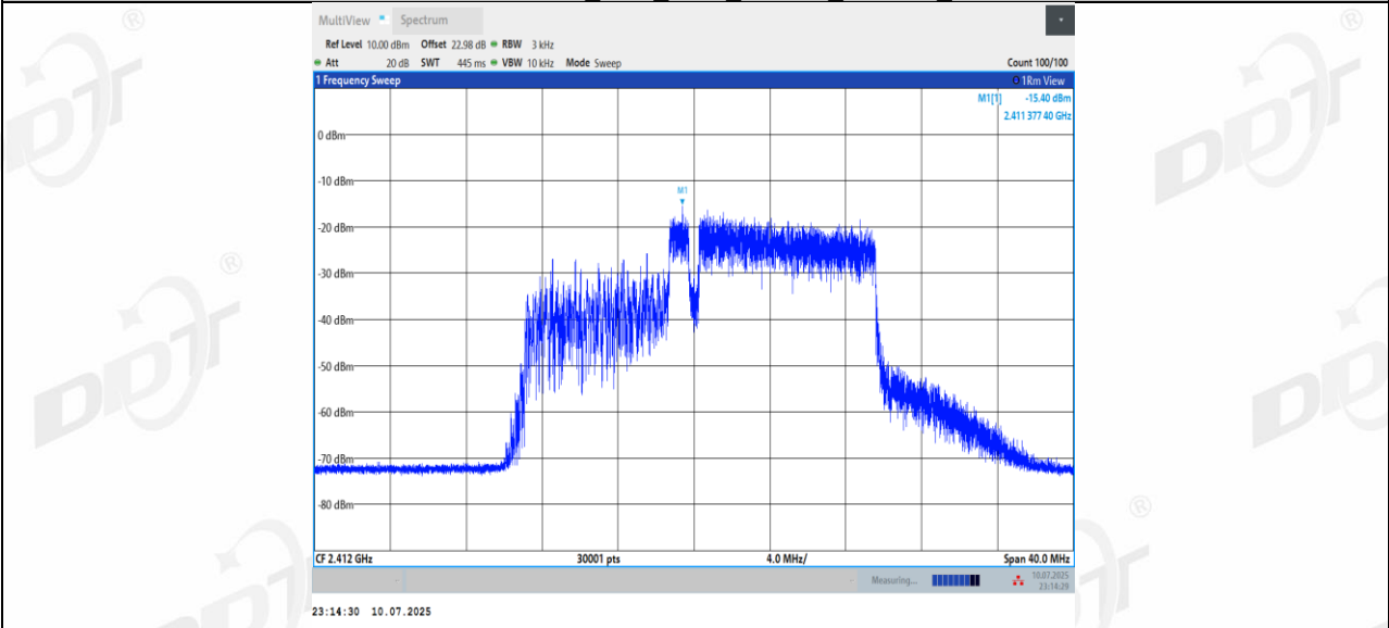
11BE20MIMO_Ant2_2412_52+26_OFDMA_1
