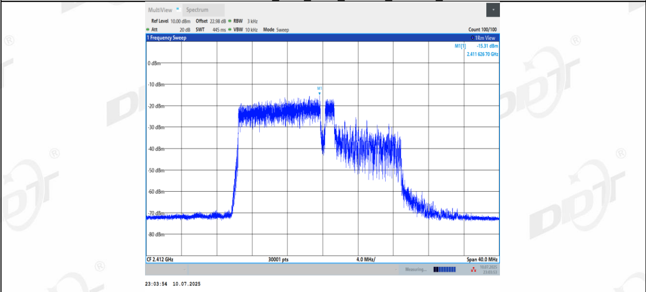
11BE20MIMO_Ant2_2412_106+26_OFDMA_2
