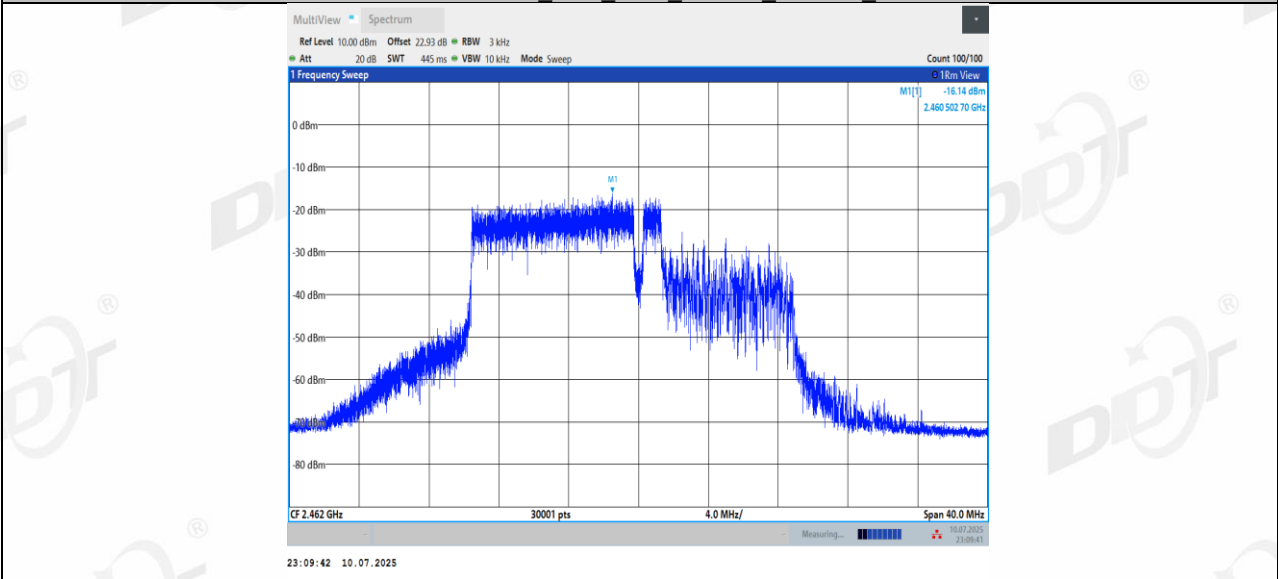
11BE20MIMO_Ant1_2462_106+26_OFDMA_2
