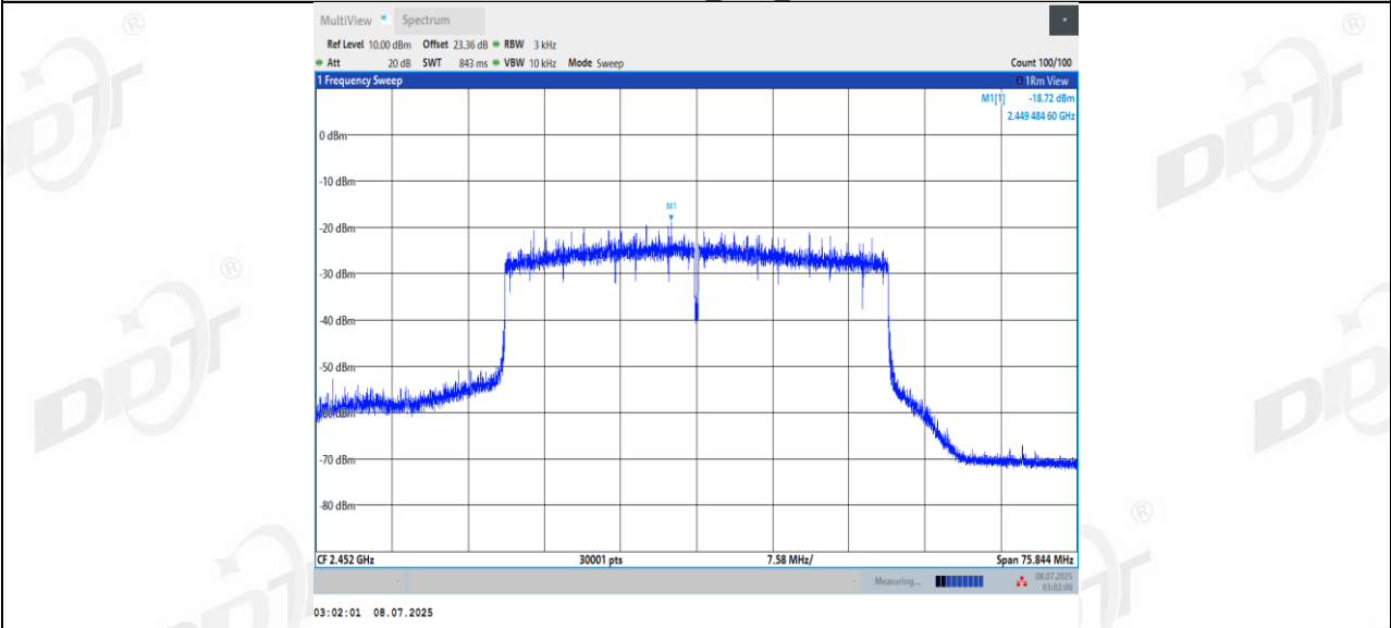
11AX40MIMO Ant2 2452
