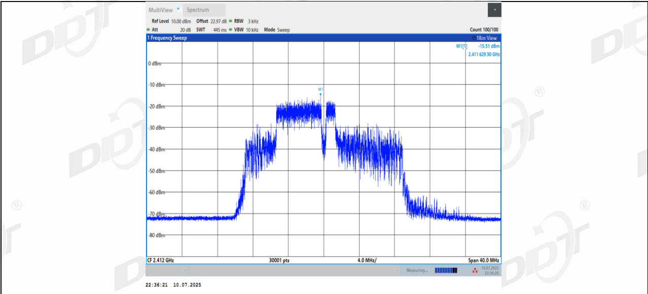
11BE20MIMO_Ant2_2412_52+26_OFDMA_3
