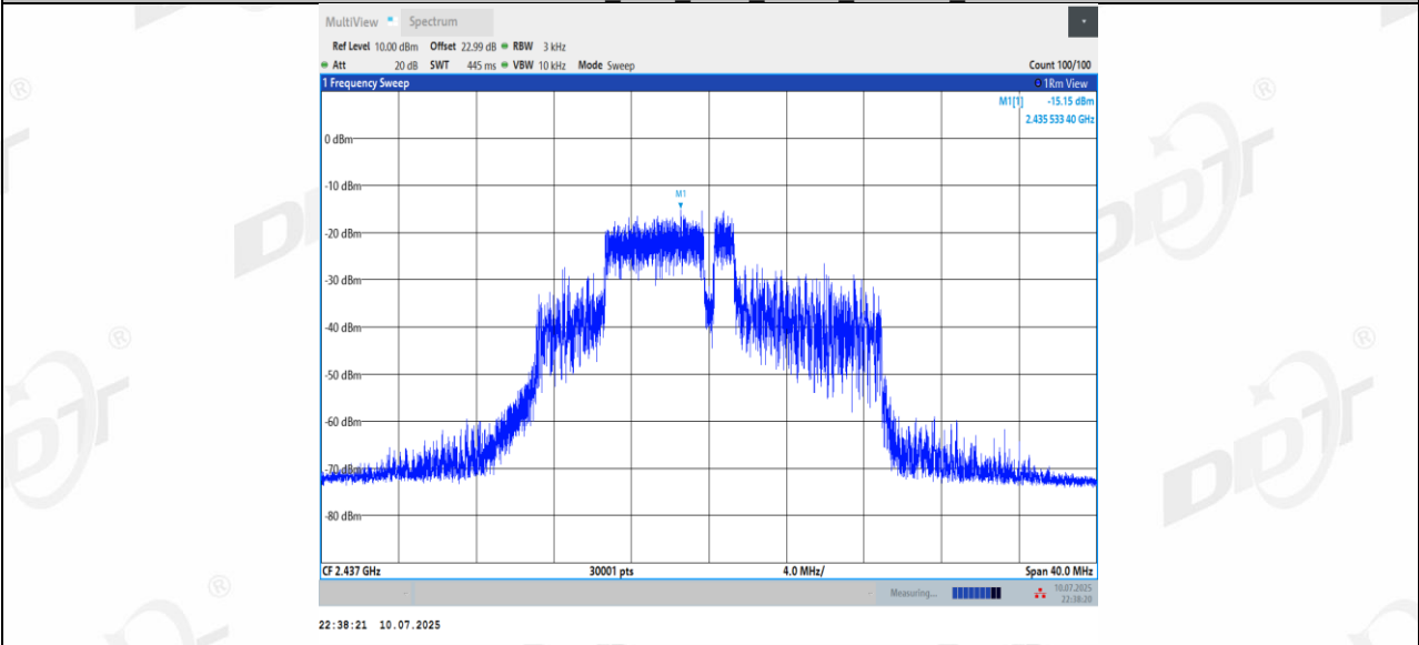
11BE20MIMO_Ant1_2437_52+26_OFDMA_3
