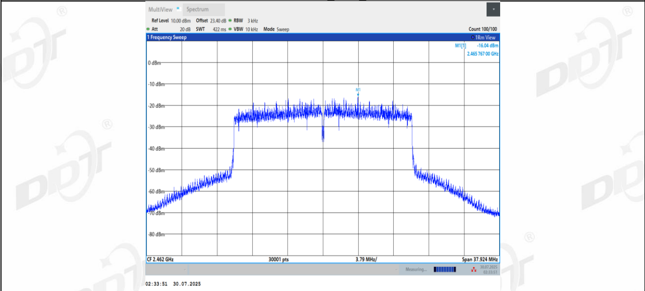
11AX20MIMO Ant2 2462
