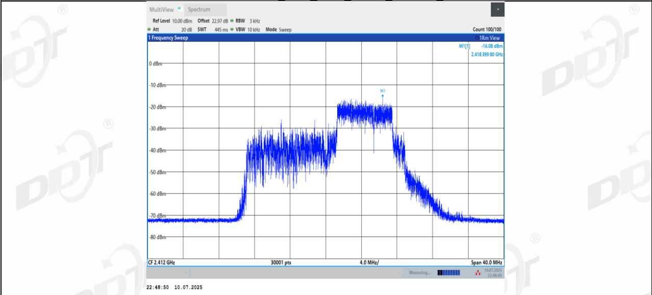
11BE20MIMO_Ant2_2412_106+26_OFDMA_1
