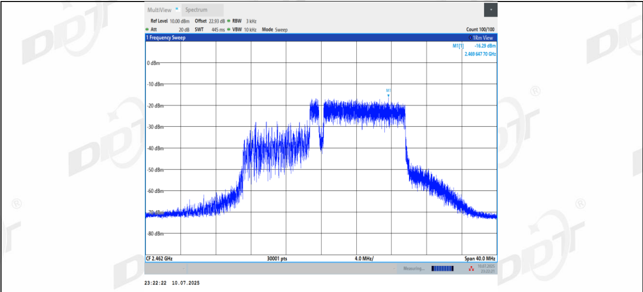
11BE20MIMO_Ant2_2462_52+26_OFDMA_1
