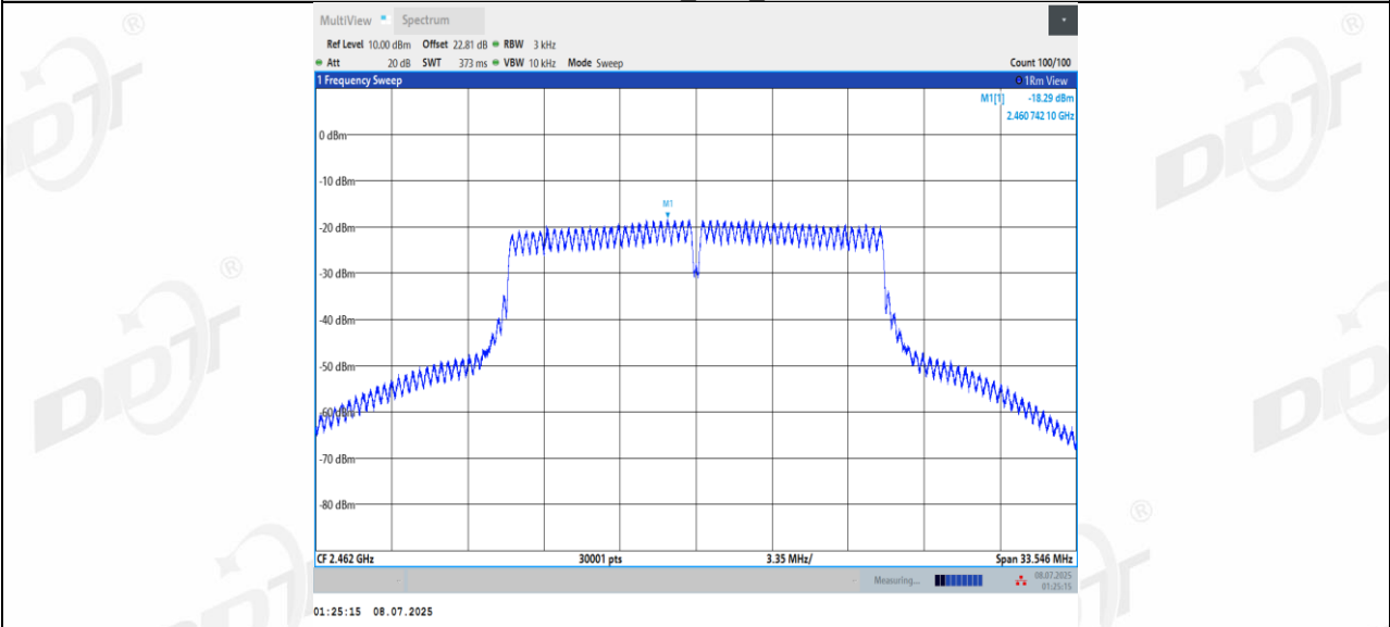
11G-CDD_Ant2_2462
