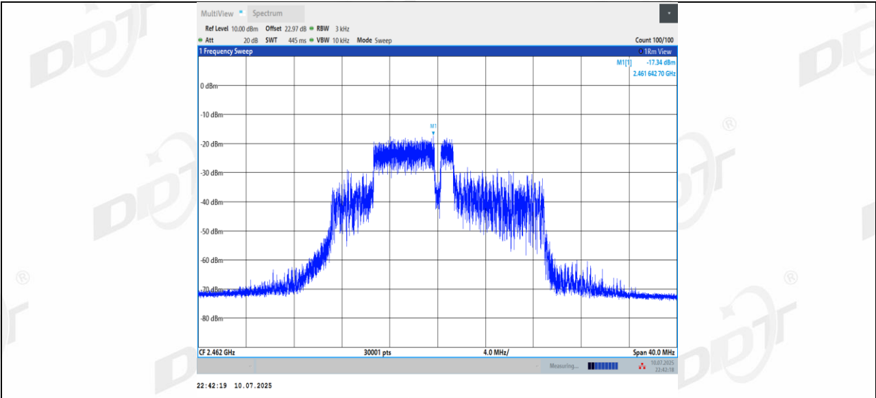
11BE20MIMO_Ant1_2462_52+26_OFDMA_3
