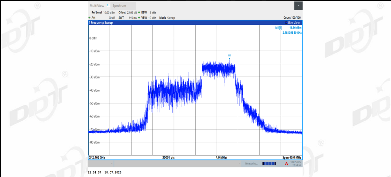
11BE20MIMO_Ant1_2462_106+26_OFDMA_1
