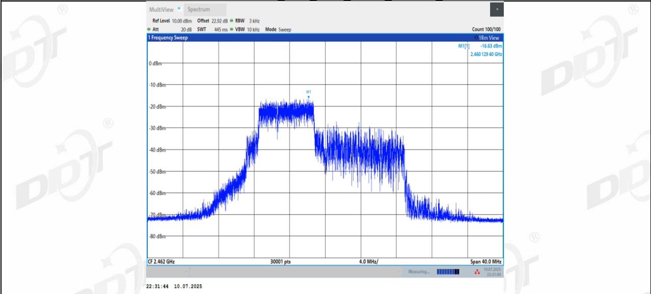
11BE20MIMO_Ant2_2462_52+26_OFDMA_2
