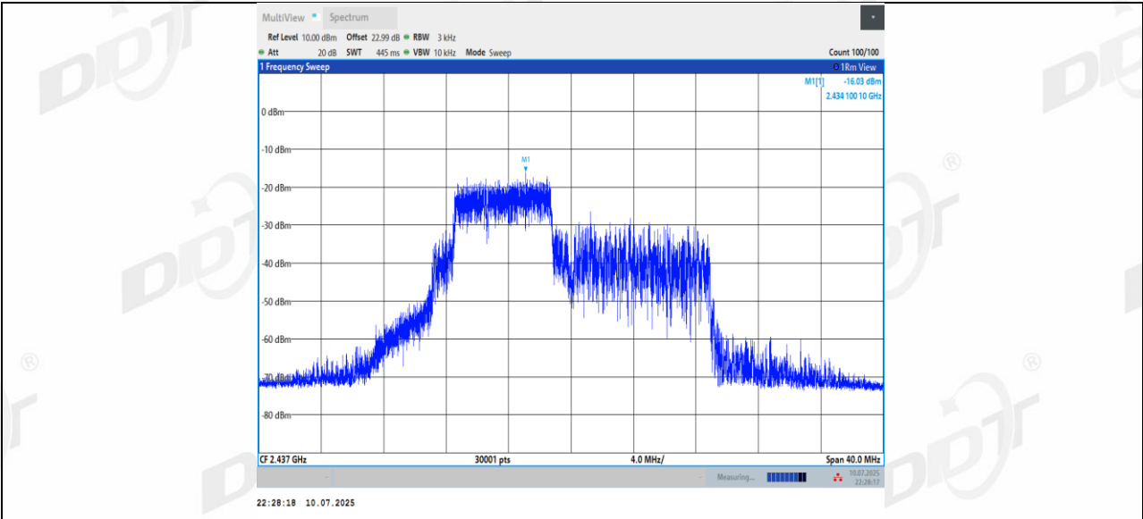
11BE20MIMO_Ant2_2437_52+26_OFDMA_2
