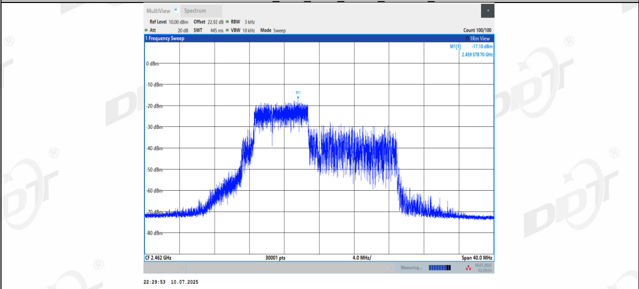
11BE20MIMO Ant1_2462_52+26_OFDMA_2
