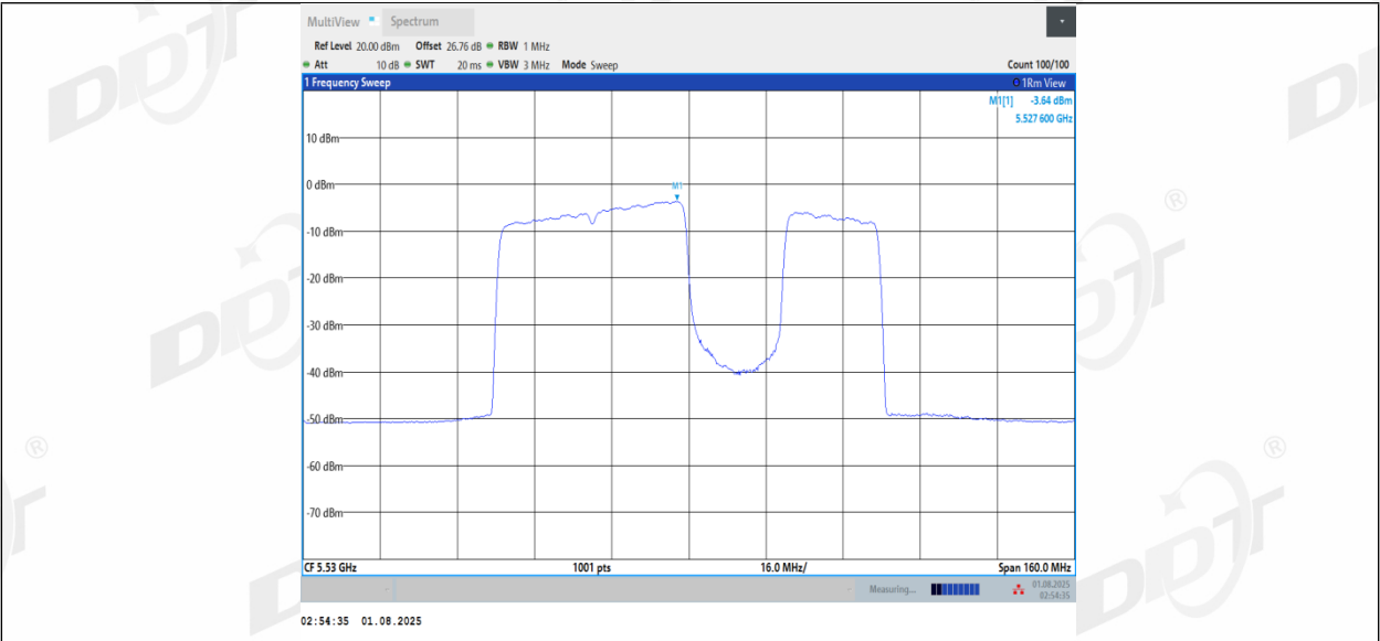
11BE80MIMO_Ant2_5530_484+242_Non-OFDMA_4
