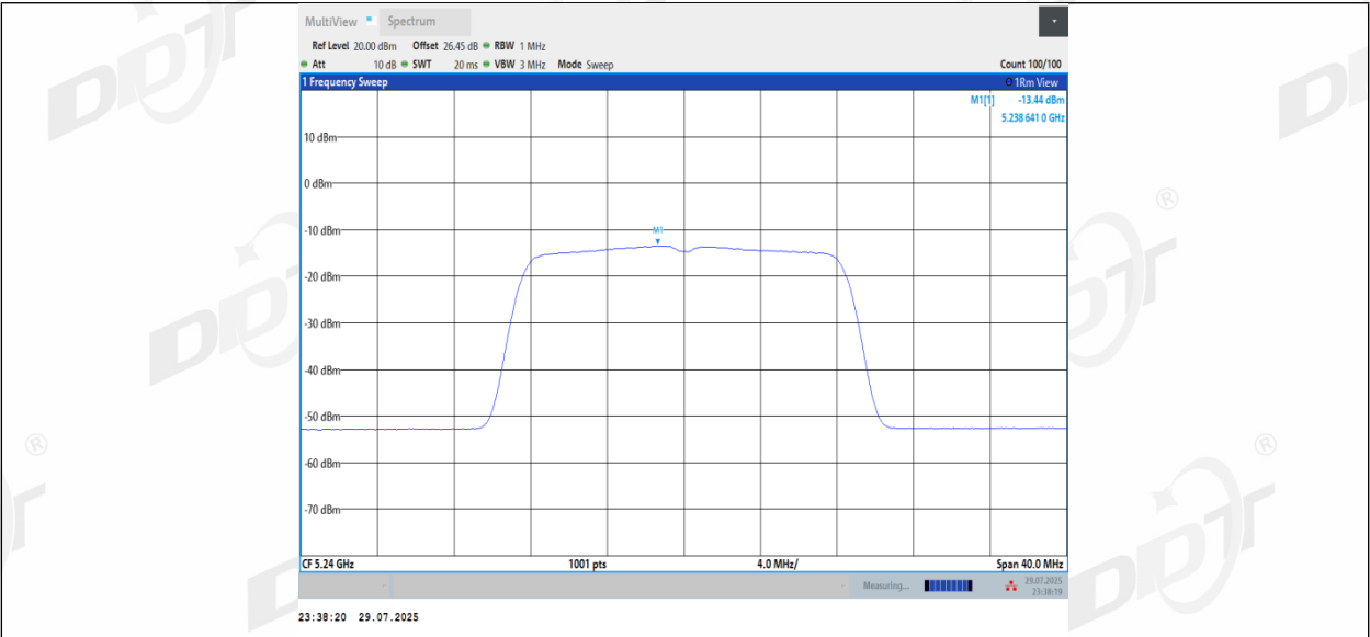
11A-CDD_Ant2_5240
