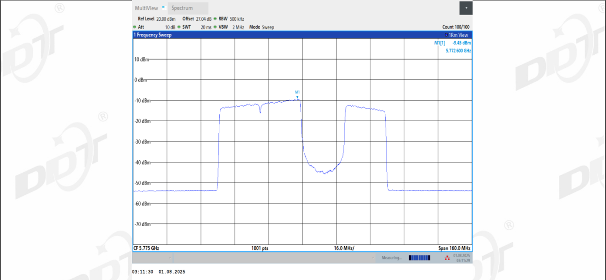
11BE80MIMO_Ant3_5775_484+242_Non-OFDMA_4
