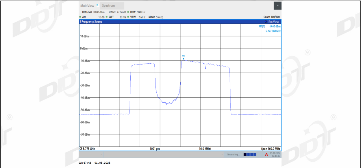
11BE80MIMO_Ant3_5775_484+242_Non-OFDMA_3
