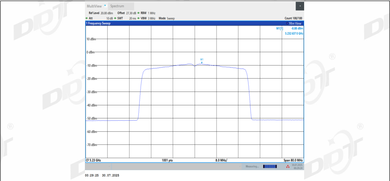
11AX40MIMO_Ant3_5230
