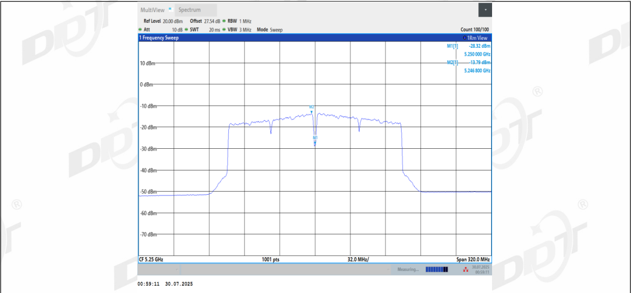
11AC160MIMO_Ant3_5250_UNII-1
