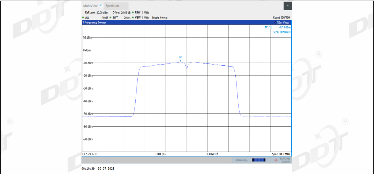
11AC40MIMO_Ant3_5230
