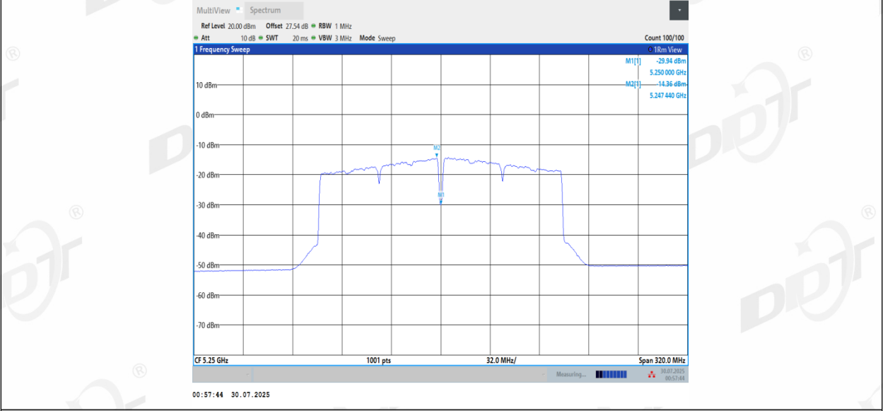
11AC160MIMO_Ant2_5250_UNII-1
