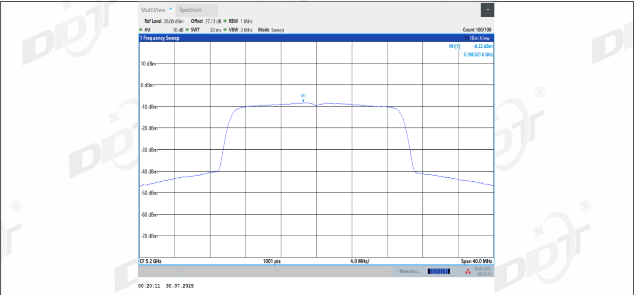
11AX20MIMO_Ant3_5200
