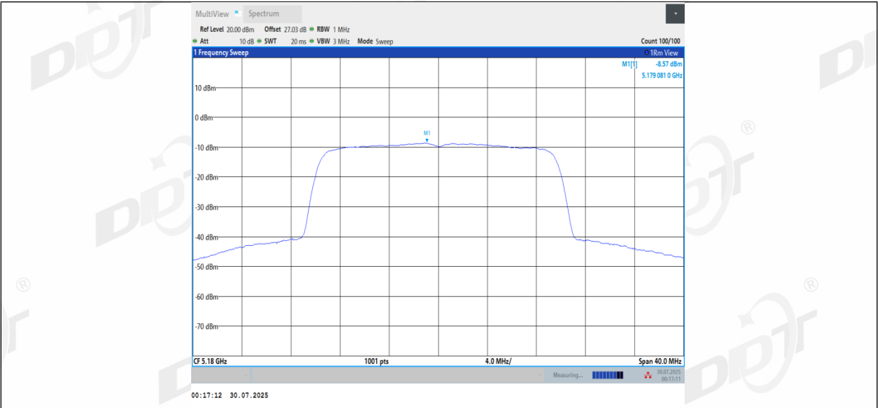
11AX20MIMO_Ant3_5180
