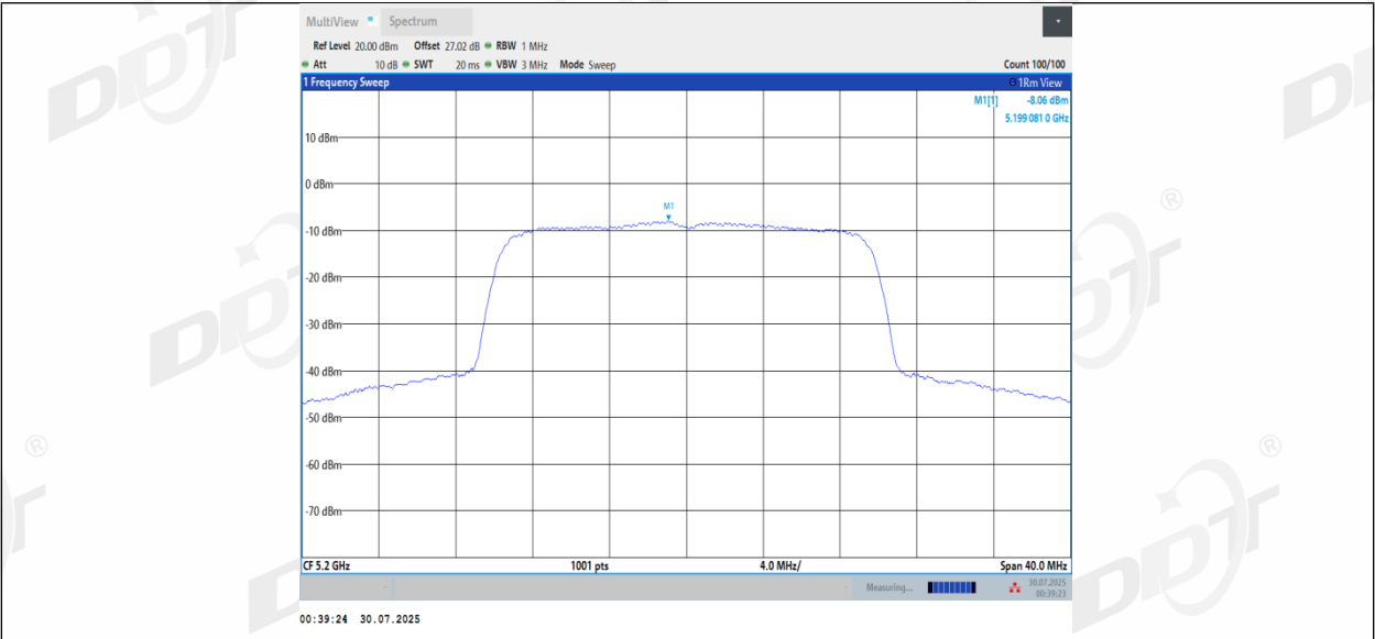
11BE20MIMO_Ant3_5200
