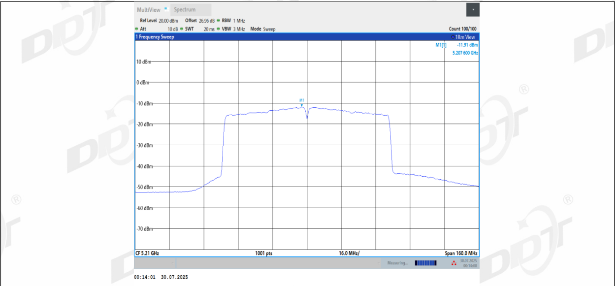
11AC80MIMO_Ant3_5210
