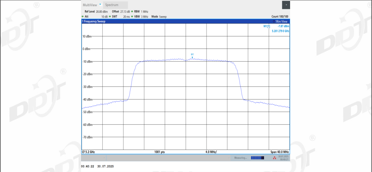
11BE20MIMO_Ant1_5240
