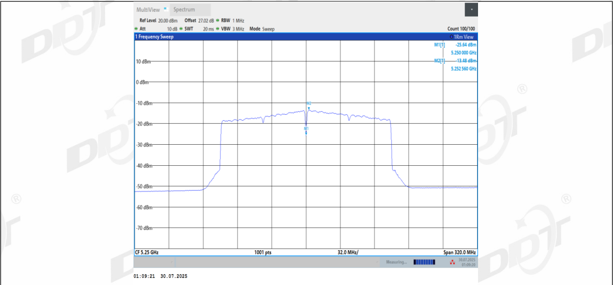
11BE160MIMO_Ant3_5250_UNII-2A
