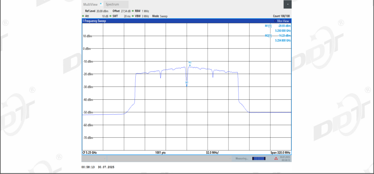
11AC160MIMO_Ant2_5250_UNII-2A
