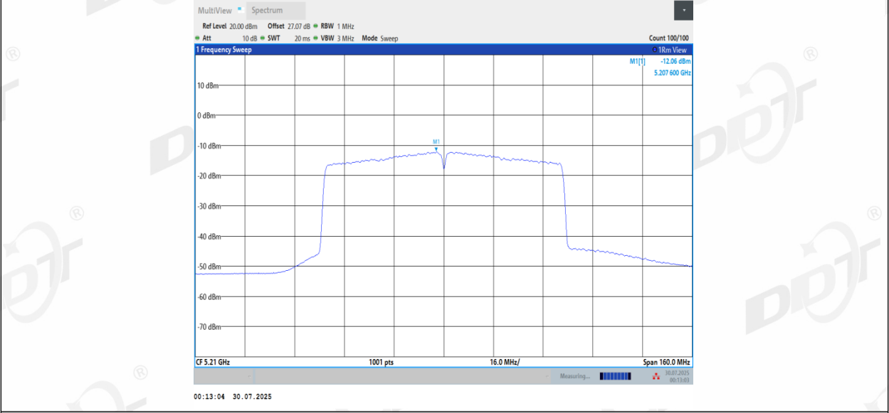
11AC80MIMO_Ant2_5210
