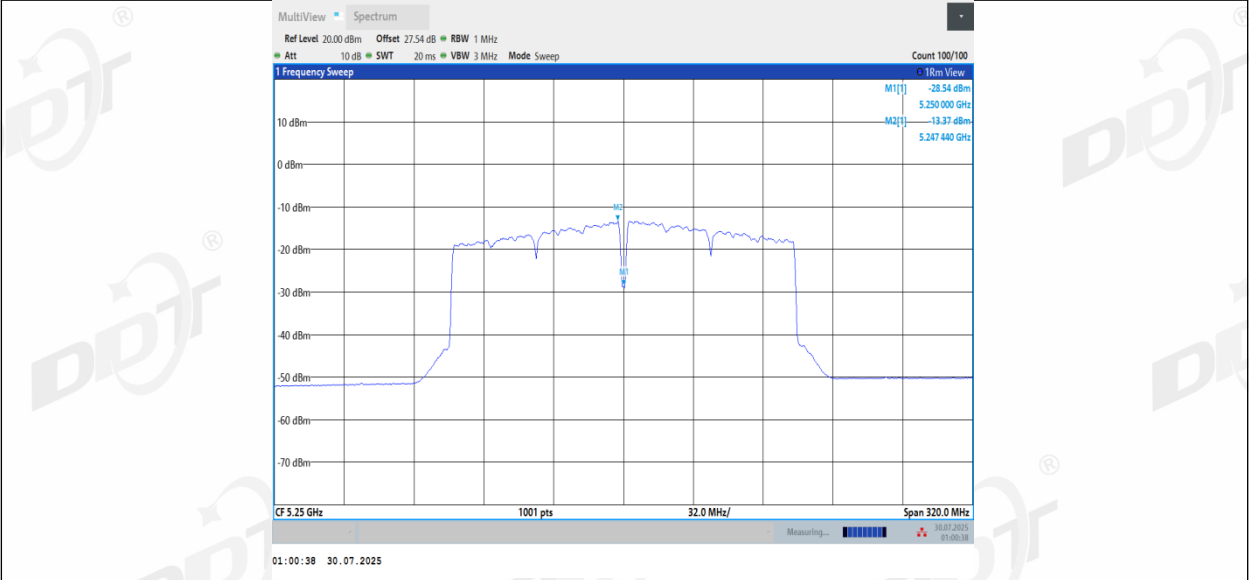
11AC160MIMO_Ant1_5250_UNII-2A
