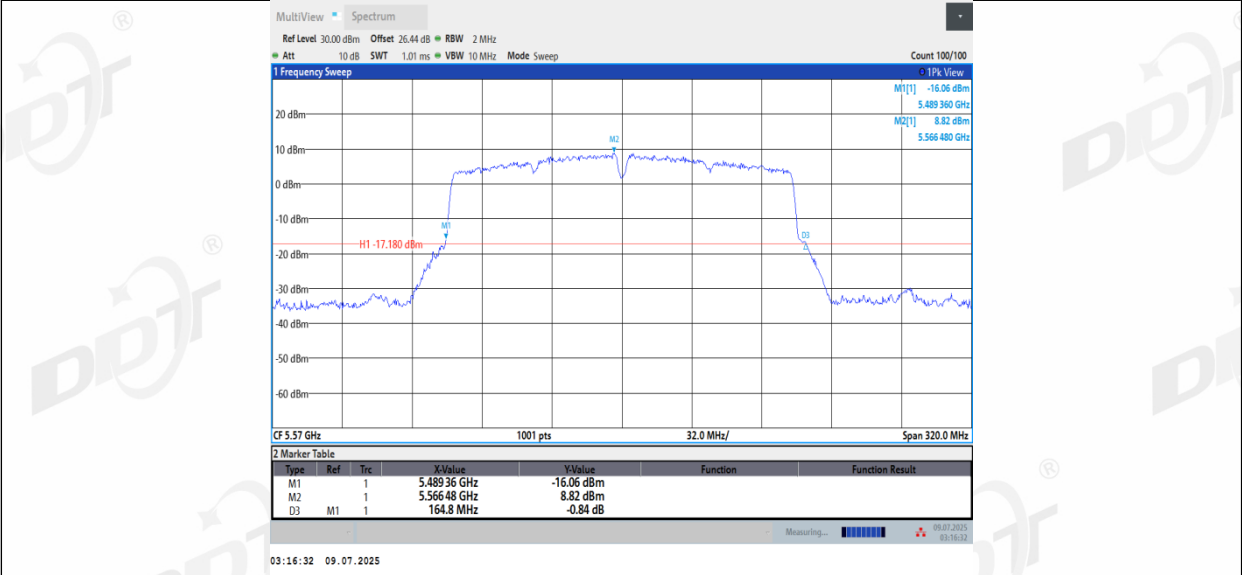
11AC160MIMO_Ant3_5570
