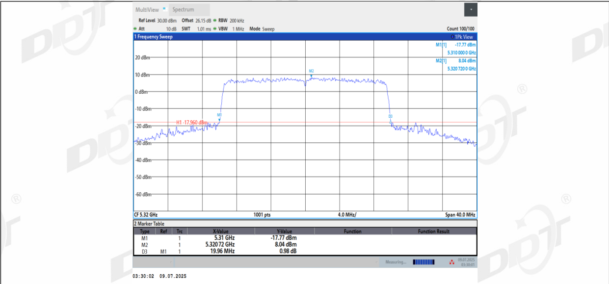
11AX20MIMO_Ant2_5320
