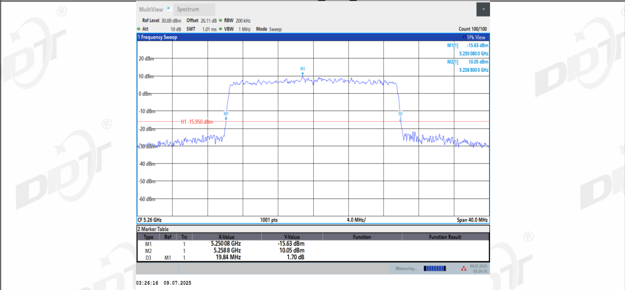
11AX20MIMO_Ant3_5260
