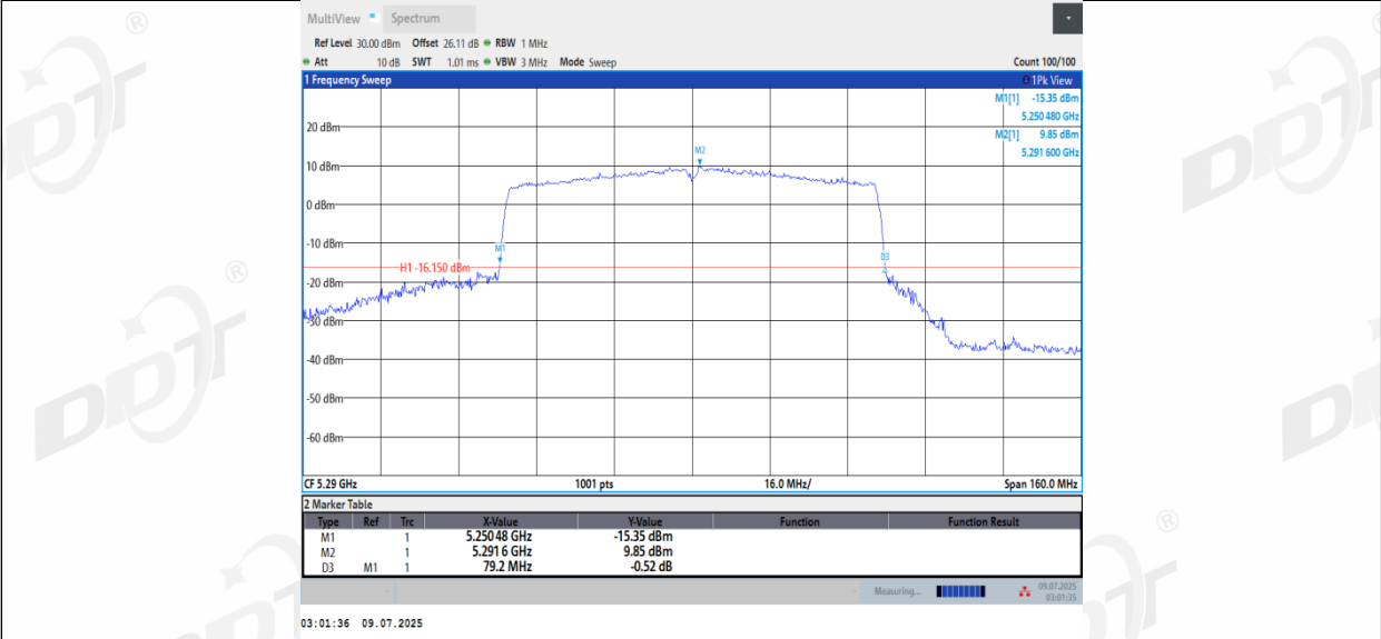
11AC80MIMO_Ant3_5290
