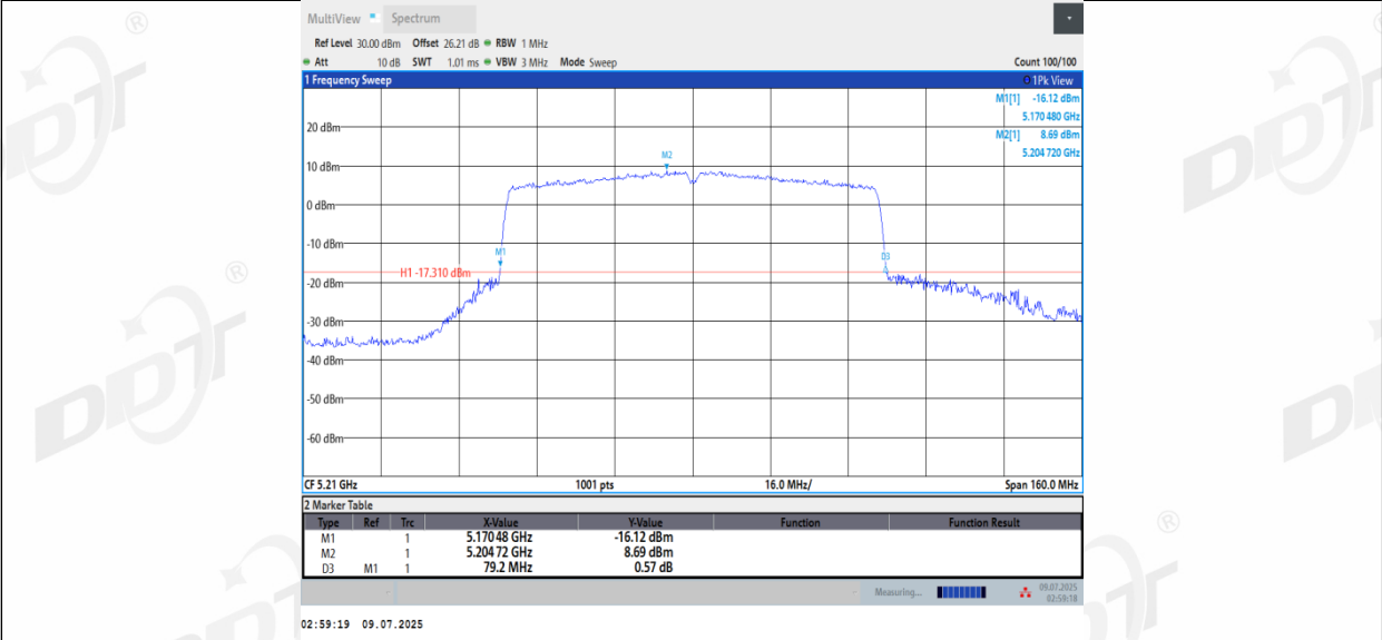
11AC80MIMO_Ant3_5210
