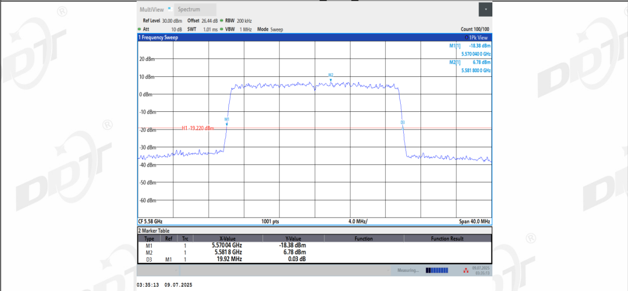
11AX20MIMO_Ant3_5580
