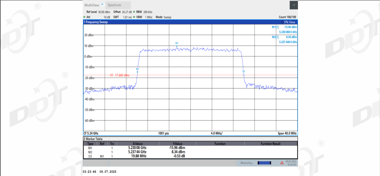
11AX20MIMO_Ant3_5240
