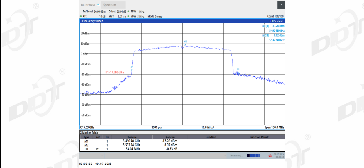
11AC80MIMO_Ant3_5530
