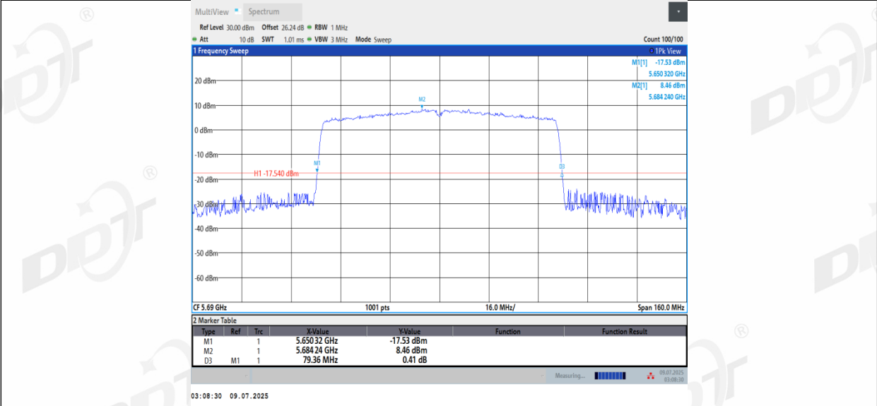
11AC80MIMO_Ant3_5690
