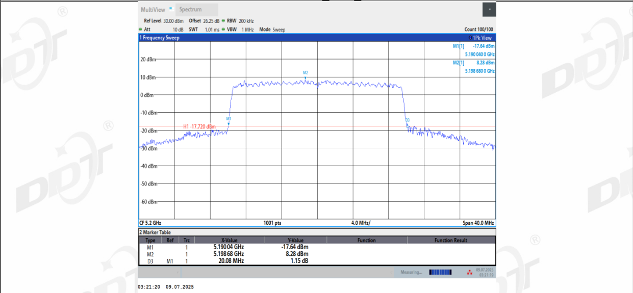
11AX20MIMO_Ant3_5200
