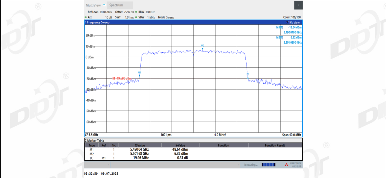
11AX20MIMO_Ant3_5500
