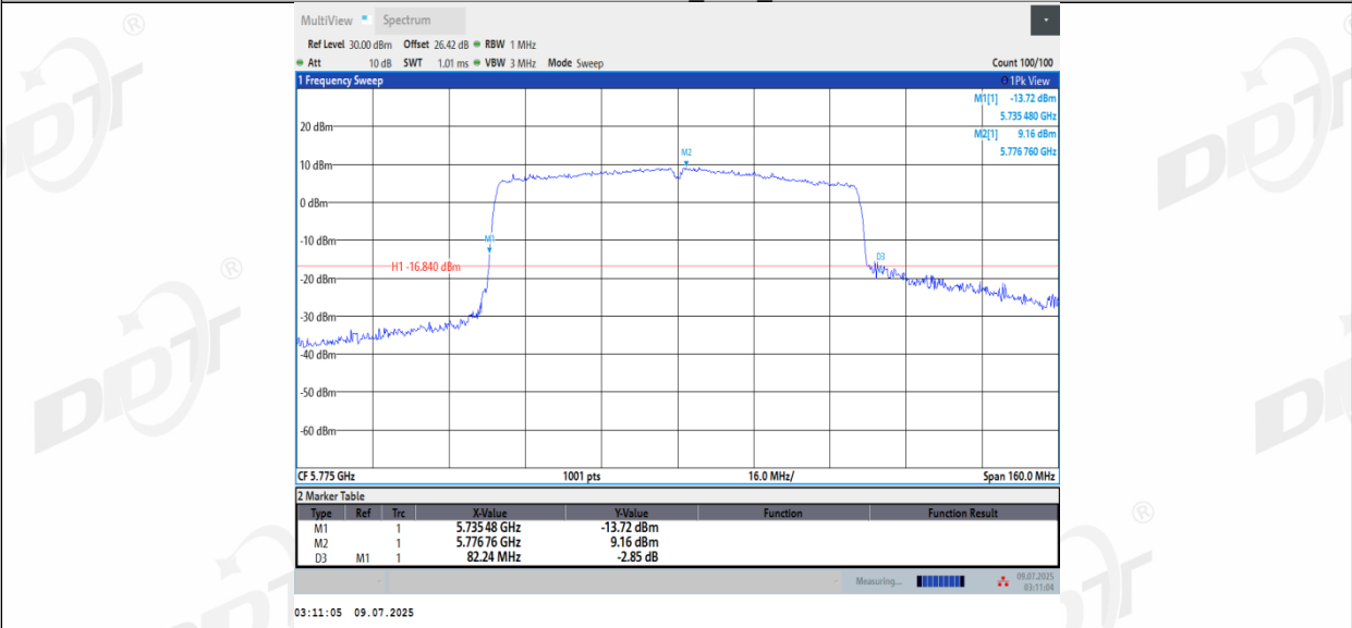
11AC80MIMO_Ant3_5775
