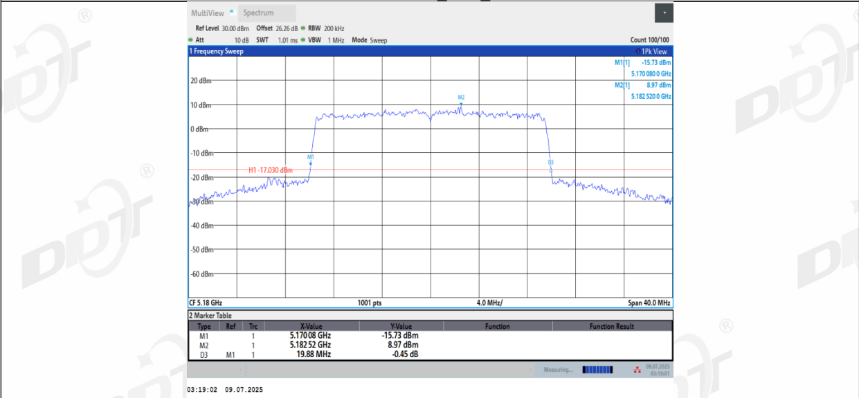
11AX20MIMO_Ant3_5180
