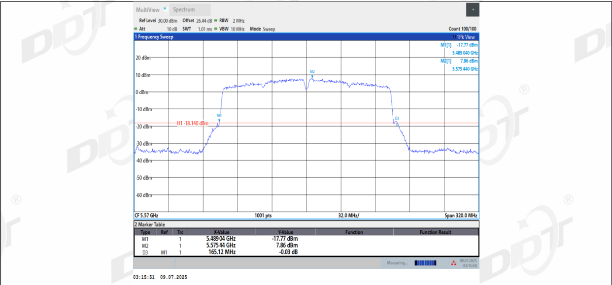
11AC160MIMO_Ant2_5570
