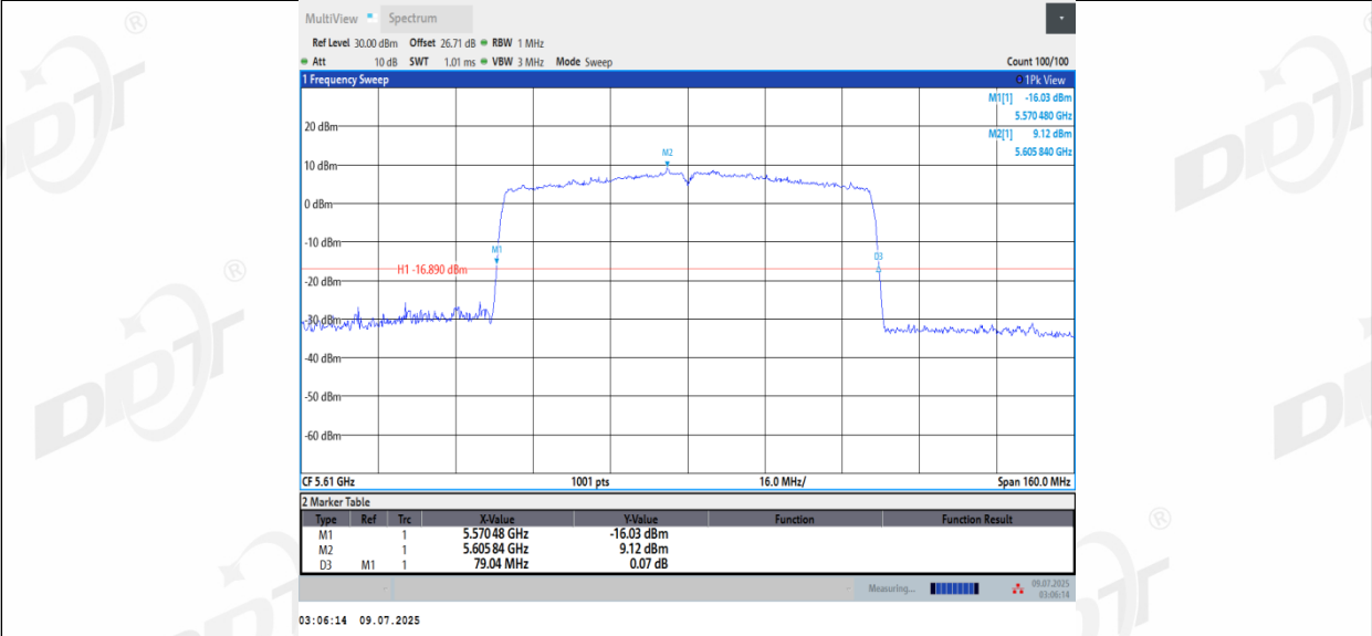
11AC80MIMO_Ant3_5610
