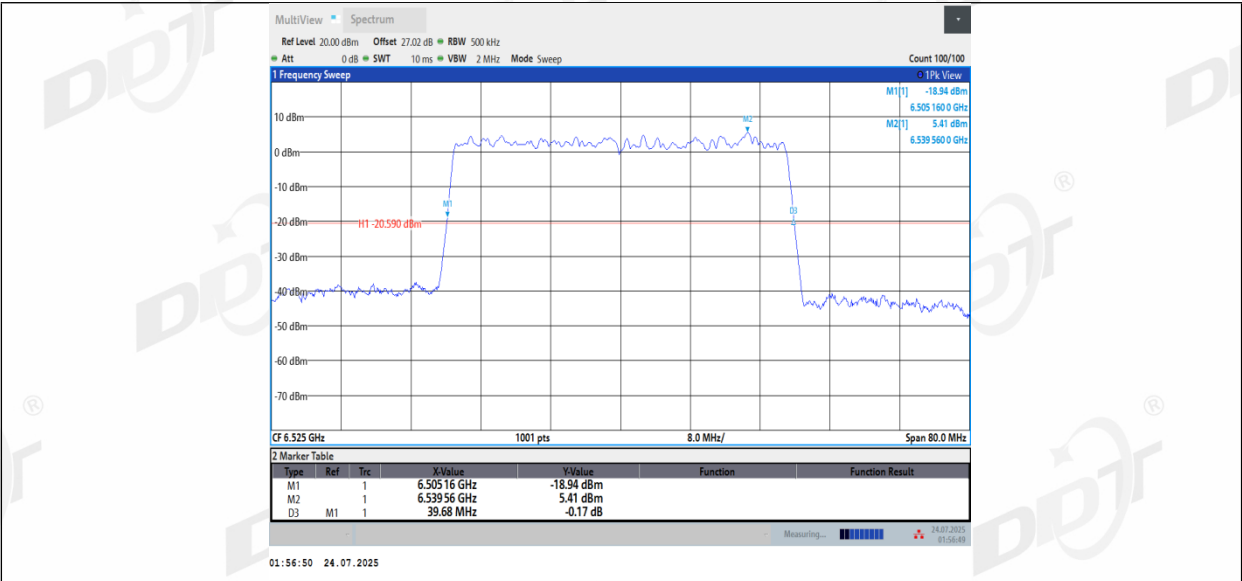
11BE40MIMO_Ant2_6525
