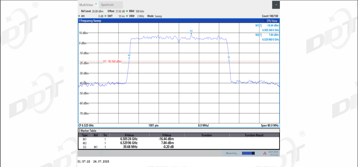
11BE40MIMO_Ant3_6525
