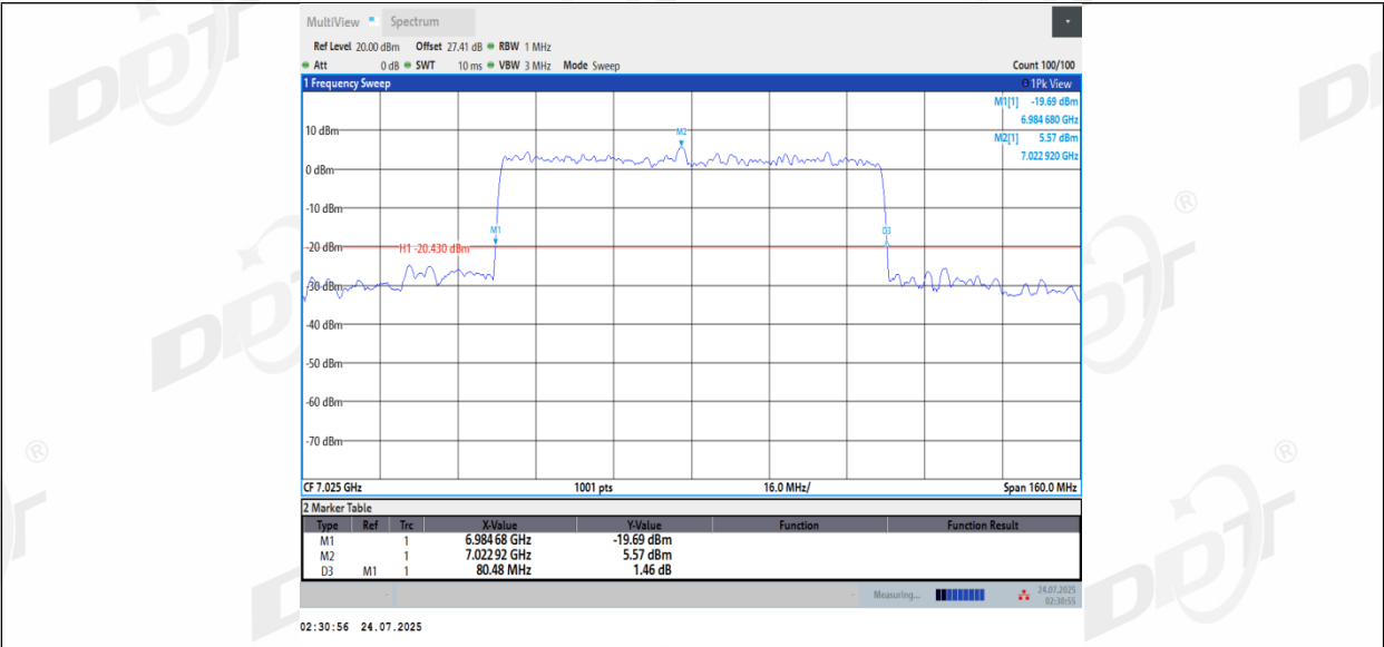
11BE80MIMO_Ant2_7025
