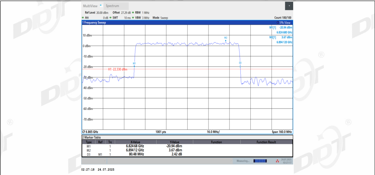
11BE80MIMO_Ant2_6865
