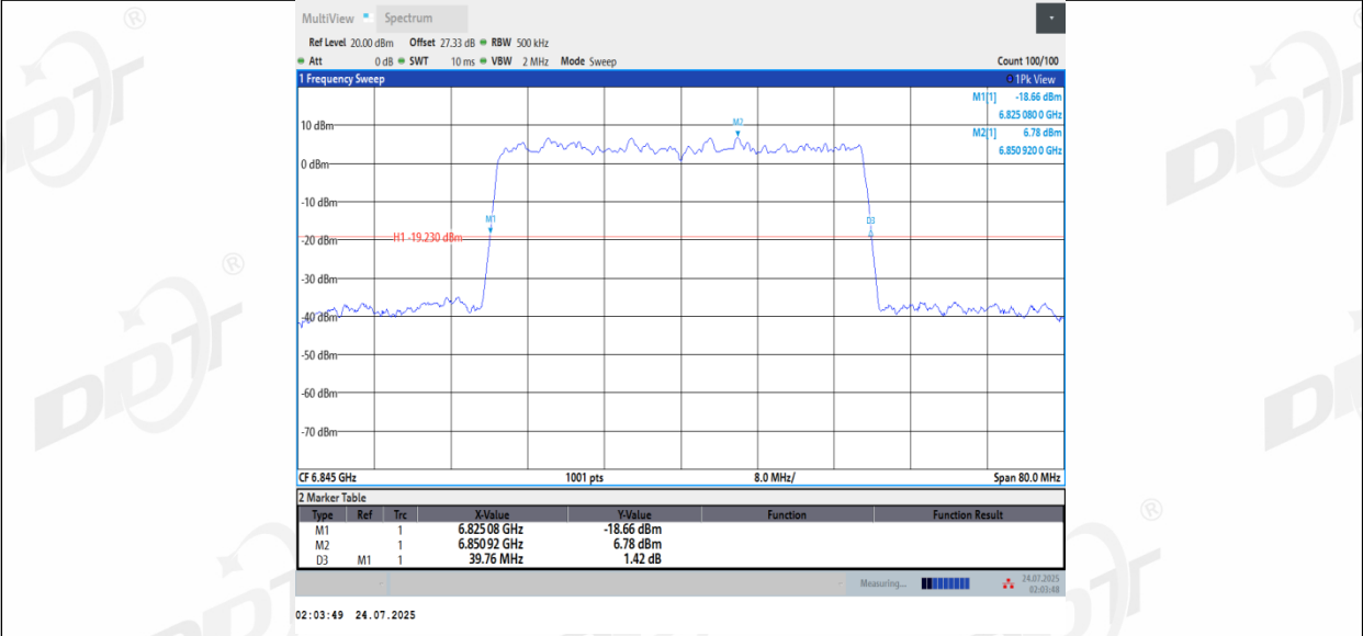
11BE40MIMO_Ant3_6845
