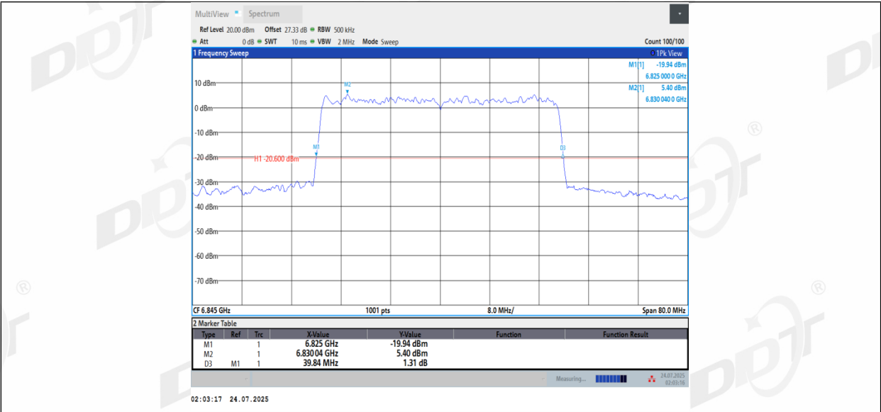
11BE40MIMO_Ant2_6845
