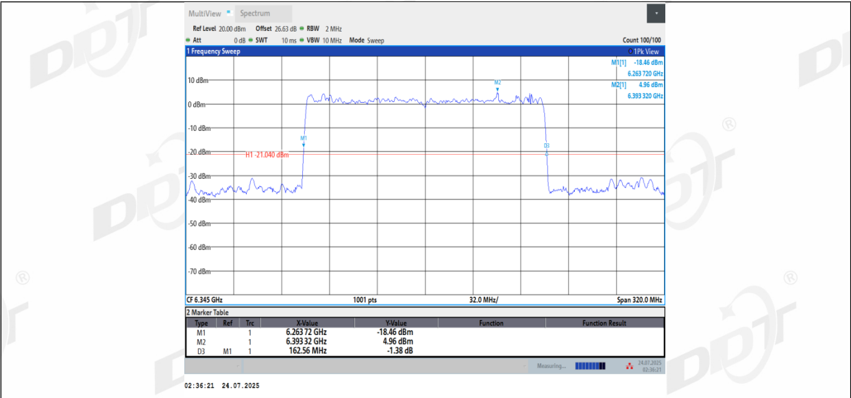
11BE160MIMO_Ant2_6345
