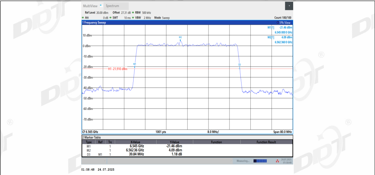
11BE40MIMO_Ant2_6565
