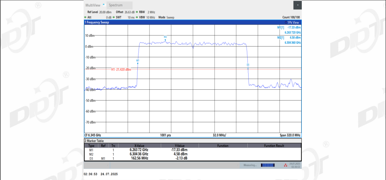
11BE160MIMO_Ant3_6345
