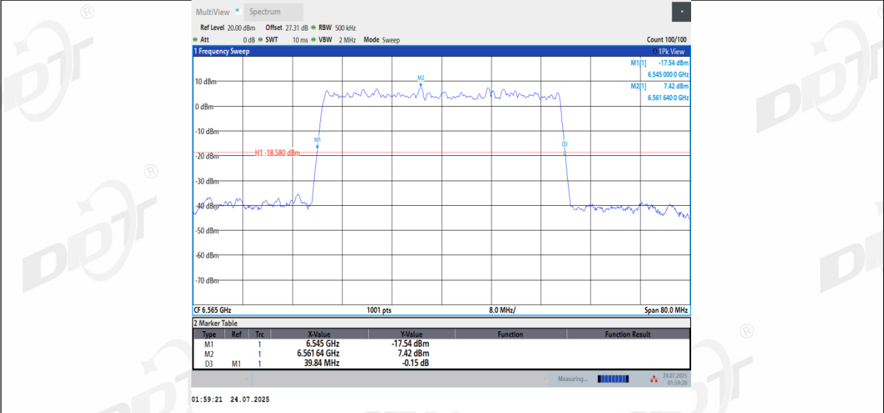
11BE40MIMO_Ant3_6565
