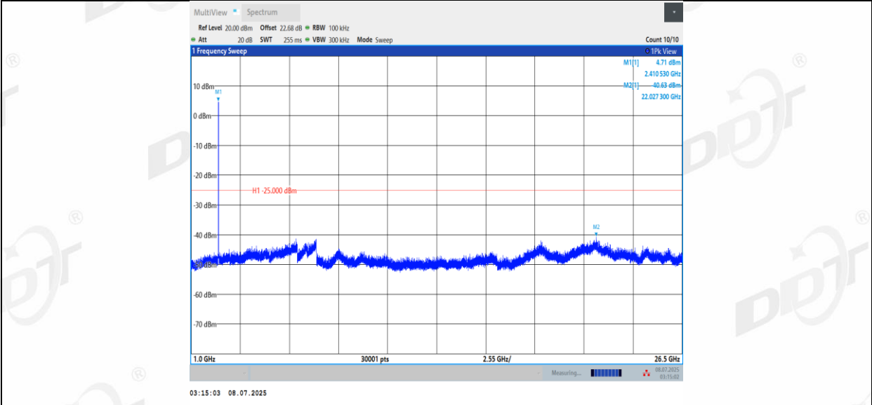
11BE20MIMO_Ant1_2437_0~Reference
