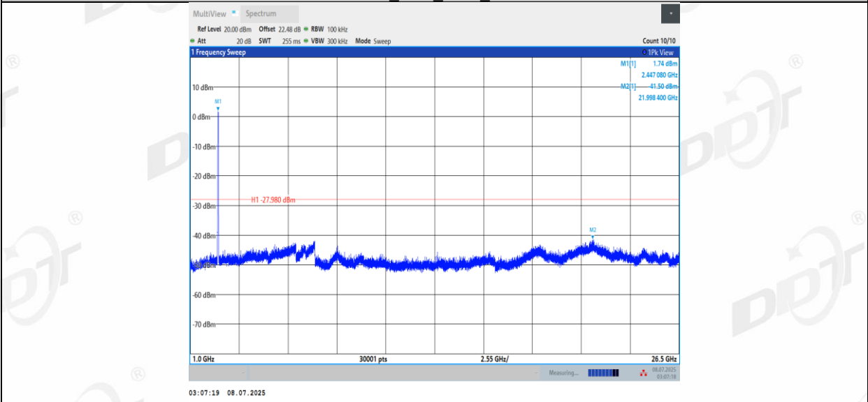
11BE20MIMO_Ant1_2412_0~Reference
