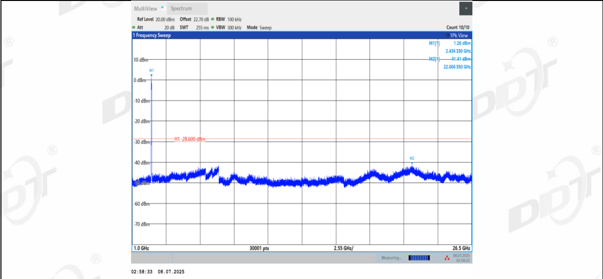
11AX40MIMO_Ant1_2452_0~Reference
