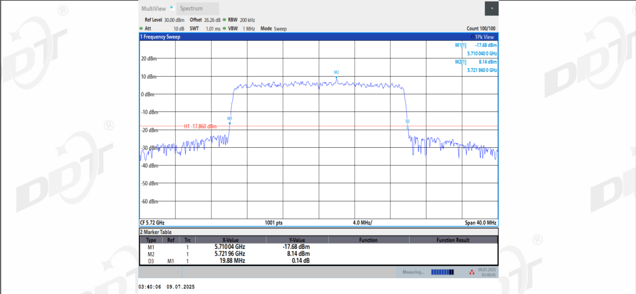
11AX20MIMO_Ant3_5720
