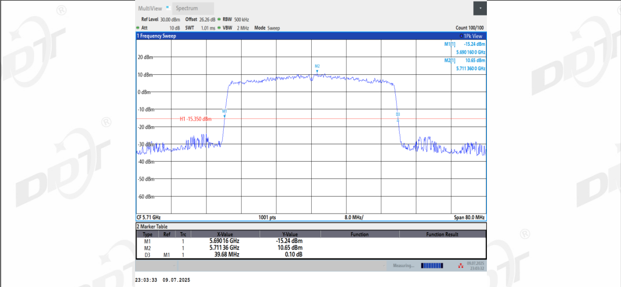
11AX40MIMO_Ant3_5710
