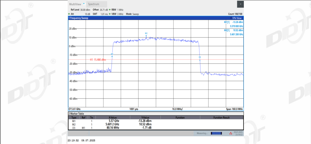
11AX80MIMO_Ant3_5610
