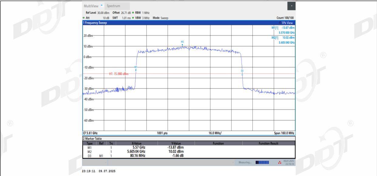
11AX80MIMO_Ant2_5610
