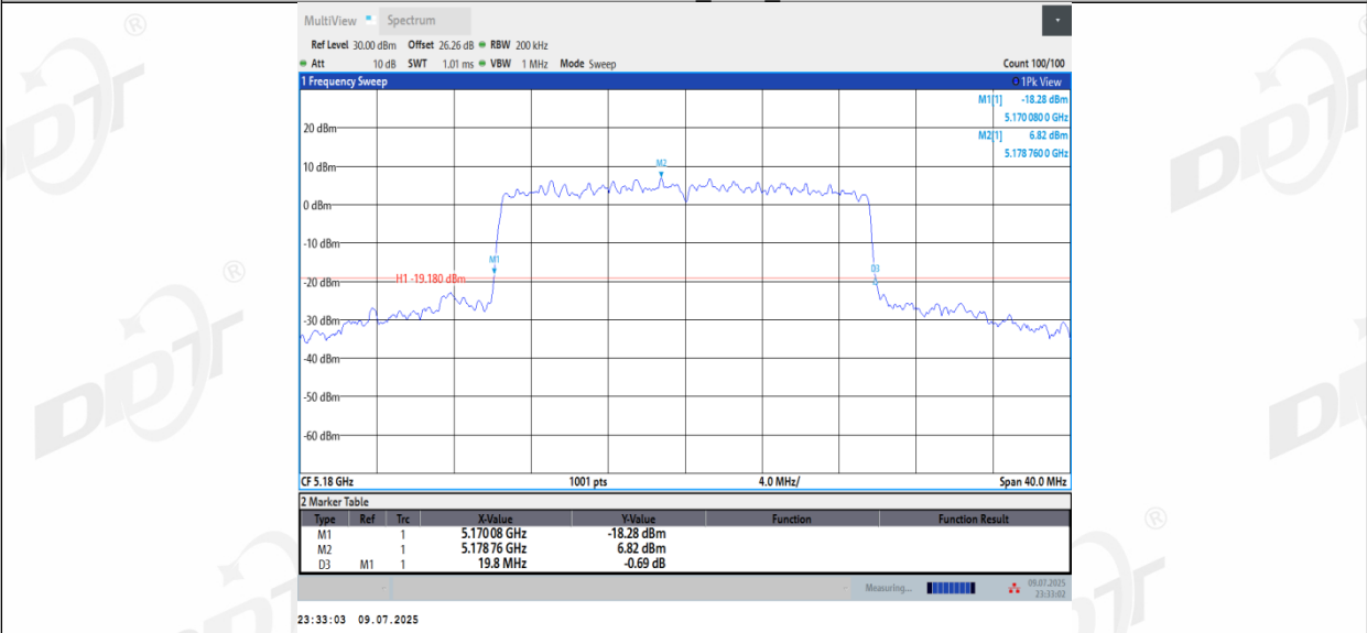
11BE20MIMO_Ant3_5180
