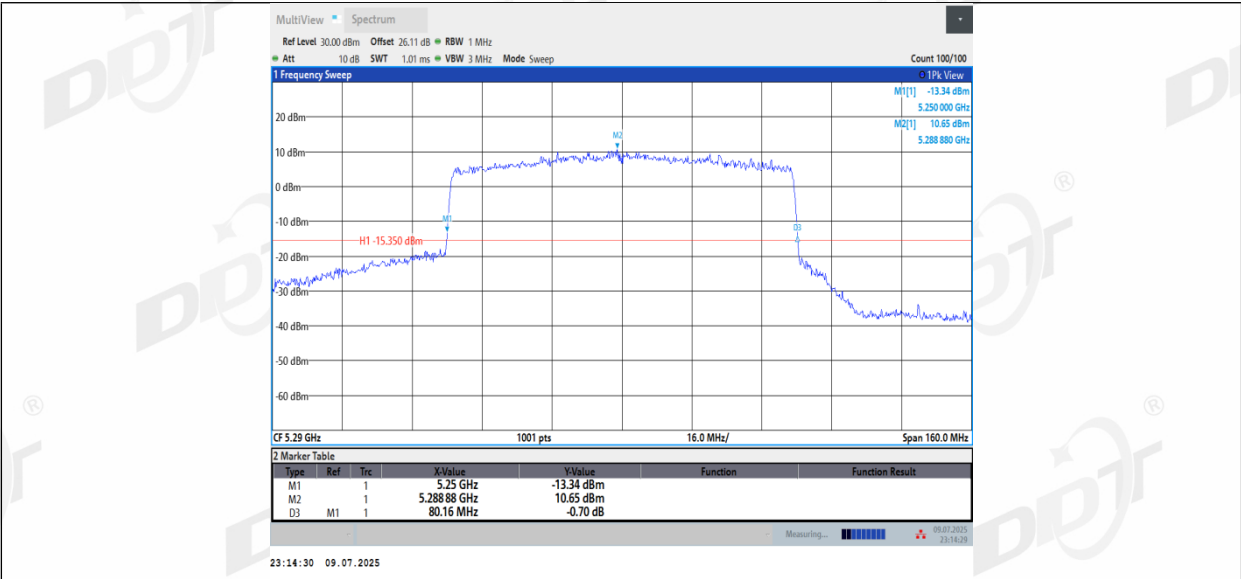
11AX80MIMO_Ant2_5290
