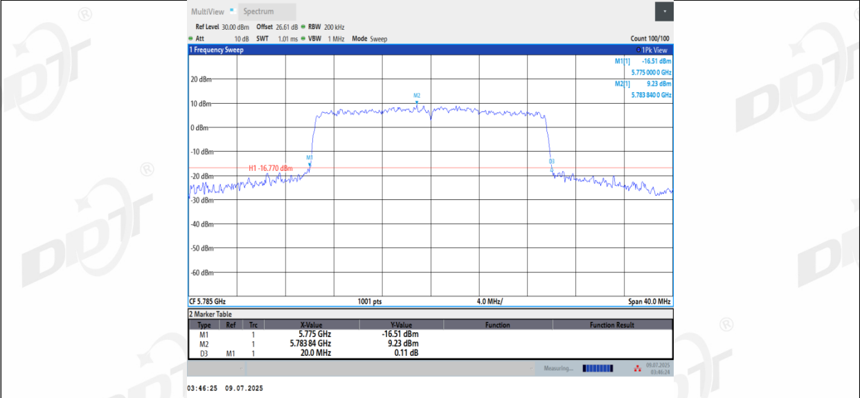
11AX20MIMO_Ant3_5785
