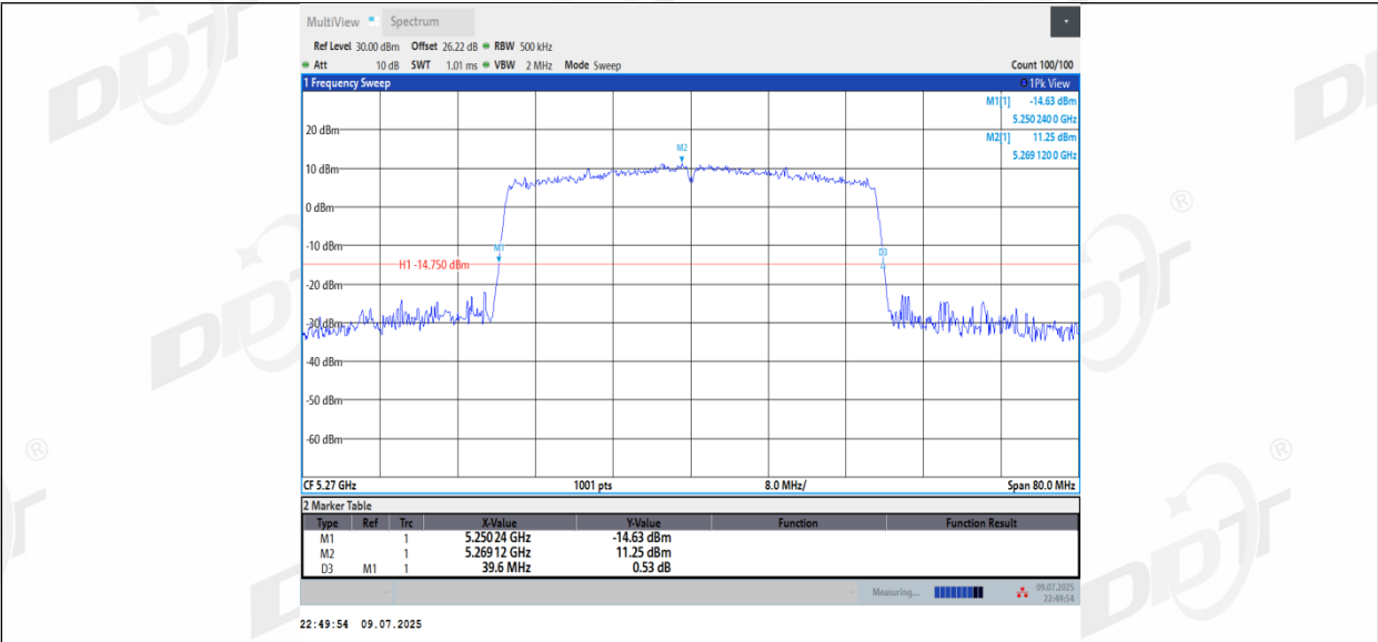
11AX40MIMO_Ant2_5270
