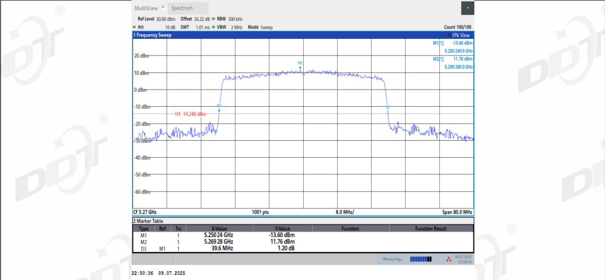
11AX40MIMO_Ant3_5270
