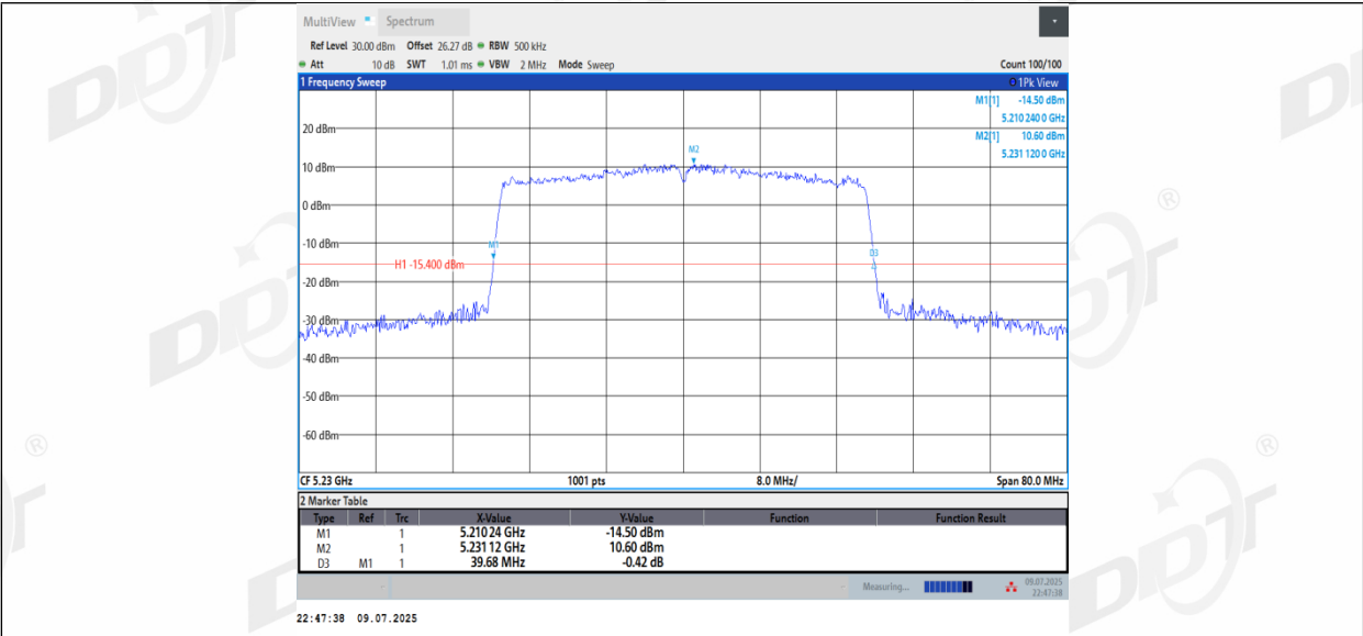
11AX40MIMO_Ant2_5230
