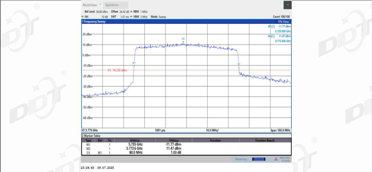
11AX80MIMO_Ant3_5775
