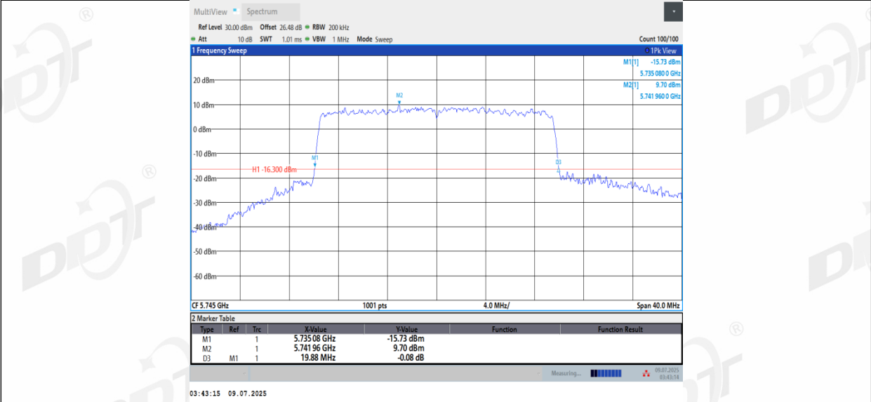
11AX20MIMO_Ant3_5745
