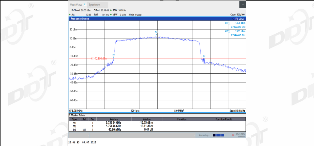
11AX40MIMO_Ant3_5755
