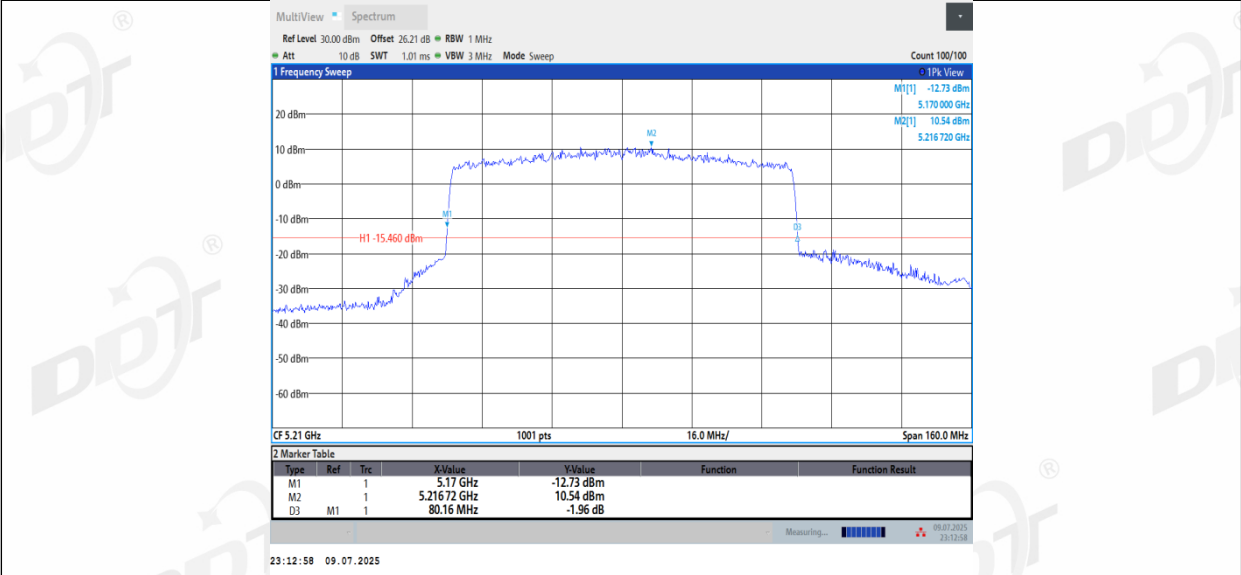
11AX80MIMO_Ant3_5210
