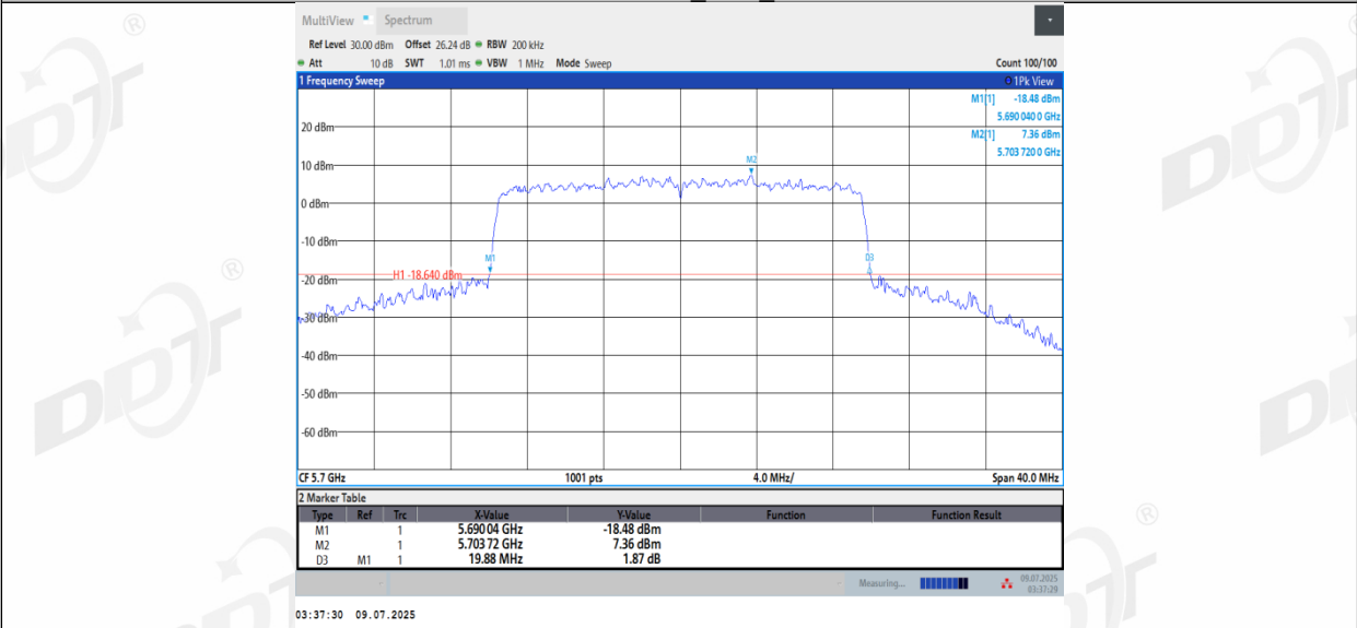
11AX20MIMO_Ant3_5700
