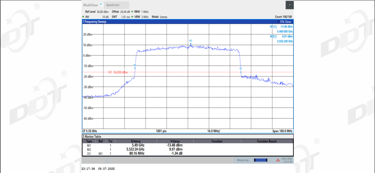
11AX80MIMO_Ant3_5530
