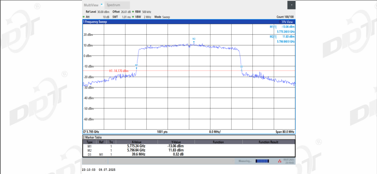
11AX40MIMO_Ant3_5795
