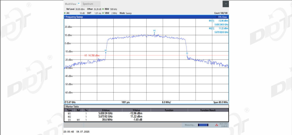
11AX40MIMO_Ant3_5670
