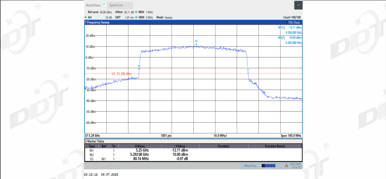
11AX80MIMO_Ant3_5290
