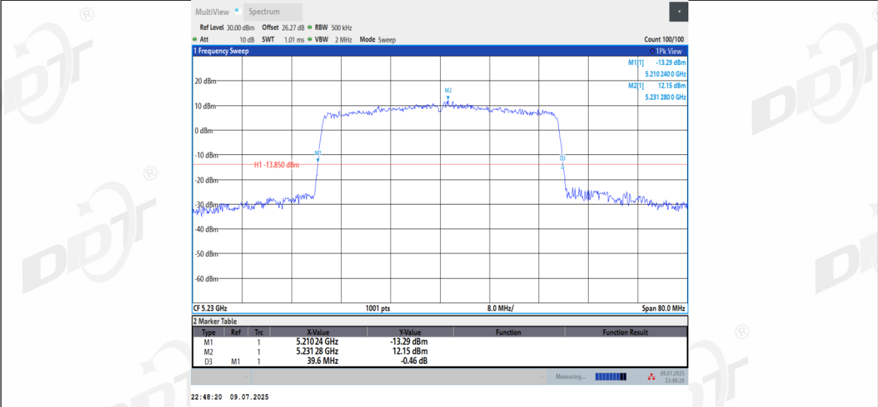
11AX40MIMO_Ant3_5230
