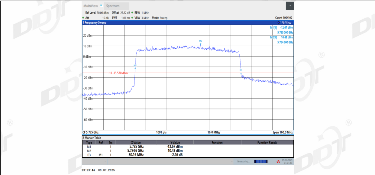
11AX80MIMO_Ant2_5775
