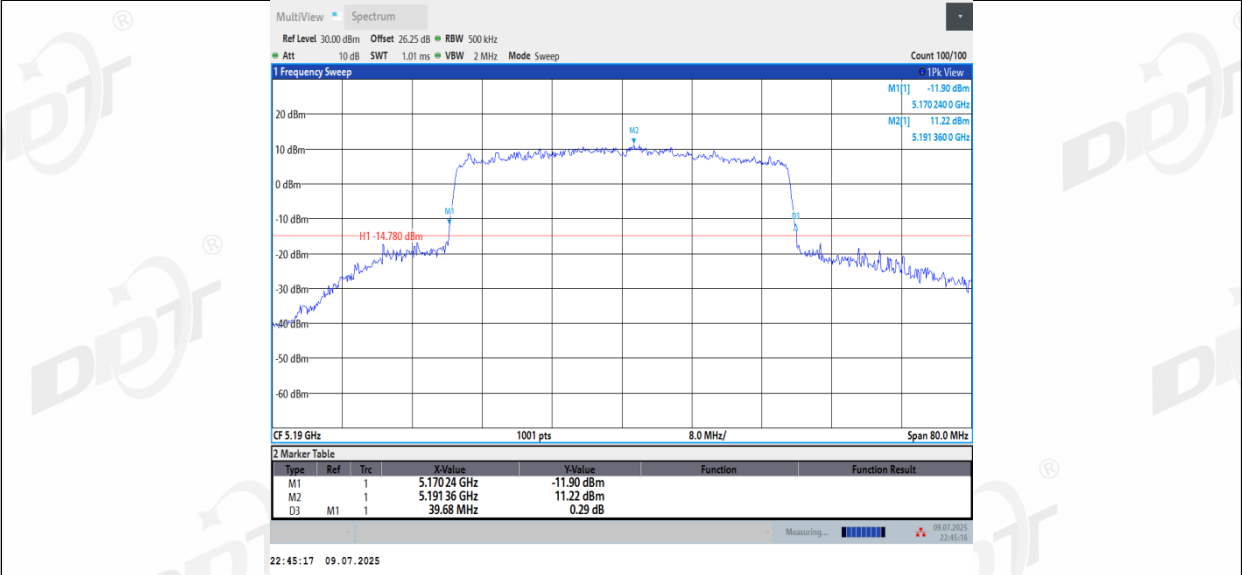
11AX40MIMO_Ant3_5190
