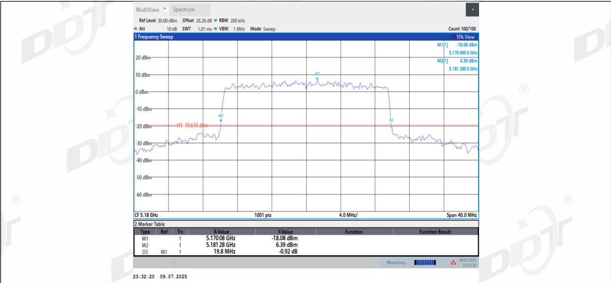
11BE20MIMO_Ant2_5180
