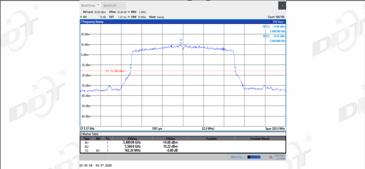
11AX160MIMO_Ant3_5570
