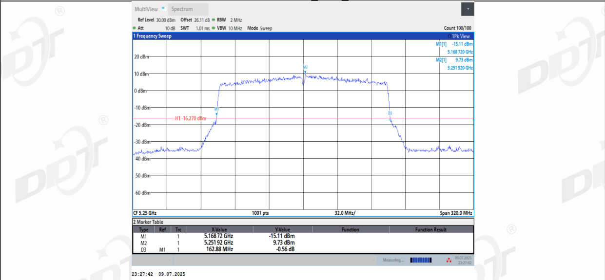
11AX160MIMO_Ant3_5250
