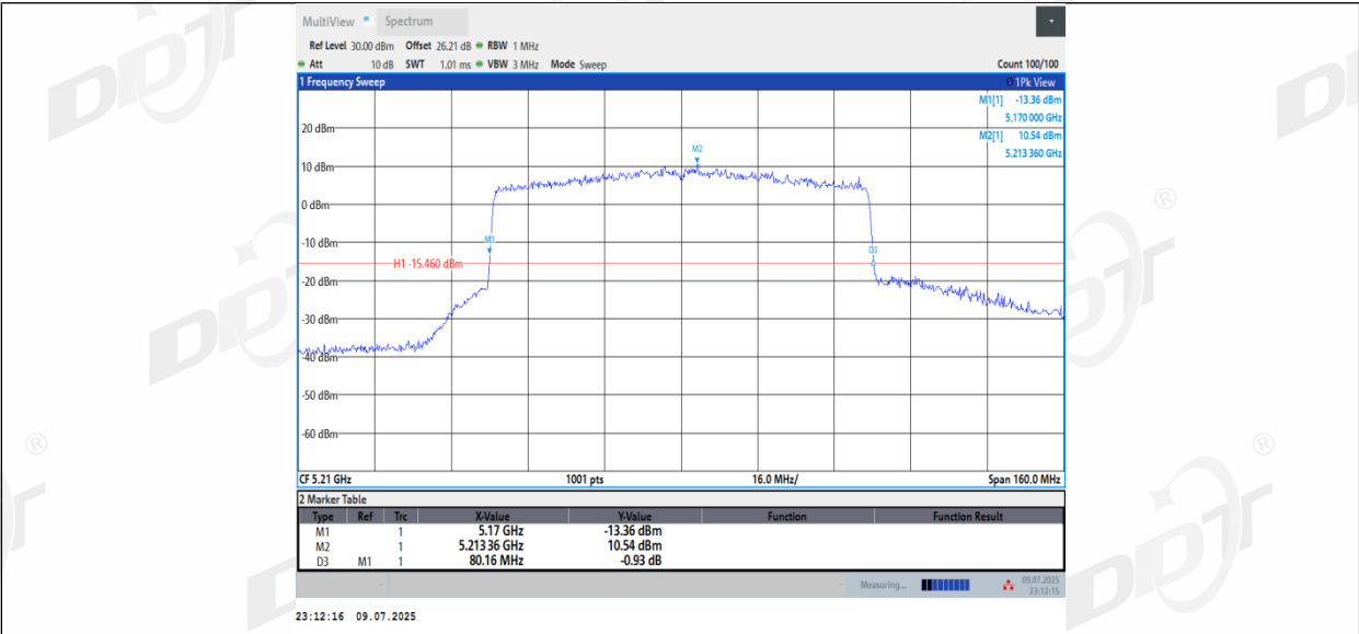
11AX80MIMO_Ant2_5210
