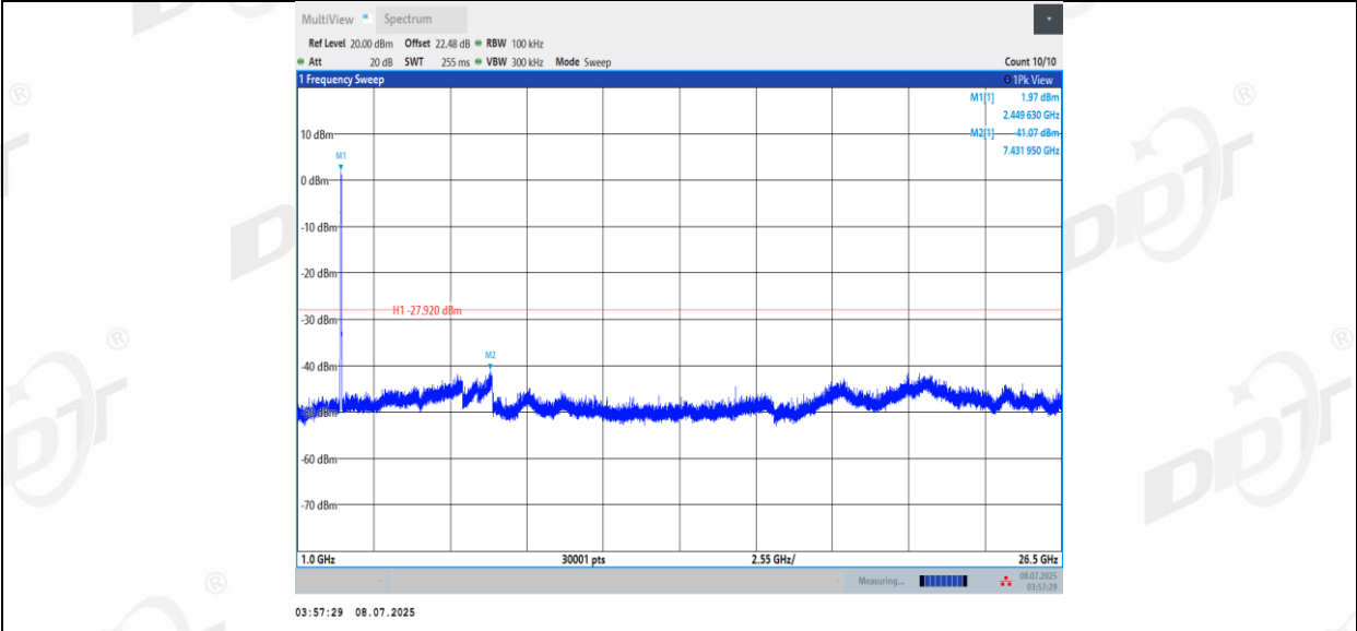
11BE40MIMO_Ant2_2452_1000~26500
