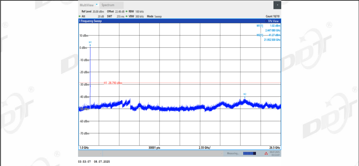
11BE40MIMO_Ant2_2452_0~Reference
