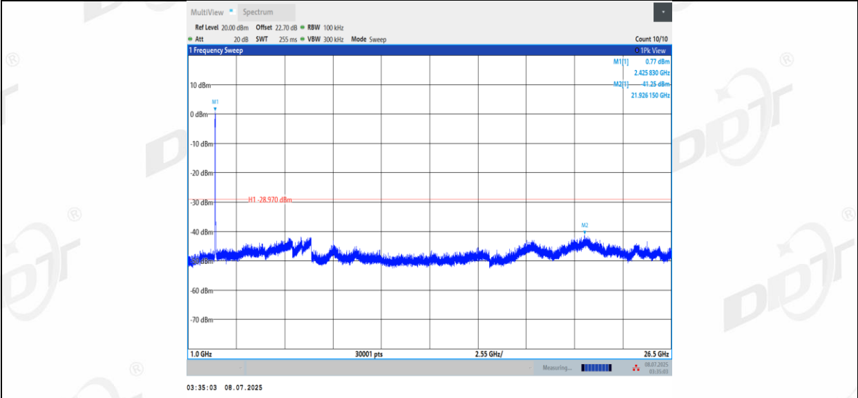
11BE40MIMO_Ant2_2422_0~Reference
