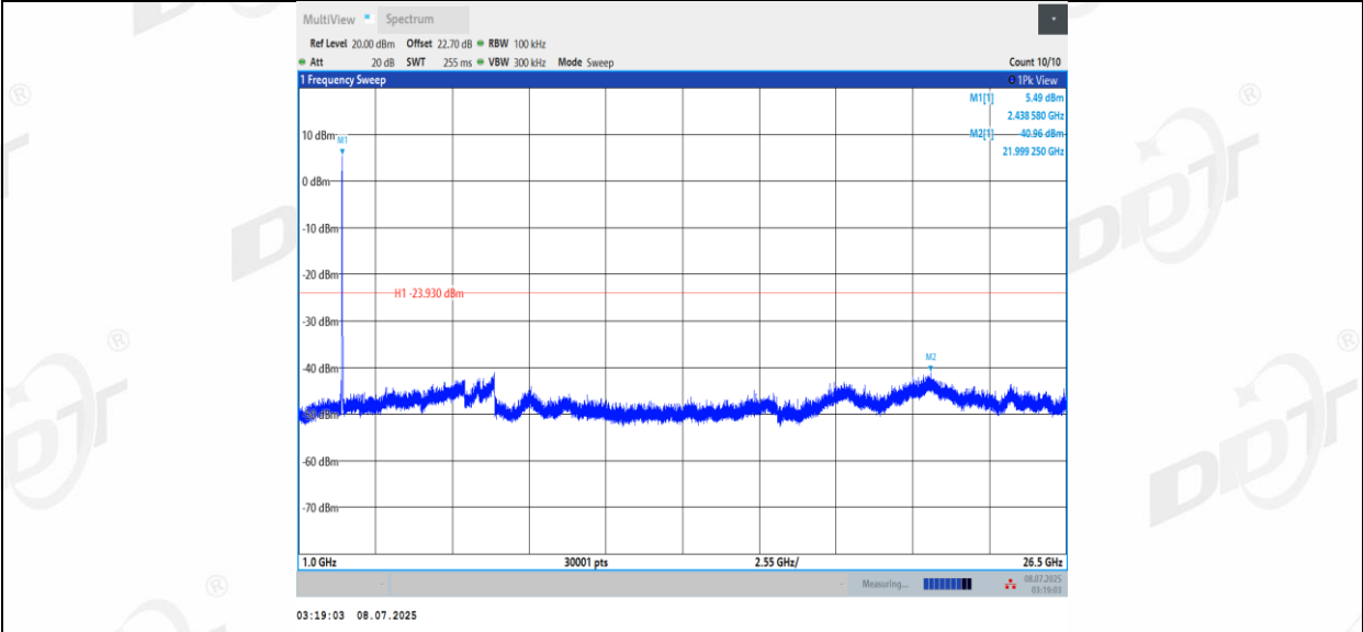
11BE20MIMO_Ant2_2437_0~Reference
