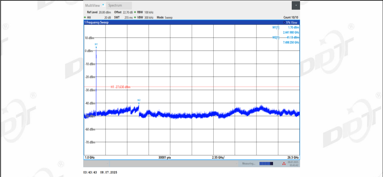
11BE40MIMO_Ant2_2437_0~Reference
