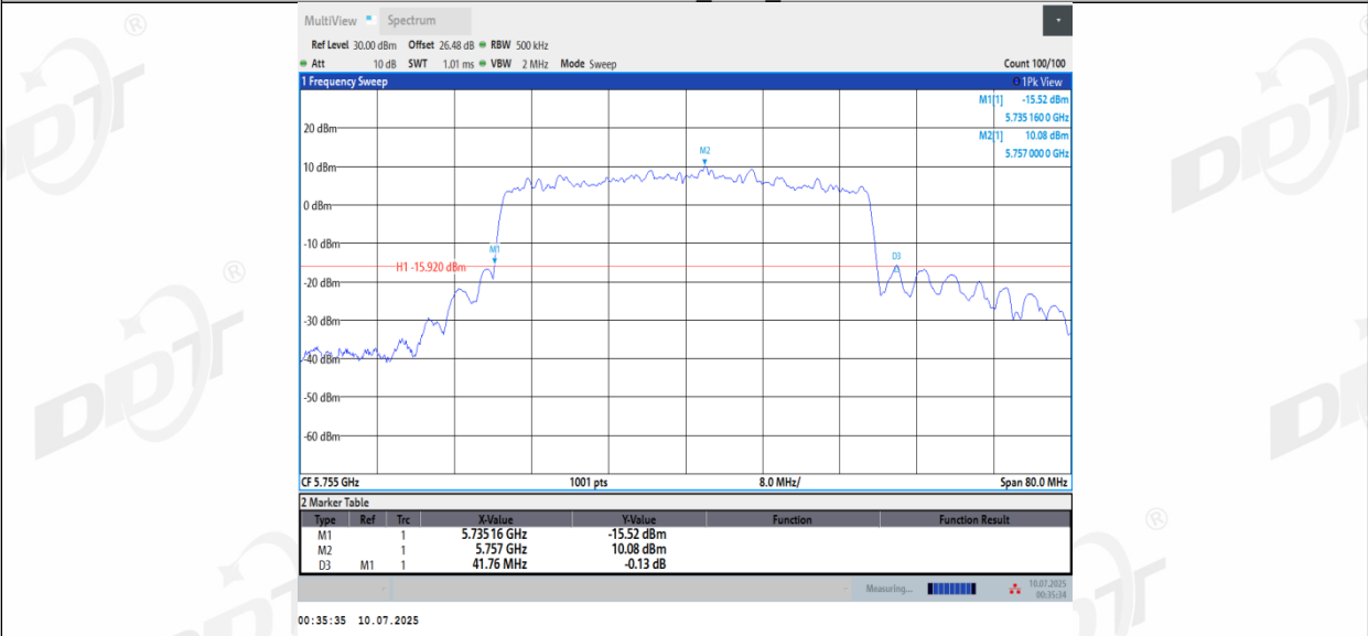
11BE40MIMO_Ant3_5755
