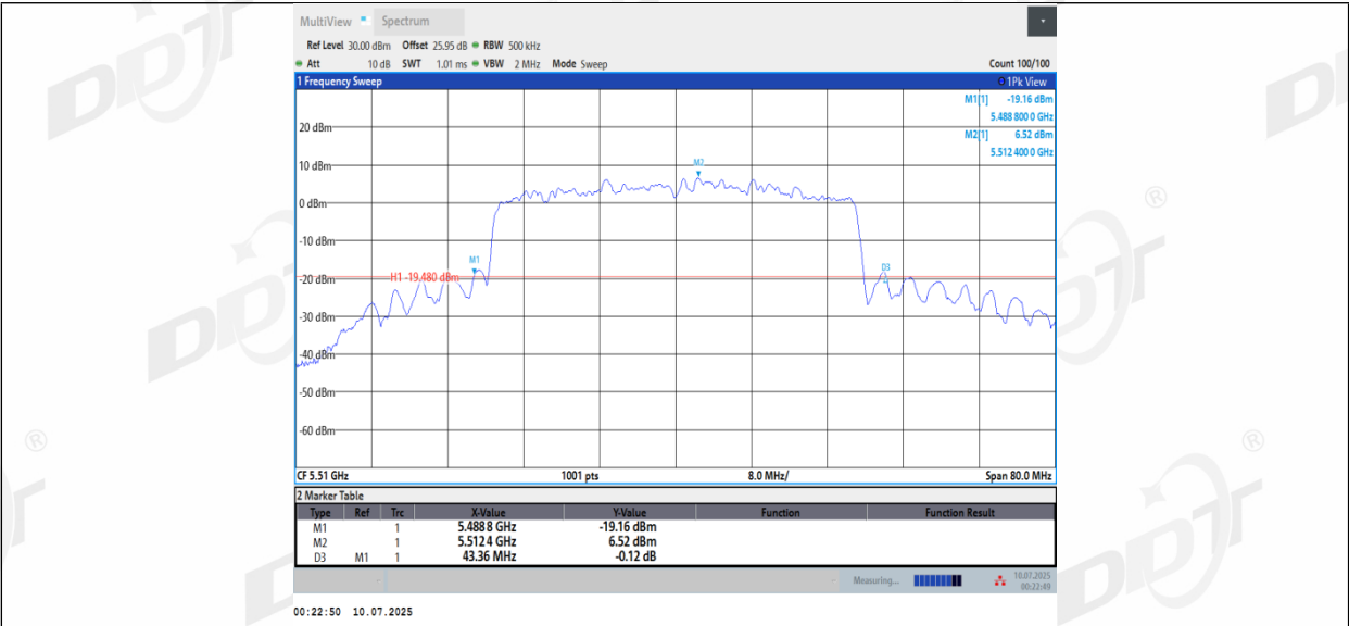
11BE40MIMO_Ant2_5510
