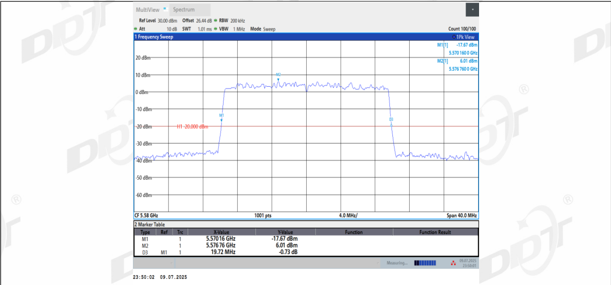
11BE20MIMO_Ant2_5580
