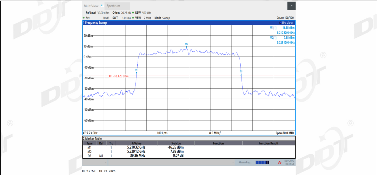
11BE40MIMO_Ant2_5230
