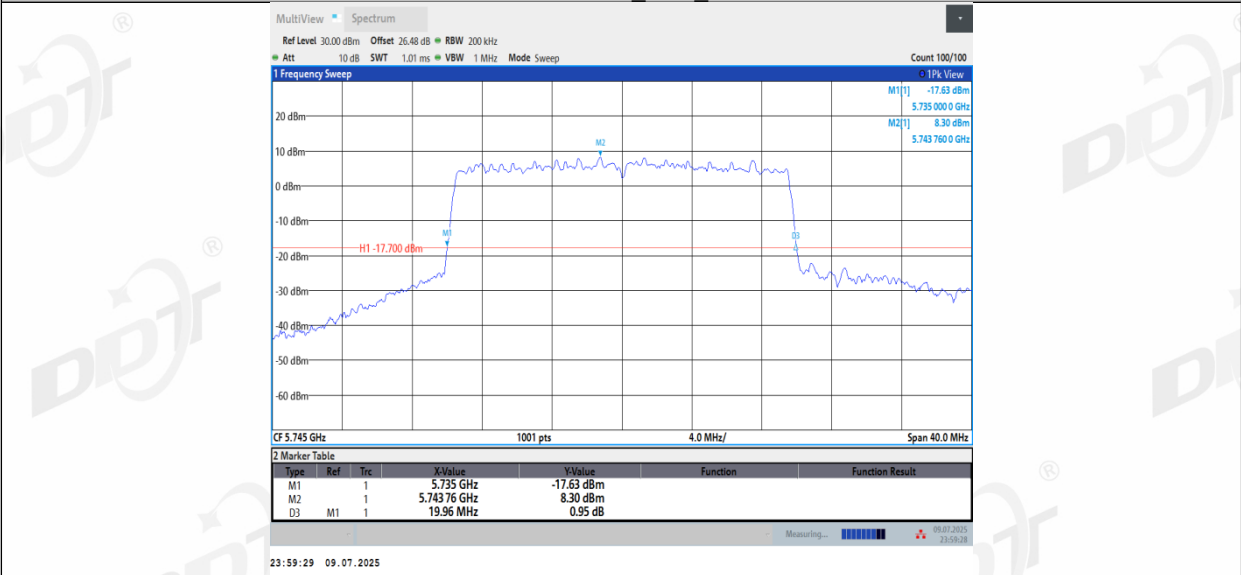
11BE20MIMO_Ant3_5745
