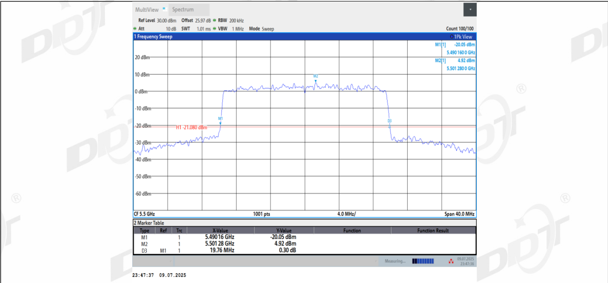
11BE20MIMO_Ant2_5500
