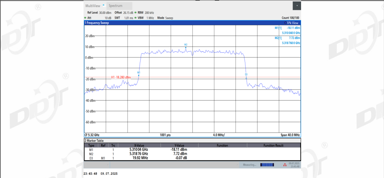
11BE20MIMO_Ant3_5320
