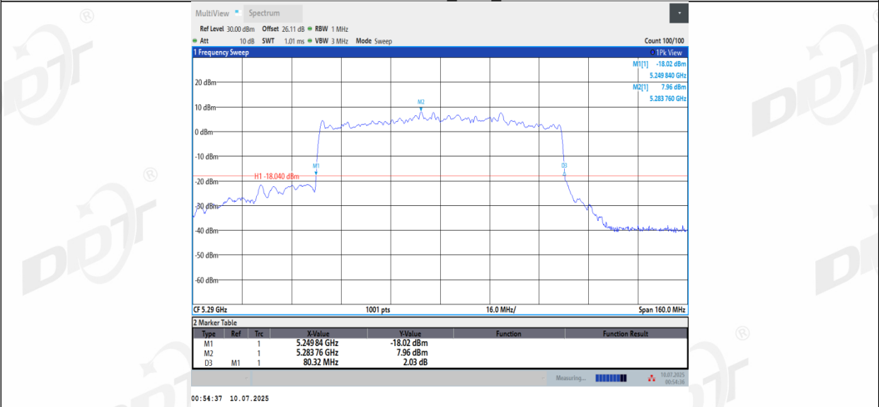
11BE80MIMO_Ant3_5290
