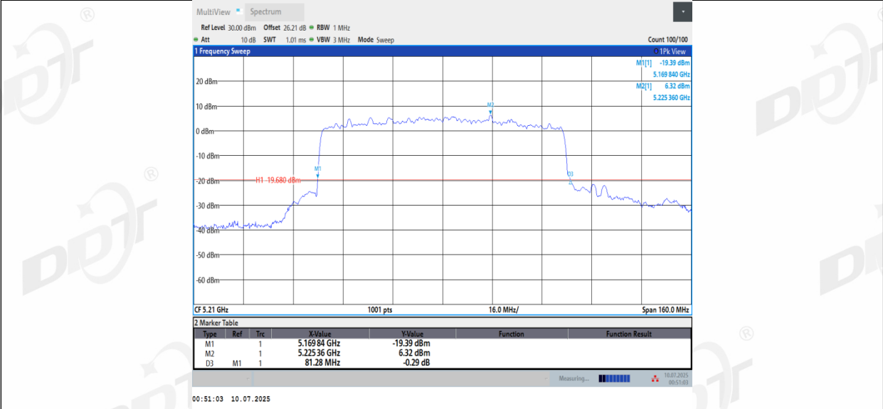
11BE80MIMO_Ant3_5210
