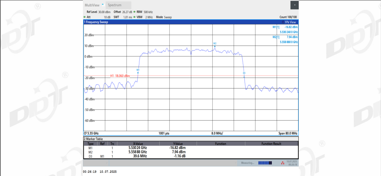
11BE40MIMO_Ant3_5550
