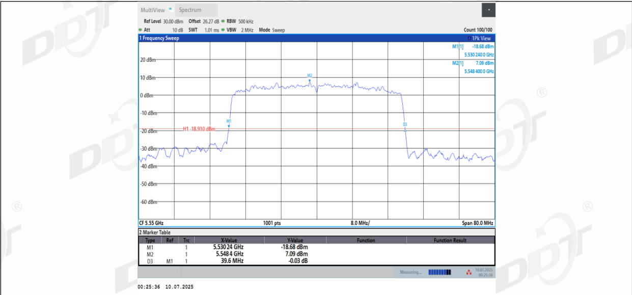
11BE40MIMO_Ant2_5550
