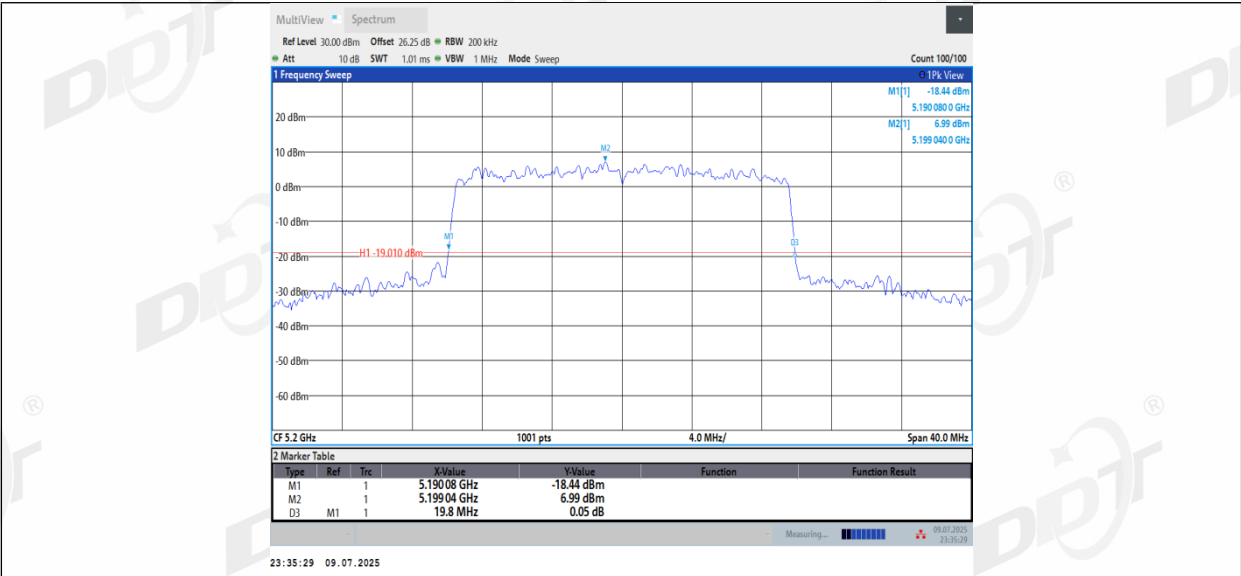
11BE20MIMO_Ant2_5200
