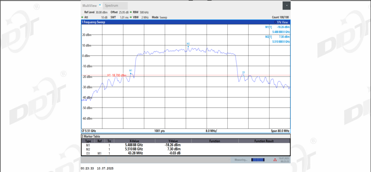
11BE40MIMO_Ant3_5510
