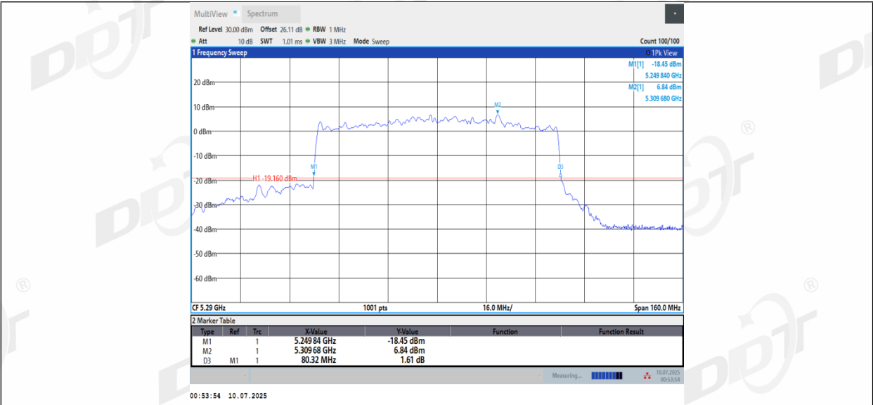
11BE80MIMO_Ant2_5290
