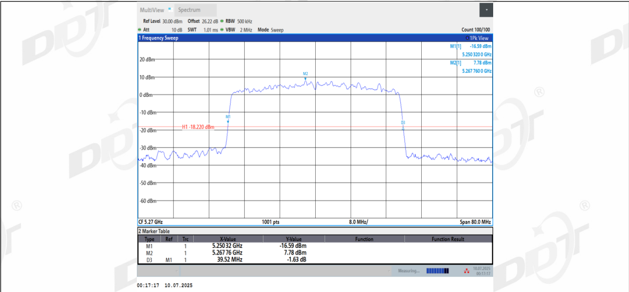
11BE40MIMO_Ant2_5270
