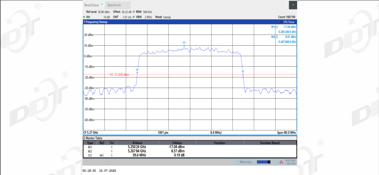
11BE40MIMO_Ant3_5270
