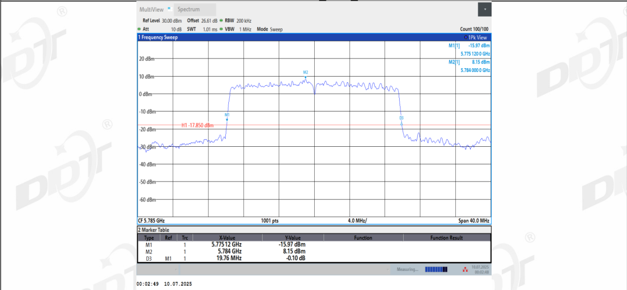
11BE20MIMO_Ant3_5785
