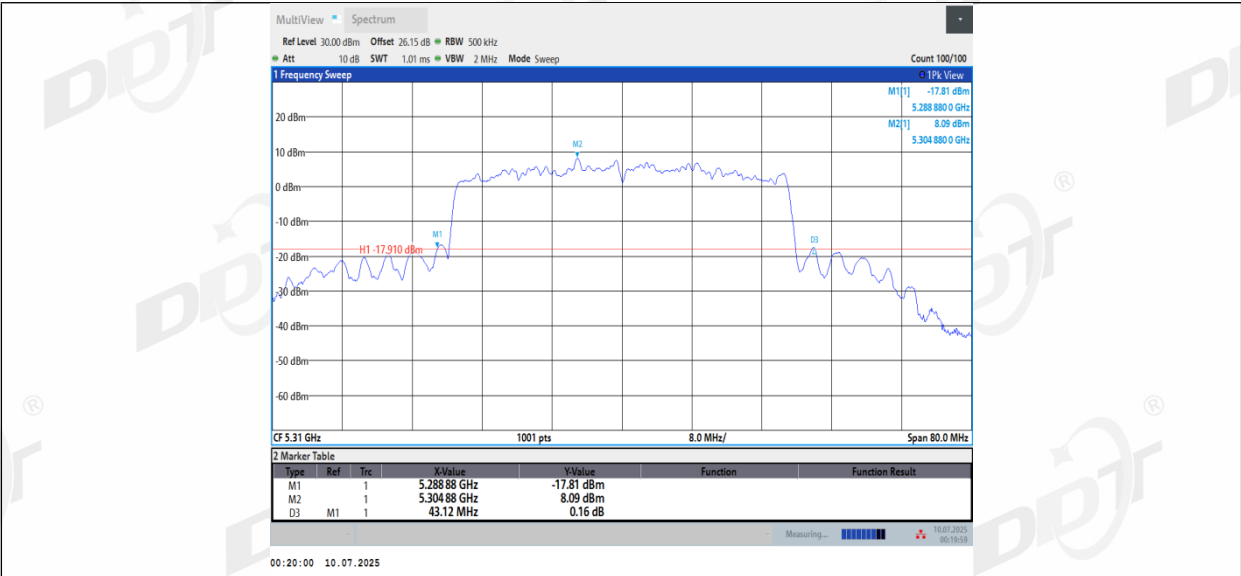
11BE40MIMO_Ant2_5310
