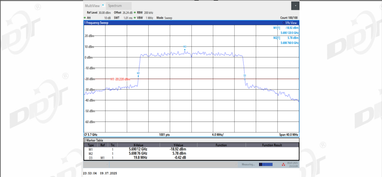
11BE20MIMO_Ant3_5700
