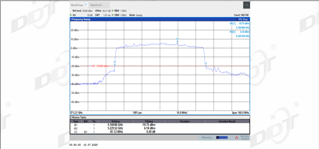
11BE80MIMO_Ant2_5210
