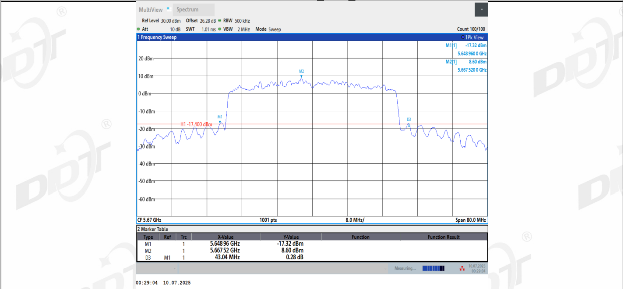
11BE40MIMO_Ant3_5670
