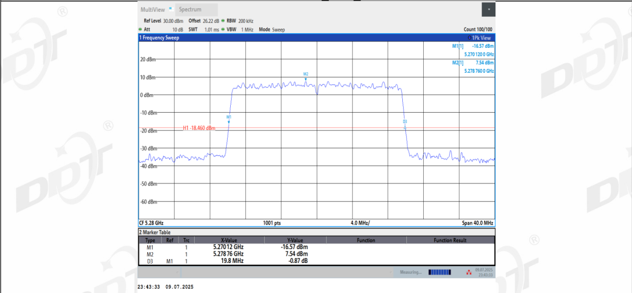
11BE20MIMO_Ant3_5280
