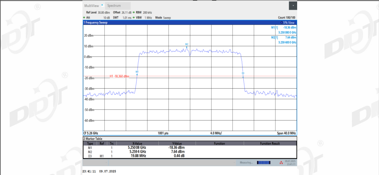
11BE20MIMO_Ant3_5260
