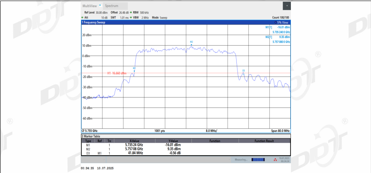
11BE40MIMO_Ant2_5755
