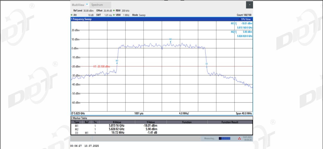
11BE20MIMO_Ant3_5825
