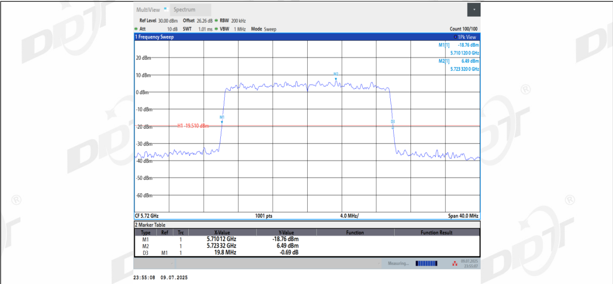
11BE20MIMO_Ant2_5720
