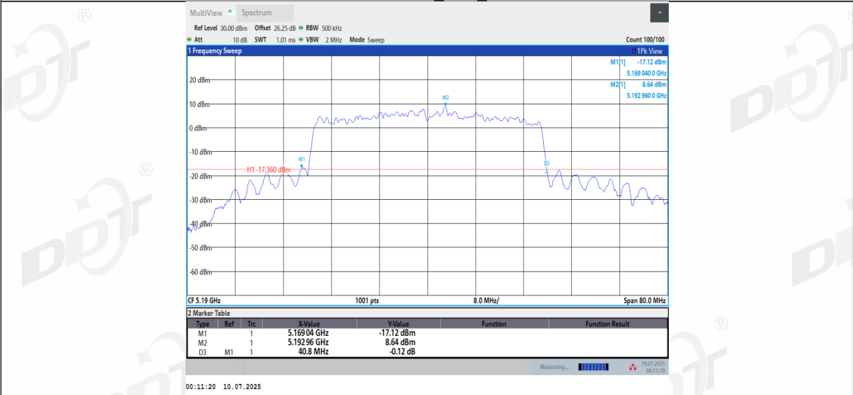
11BE40MIMO_Ant3_5190
