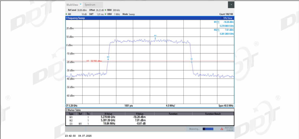
11BE20MIMO_Ant2_5280
