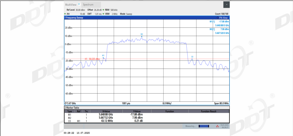
11BE40MIMO_Ant2_5670
