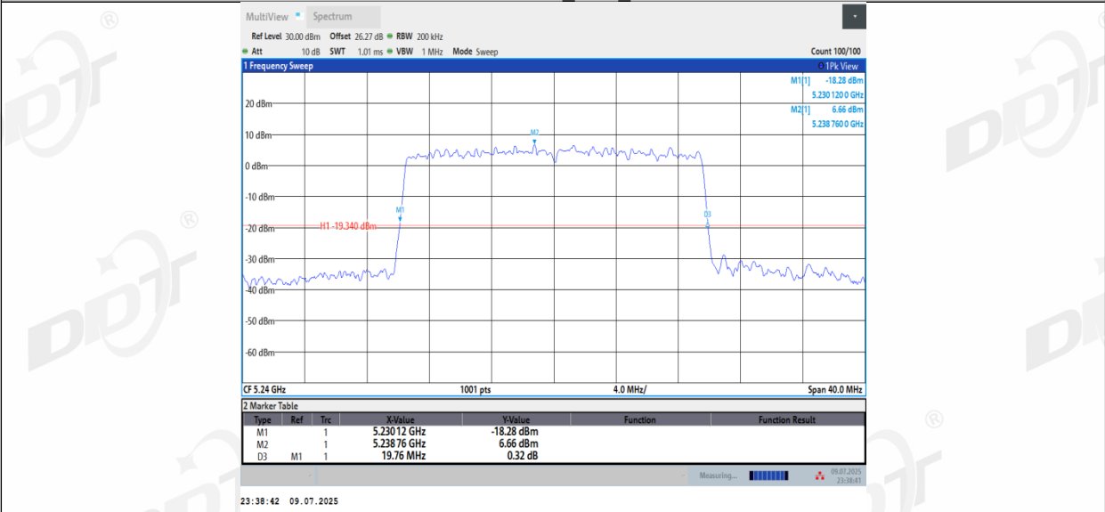
11BE20MIMO_Ant3_5240
