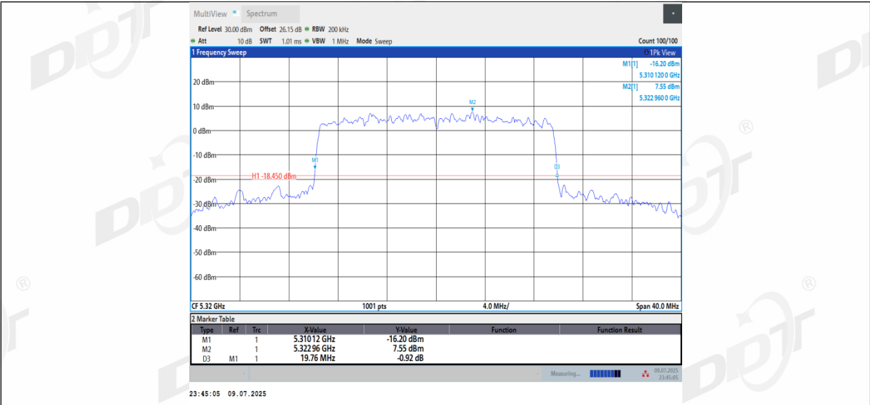
11BE20MIMO_Ant2_5320
