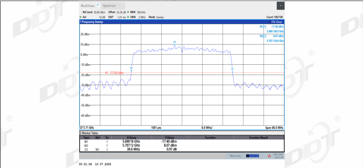
11BE40MIMO_Ant2_5710
