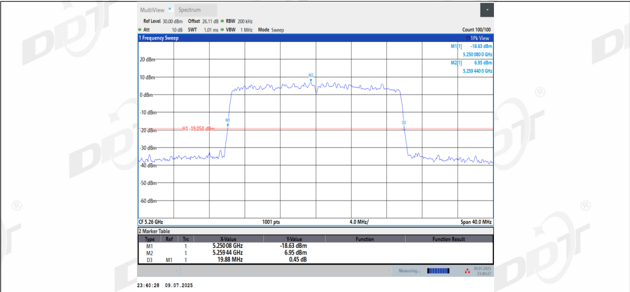
11BE20MIMO_Ant2_5260
