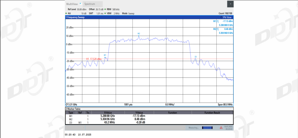
11BE40MIMO_Ant3_5310
