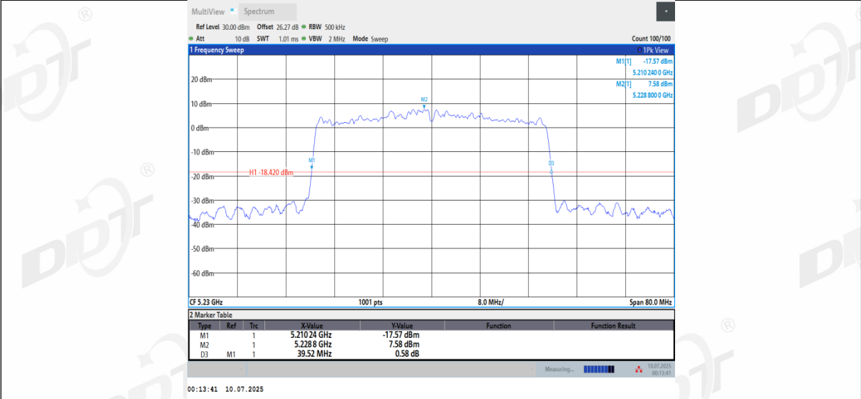
11BE40MIMO_Ant3_5230
