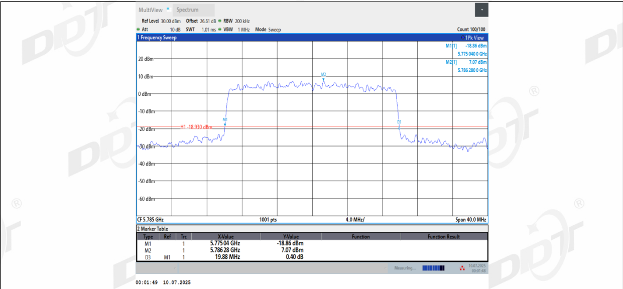
11BE20MIMO_Ant2_5785
