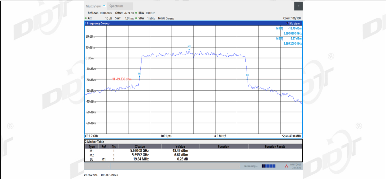
11BE20MIMO_Ant2_5700
