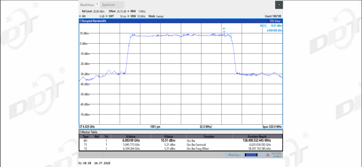
11AX160MIMO_Ant3_6025
