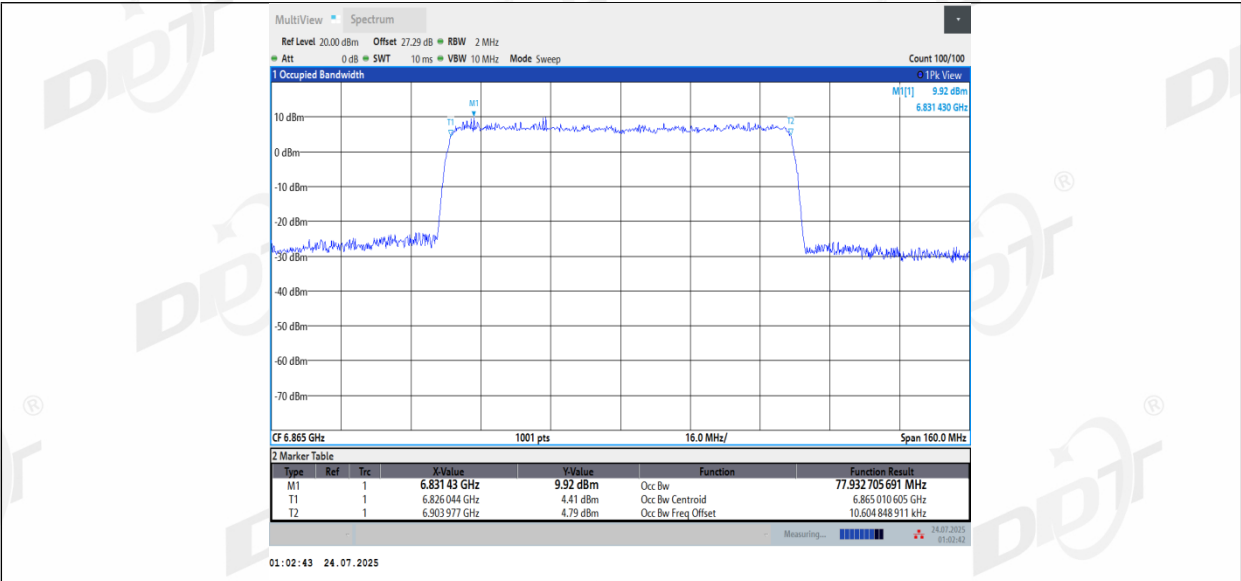
11AX80MIMO_Ant2_6865
