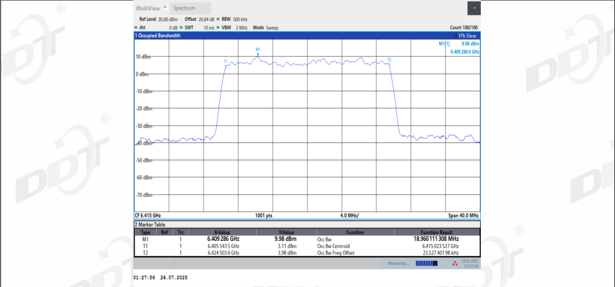
11BE20MIMO_Ant3_6415
