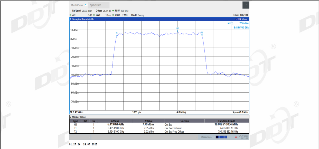
11BE20MIMO_Ant2_6415
