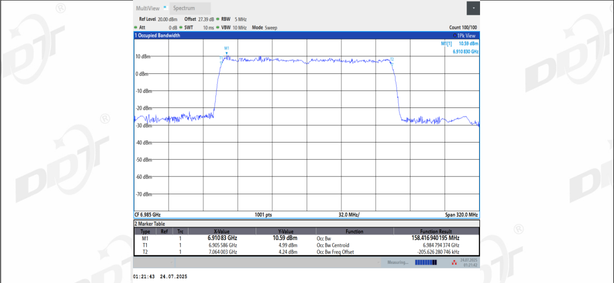
11AX160MIMO_Ant3_6985
