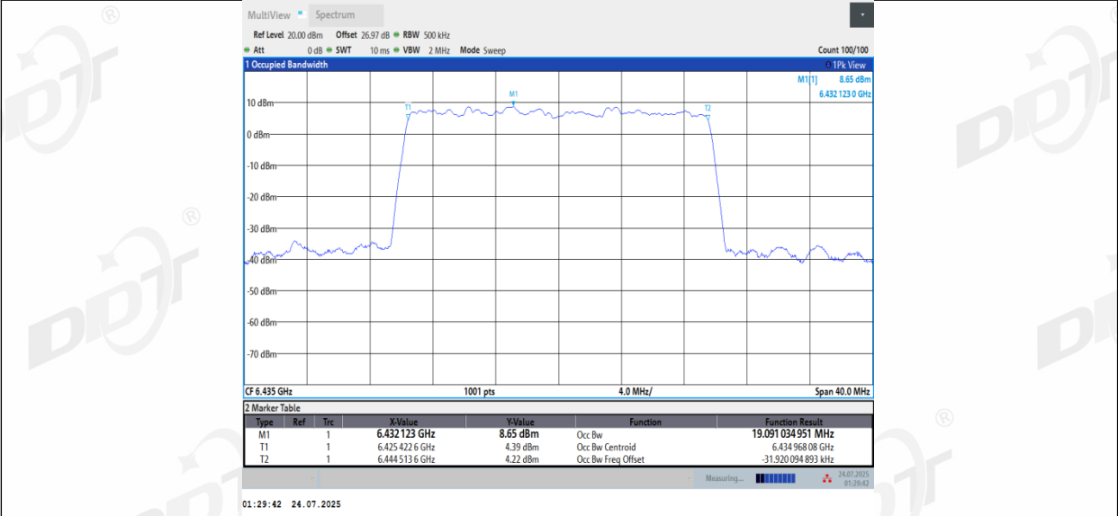
11BE20MIMO_Ant3_6435
