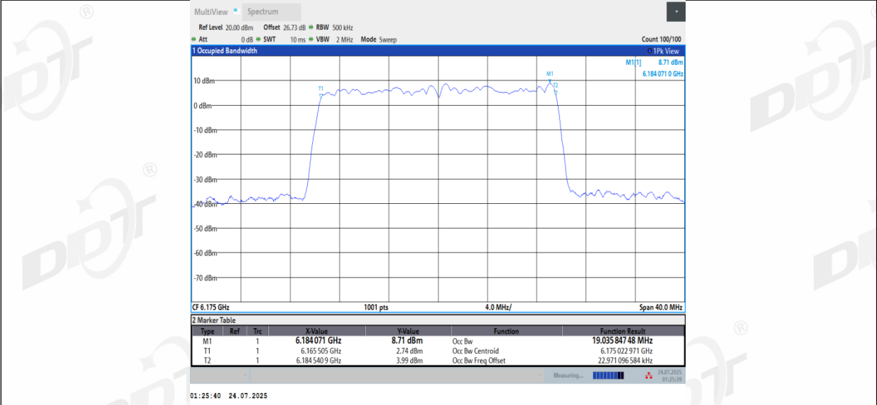
11BE20MIMO_Ant3_6175
