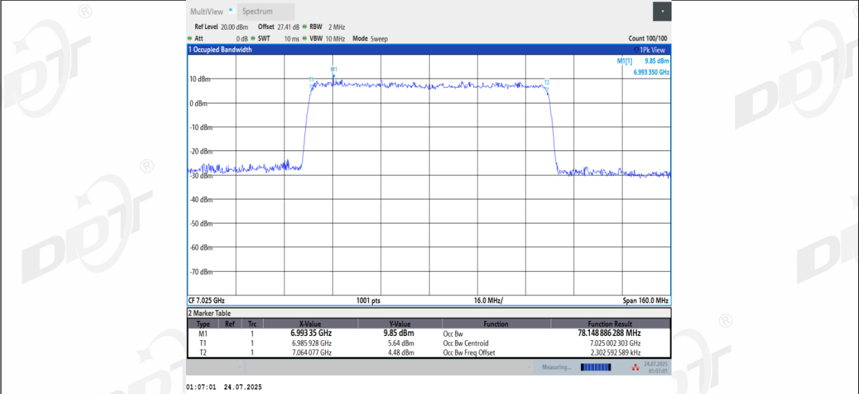
11AX80MIMO_Ant3_7025
