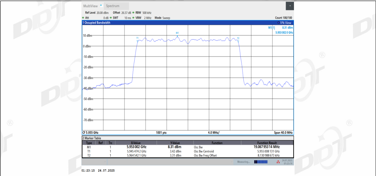
11BE20MIMO_Ant2_5955
