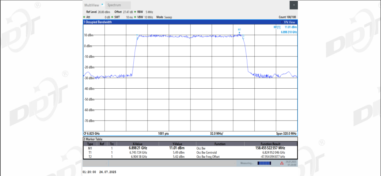
11AX160MIMO_Ant3_6825
