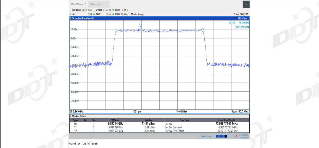
11AX80MIMO_Ant3_6865
