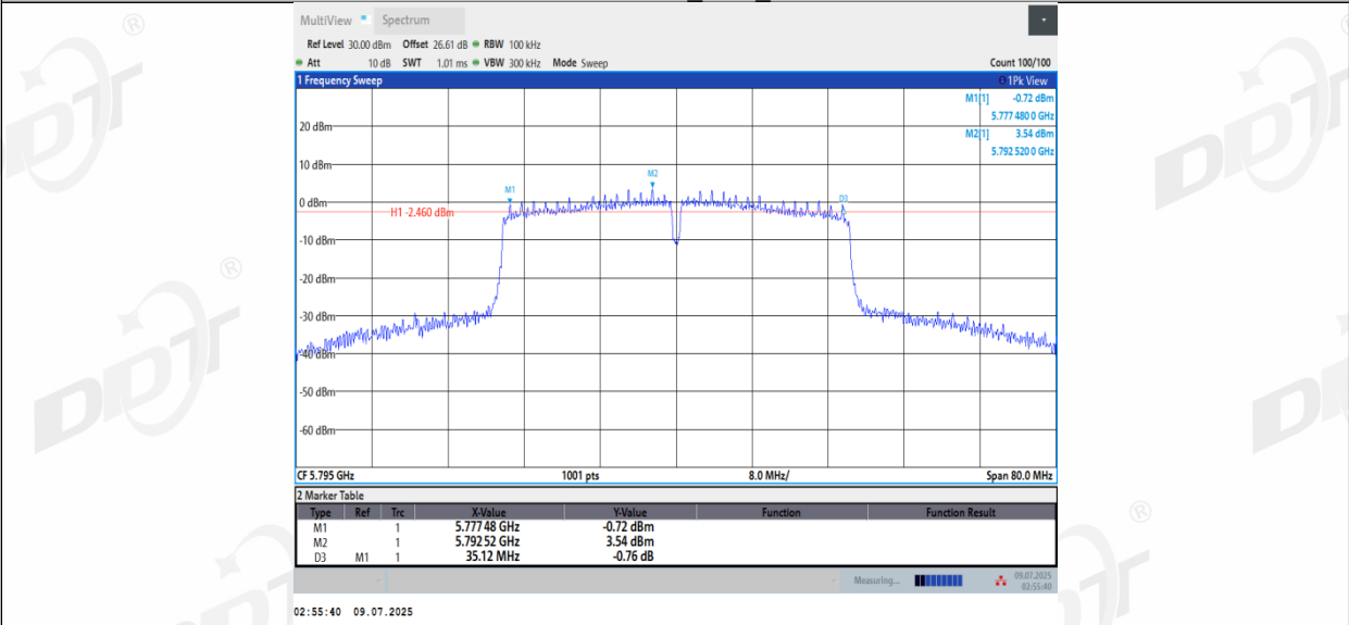
11AC40MIMO_Ant3_5795
