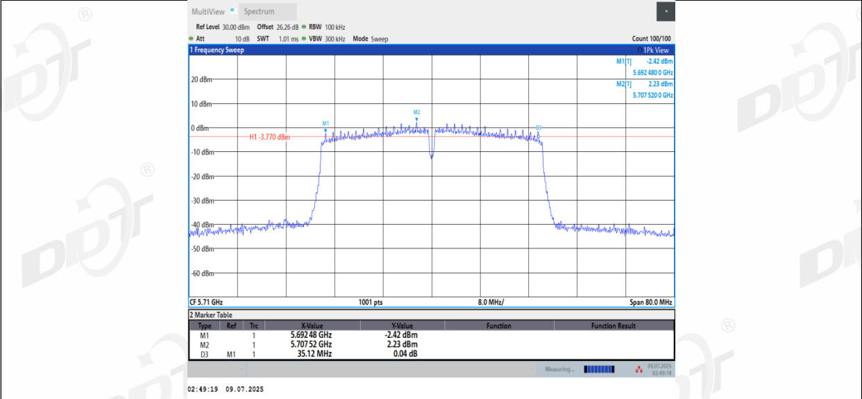
11AC40MIMO_Ant3_5710
