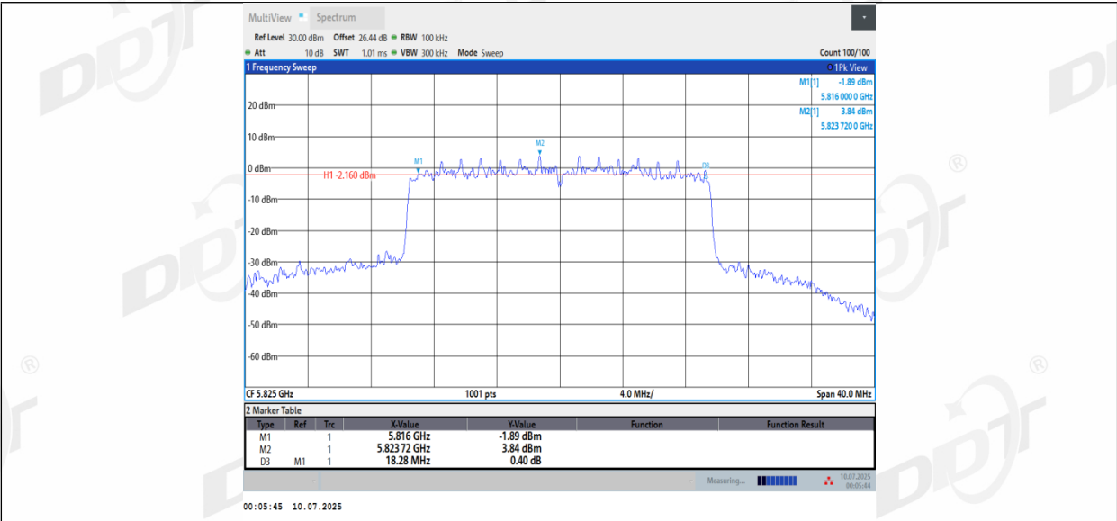
11BE20MIMO_Ant2_5825
