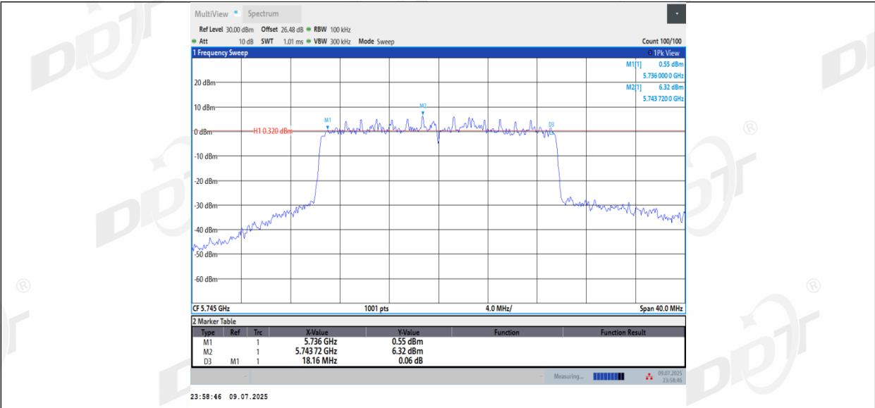
11BE20MIMO_Ant2_5745
