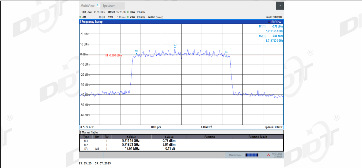
11BE20MIMO_Ant2_5720
