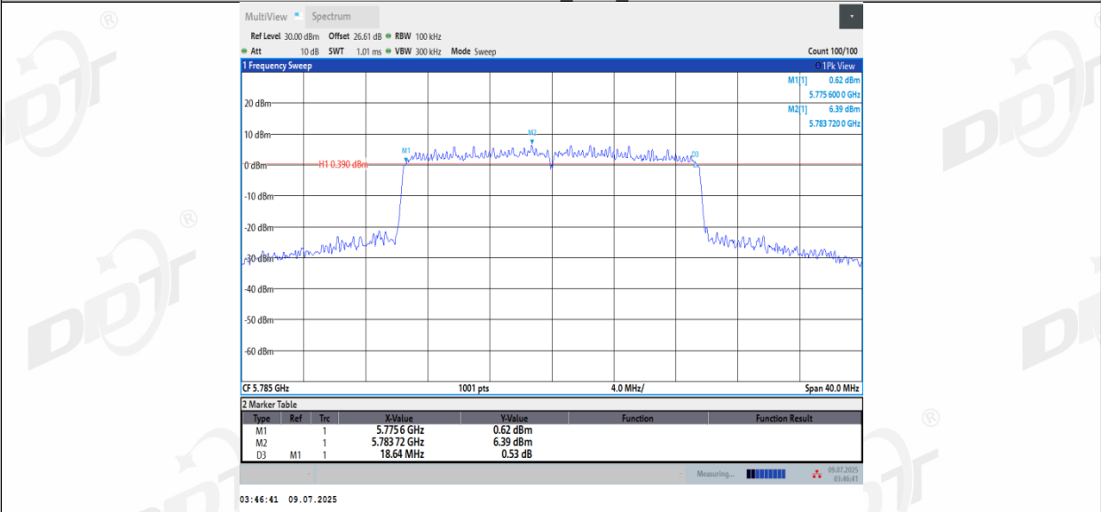
11AX20MIMO_Ant3_5785
