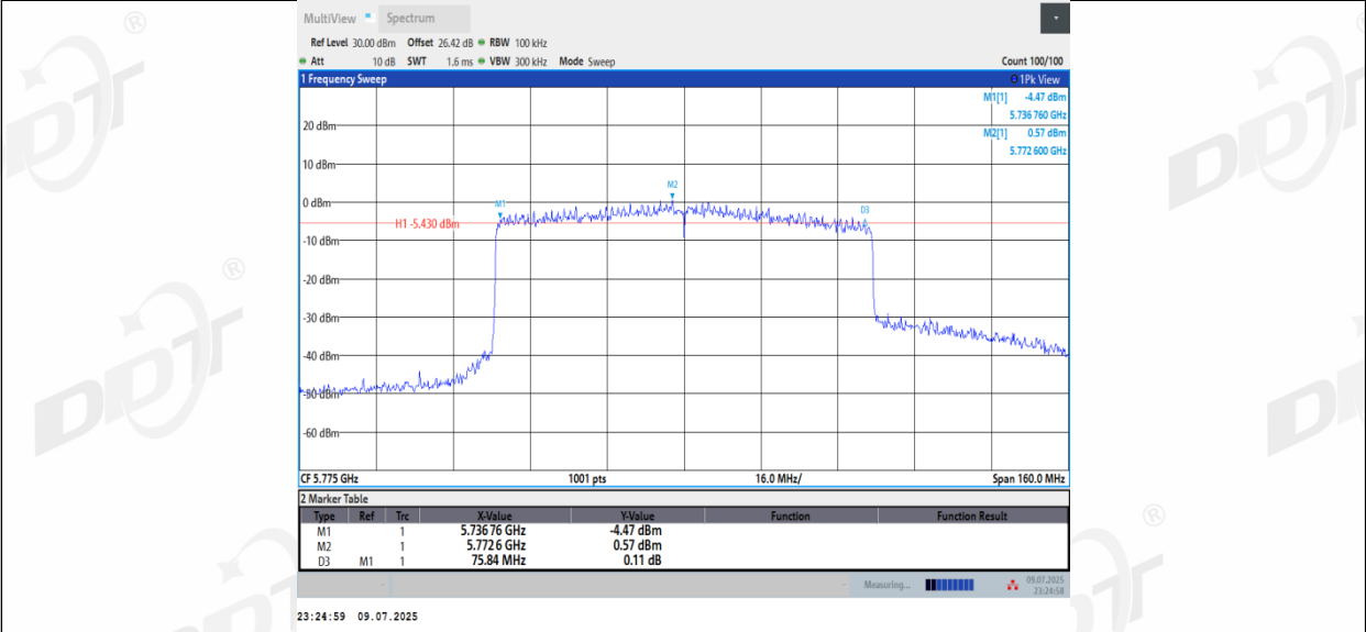
11AX80MIMO_Ant3_5775
