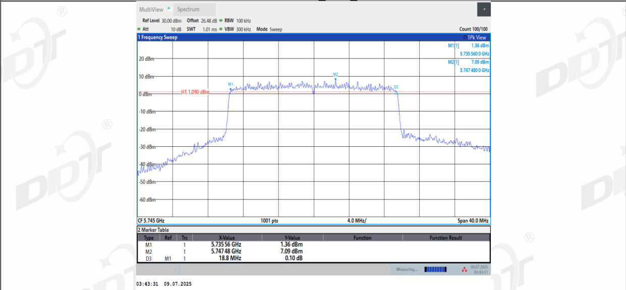
11AX20MIMO_Ant3_5745
