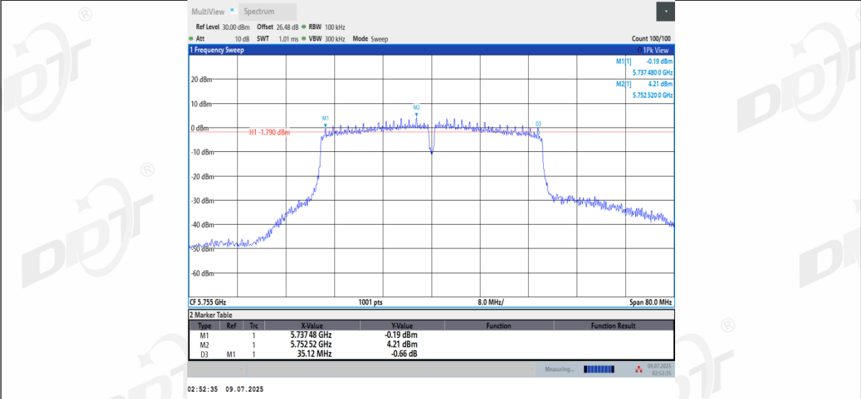
11AC40MIMO_Ant3_5755
