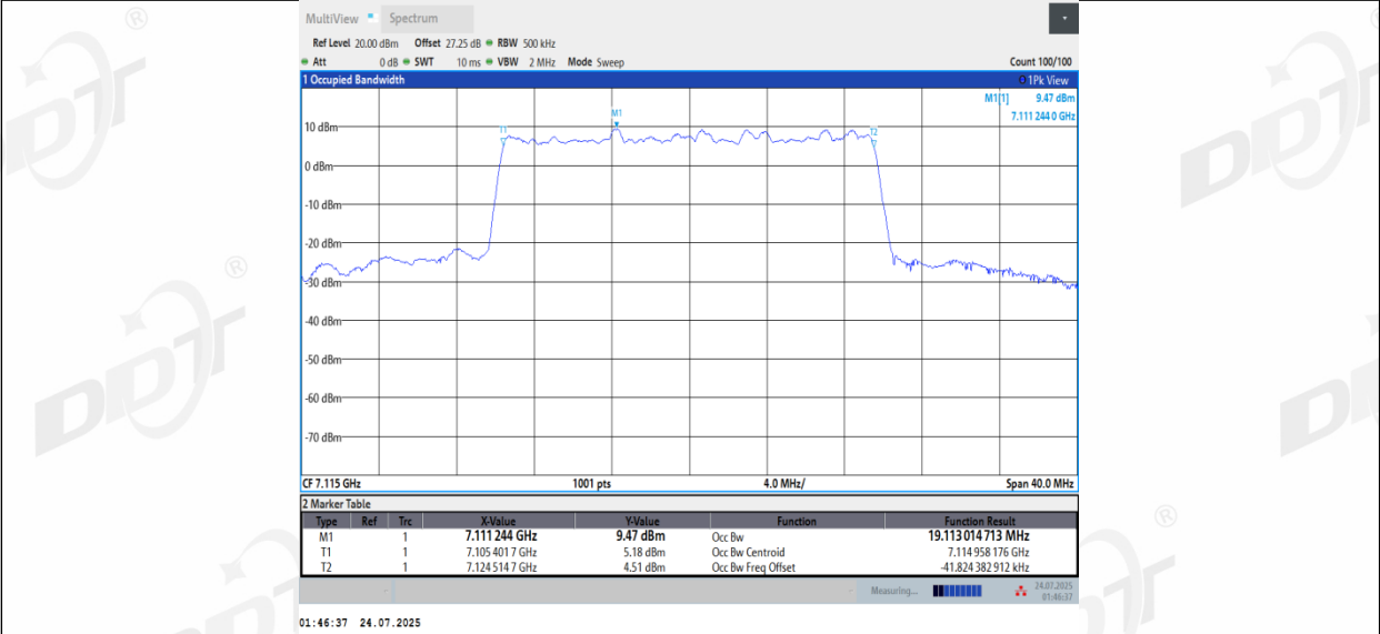
11BE20MIMO_Ant3_7115
