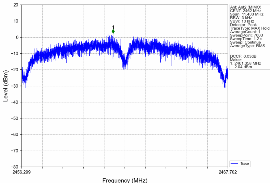
802.11b_HCH_2462MHz_Ant2 (MIMO)_NTNV
