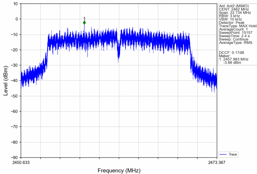
802.11g_HCH_2462MHz_MIMO_NTNV
