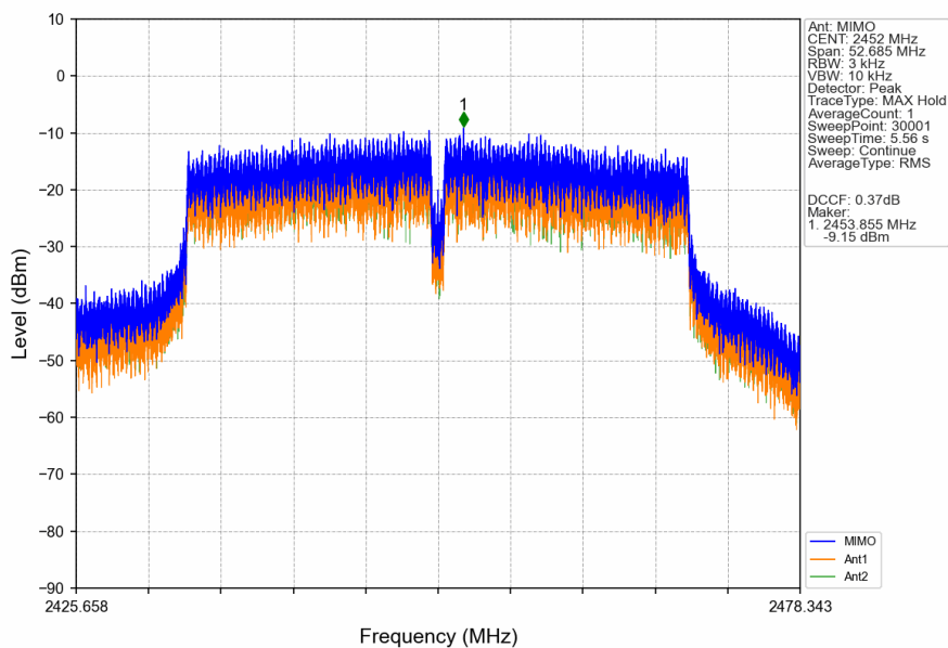
802.11n(HT40)_HCH_2452MHz_MIMO_NTNV
