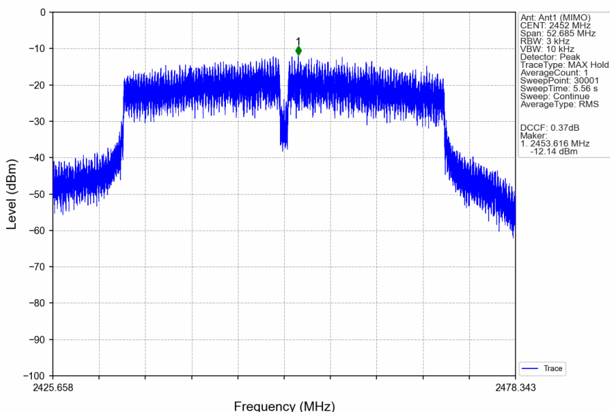
802.11n(HT40)_HCH_2452MHz_Ant1 (MIMO)_NTNV
