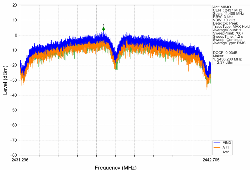
802.11b_MCH_2437MHz_MIMO_NTNV
