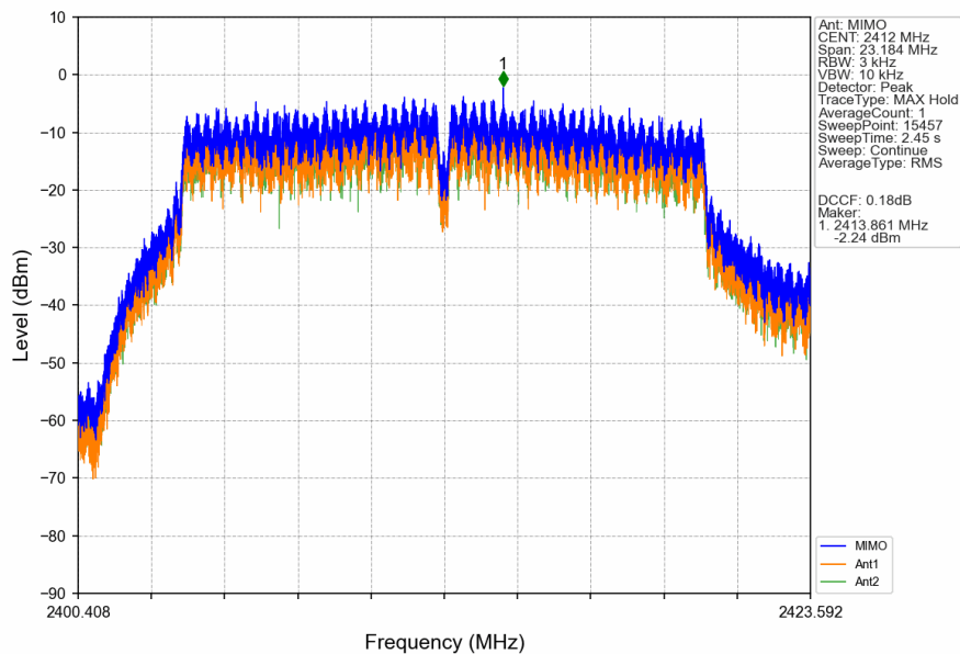
802.11g_LCH_2412MHz_MIMO_NTNV
