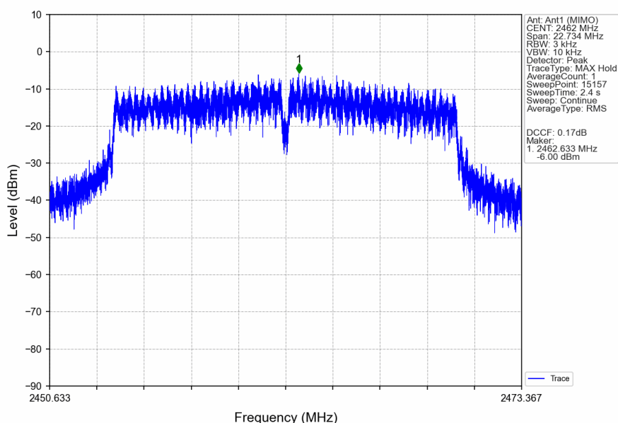
802.11g_HCH_2462MHz_Ant1 (MIMO)_NTNV
