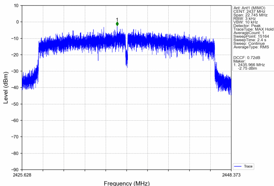
802.11ax(HEW20)_MCH_2437MHz_RU242_Left_Ant1 (MIMO)_NTNV
