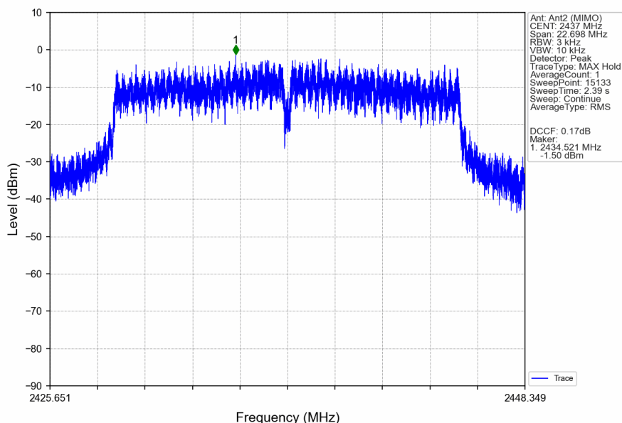
802.11g_MCH_2437MHz_Ant2 (MIMO)_NTNV
