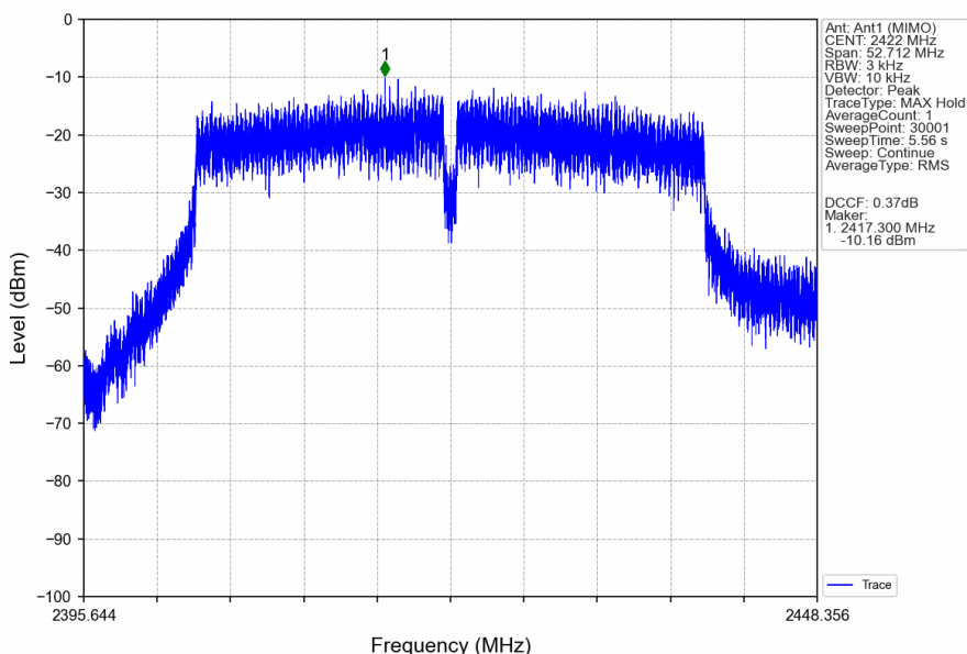
802.11n(HT40)_LCH_2422MHz_Ant1 (MIMO)_NTNV
