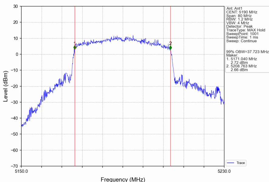
802.11ax(HEW40)_LCH_5190MHz_RU484_Left_Ant1_NTNV
