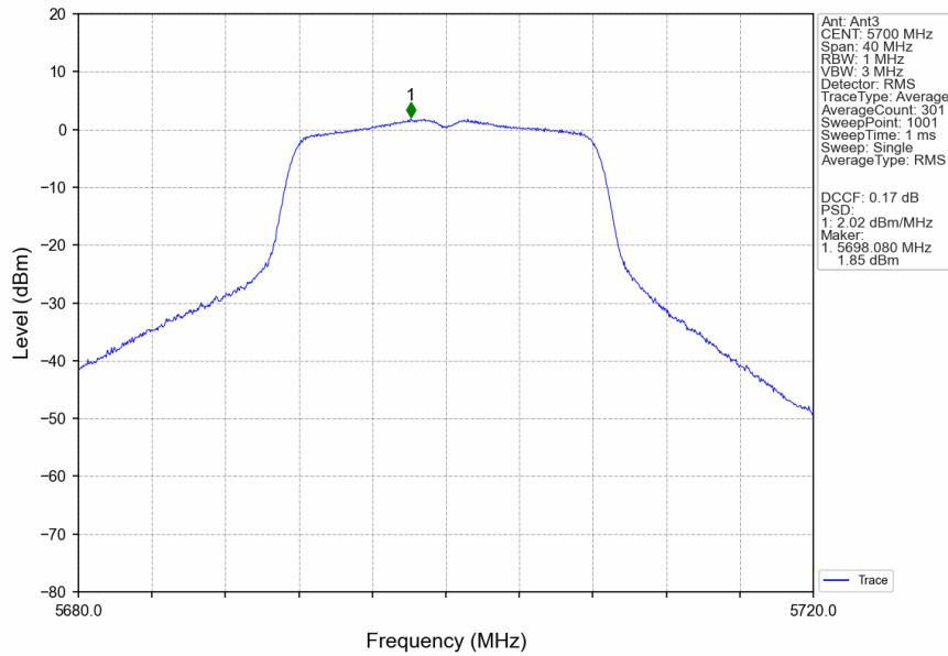
802.11a_HCH_5700MHz_MIMO_NTNV
