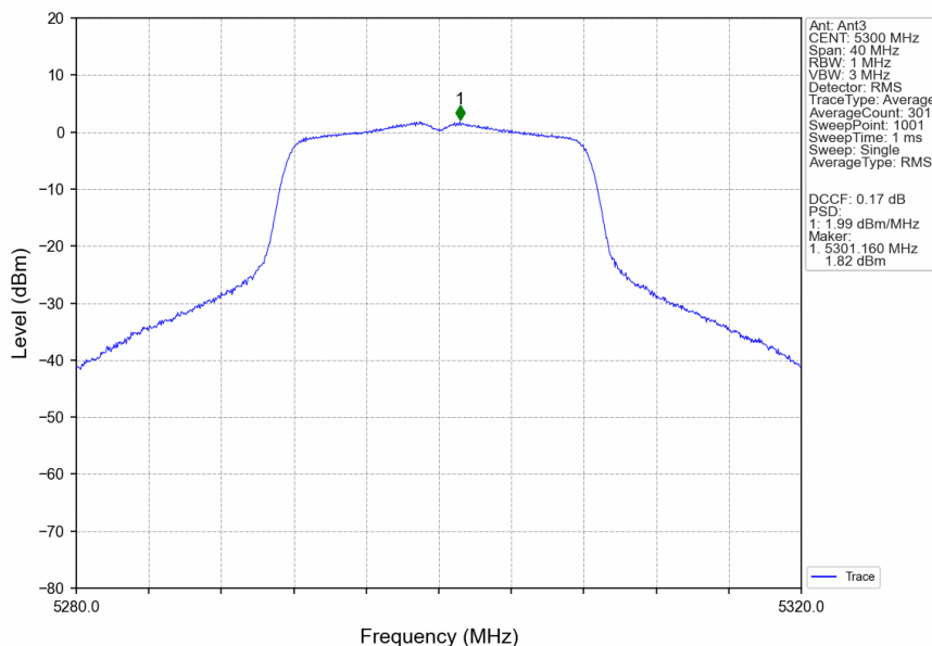
802.11a_MCH_5300MHz_MIMO_NTNV
