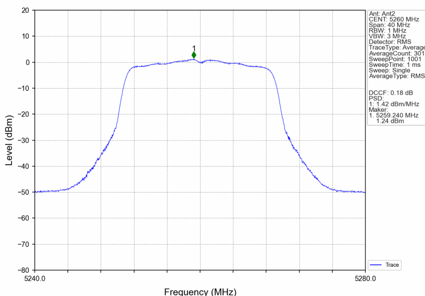
802.11n(HT20)_LCH_5260MHz_Ant2_NTNV
