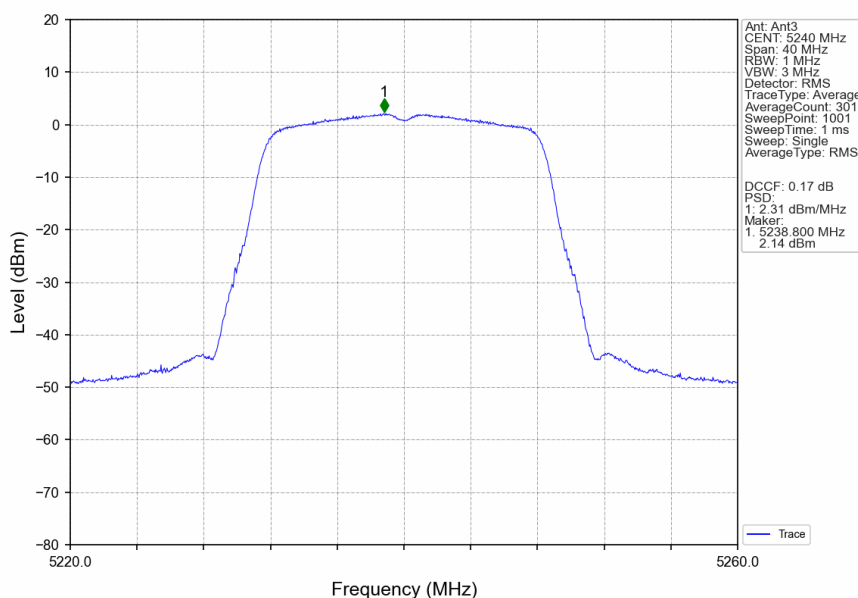
802.11a_HCH_5240MHz_MIMO_NTNV
