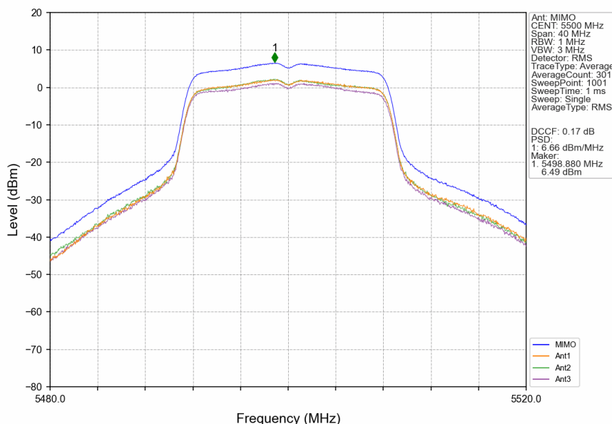
802.11a_LCH_5500MHz_MIMO_NTNV
