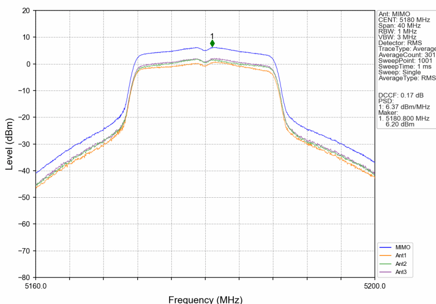
802.11a_LCH_5180MHz_MIMO_NTNV
