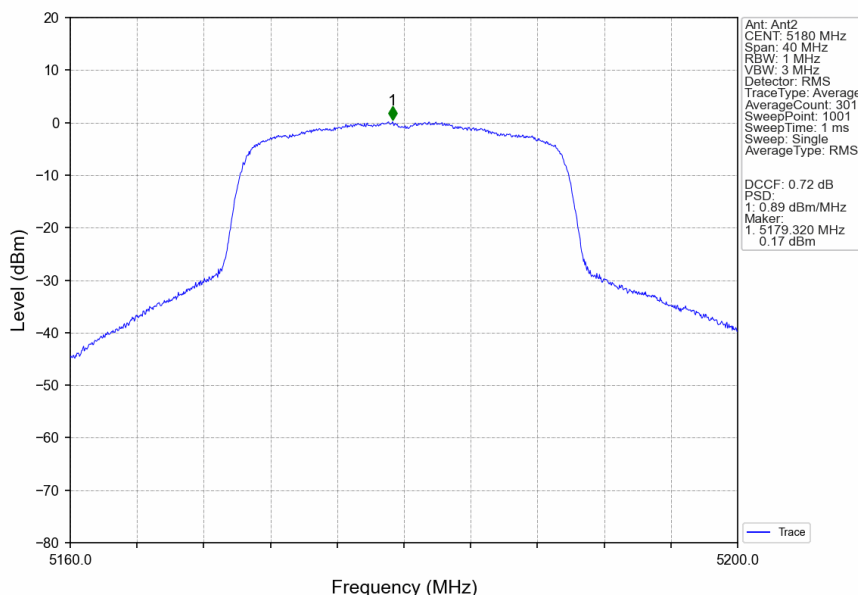
802.11ax(HEW20)_LCH_5180MHz_RU242_Left_Ant2_NTNV
