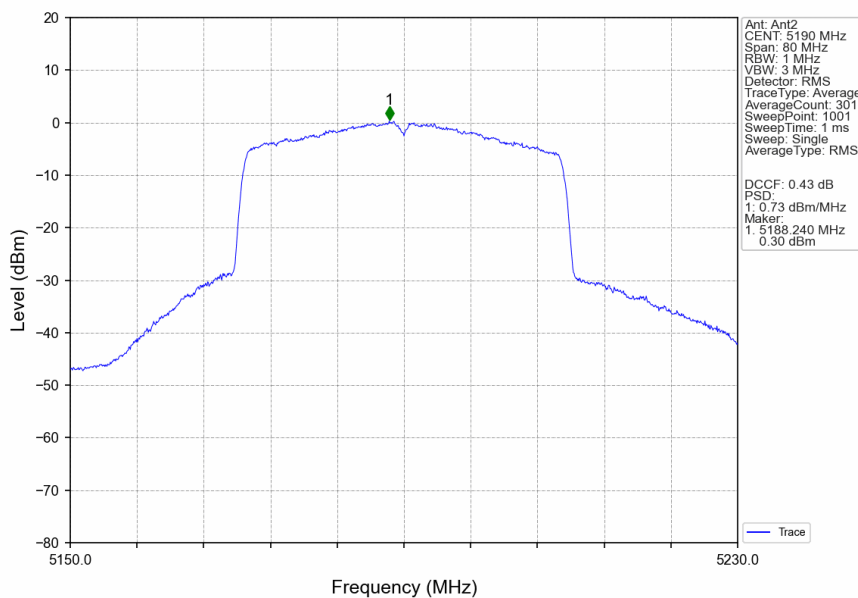
802.11ax(HEW40)_LCH_5190MHz_RU484_Left_Ant2_NTNV
