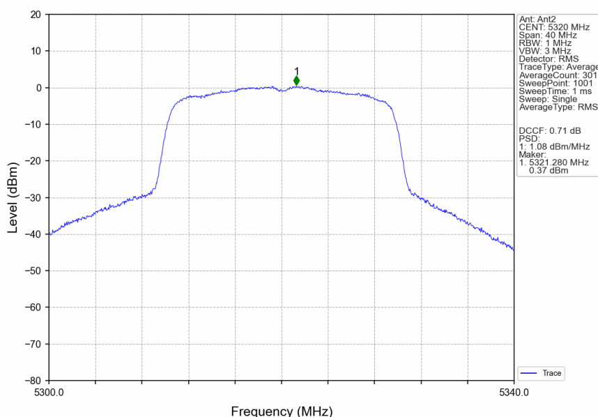
802.11ax(HEW20)_HCH_5320MHz_RU242_Left_Ant2_NTNV
