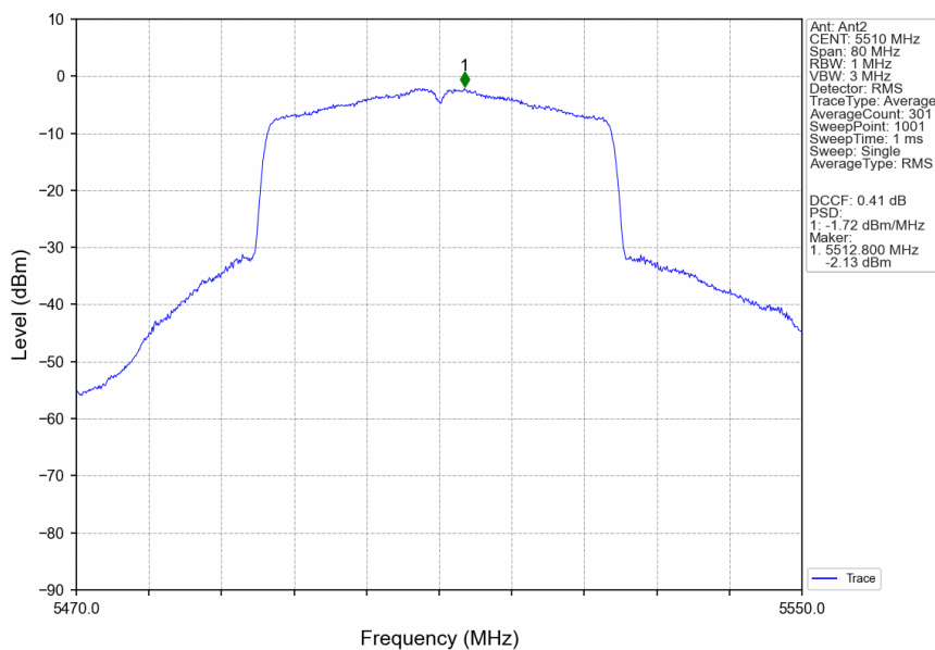
802.11ax(HEW40)_LCH_5510MHz_RU484_Left_Ant2_NTNV
