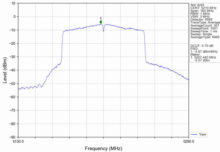
802.11ac(VHT80)_MCH_5210MHz_MIMO_NTNV
