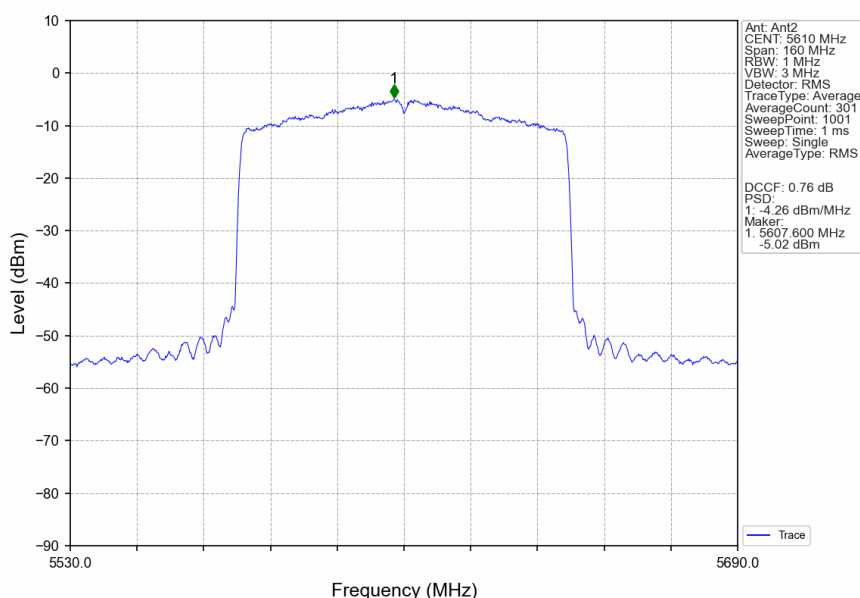
802.11ax(HEW80)_HCH_5610MHz_RU996_Left_Ant2_NTNV
