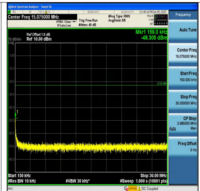
GSM850-128-5-0.15~30MHz-PASS
