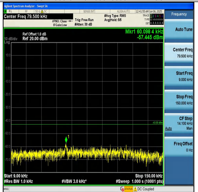
GSM1900-661-0-0.009~0.15MHz-PASS
