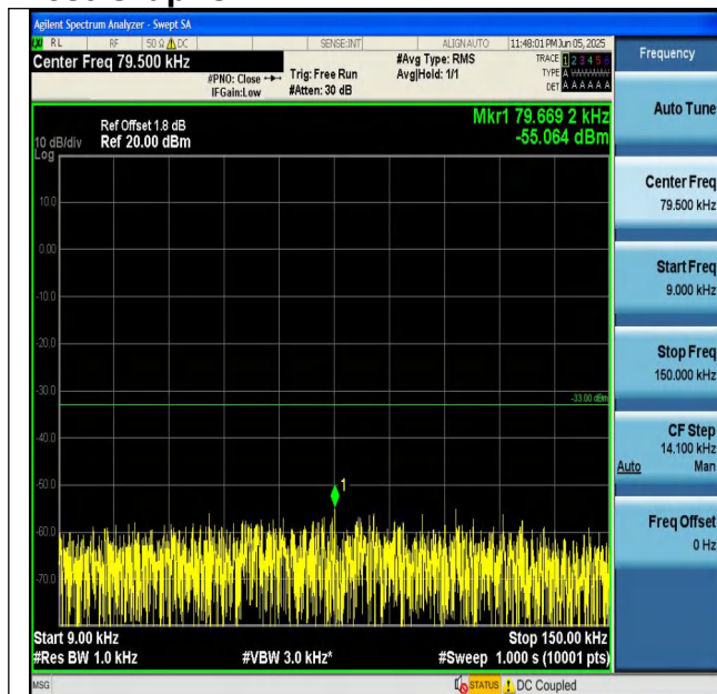
GSM850-128-5-0.009~0.15MHz-PASS
