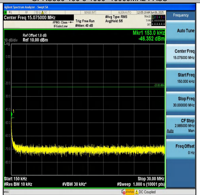
GPRS850-251-5-0.15~30MHz-PASS
