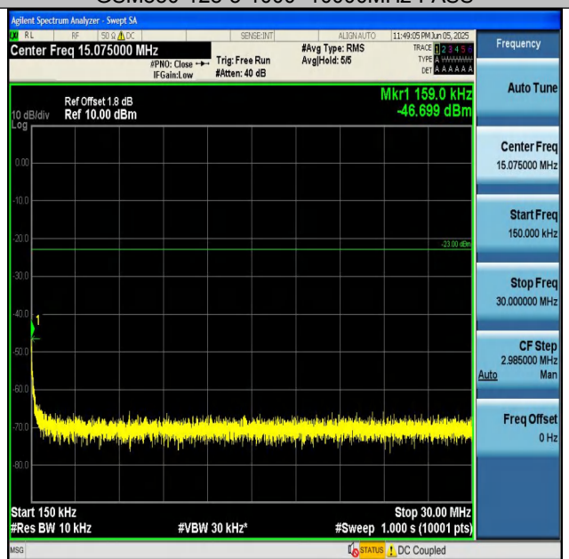
GSM850-190-5-0.15~30MHz-PASS
