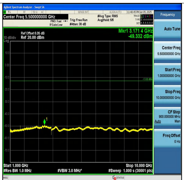
GSM850-128-5-1000~10000MHz-PASS
