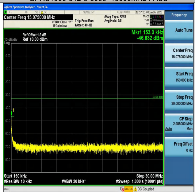
GPRS1900-661-0-0.15~30MHz-PASS
