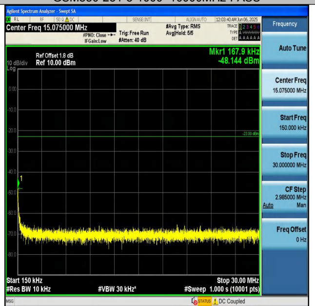
GPRS850-128-5-0.15~30MHz-PASS
