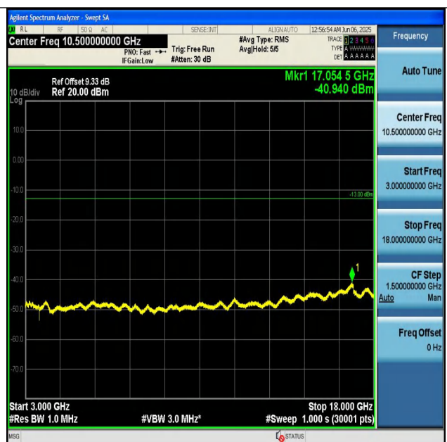
GPRS1900-512-0-3000~18000MHz-PASS
