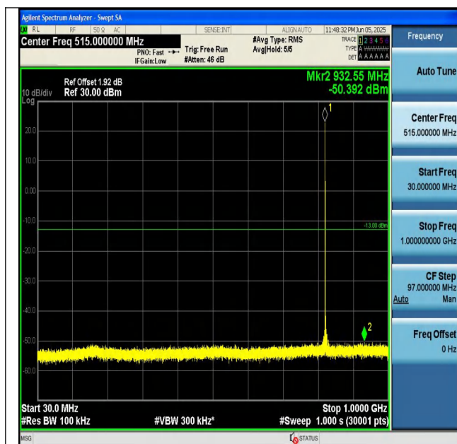
GSM850-128-5-30~1000MHz-PASS
