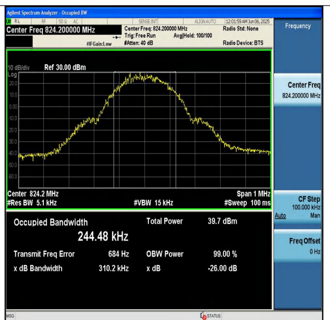
GPRS850-128-5-PASS
