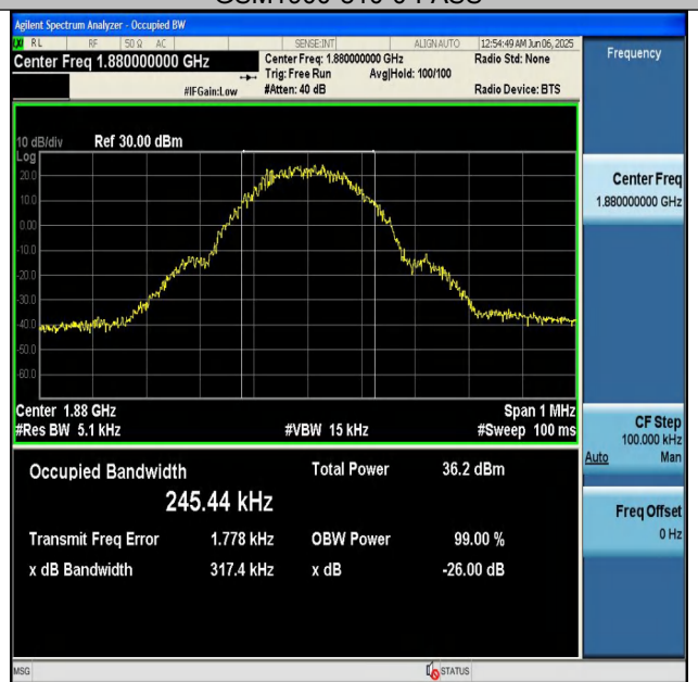
GPRS1900-661-0-PASS
