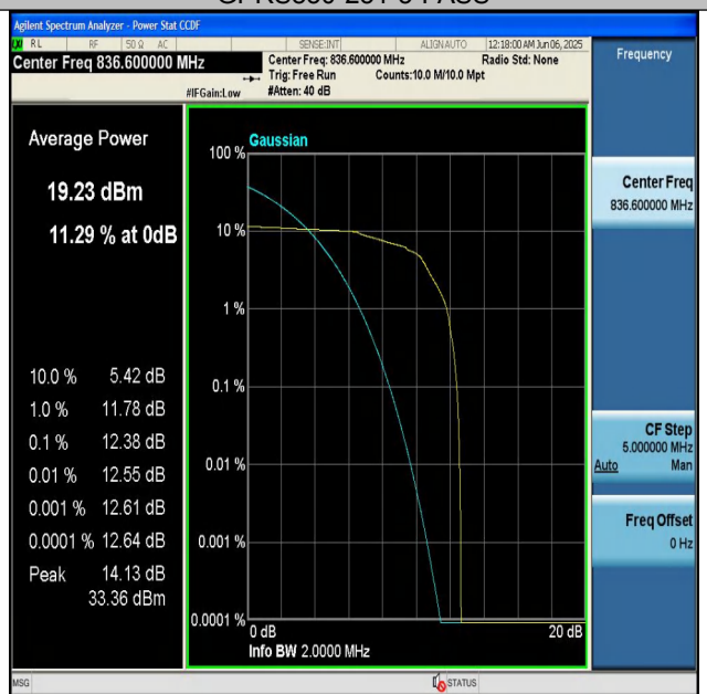
EGPRS850-190-8-PASS
