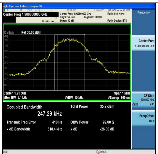
GSM1900-810-0-PASS
