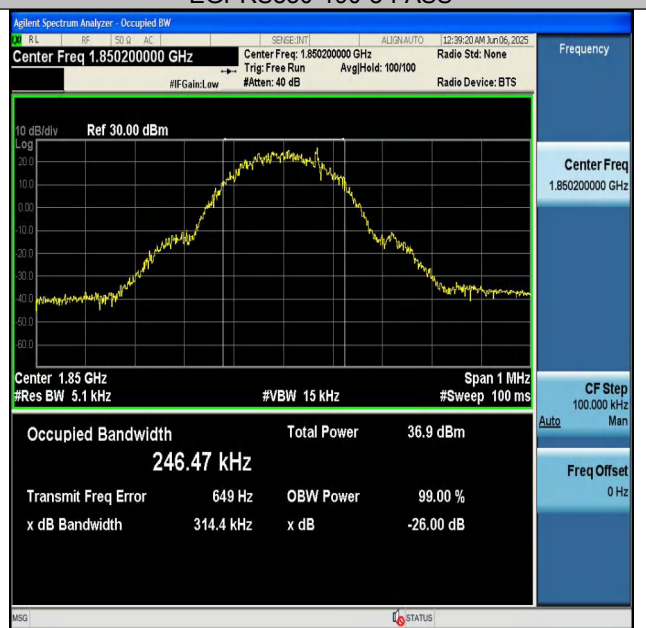
GSM1900-512-0-PASS
