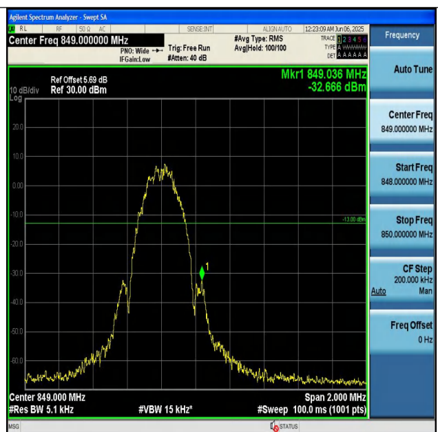
EGPRS850-251-8-PASS
