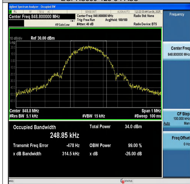
EGPRS850-251-8-PASS
