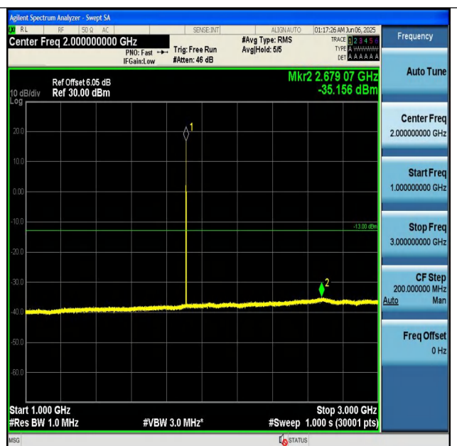
EGPRS1900-810-2-1000~3000MHz-PASS
