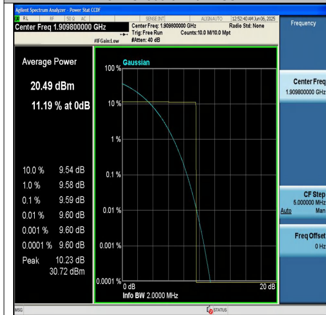
GPRS1900-810-0-PASS
