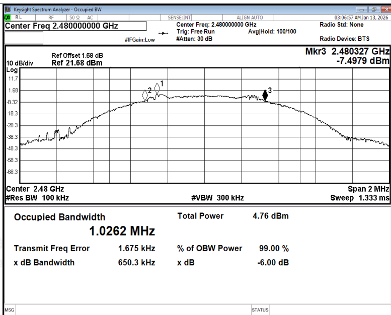
-6dB Bandwidth NVNT BLE 1M 2480MHz Ant1
