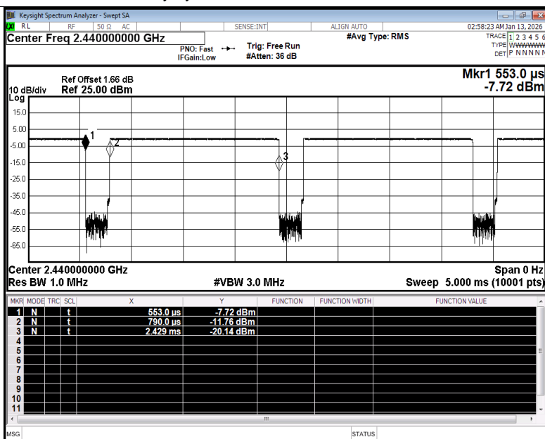
Duty Cycle NVNT BLE 1M 2440MHz Ant1
