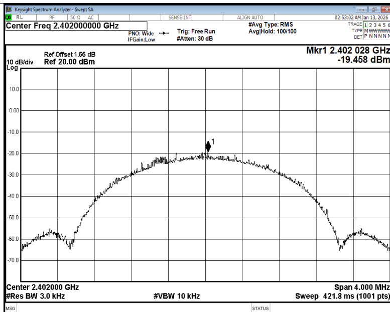
PSD NVNT BLE 2M 2402MHz Ant1
