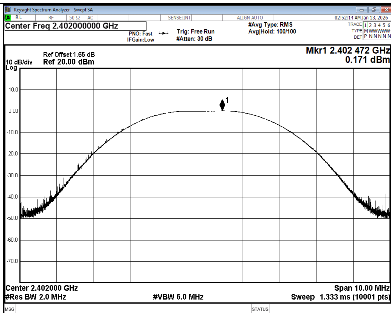
Peak Power NVNT BLE 2M 2402MHz Ant1
