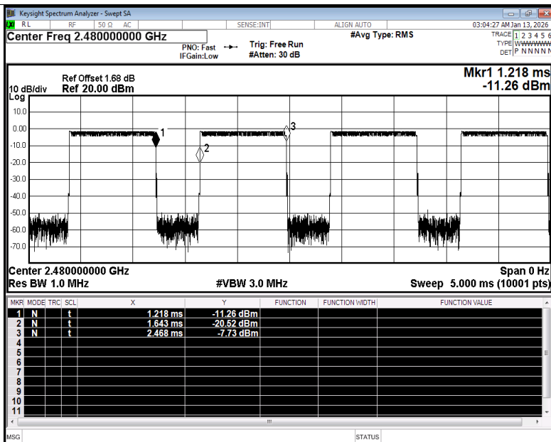
Duty Cycle NVNT BLE 2M 2480MHz Ant1
