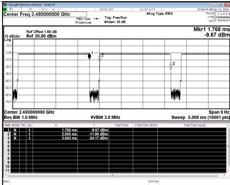
Duty Cycle NVNT BLE 1M 2480MHz Ant1
