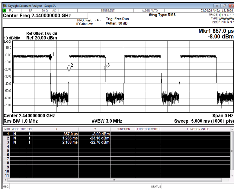
Duty Cycle NVNT BLE 2M 2440MHz Ant1
