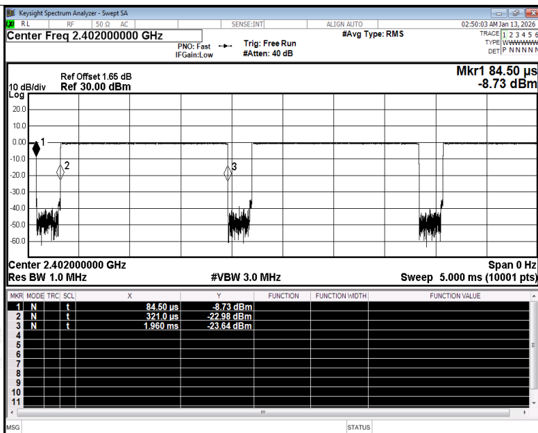
Duty Cycle NVNT BLE 1M 2402MHz Ant1
