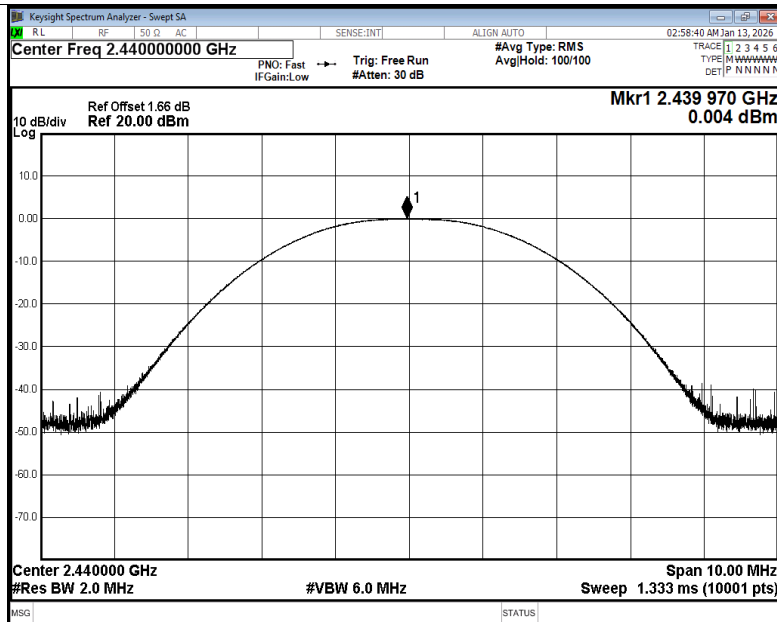
Peak Power NVNT BLE 1M 2440MHz Ant1
