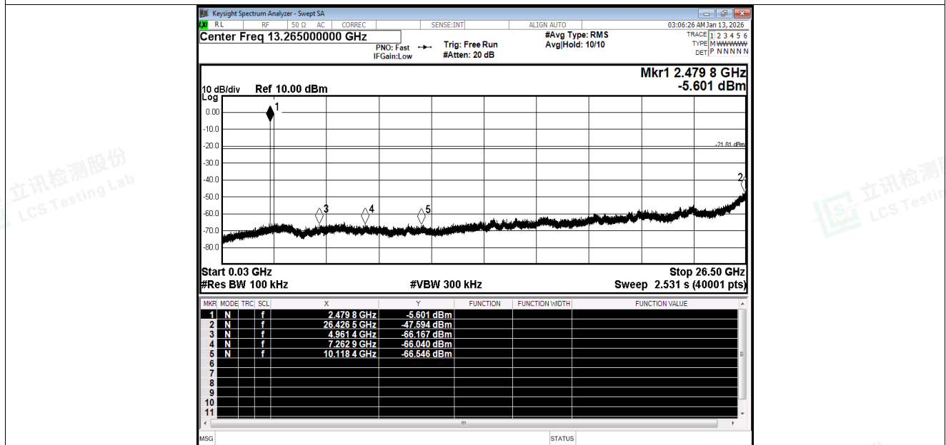
Tx. Spurious NVNT BLE 2M 2480MHz Ant1 Emission
