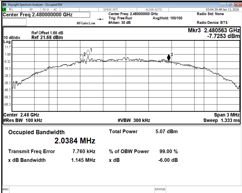
-6dB Bandwidth NVNT BLE 2M 2480MHz Ant1
