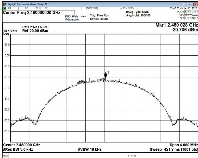
PSD NVNT BLE 2M 2480MHz Ant1
