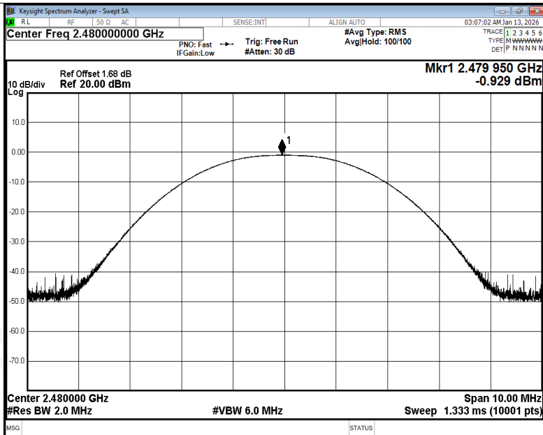
Peak Power NVNT BLE 1M 2480MHz Ant1
