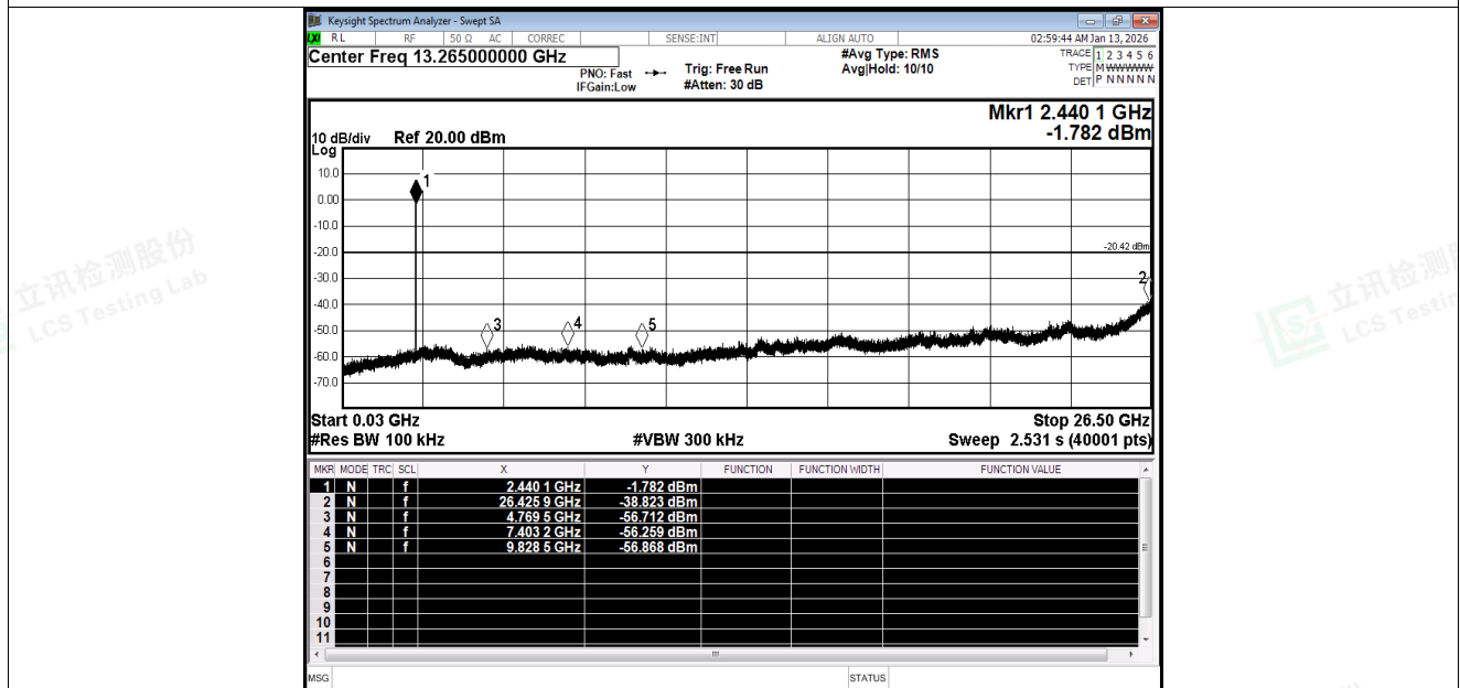
Tx. Spurious NVNT BLE 1M 2440MHz Ant1 Emission
