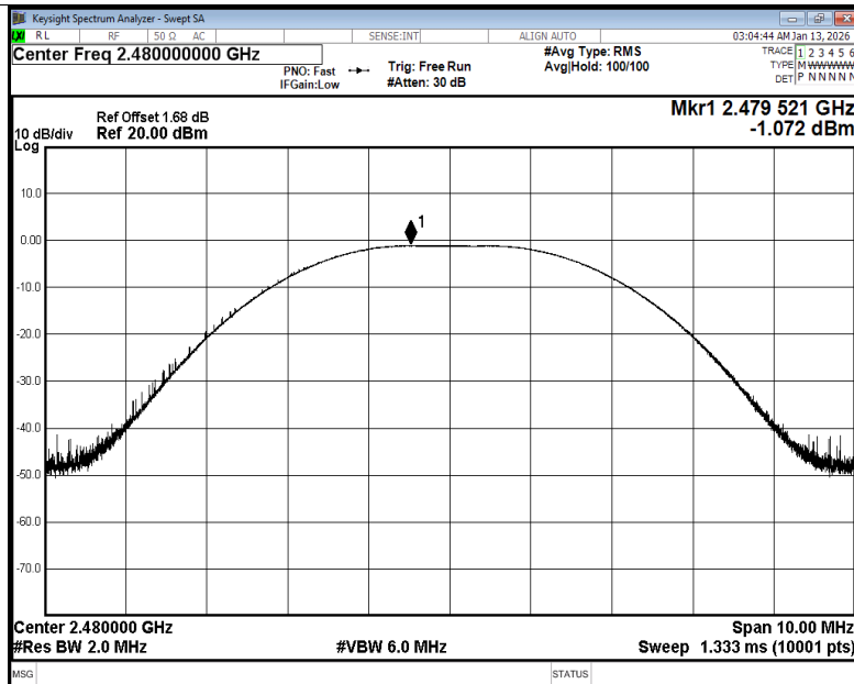
Peak Power NVNT BLE 2M 2480MHz Ant1
