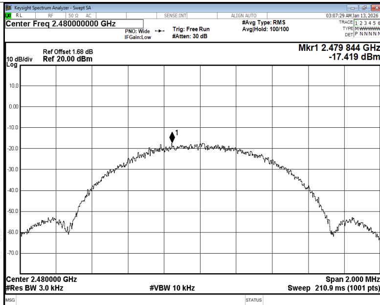
PSD NVNT BLE 1M 2480MHz Ant1
