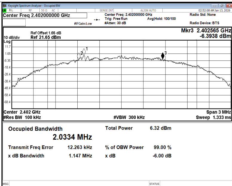
-6dB Bandwidth NVNT BLE 2M 2402MHz Ant1
