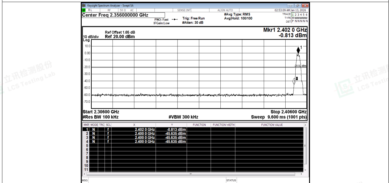
Band Edge NVNT BLE 2M 2402MHz Ant1 Emission
