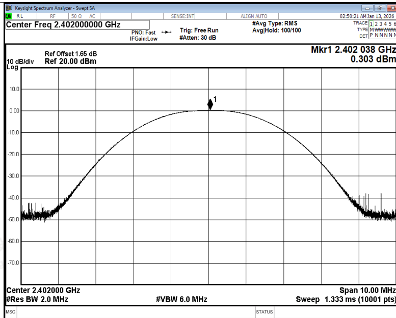
Peak Power NVNT BLE 1M 2402MHz Ant1
