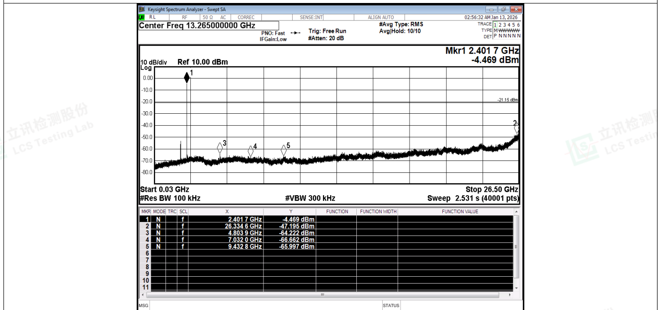
Tx. Spurious NVNT BLE 2M 2402MHz Ant1 Emission
