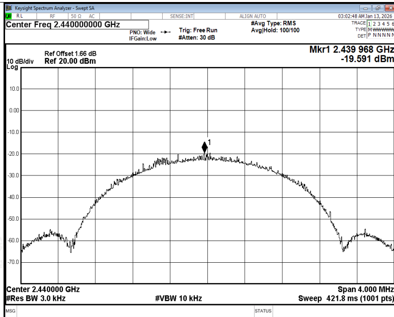
PSD NVNT BLE 2M 2440MHz Ant1
