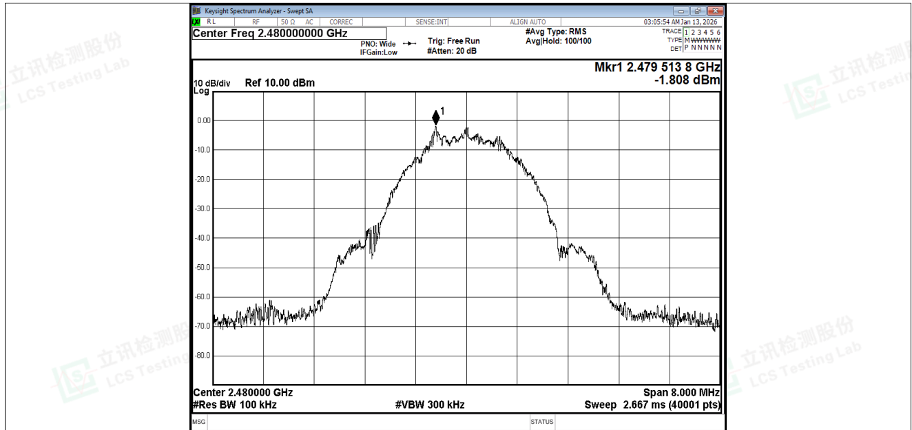
Tx. Spurious NVNT BLE 2M 2480MHz Ant1 Ref
