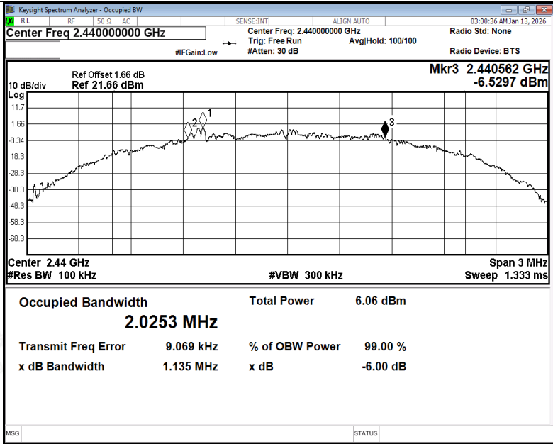
-6dB Bandwidth NVNT BLE 2M 2440MHz Ant1
