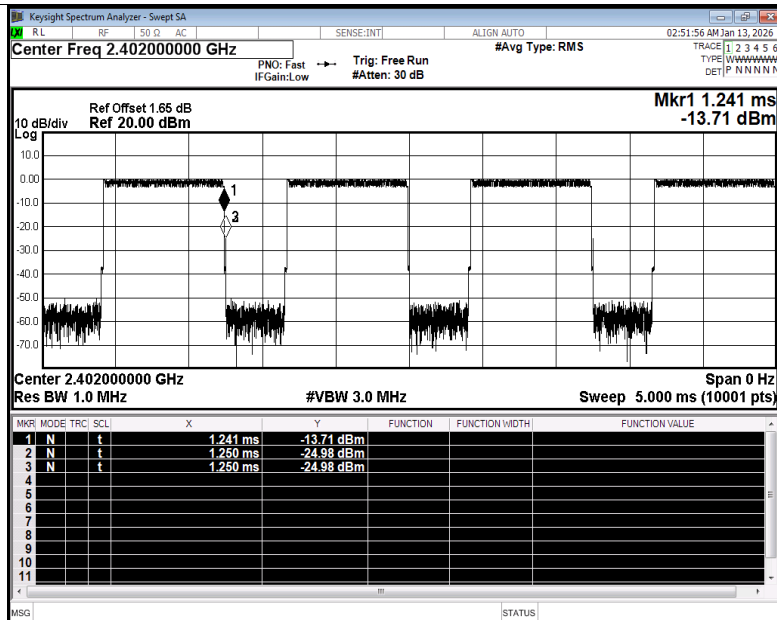
Duty Cycle NVNT BLE 2M 2402MHz Ant1
