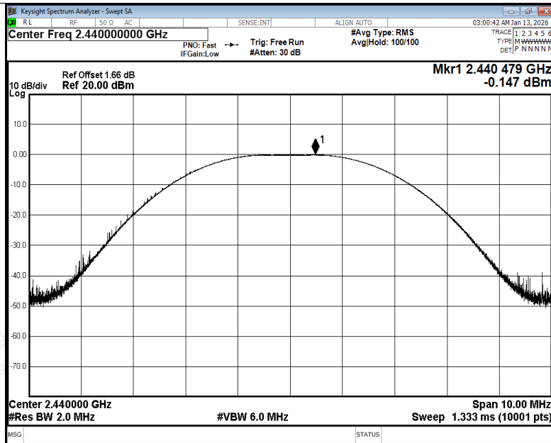
Peak Power NVNT BLE 2M 2440MHz Ant1
