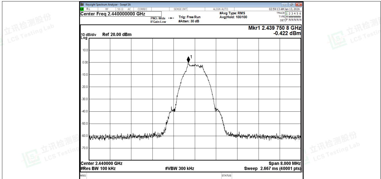
Tx. Spurious NVNT BLE 1M 2440MHz Ant1 Ref
