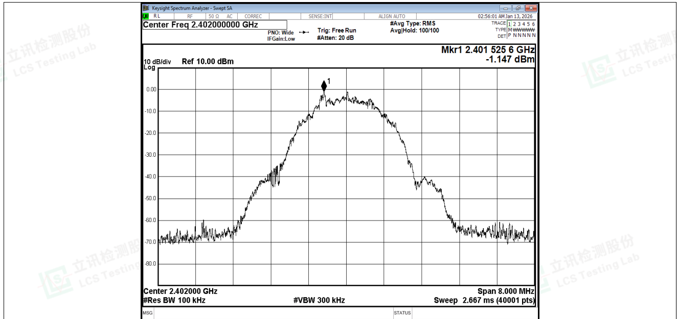
Tx. Spurious NVNT BLE 2M 2402MHz Ant1 Ref
