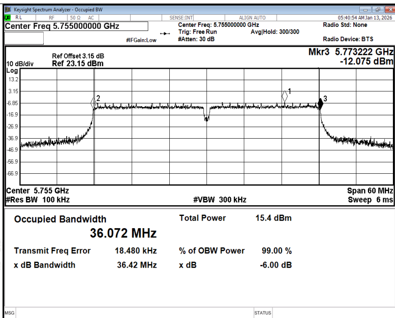
-6dB Bandwidth NVNT n40 5755MHz Ant1
