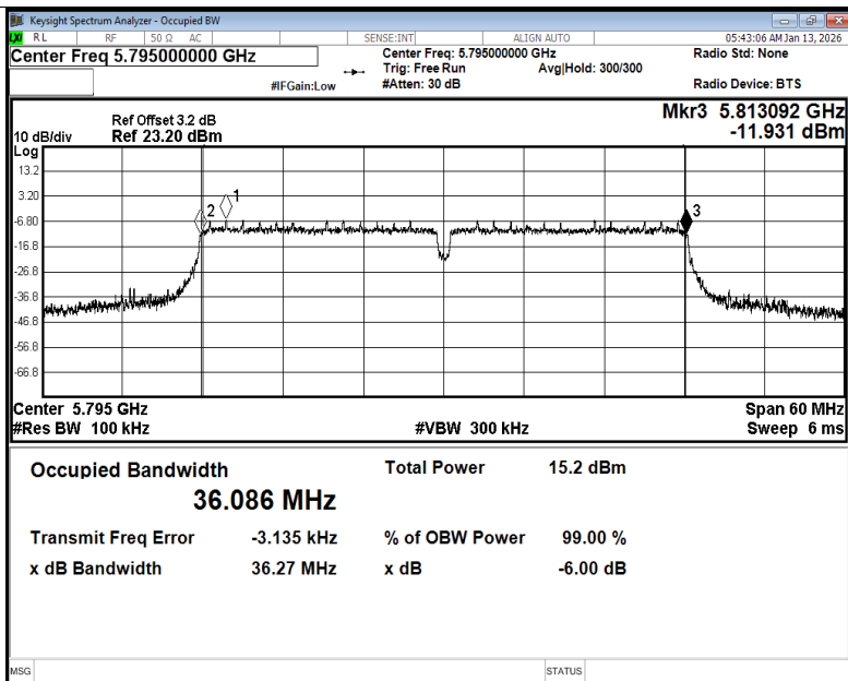
-6dB Bandwidth NVNT n40 5795MHz Ant1
