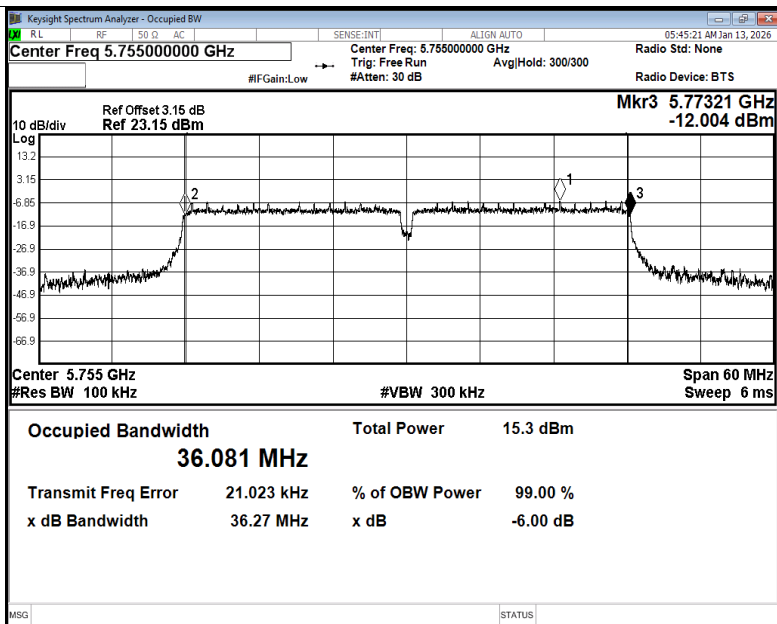
-6dB Bandwidth NVNT ac40 5755MHz Ant1
