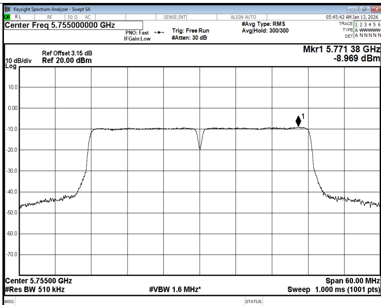
PSD NVNT ac40 5755MHz Ant1
