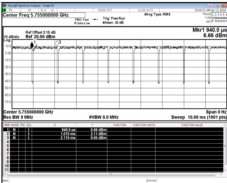
Duty Cycle NVNT n40 5755MHz Ant1
