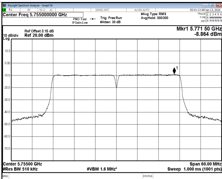
PSD NVNT n40 5755MHz Ant1
