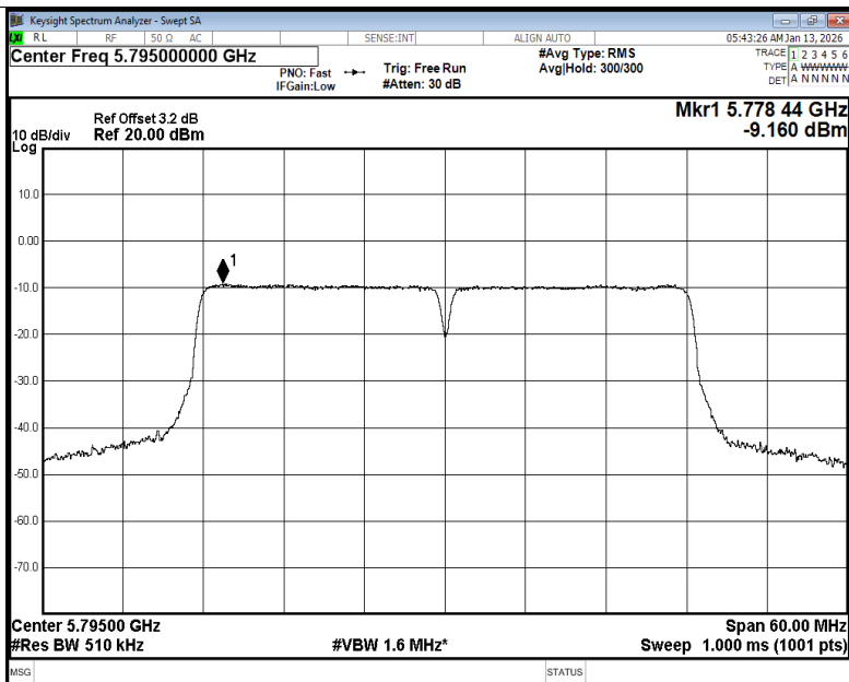
PSD NVNT n40 5795MHz Ant1
