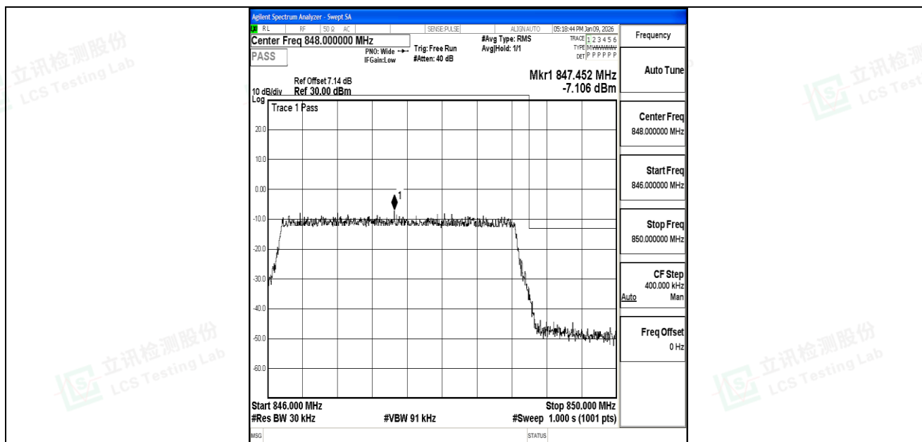
Band5_3MHz_16QAM_20635_15RB#0
