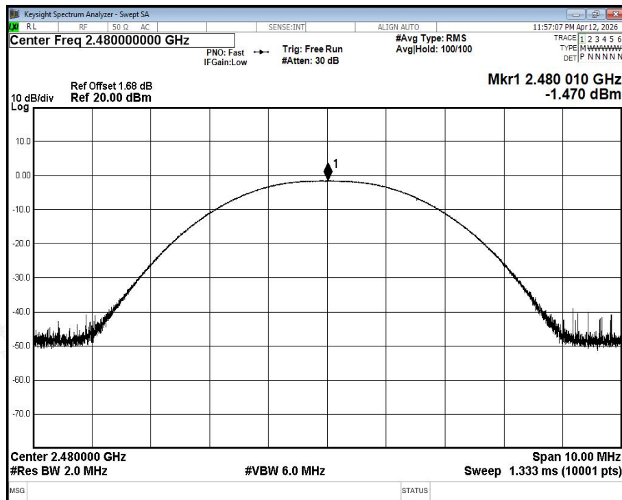
Peak Power NVNT BLE 1M 2480MHz Ant1
