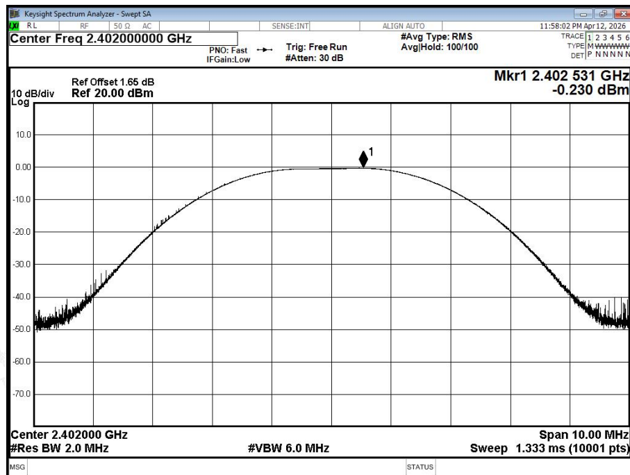
Peak Power NVNT BLE 2M 2402MHz Ant1
