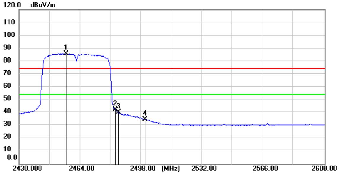
11n(HT40)_TX_CH_09_Horizontal_Average
