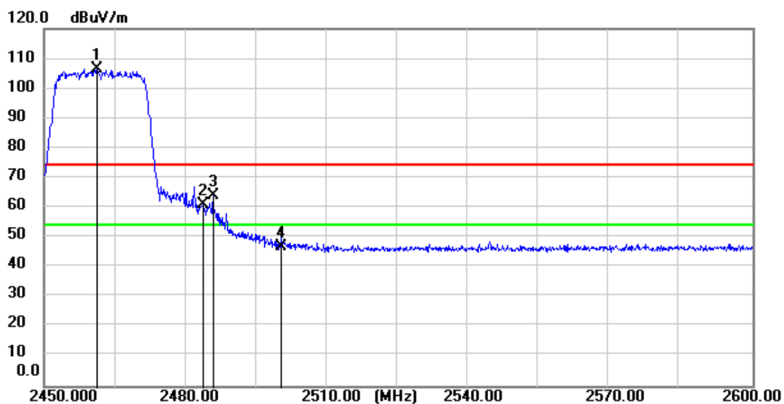
11(HE20)_TX_CH_11_Horizontal_Peak
