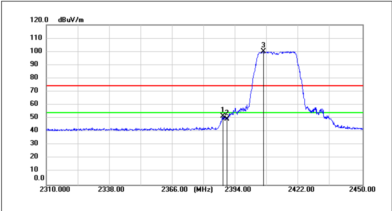
11n(HT20)_TX_CH_01_Horizontal_Peak
