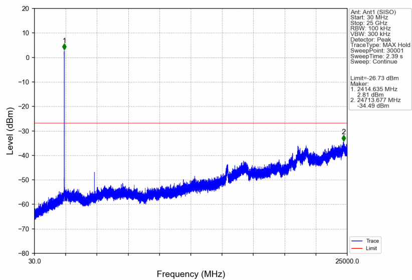
802.11b_LCH_2412MHz_Ant1 (SISO)_NTNV
