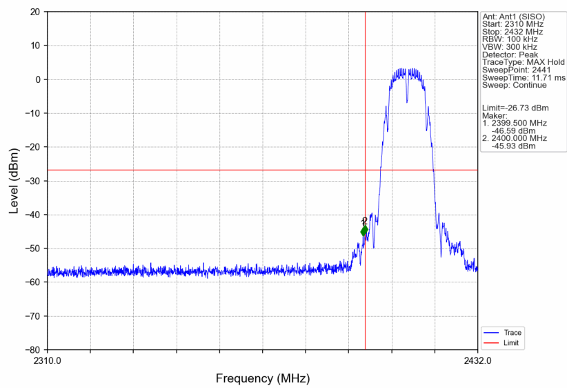
802.11b_LCH_2412MHz_Ant1 (SISO)_NTNV
