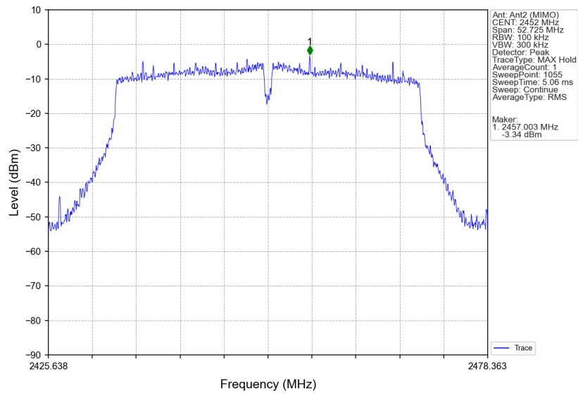
802.11n(HT40)_HCH_2452MHz_MIMO_NTNV
