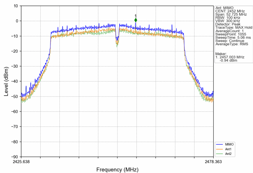
802.11n(HT40)_HCH_2452MHz_MIMO_NTNV
