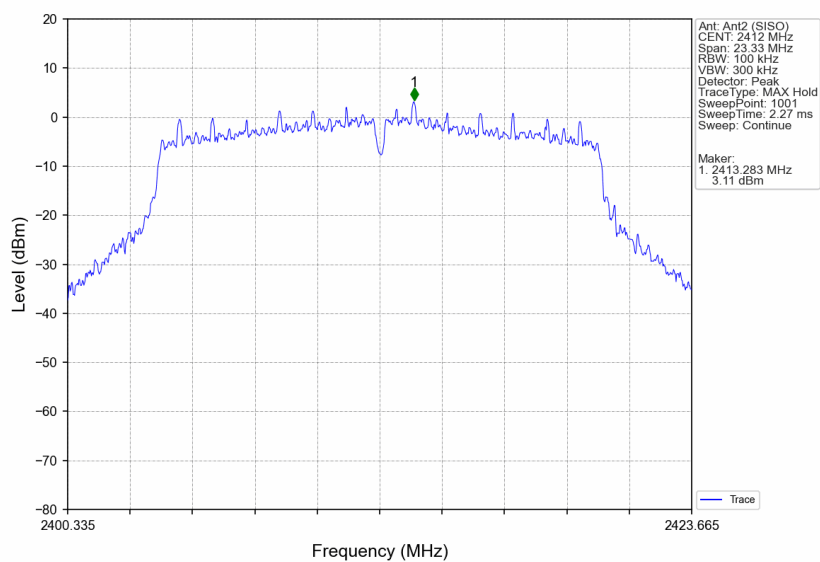
802.11g_LCH_2412MHz_Ant2 (SISO)_NTNV
