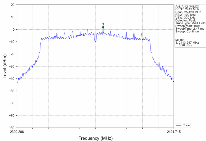
802.11n(HT20)_LCH_2412MHz_Ant2 (MIMO)_NTNV
