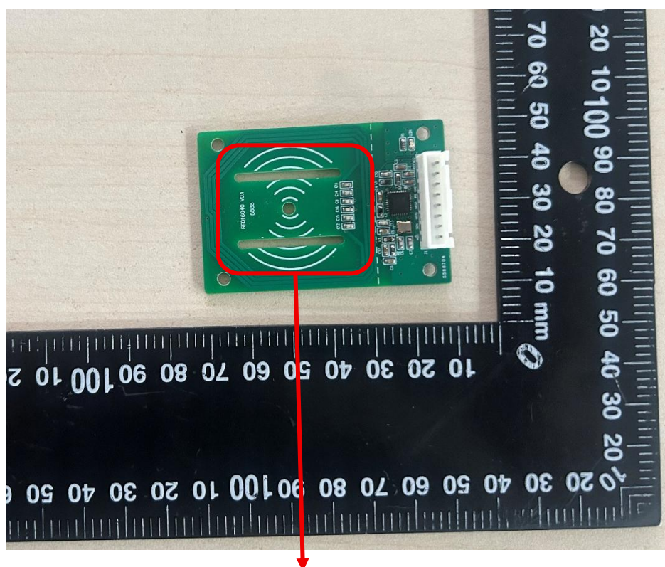
Antenna
