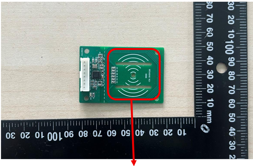
Antenna
