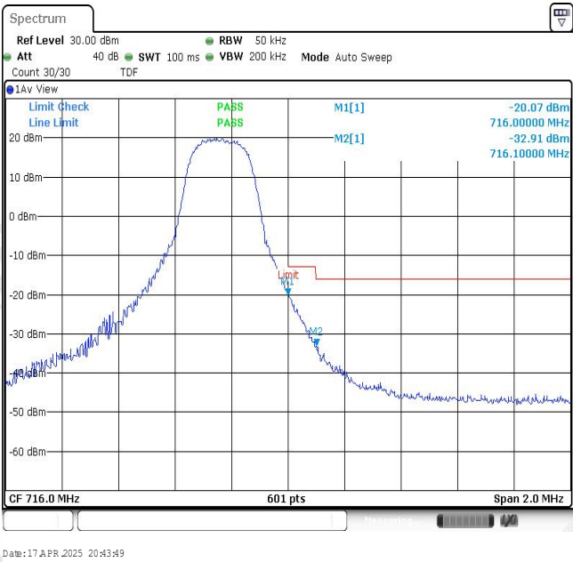
Band12-3MHz-QPSK-23165-1RB#14
