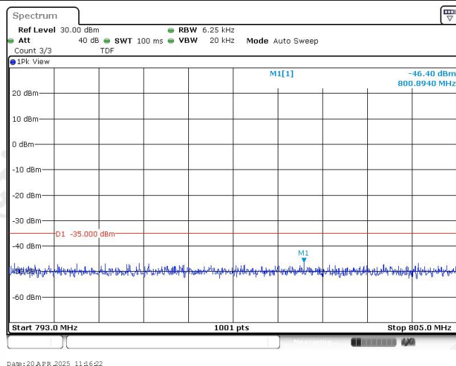
Band13-10MHz-QPSK-23230-1RB#0-Range2:793~805MHz
