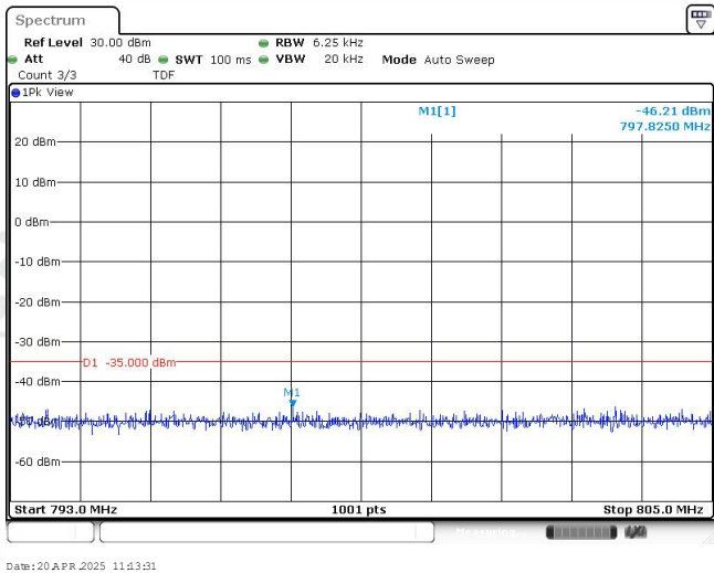
Band13-5MHz-QPSK-23205-1RB#0-Range2:793~805MHz
