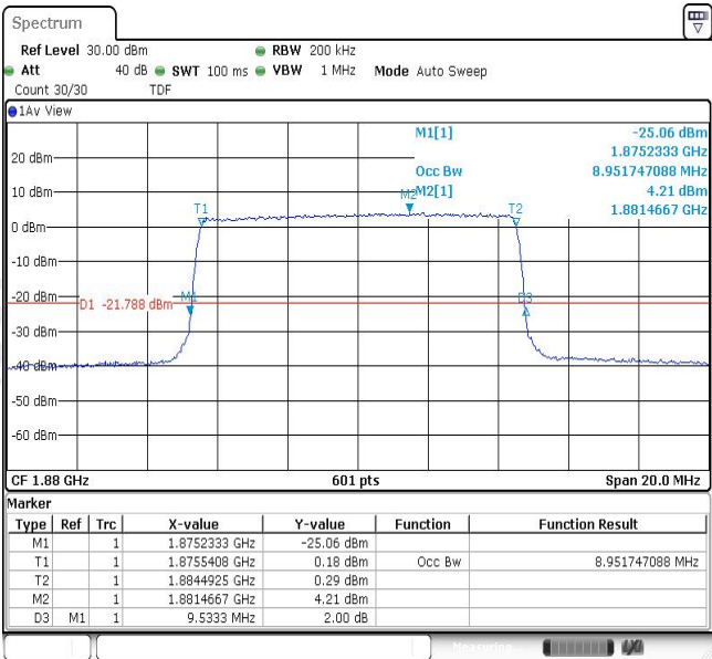
Band2-10MHz-16QAM-18900-50RB#0-8.952
