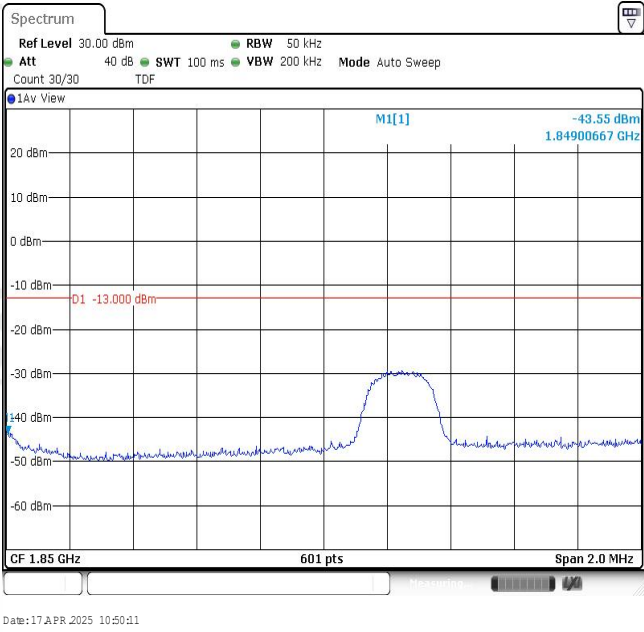
Band2-3MHz-QPSK-18615-1RB#14
