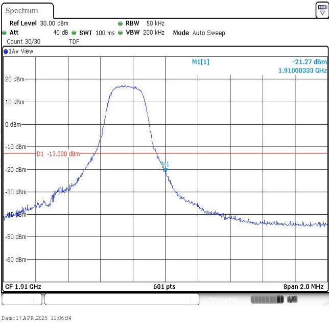
Band2-3MHz-QPSK-19185-1RB#14
