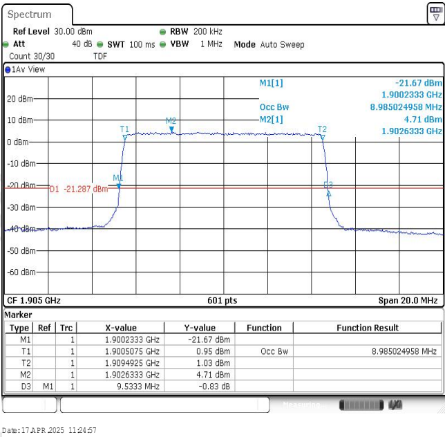
Band2-10MHz-QPSK-19150-50RB#0-8.985
