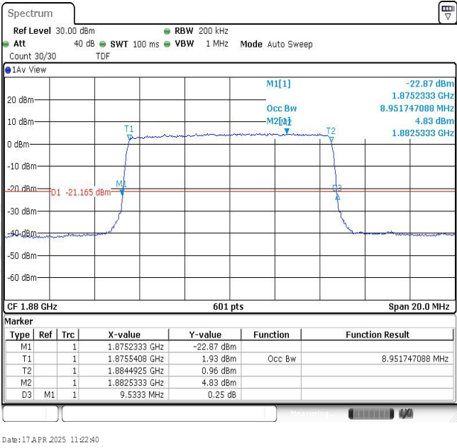
Band2-10MHz-QPSK-18900-50RB#0-8.952
