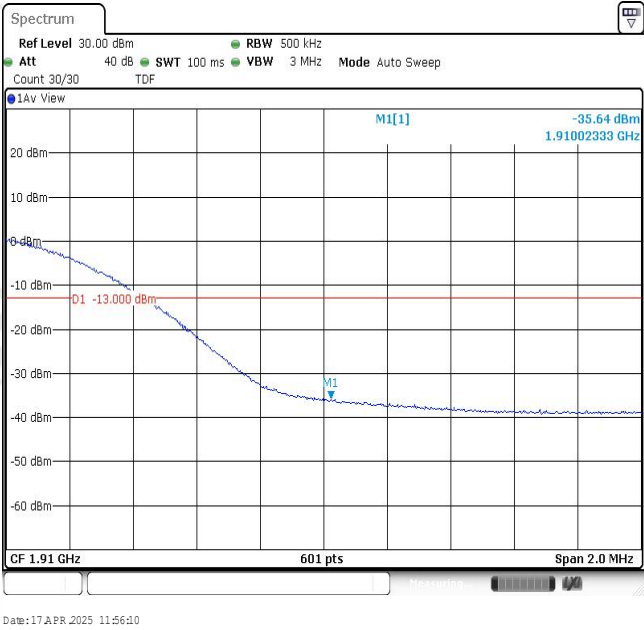
Band2-20MHz-QPSK-19100-100RB#0
