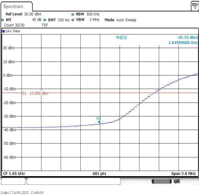
Band2-20MHz-QPSK-18700-100RB#0
