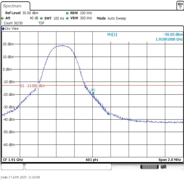
Band2-5MHz-QPSK-19175-1RB#24
