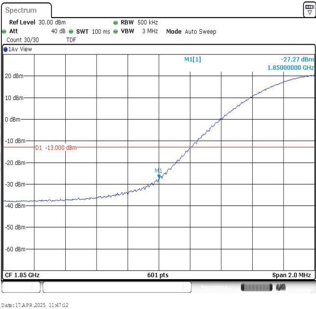
Band2-20MHz-QPSK-18700-1RB#0
