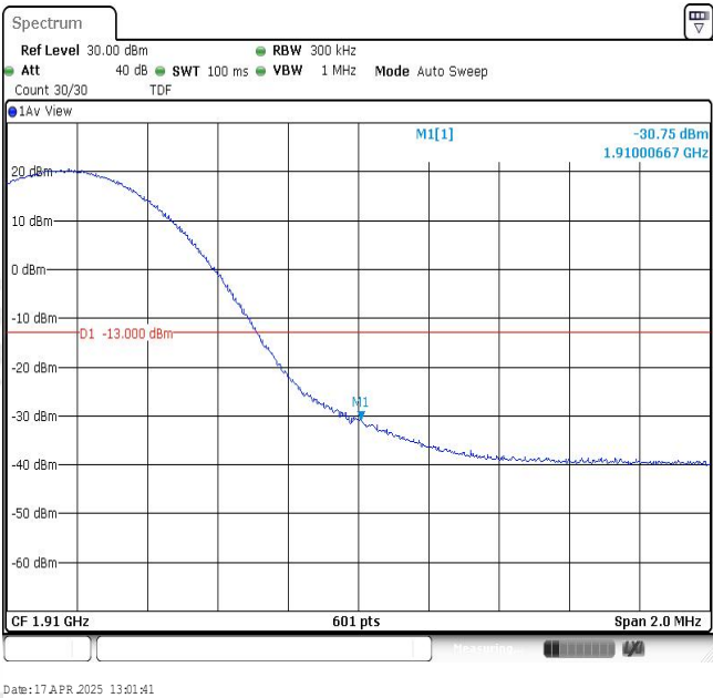
Band2-15MHz-16QAM-19125-1RB#74
