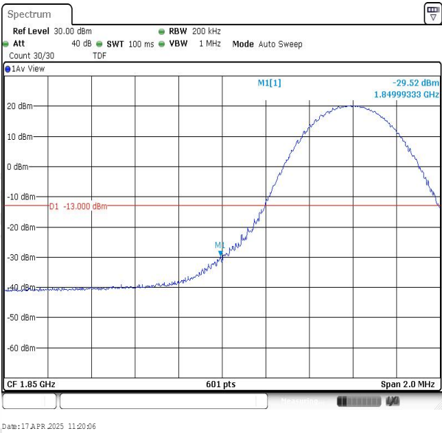
Band2-10MHz-QPSK-18650-1RB#0
