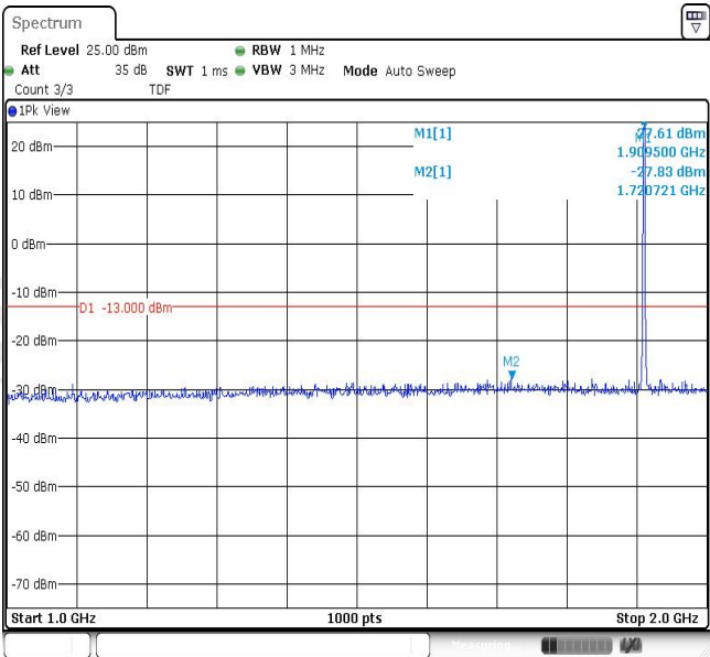
Band2-1.4MHz-QPSK-19193-1RB#0-Range2:1000~2000MHz
