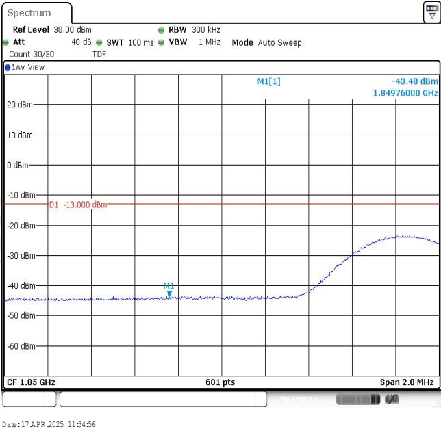
Band2-15MHz-QPSK-18675-1RB#74
