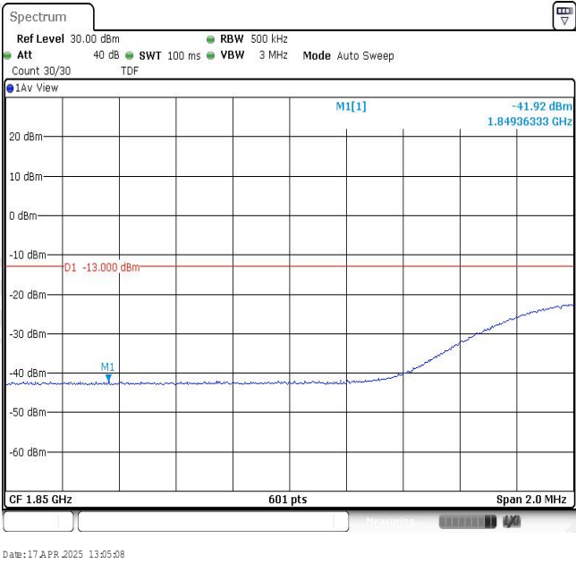
Band2-20MHz-16QAM-18700-1RB#99
