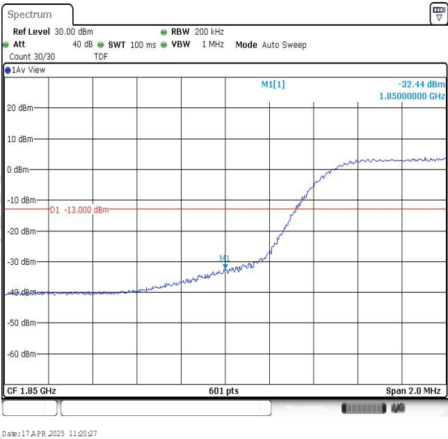
Band2-10MHz-QPSK-18650-50RB#0
