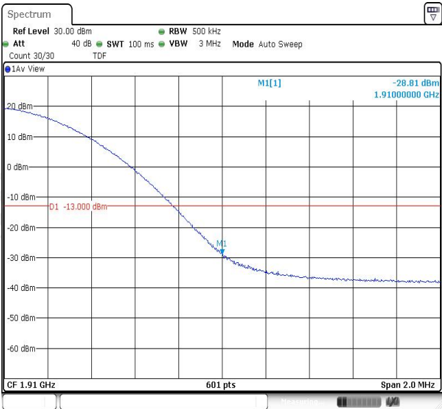
Band2-20MHz-16QAM-19100-1RB#99
