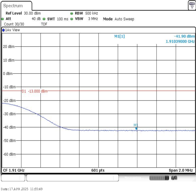
Band2-20MHz-QPSK-19100-1RB#0
