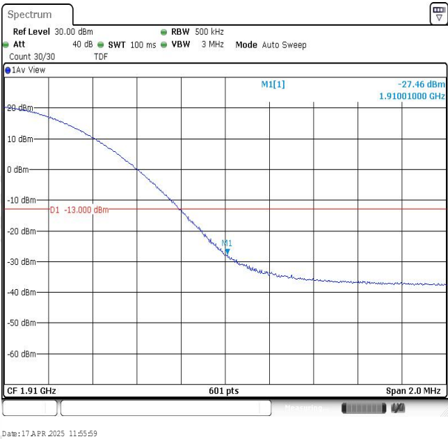
Band2-20MHz-QPSK-19100-1RB#99
