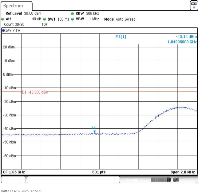
Band2-15MHz-16QAM-18675-1RB#74
