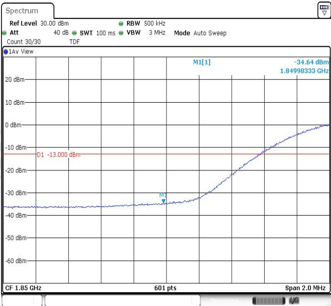
Band2-20MHz-16QAM-18700-100RB#0
