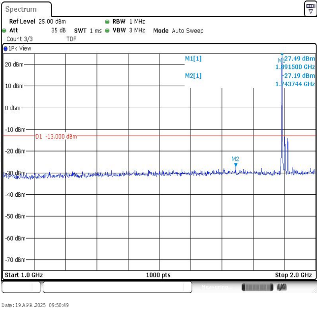
Band2-20MHz-16QAM-19100-1RB#0-Range2:1000~2000MHz
