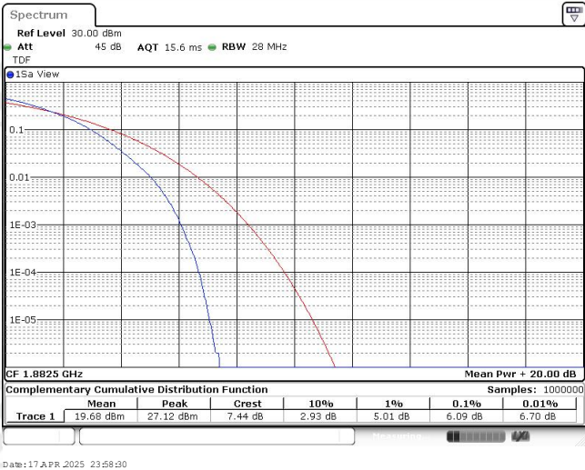
Band25-20MHz-16QAM-26365-100RB#0
