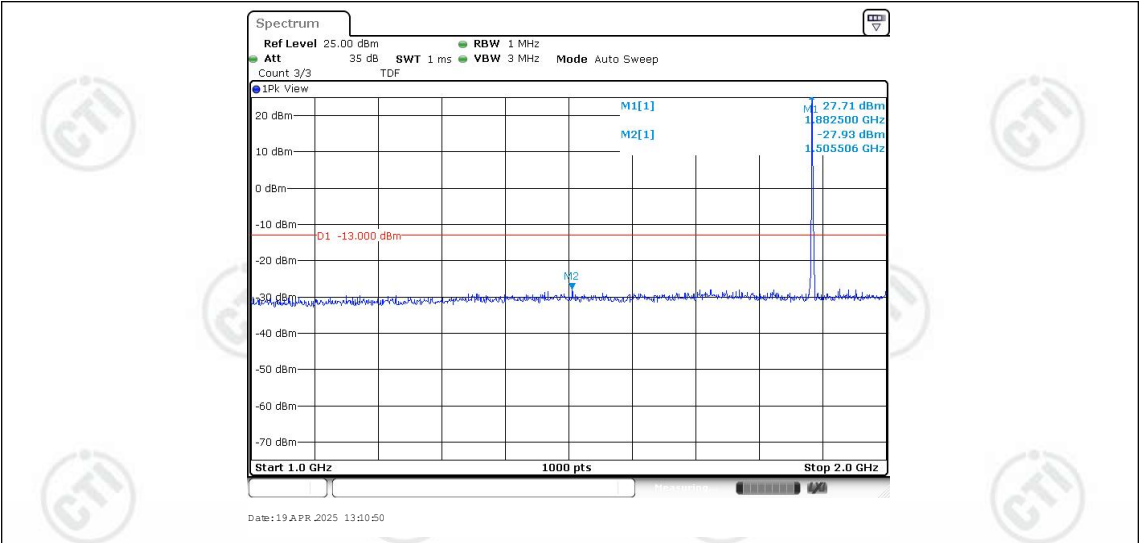
Band25-1.4MHz-QPSK-26365-1RB#0-Range2:1000~2000MHz
