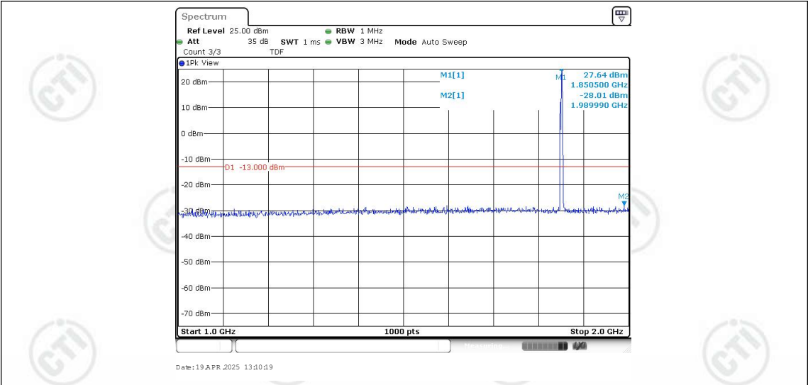
Band25-1.4MHz-QPSK-26047-1RB#0-Range2:1000~2000MHz
