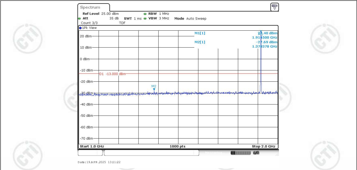
Band25-1.4MHz-QPSK-26683-1RB#0-Range2:1000~2000MHz
