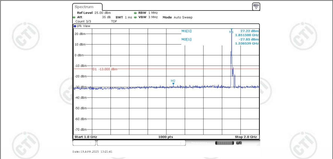
Band25-10MHz-QPSK-26090-1RB#0-Range2:1000~2000MHz
