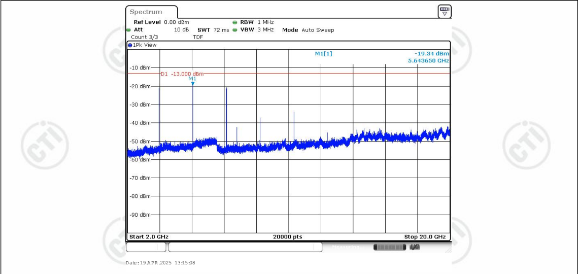
Band25-3MHz-QPSK-26365-1RB#0-Range3:2000~20000MHz
