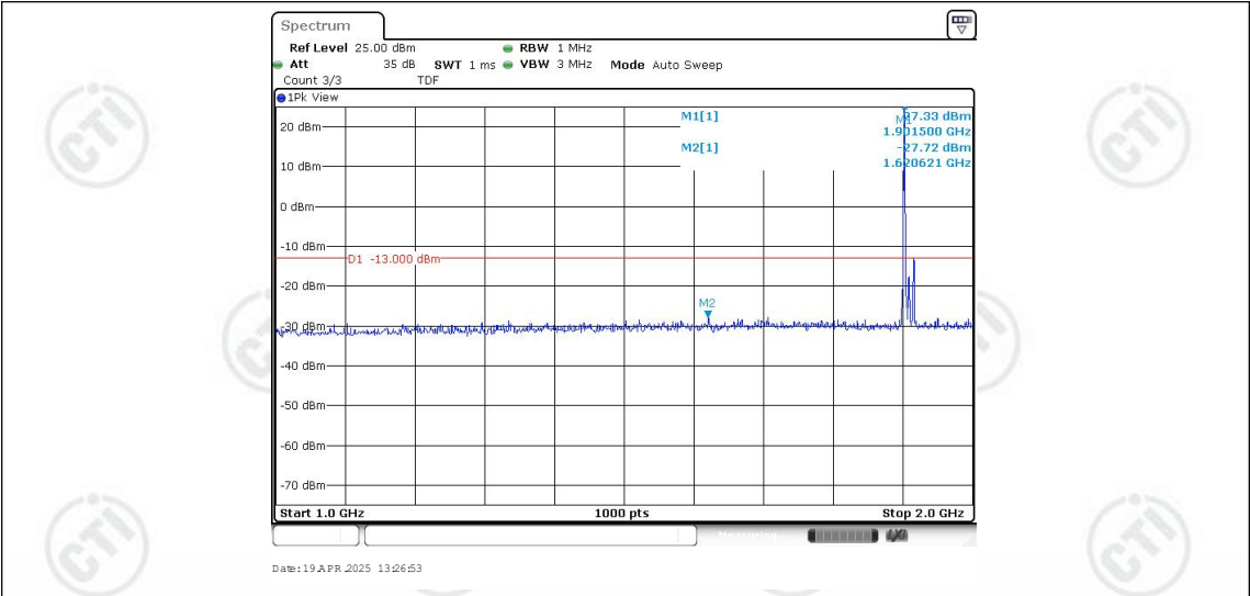
Band25-15MHz-QPSK-26615-1RB#0-Range2:1000~2000MHz
