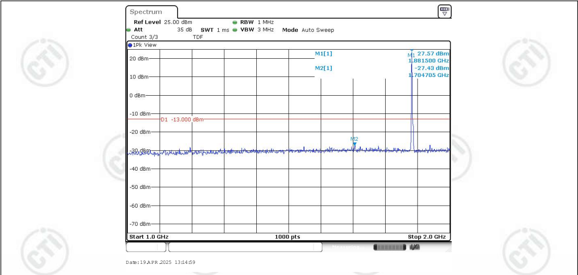
Band25-3MHz-QPSK-26365-1RB#0-Range2:1000~2000MHz
