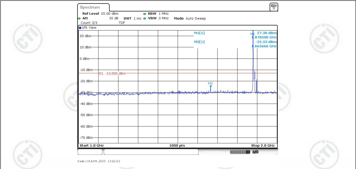
Band25-10MHz-QPSK-26365-1RB#0-Range2:1000~2000MHz
