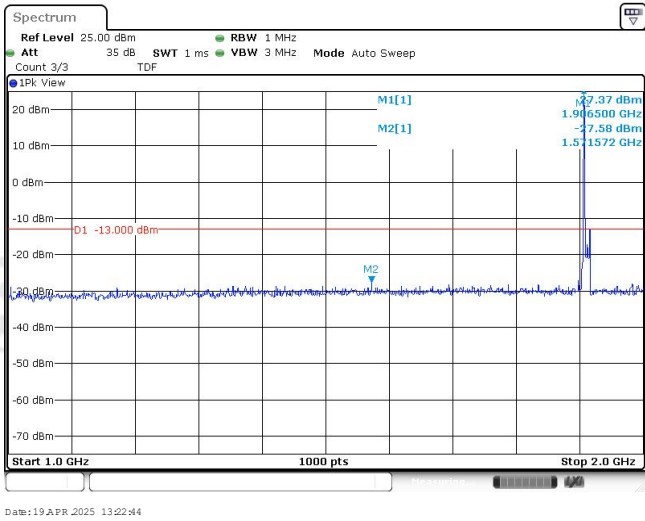
Band25-10MHz-QPSK-26640-1RB#0-Range2:1000~2000MHz
