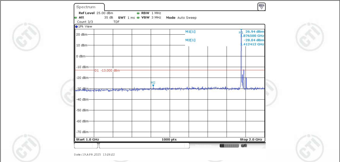
Band25-15MHz-QPSK-26365-1RB#0-Range2:1000~2000MHz
