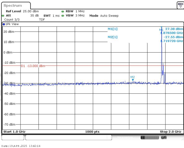
Band25-10MHz-16QAM-26365-1RB#0-Range2:1000~2000MHz
