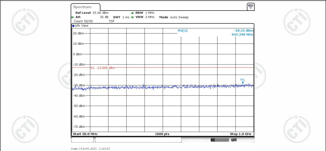
Band25-10MHz-QPSK-26365-1RB#0-Range1:30~1000MHz
