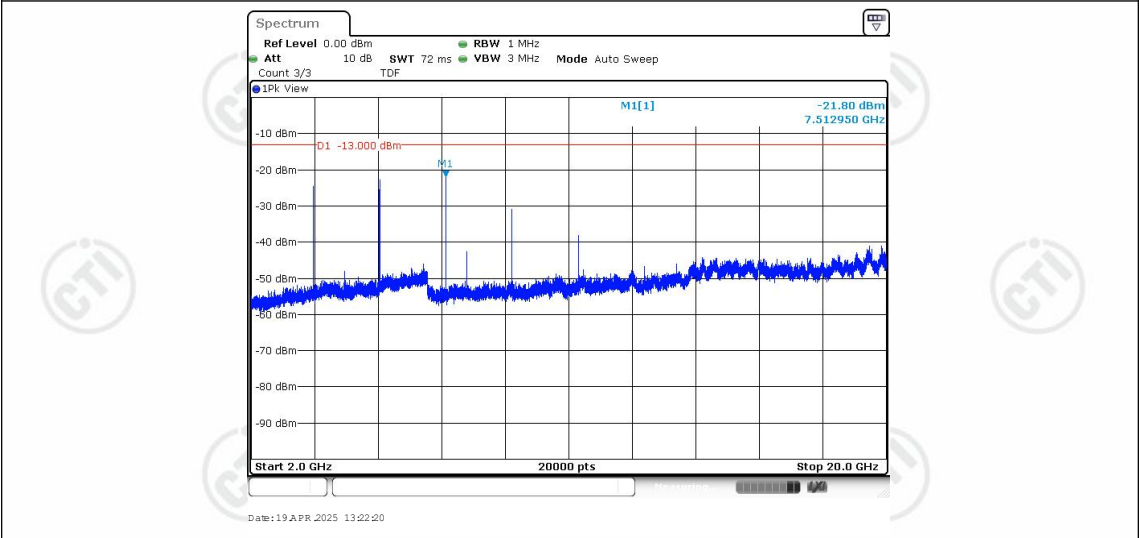
Band25-10MHz-QPSK-26365-1RB#0-Range3:2000~20000MHz
