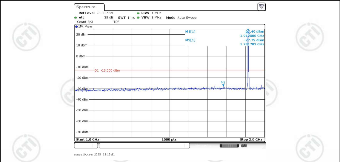
Band25-3MHz-QPSK-26675-1RB#0-Range2:1000~2000MHz
